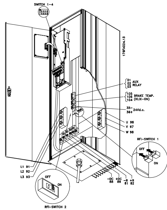
紧凑型 IP 54 VLT 6042-6062, 200-240 V
