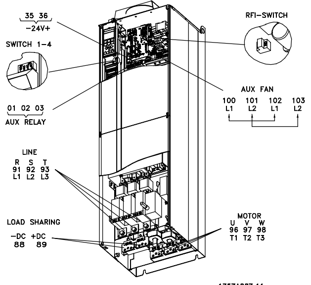
带有断路器和保险丝的 IP 00 VLT 6152-6352, 380-460 V
