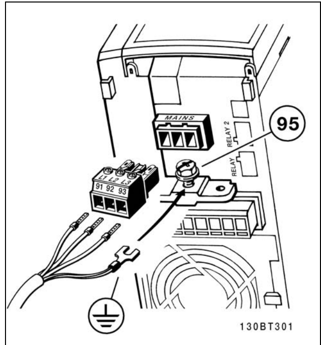
Подключение к питающей сети и заземлению (корпуса A2 и A3).
