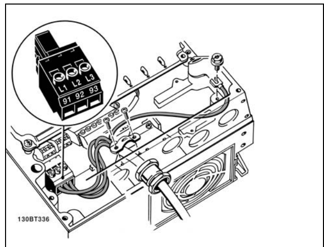
Подключение к питающей сети и заземлению (корпус A5).
