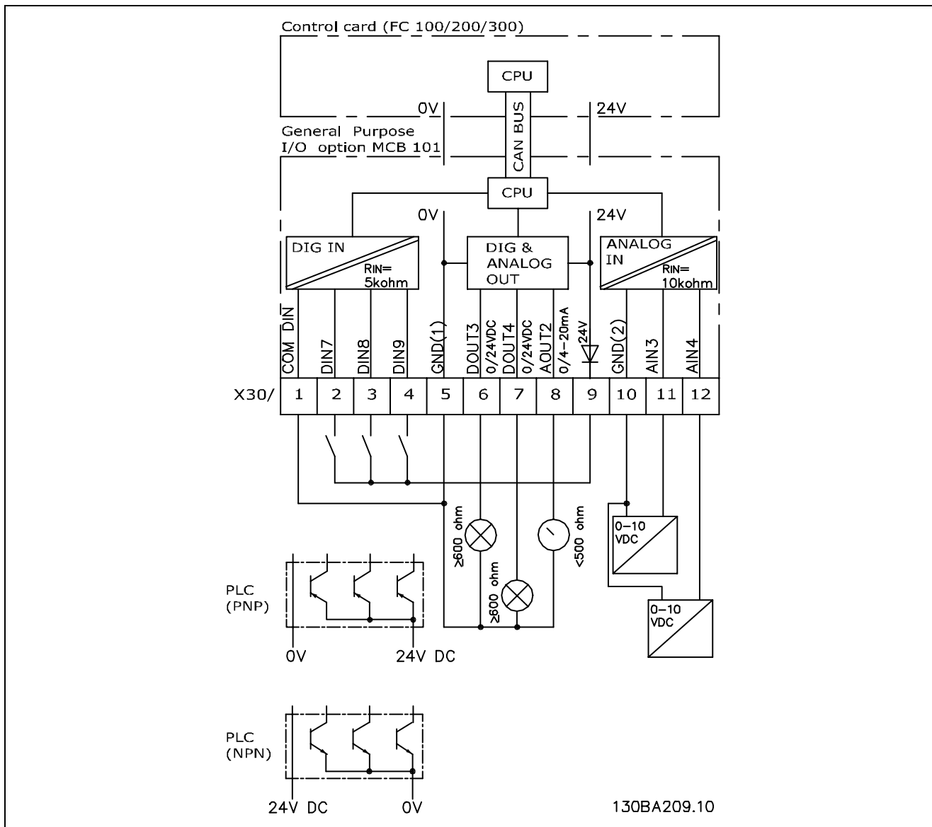
Принципиальная схема
