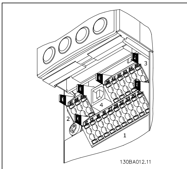
Клеммы управления (все корпуса)
