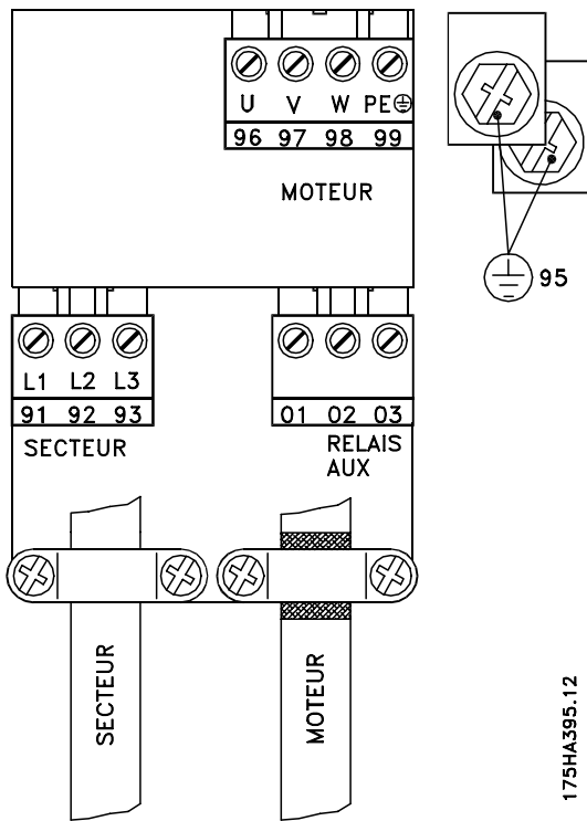
Format livre IP 20 VLT 6002-6005, 200-240 V VLT 6002-6011, 380-460 V
