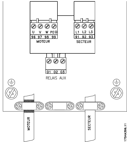
Compact IP 20, NEMA 1 et IP 54 VLT 6002-6005, 200-240 V VLT 6002-6011, 380-460 V VLT 6002-6011, 525-600 V
