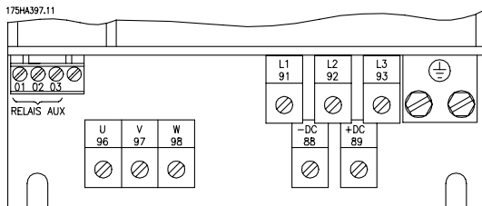
Format livre IP 20 VLT 6002-6005, 200-240 V VLT 6002-6011, 380-460 V
