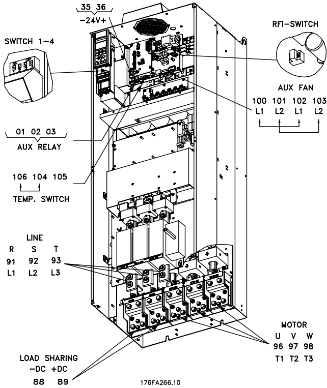
Position des bornes de terre, IP00
