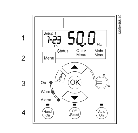
图 4.1: 带有电位计的 LCP 12
