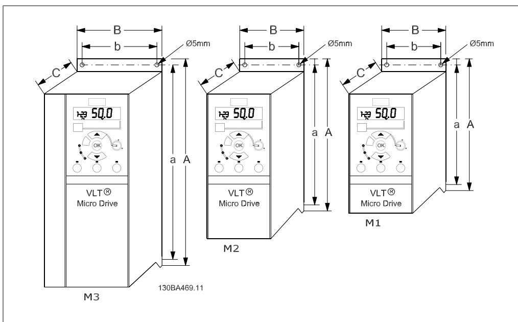
图 2.3: 机械尺寸。
