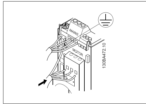
图 3.4: 安装接地电缆和电动机电线。
