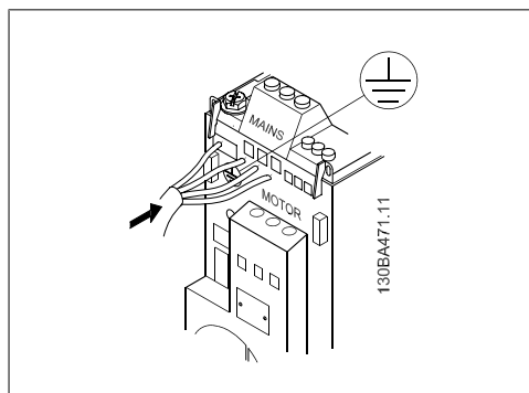
图 3.1: 安装接地电缆和主电源线。
