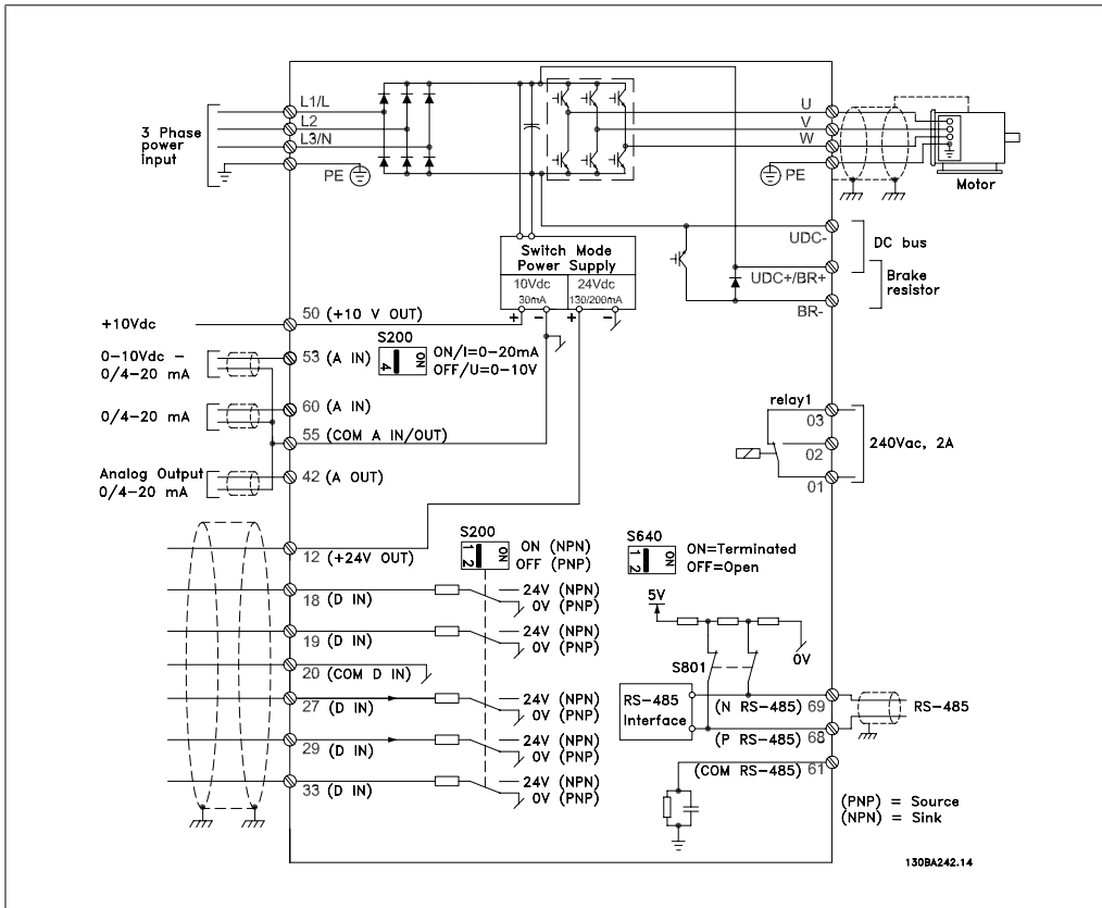
图 3.10: 图示显示了所有电气端子。
