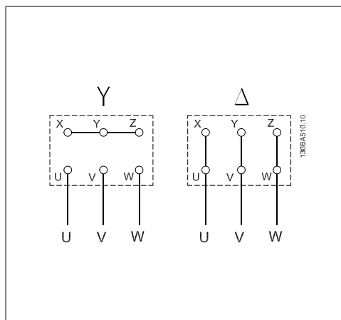
图 3.3: 星形和三角形连接。
