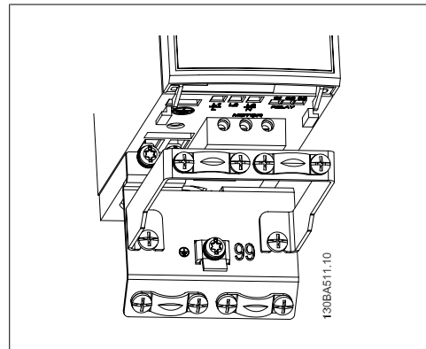
图 3.5: 带去耦板的 VLT Micro Drive
