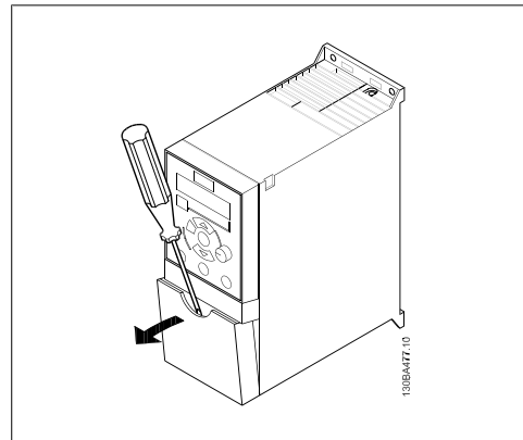
图 3.6: 取下端子盖。
