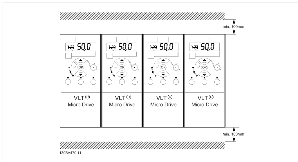
图 2.2: 并排安装。
