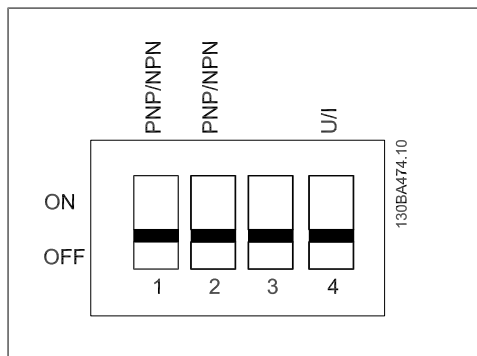
图 3.9: S200 开关 1-4
