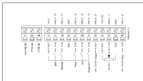
图 3.7: PNP 配置和出厂设置中的控制端子概述。
