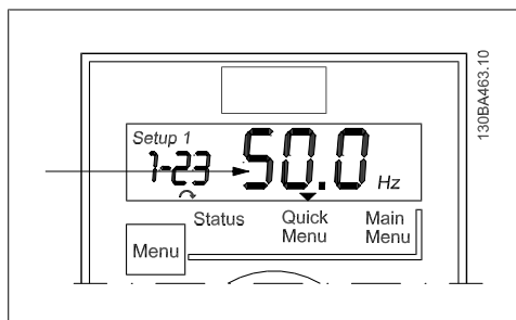
图 4.5: 指示选定参数的值
