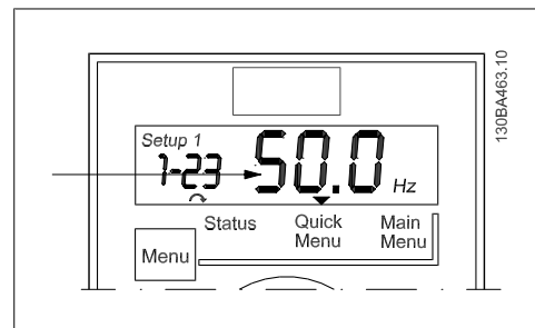
Illustration 3.5: 指示选定参数的值
