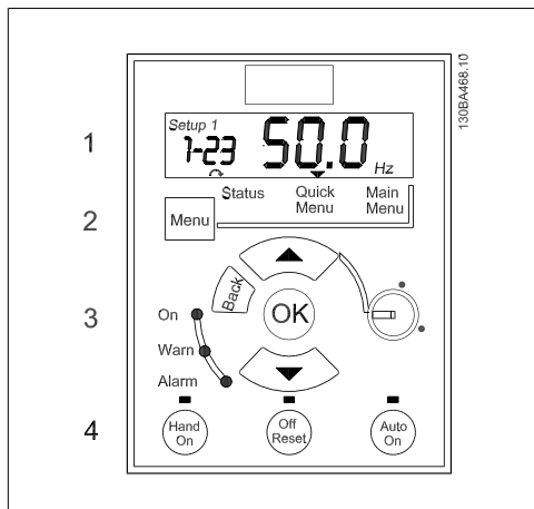
Illustration 3.1: 带有电位计的 LCP 12
