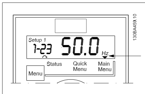
Illustration 3.10: 指示主菜单模式
