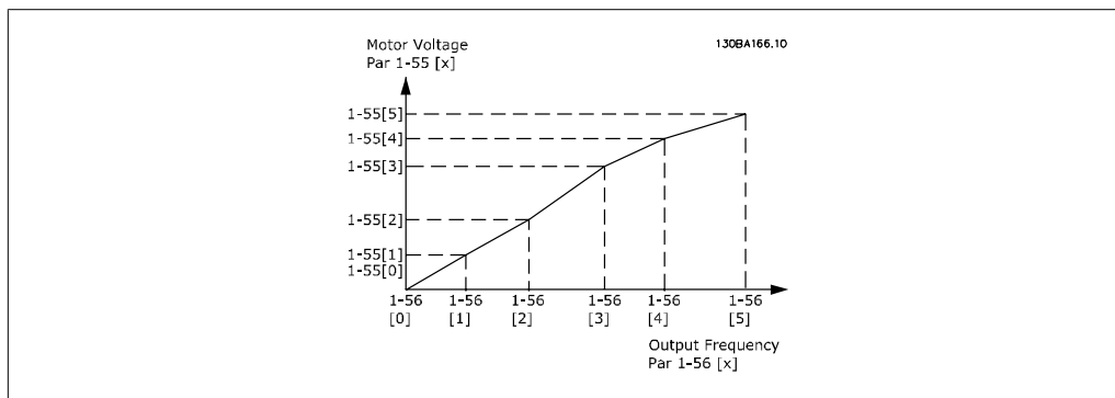
Illustration 4.1: 图 1 U/f 特性
