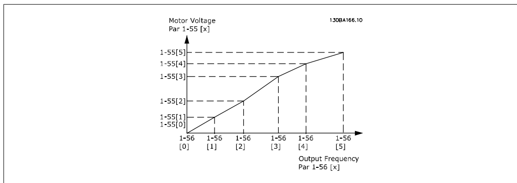
图 4.1: 图 1 U/f 特性
