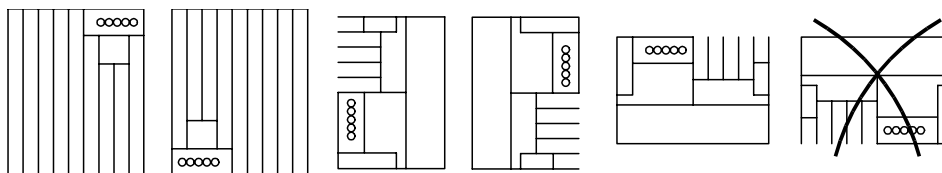
Abbildung 2.2: Zulässige Einbaupositionen
