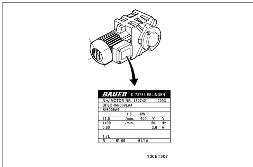
Illustration 4.31: Exemple de plaque signalétique du moteur.
