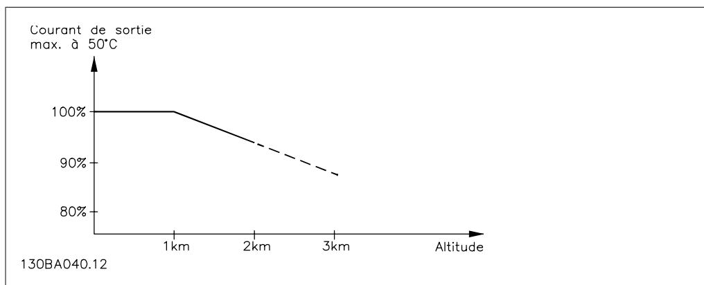
Illustration 8.9: Déclassement du courant de sortie en fonction de l'altitude à T_{AMB, MAX} . À des altitudes de plus de 2000 m, merci de contacter Danfoss Drives en ce qui concerne la norme PELV.
