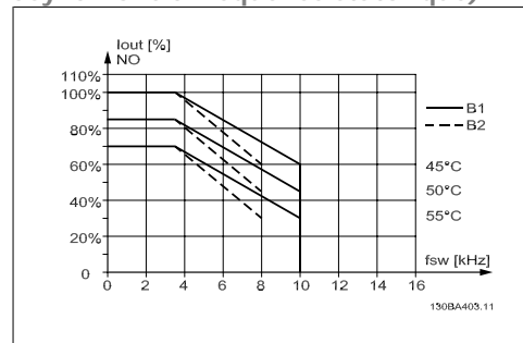
Illustration 8.6: Déclassement de I sortie pour différentes T AMB, MAX pour protection B, utilisant SFAVM en mode couple normal (surcouple de 110 %)
