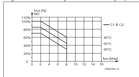
Illustration 8.8: Déclassement de I sortie pour différentes T AMB, MAX pour protection C, utilisant SFAVM en mode couple normal (surcouple de 110 %)
