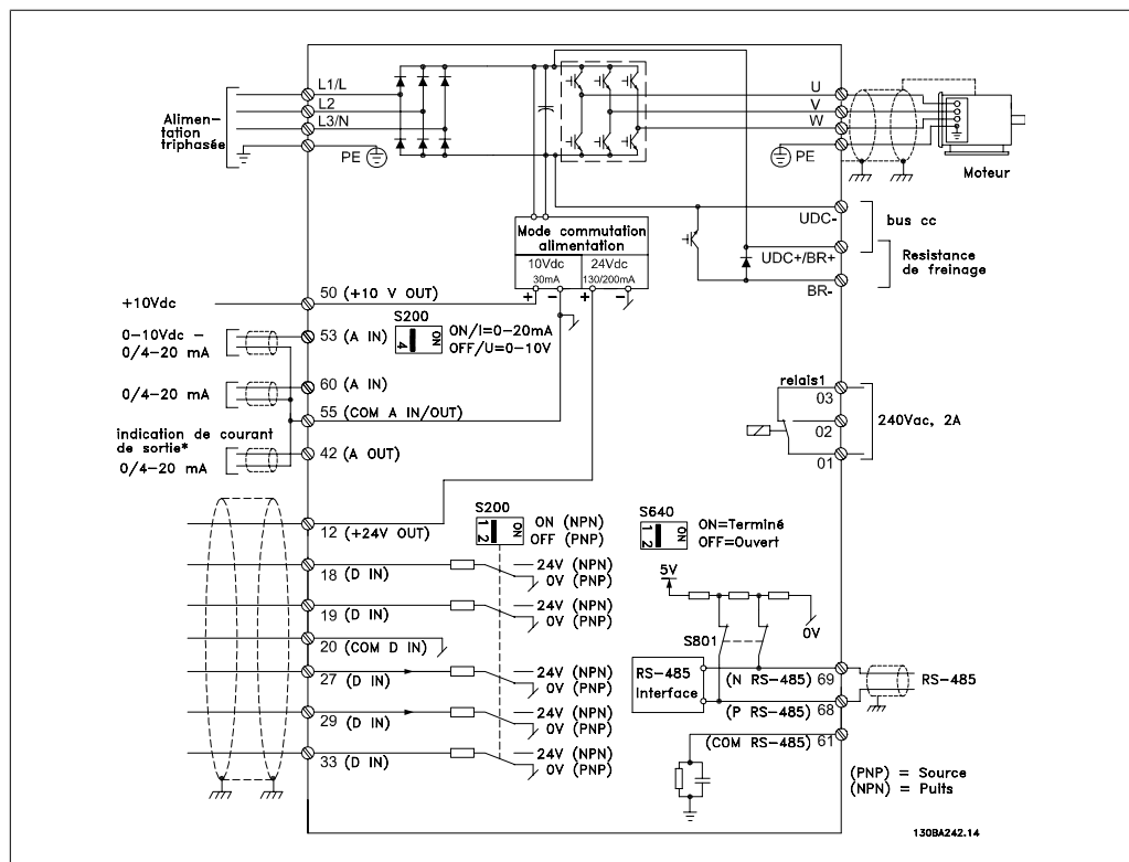
Illustration 4.28: Schéma représentant toutes les bornes. (La borne 37 n'existe que sur les unités avec fonction d'arrêt de sécurité.)
