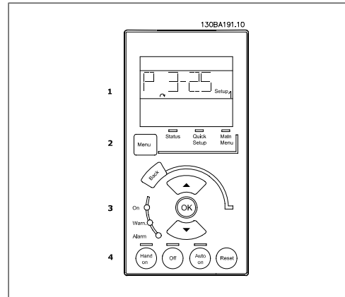
Illustration 5.1: LCP numérique (NLCP)
