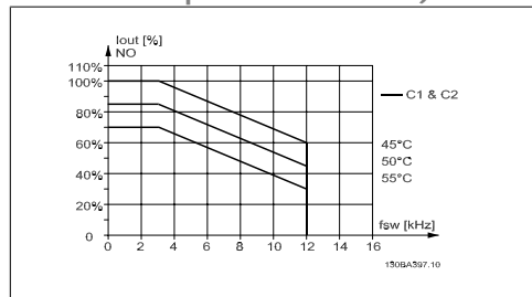
Illustration 8.7: Déclassement de I sortie pour différentes T AMB, MAX pour protection C, utilisant 60 PWM en mode couple normal (surcouple de 110 %)
