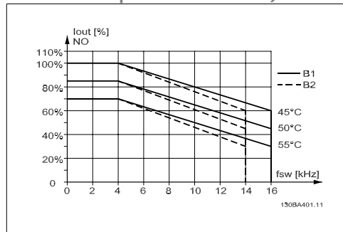
Illustration 8.5: Déclassement de I sortie pour différentes T AMB, MAX pour protection B, utilisant 60 PWM en mode couple normal (surcouple de 110 %)
