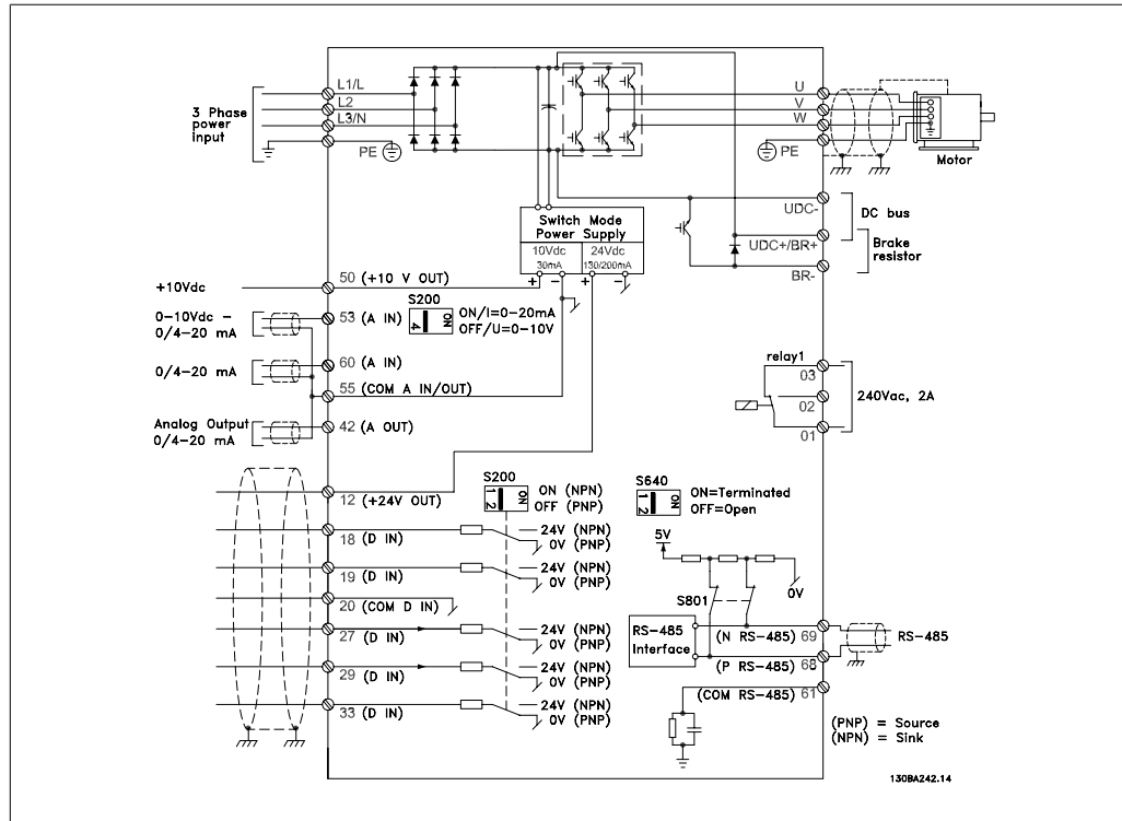
Illustration 4.28: Tüm elektrik terminallerini gösteren diyagram. (Terminal 37 yalnızca Güvenli Durdurma işlevine sahip birimlerde mevcuttur.)
