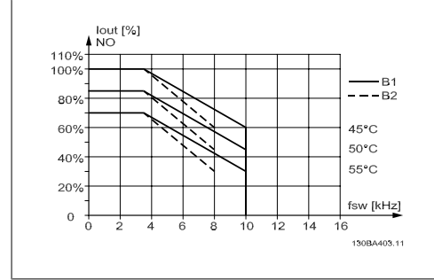
Illustration 8.6: B muhafazası için Normal tork modunda SFAVM kullanarak farklı T_{AMB, MAX} için I_{out} azaltma (%110 aşırı tork)
