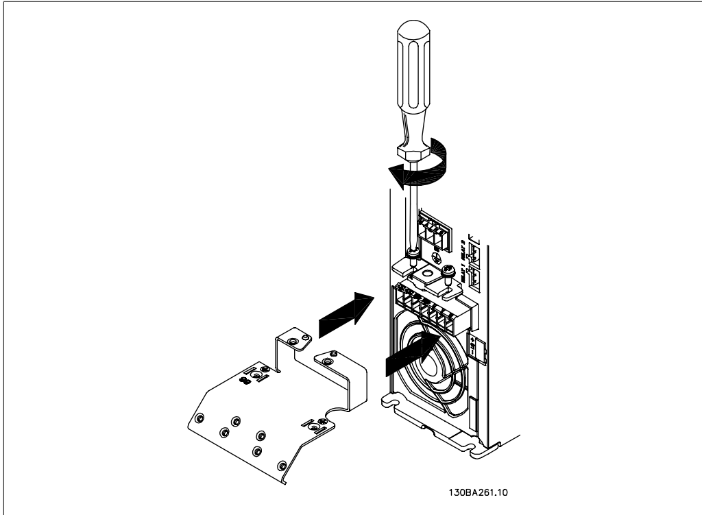
Illustration 4.2: Önce montaj plakasındaki iki vidayı monte edin ve plakayı yerine kaydırıp tam olarak sıkıştırın.
