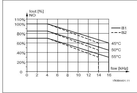
Illustration 8.5: B muhafazası için Normal tork modunda 60 PWM kullanarak farklı T_{AMB, MAX} için I_{out} azaltma (%110 aşırı tork)
