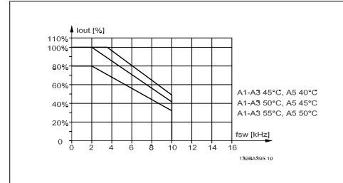
Illustration 8.2: A muhafazası için SFAVM kullanarak farklı T_{AMB, MAX} için I_{out} azaltma
