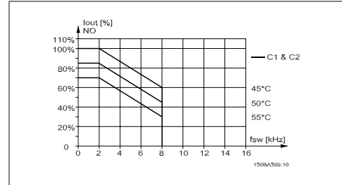
Illustration 8.8: C muhafazası için Normal tork modunda SFAVM kullanarak farklı T_{AMB, MAX} için I_{out} azaltma (%110 aşırı tork)
