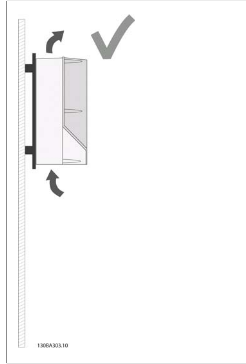
Illustration 3.4: Birimin duvarla az bir mesafe kalacak şekilde monte edilmesi gerekiyor ise, lütfen arka plakaya sahip bir birim seçin (bkz. Sıralama türü kod konumu 14-15). A2 ve A3 birimleri standart olarak arka plakaya sahiptirler.
