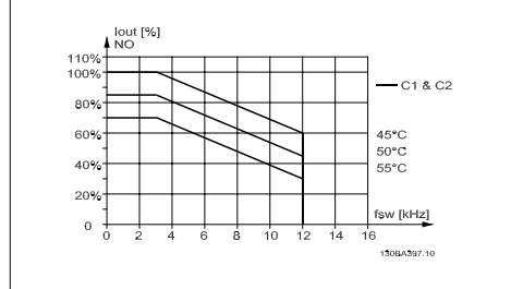
Illustration 8.7: C muhafazası için Normal tork modunda 60 PWM kullanarak farklı T_{AMB, MAX} için I_{out} azaltma (%110 aşırı tork)
