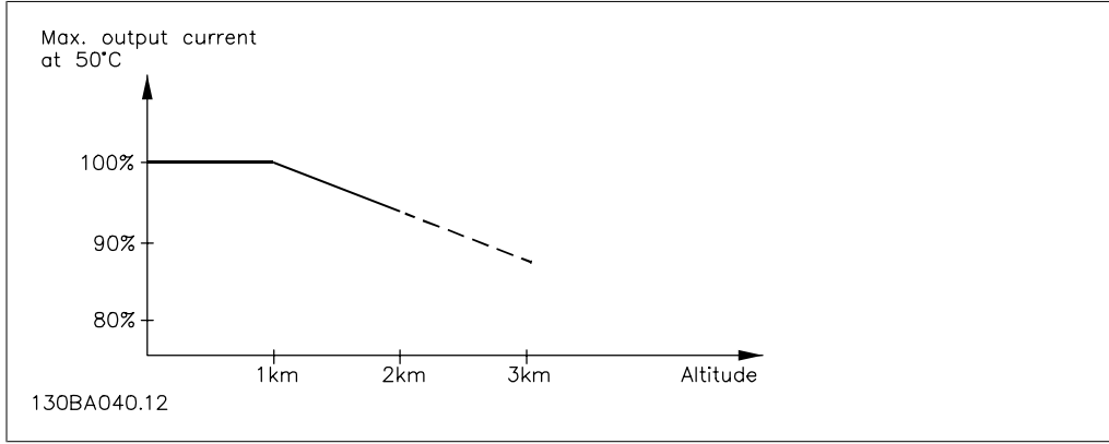
Illustration 8.9: T_{AMB, MAX} değerinde maksimum çıkış akımını denizden yüksekliğe göre azaltma. Denizden 2 km'den daha yüksek yerlerde, PELV ile ilgili lütfen Danfoss Drives ile irtibat kurun.
