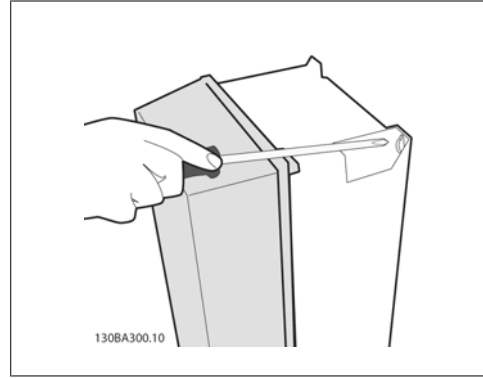
Illustration 3.14: Vidaların sıklığı
