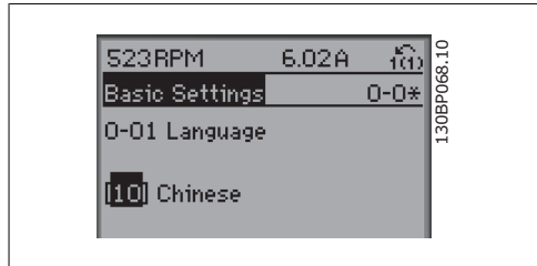
Illustration 6.11: Ekran örneği.
