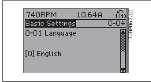
Illustration 6.10: Ekran örneği.
