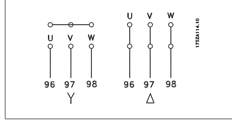
Illustration 4.10: Motor bağlantısı için terminaler.
