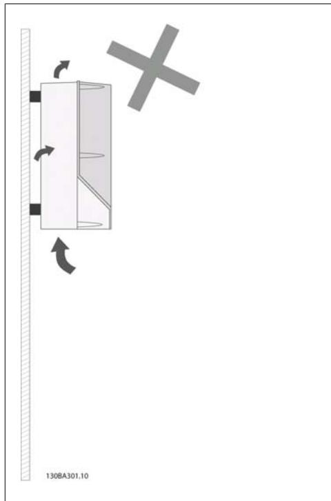
Illustration 3.3: A2 ve A3 haricindeki muhafazalar, arka plaka olmaksızın gösterilen birimlere monte edilmezler. Soğutma yetersiz olur ve servis ömrü büyük ölçüde kısalabilir.
