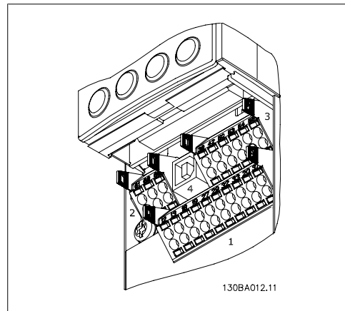
Illustration 4.18: Kontrol terminalleri (tüm muhafazalar)
