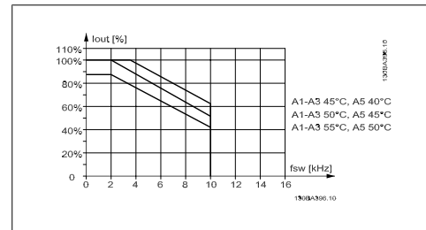
Illustration 8.4: A muhafazası için SFAVM ve maksimum 10 m motor kablosu kullanarak farklı T_{AMB, MAX} için I_{out} azaltma
