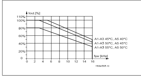
Illustration 8.1: A muhafazası için 60 PWM kullanarak farklı T_{AMB, MAX} için I_{out} azaltma
