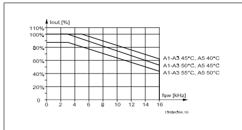
Illustration 8.3: A muhafazası için 60 PWM ve maksimum 10 m motor kablosu kullanarak farklı T_{AMB, MAX} için I_{out} azaltma
