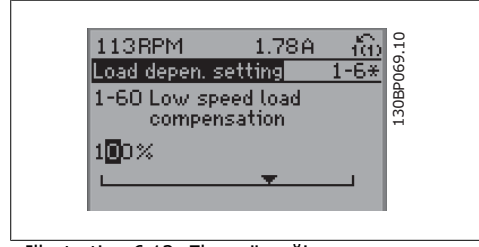
Illustration 6.12: Ekran örneği.
