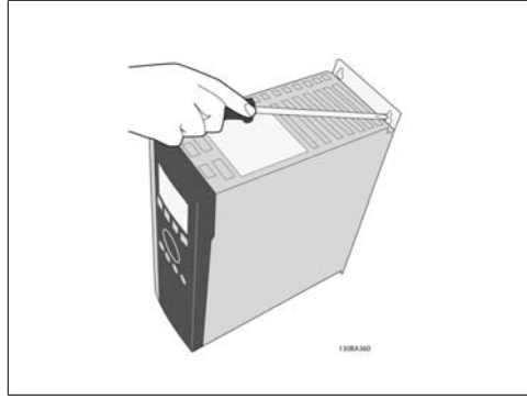
Illustration 3.9: Vidaların sıkılışı
