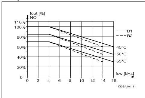
Illustration 8.5: Понижаване на I_{out} за различни T_{AMB, MAX} за обвивка В чрез използване на 60 PWM в режим на нормален въртящ момент (110% свръх въртящ момент)
