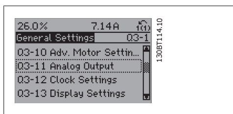
Illustration 6.6: Стъпка 5: Използвайте бутоните за навигация нагоре/надолу, за да превъртите до напр. Q3-11 Аналогови изходи . Натиснете [OK].
