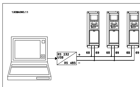
Illustration 5.6: Пример за свързване.
