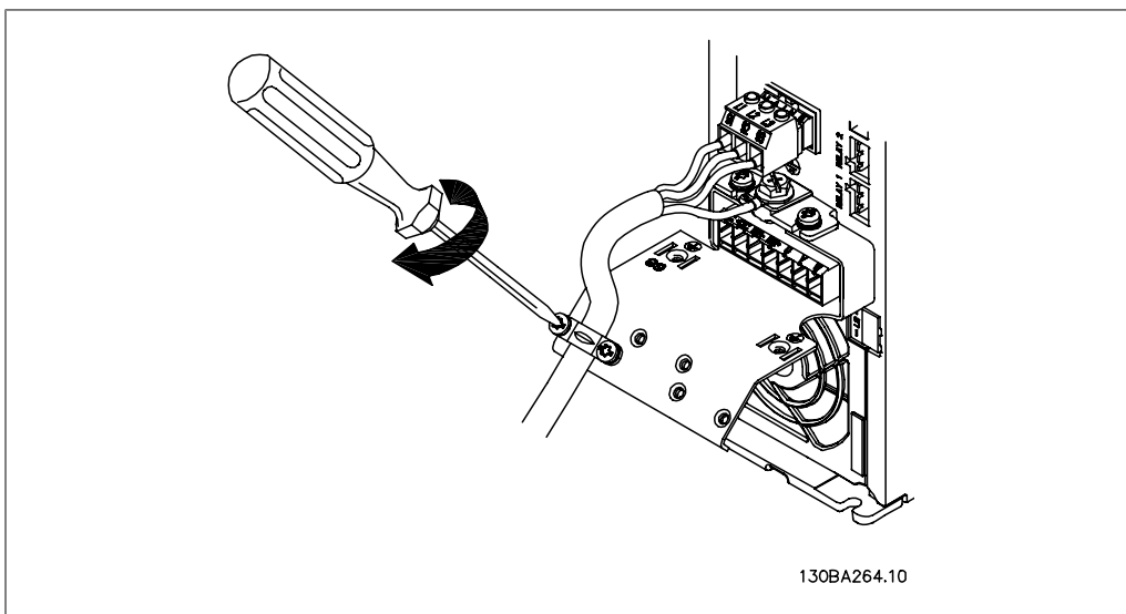
Illustration 4.5: Накрая затегнете скобата за закрепване върху мрежовите проводници.
