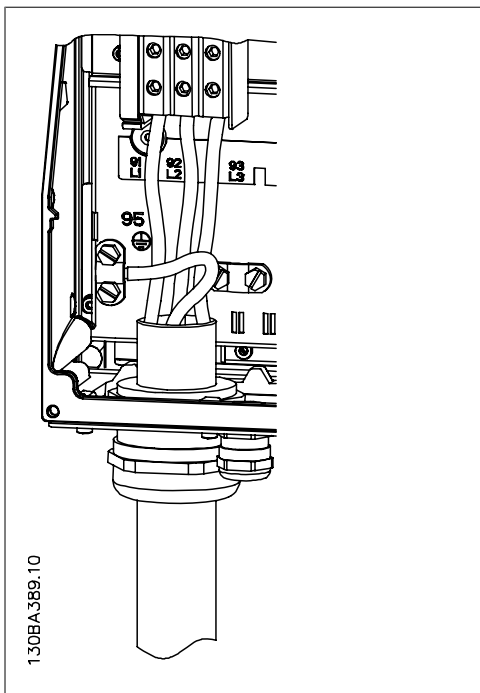
Illustration 4.9: Свързване към мрежата и заземяването.
