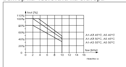
Illustration 8.2: Понижаване на I_{out} за различни T_{AMB, MAX} за обвивка A чрез използване на SFAVM
