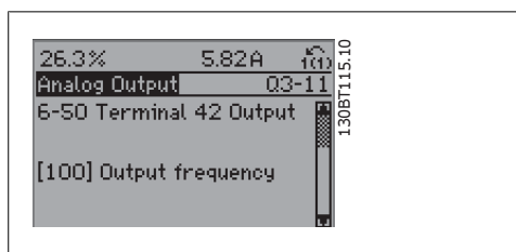
Illustration 6.7: Стъпка 6: Изберете параметър 6-50 Изход на клемма 42 . Натиснете [OK].
