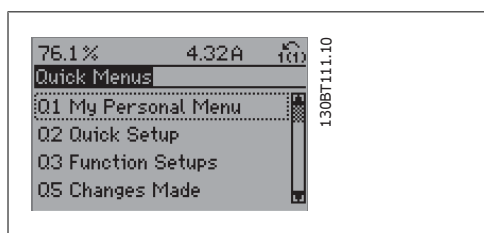
Illustration 6.3: Стъпка 2: Натиснете бутона [Quick Menus] (появява се изборът "Бързи менюта").
