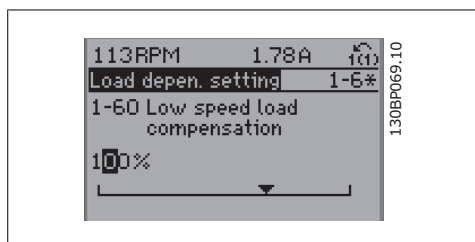
Illustration 6.12: Пример за показване на дисплея.
