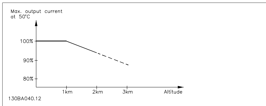
Illustration 8.9: Понижаване на изходния ток по отношение на надморската височина при T_{amb, max} . За надморска височина над 2 км трябва да се направи справка от Danfoss Drives по отношение на PELV.
