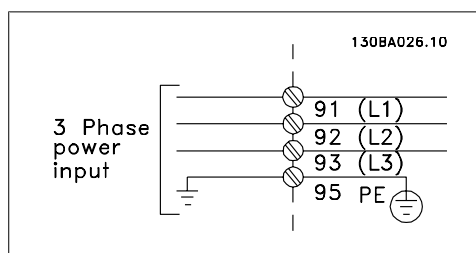
Illustration 4.1: Клеми за мрежата и заземяването
