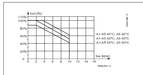
Illustration 8.4: Понижаване на I_{out} за различни T_{AMB, MAX} за обвивка A чрез използване на SFAVM и максимална дължина на кабела на електродвигателя 10 m
