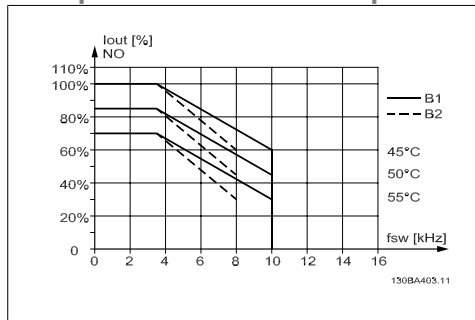
Illustration 8.6: Понижаване на I_{out} за различни T_{AMB, MAX} за обвивка В чрез използване на SFAVM в режим на нормален въртящ момент (110% свръх въртящ момент)
