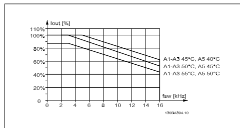
Illustration 8.3: Понижаване на I_{out} за различни T_{AMB, MAX} за обвивка A чрез използване на 60 PWM и максимална дължина на кабела на електродвигателя 10m
