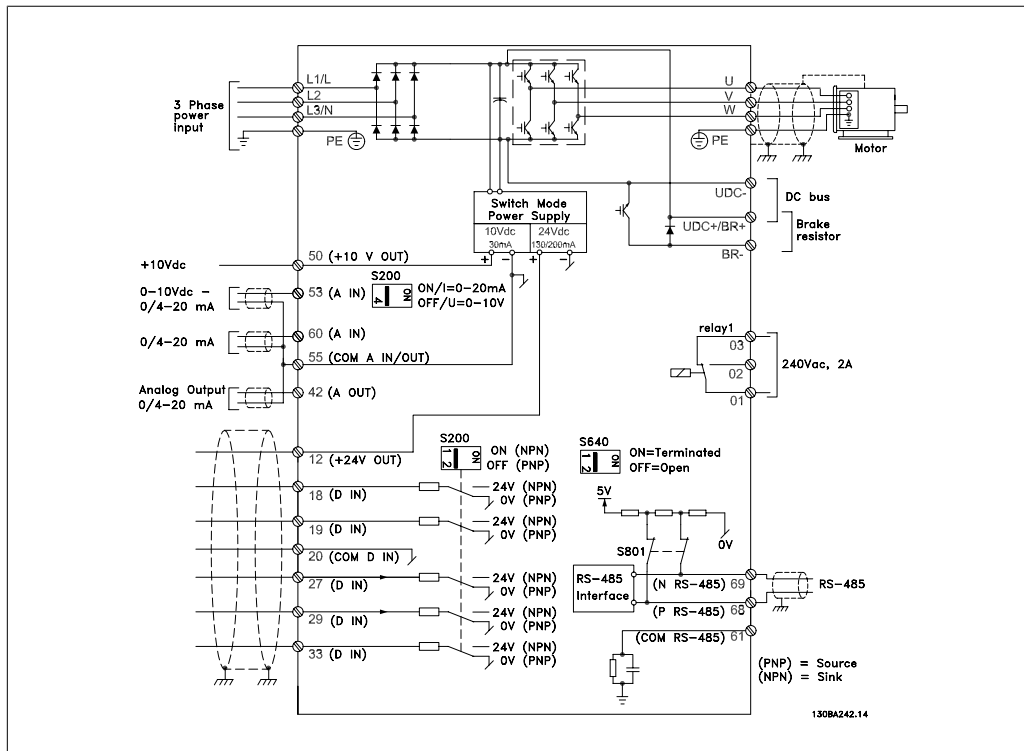
Illustration 4.28: Схема, показваща всички електрически клеми. (Клема 37 присъства само за устройства с функция безопасен стоп.)
