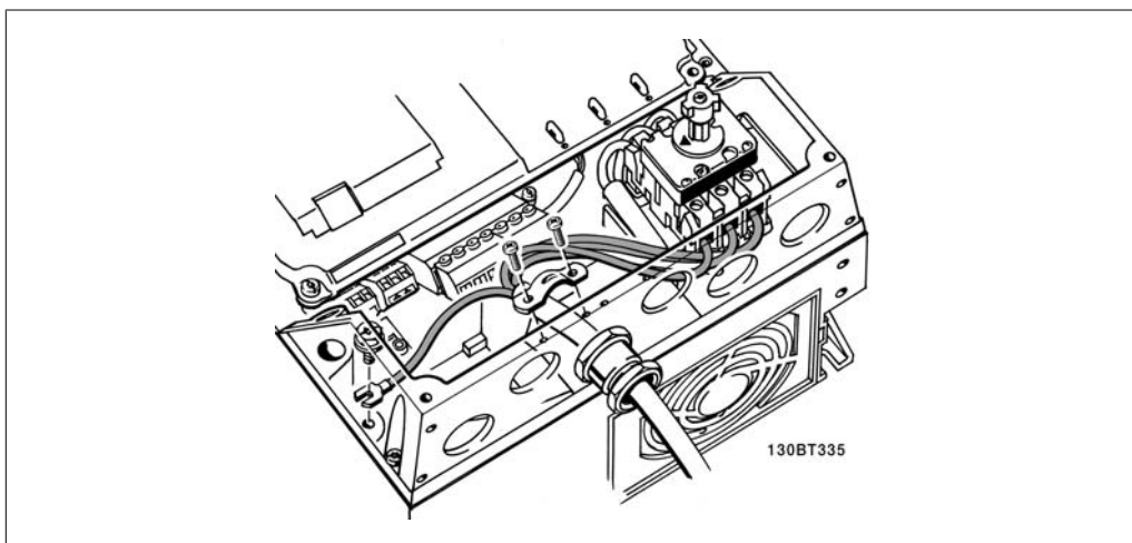
Illustration 4.7: Свързване към мрежата и заземяването с мрежов прекъсвач.
