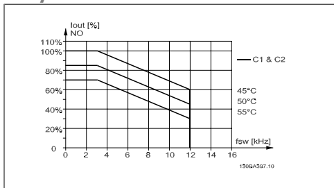
Illustration 8.7: Понижаване на I_{out} за различни T_{AMB, MAX} за обвивка С чрез използване на 60 PWM в режим на нормален въртящ момент (110% свръх въртящ момент)
