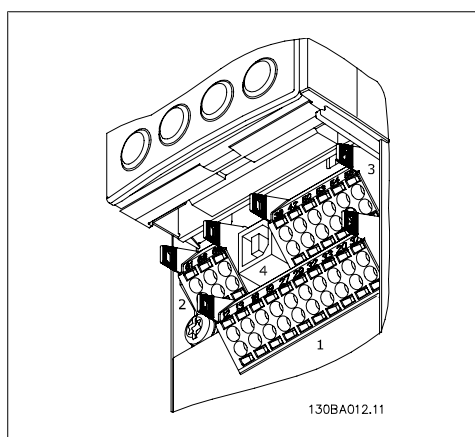
Illustration 4.18: Управляващи клеми (всички обвивки)
