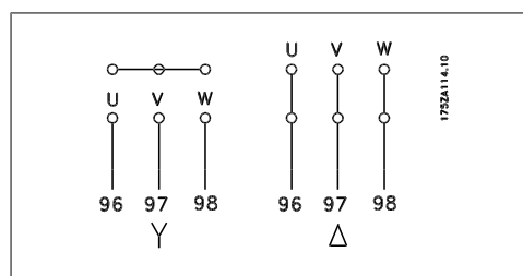
Illustration 4.10: Клеми за свързване на електродвигателя
