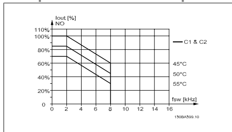
Illustration 8.8: Понижаване на I_{out} за различни T_{AMB, MAX} за обвивка С чрез използване на SFAVM в режим на нормален въртящ момент (110% свръх въртящ момент)
