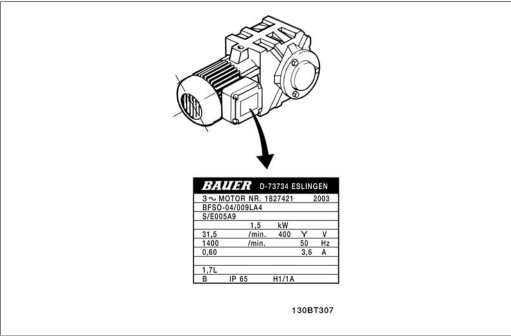
Illustration 4.31: Пример за табелката на електродвигателя
