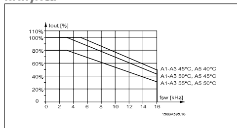
Illustration 8.1: Понижаване на I_{out} за различни T_{AMB, MAX} за обвивка A чрез използване на 60 PWM
