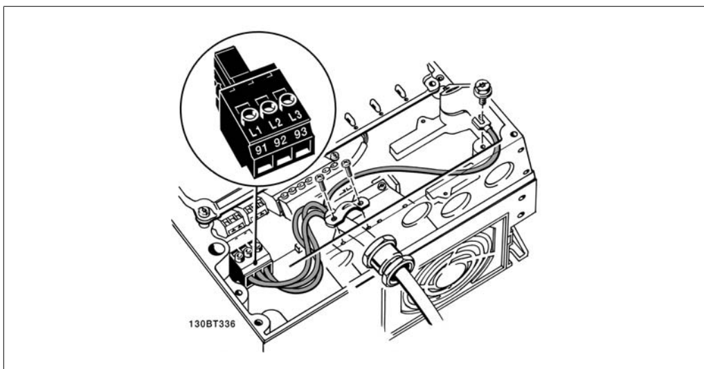
Illustration 4.6: Свързване към мрежата и заземяването без мрежов прекъсвач. Отбележете, че се използва кабелна скоба.
