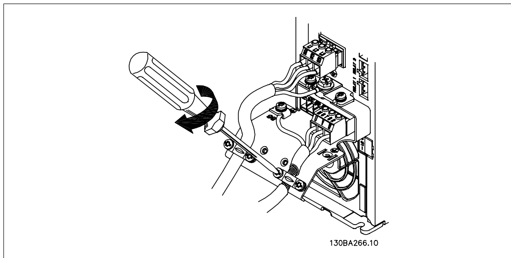
Illustration 4.12: Монтирайте кабелна скоба, за да осигурите свързване на 360 градуса между шасито и екрана, като отбележите, че външната изолация на кабела на електродвигателя се отстранява под скобата.
