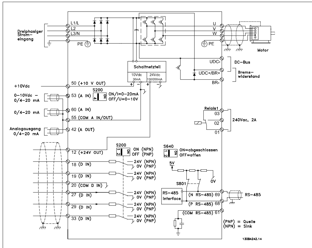
Abbildung 4.28: Abbildung 1.1: Elektrische Installation, Übersicht (Klemme 37 nur für Geräte mit Funktion „Sicherer Stopp“.)
