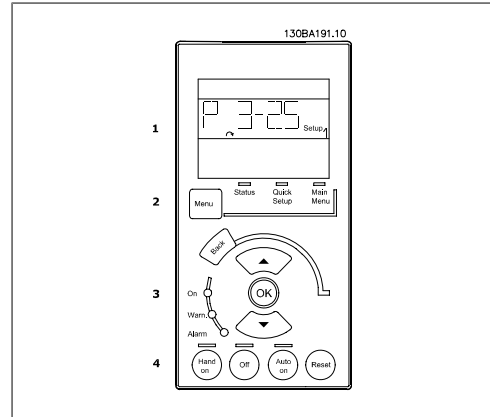
Abbildung 5.1: Numerische LCP Bedieneinheit LCP101
