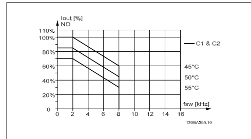
Abbildung 8.8: Leistungsreduzierung von I_{aus} für verschiedene T_{AMB, MAX} für Gehäuse C über SFAVM in normalem Drehmomentmodus (110 % Überlastmoment)
