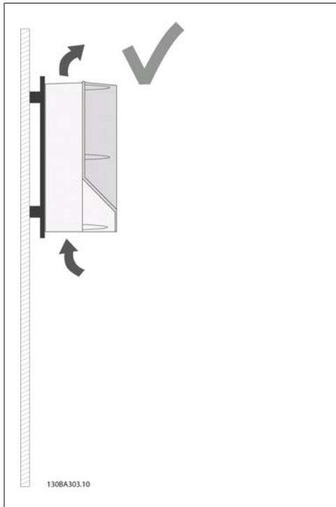
Abbildung 3.4: Wenn das Gerät mit geringem Abstand von der Wand befestigt werden muss, bestellen Sie bitte eine Rückplatte für das Gerät (siehe Bestellnummernposition 14-15). A2- und A3-Geräte haben serienmäßig eine Rückplatte.
