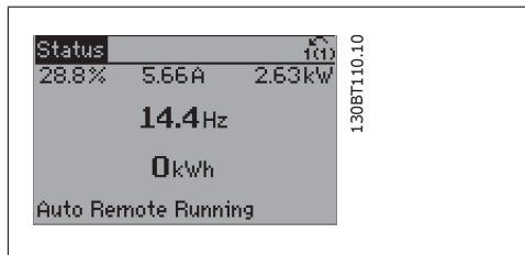
Abbildung 6.2: 1. Schritt: Den Frequenzumrichter einschalten (LEDs leuchten auf).
