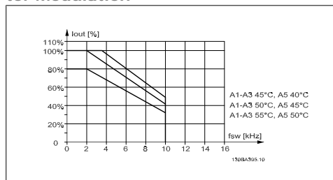
Abbildung 8.2: Leistungsreduzierung I_{aus} für verschiedene T_{AMB, MAX} für Gehäuse A über SFAVM
