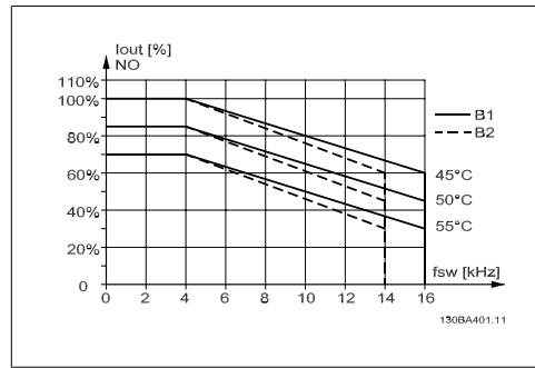
Abbildung 8.5: Leistungsreduzierung von I_{aus} für verschiedene T_{AMB, MAX} für Gehäuse B über 60° PWM in normalem Drehmomentmodus (110 % Überlastmoment)
