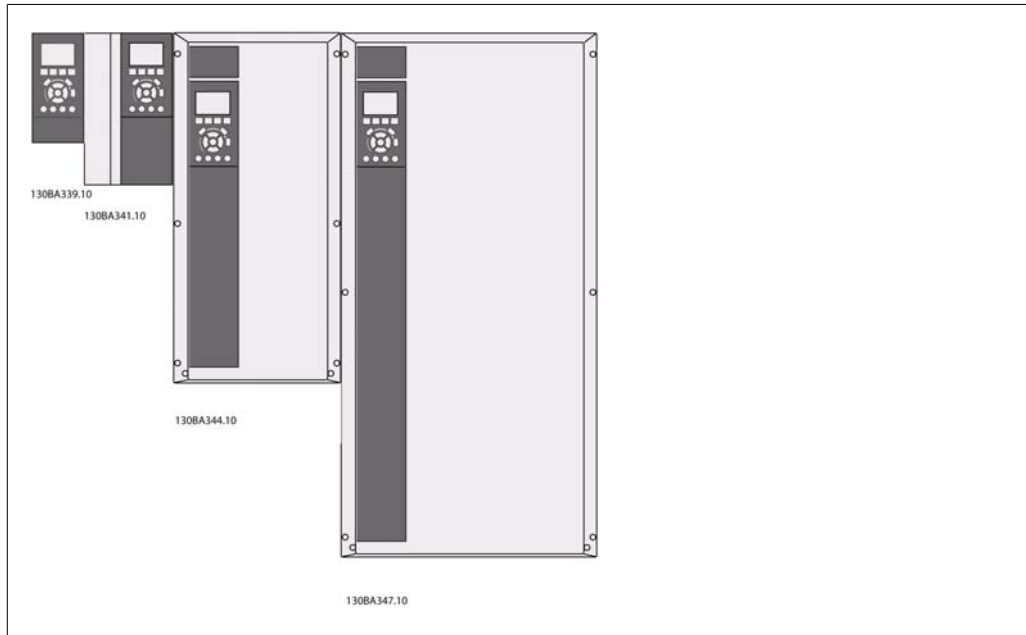
Abbildung 3.1: Montage nebeneinander für alle Gehäusegrößen.
