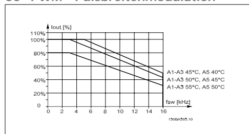
Abbildung 8.1: Leistungsreduzierung von I_{aus} für verschiedene T_{AMB, MAX} für Gehäuse A bei 60° PWM
