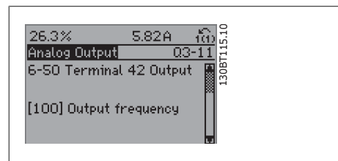
Abbildung 6.7: 6. Schritt: Parameter 6-50 Klemme 42 Analogausgang wählen. [OK] drücken.
