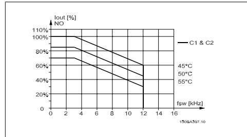
Abbildung 8.7: Leistungsreduzierung von I_{aus} für verschiedene T_{AMB, MAX} für Gehäuse C über 60° PWM in normalem Drehmomentmodus (110 % Überlastmoment)
