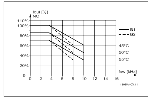
Abbildung 8.6: Leistungsreduzierung von I_{aus} für verschiedene T_{AMB, MAX} für Gehäuse B über SFAVM in normalem Drehmomentmodus (110 % Überlastmoment)
