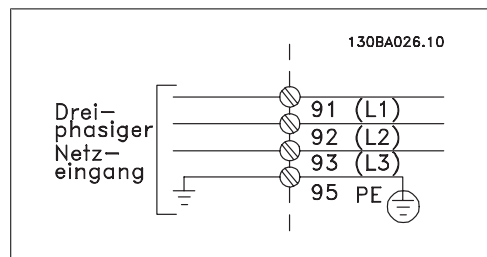
Abbildung 4.1: Klemmen für Netz- und Erdanschluss
