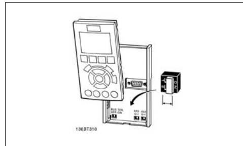
Abbildung 4.30: Position der Schalter
