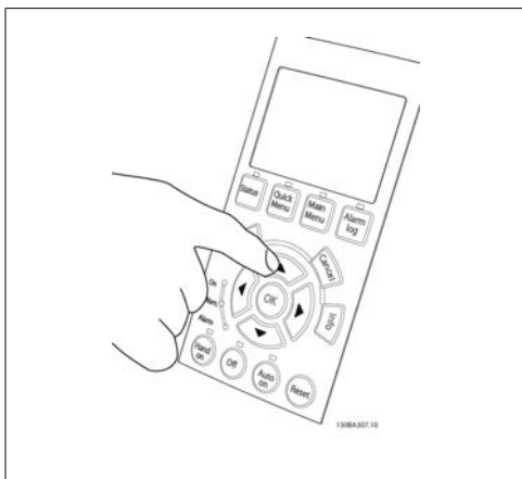
Abbildung 4.24: 6. Schritt: Die Drehzahl des Motors wird auf dem LCP angezeigt. Sie kann über die Pfeiltasten nach oben ▲ und unten ▼ geändert werden.
