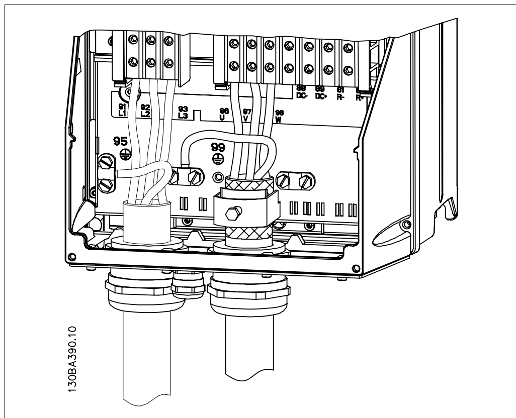
Abbildung 4.15: Terminieren Sie zuerst die Motorerde und setzen Sie dann die U-, V- und W-Drähte des Motors in die Klemme und ziehen Sie sie fest. Bitte stellen Sie sicher, dass die äußere Isolierung des Motor-kabels unter dem EMV-Schirmbügel entfernt wird.
