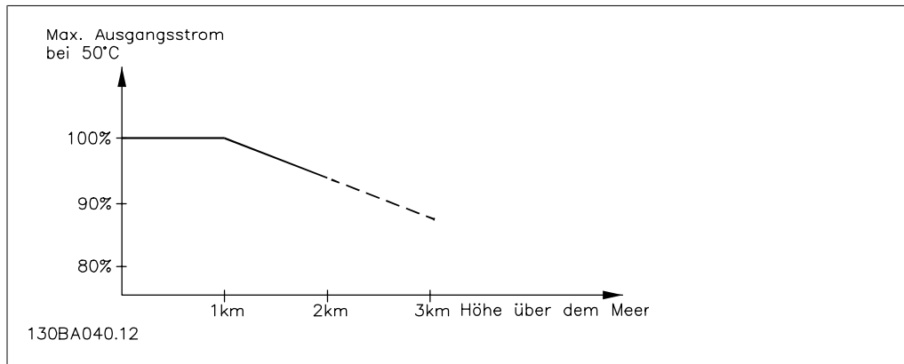
Abbildung 8.9: Reduzierung des Ausgangsstroms in Abhängigkeit von der Höhe bei T_{AMB, MAX} . Bei Höhen über 2 km über NN ziehen Sie bitte Danfoss Drives zu PELV (Schutzkleinspannung) zurate.
