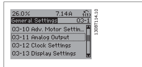
Abbildung 6.6: 5. Schritt: Mit den Auf/Ab-Navigationstasten zu 03-11 Analogausgang blättern. [OK] drücken.
