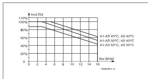
Abbildung 8.3: Leistungsreduzierung von I_{aus} für verschiedene T_{AMB, MAX} für Gehäuse A über 60° PWM und maximales 10 m Motorkabel
