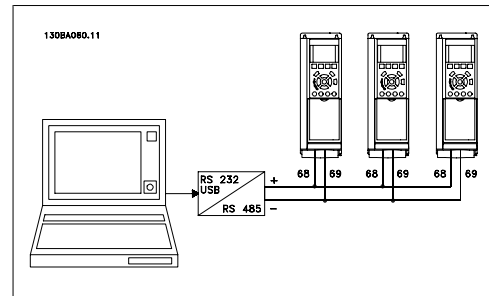
Abbildung 5.6: Anschlussbeispiel
