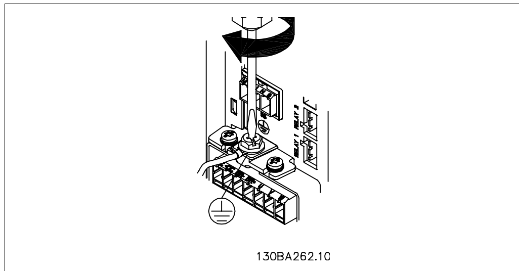
Abbildung 4.3: Befestigen Sie beim Montieren von Kabeln zuerst das Erdkabel und ziehen Sie es fest.
