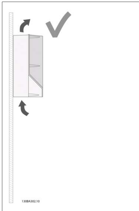
Abbildung 3.2: Dies ist die richtige Einbauweise der Geräte.
