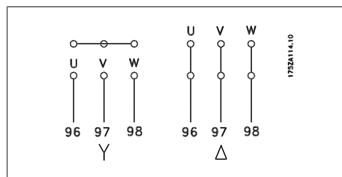
Abbildung 4.10: Klemmen für Motoranschluss
