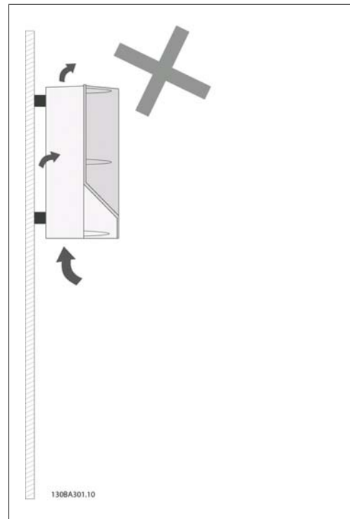
Abbildung 3.3: Befestigen Sie die Geräte nicht wie abgebildet ohne Rückplatte (außer bei A2- und A3-Gehäuse). In diesem Fall ist die Kühlung unzureichend und die Lebensdauer kann sich drastisch reduzieren.
