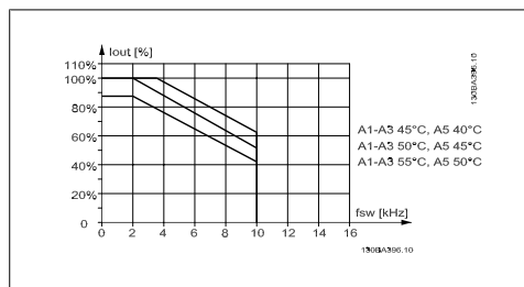
Abbildung 8.4: Leistungsreduzierung I_{aus} für verschiedene T_{AMB, MAX} für Gehäuse A über SFAVM und maximales 10 m Motorkabel
