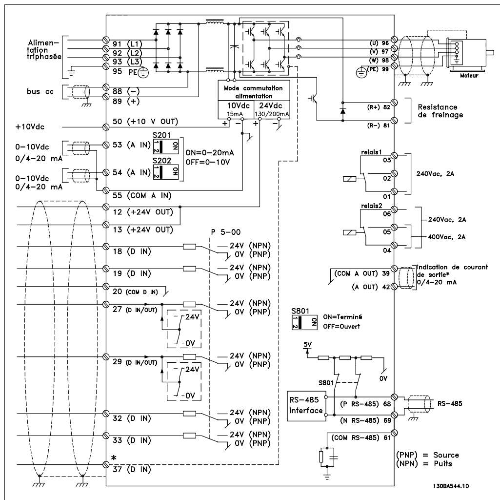
Illustration 4.28: Schéma présentant toutes les bornes électriques. (La borne 37 n'existe que sur les unités avec fonction d'arrêt de sécurité.)
