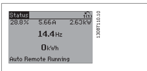
Illustration 6.2: Étape 1 : mettre le variateur de fréquence sous tension (voyant jaune allumé).
