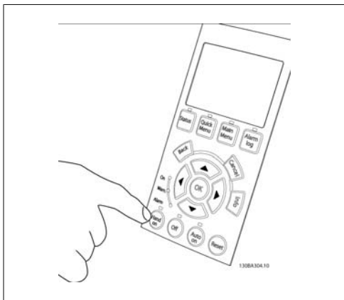
Disegno 4.23: Fase 5: Premendo il pulsante [Hand on], il LED sopra il pulsante dovrebbe essere illuminato e il motore può ruotare.
