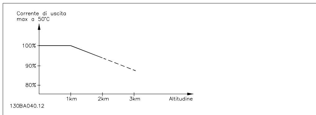
Disegno 8.9: Declassamento della corrente di uscita rispetto all'altitudine, con T_{AMB, MAX} . Per altitudini superiori ai 2 km, contattare Danfoss Drives riguardo alle disposizioni PELV.
