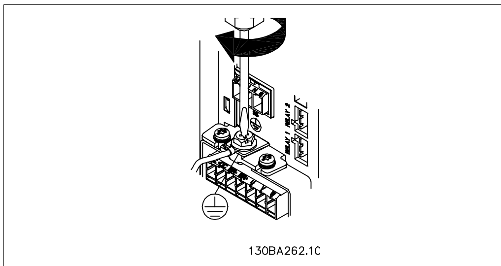
Disegno 4.3: Quando si montano i cavi, prima deve essere montato e serrato il cavo di terra.
