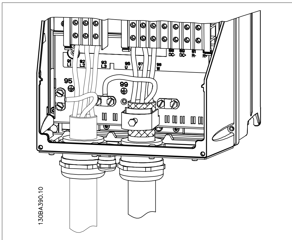
Disegno 4.15: Prima fissare il conduttore di terra del motore, quindi inserire i fili U, V e W del motore nel morsetto e serrarli. Assicurare che l'isolamento esterno del cavo motore viene rimosso sotto il pressacavo EMC.
