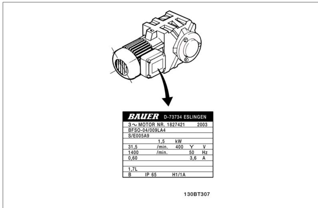
Disegno 4.31: Esempio di targhetta del motore
