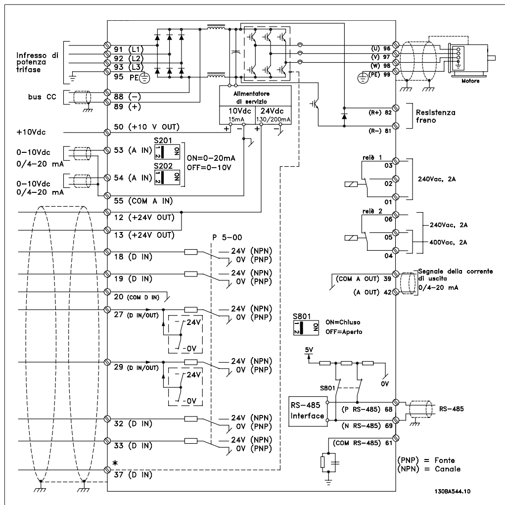
Disegno 4.28: Il diagramma mostra tutti i morsetti elettrici. (Il morsetto 37 è solo presente per unità con funzione di arresto di sicurezza).
