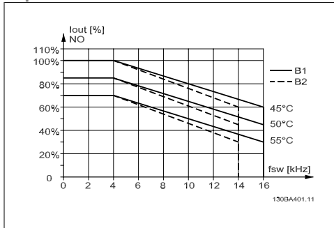
Disegno 8.5: Declassamento di I_{out} in base a diverse T_{AMB, MAX} per la custodia B utilizzando 60 PWM nel modo coppia normale (110% sovrapposizione)
