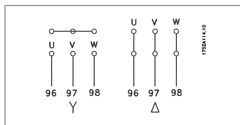
Disegno 4.10: Morsetti per il collegamento del motore
