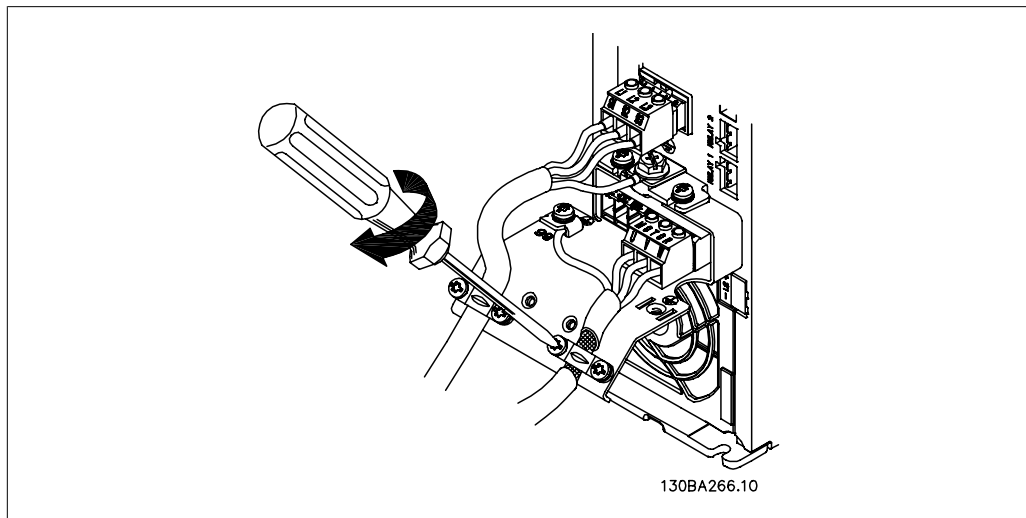
Disegno 4.12: Montare il pressacavo per assicurare una connessione a 360 gradi tra telaio e schermo; notare che l'isolamento esterno del cavo motore viene rimosso sotto il morsetto.
