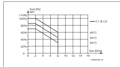
Disegno 8.8: Declassamento di I_{out} in base a diverse T_{AMB, MAX} per il custodia C utilizzando SFAVM nel modo coppia normale (110% sovrapposizione)
