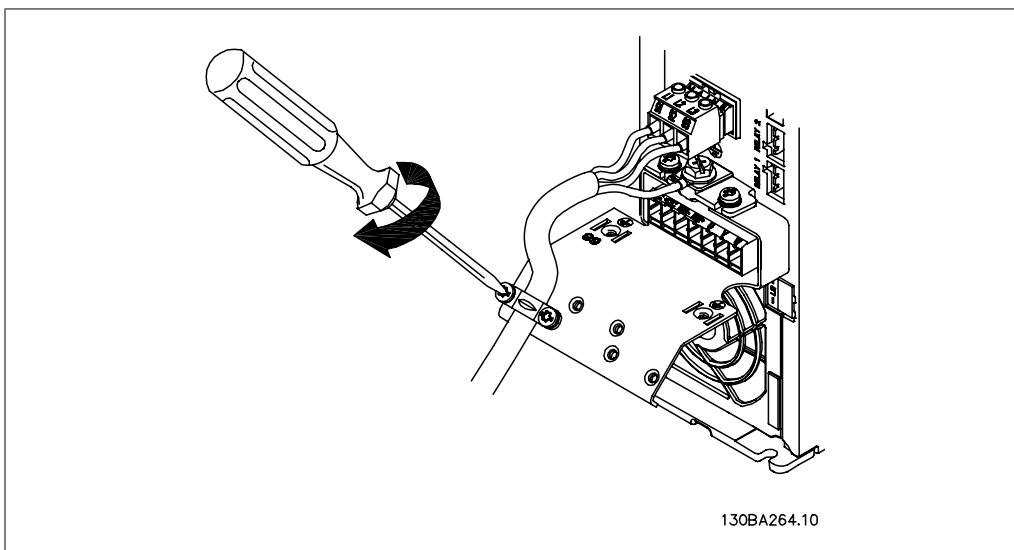
Disegno 4.5: Infine serrare la staffa di supporto sui cavi di rete.
