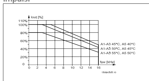
Disegno 8.1: Declassamento di I_{out} in base a diverse T_{AMB, MAX} per la custodia A utilizzando 60 PWM
