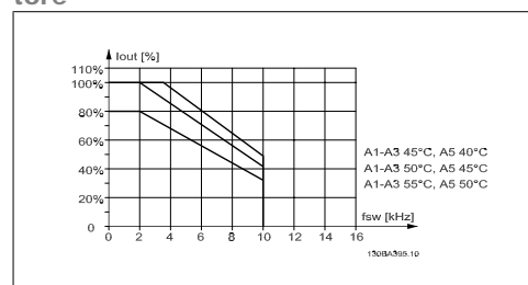
Disegno 8.2: Declassamento di I_{out} in base a diverse T_{AMB, MAX} per la custodia A utilizzando la SFAVM
