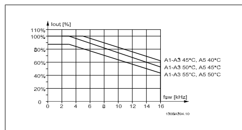
Disegno 8.3: Declassamento di I_{out} in base a diverse T_{AMB, MAX} per la custodia A utilizzando 60 PWM e un cavo motore lungo al massimo 10 m
