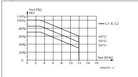
Disegno 8.7: Declassamento di I_{out} in base a diverse T_{AMB, MAX} per il custodia C utilizzando 60 PWM nel modo coppia normale (110% sovrapposizione)
