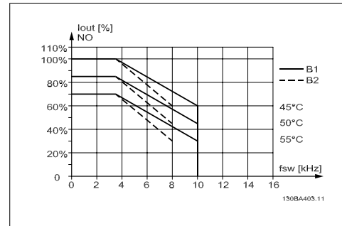
Disegno 8.6: Declassamento di I_{out} in base a diverse T_{AMB, MAX} per la custodia B utilizzando SFAVM nel modo coppia normale (110% sovrapposizione)
