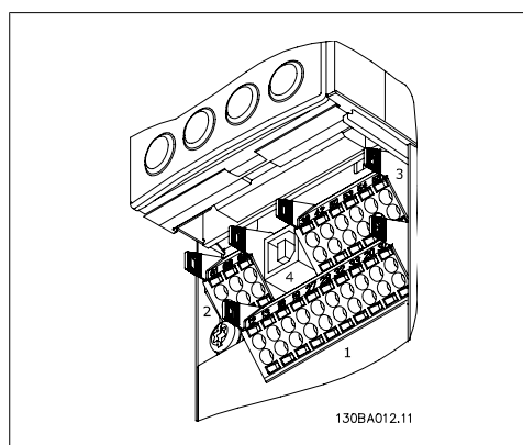
Disegno 4.18: Morsetti di controllo (tutte le custodie)
