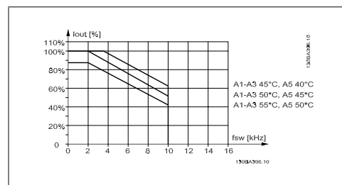
Disegno 8.4: Declassamento di I_{out} in base a diverse T_{AMB, MAX} per il custodia A utilizzando il SFAVM e un cavo motore lungo al massimo 10 m
