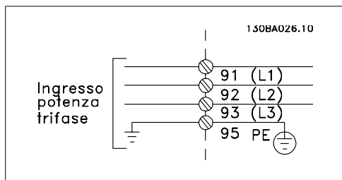
Disegno 4.1: Morsetti per la rete e la messa a terra.
