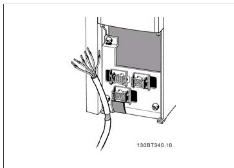
Disegno 4.29: Pressacavo per cavo di comando.
