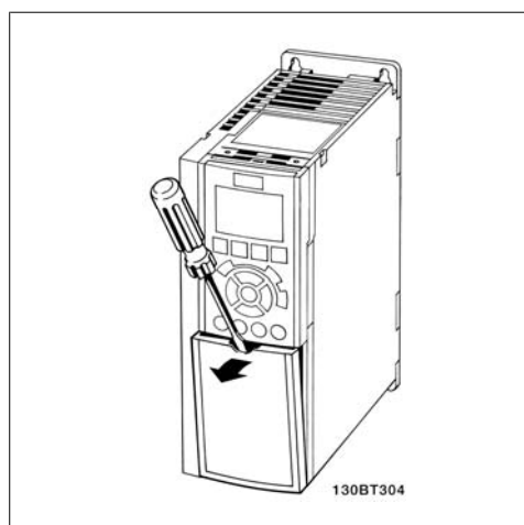
Disegno 4.16: Custodie A2 e A3
