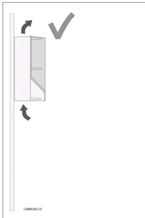
Disegno 3.2: Questo è il modo corretto per montare l'unità.
