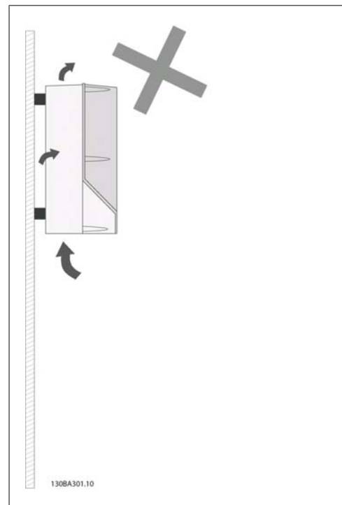
Disegno 3.3: Non montare unità con custodie diverse da A2 e A3 come mostrato senza pannello posteriore - il raffreddamento è insufficiente e la
