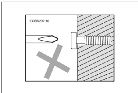
Disegno 3.7: Montaggio errato delle viti.
