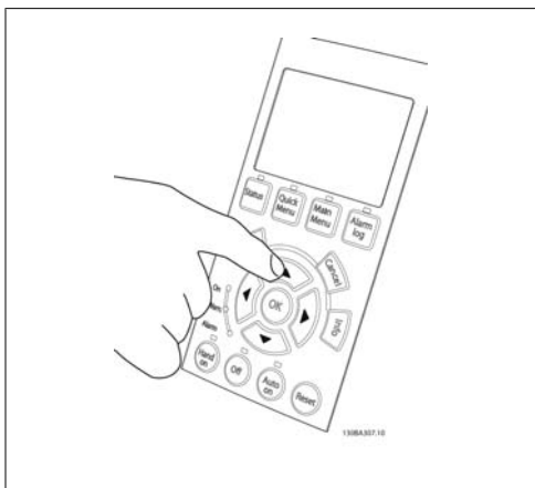
Disegno 4.24: Fase 6: La velocità del motore può essere visualizzata nell'LCP. Può essere regolata utilizzando i tasti a freccia Su ▲ e Giù ▼.
