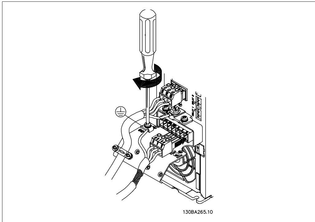
Disegno 4.11: Prima fissare il conduttore di terra del motore, quindi inserire i fili U, V e W del motore nei morsetti e serrarli.
