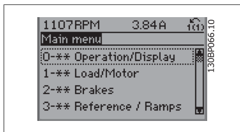
Bild 6.9: Displayexempel.
