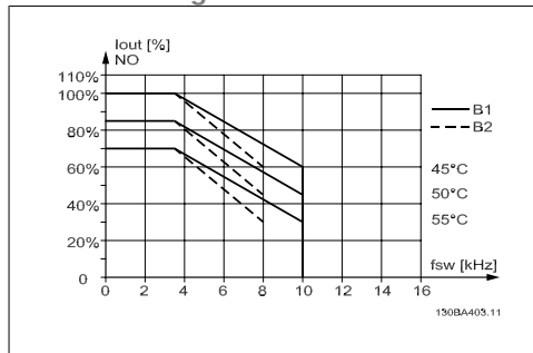
Bild 8.6: Nedstämpling av I_{out} för olika T_{AMB, MAX} för kapsling med SFAVM i läget Normalt moment (110 % övermoment)
