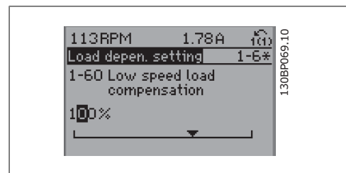
Bild 6.12: Displayexempel.
