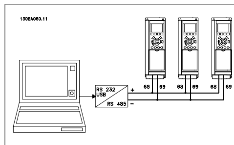
Bild 5.6: Anslutningsexempel.
