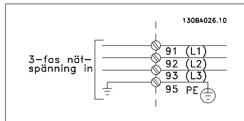
Bild 4.1: Plintar för nät och jordning.
