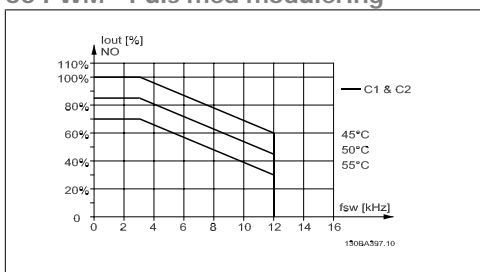
Bild 8.7: Nedstämpling av I_{out} för olika T_{AMB, MAX} för kapsling C med 60 PWM i läget Normalt moment (110 % övermoment)
