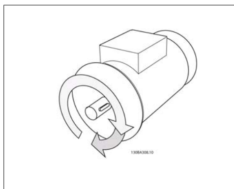
Bild 4.27: Steg 9: Byt ut två motorledningar om du inte får önskad rotationsriktning.
