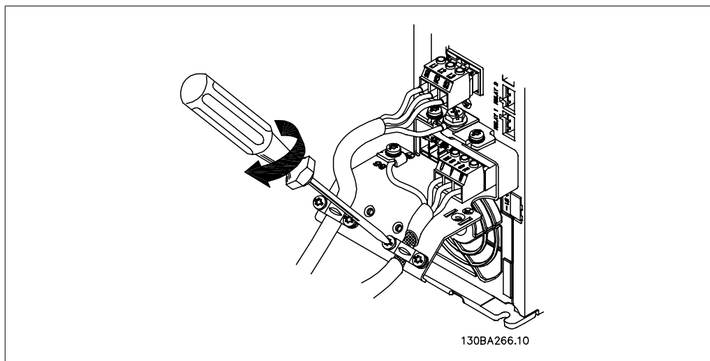
Bild 4.12: Montera kabelklämman för att säkerställa en 360-gradersanslutning mellan chassit och skärmen. Observera att kabelisoleringen är avlägsnad under klämman.
