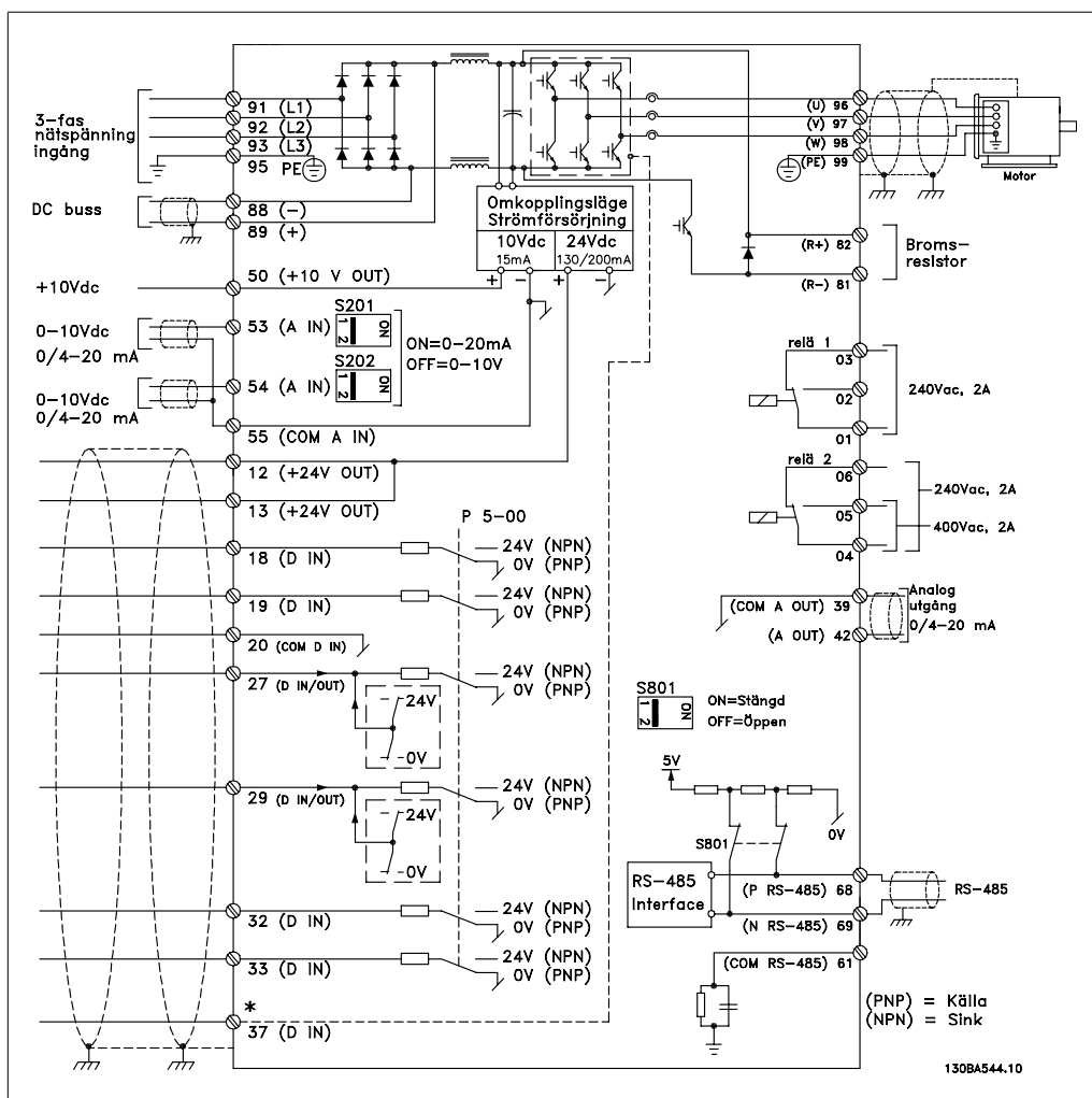
Bild 4.28: Diagram som visar alla elektriska plintar. (Plint 37 fungerar enbart med enheter som har funktionen säkerhetsstopp.)
