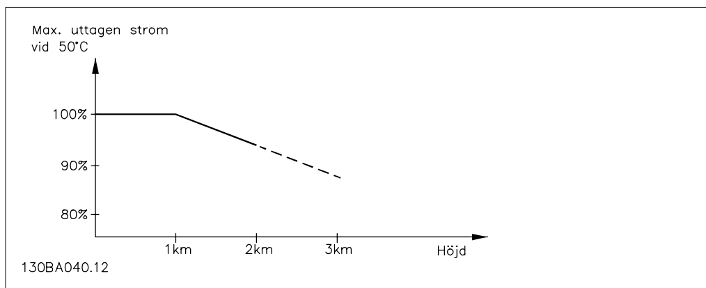
Bild 8.9: Nedstämpling av utström i förhållande till höjd vid T_{AMB} . Vid höjdskillnader över 2 km kontakta Danfoss Drives om PELV.
