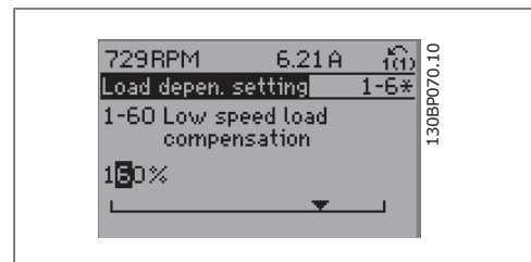
Bild 6.13: Displayexempel.
