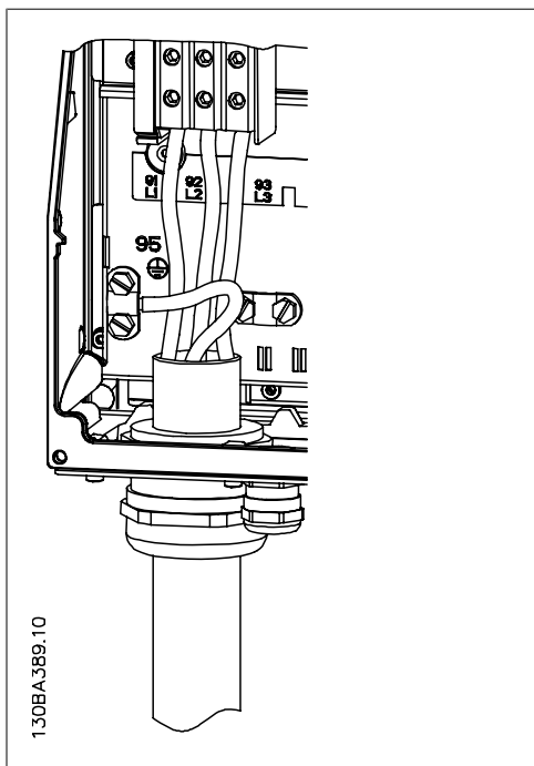
Bild 4.9: Hur du ansluter till nät och jordning.
