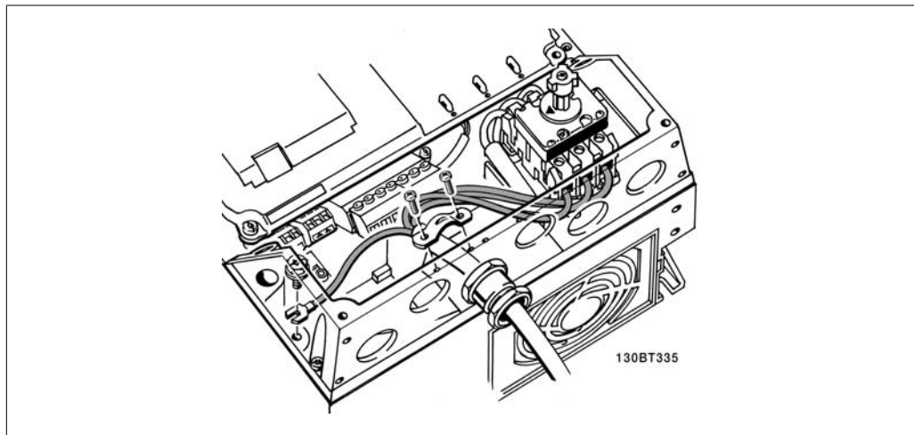
Bild 4.7: Anslutning till nät och jordning med huvudströmbrytare.
