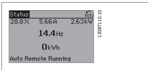
Bild 6.2: Steg 1: Starta frekvensomformaren (gul lysdiod)
