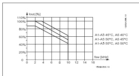
Bild 8.4: Nedstämpling av I_{out} för olika T_{AMB,MAX} för A-kapsling med SFAVM och maximum 10 m motorkabel
