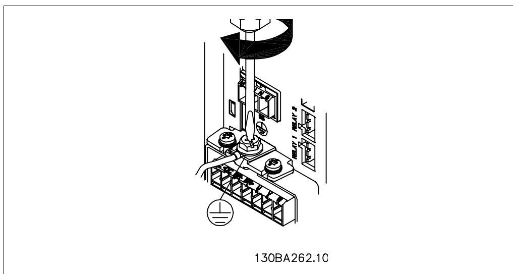
Bild 4.3: Montera först och dra åt skruven för jordkabeln när kablarna monteras.
