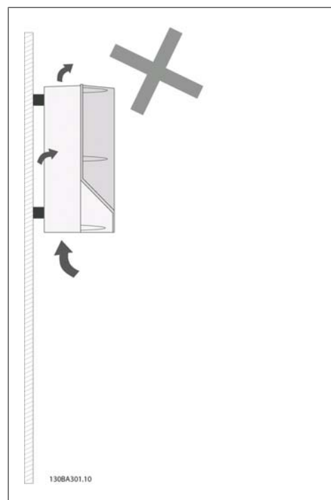
Bild 3.3: Montera inte enheter som visas på bilden utan bakvägg. Endast A2- och A3-kapslingar får
