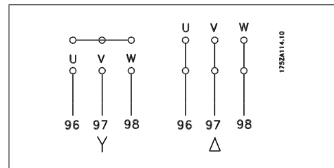
Bild 4.10: Plintar för motoranslutning
