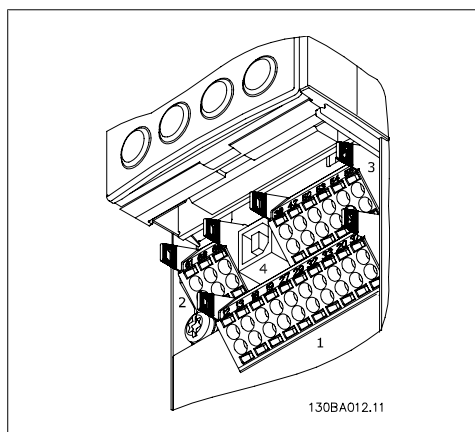
Bild 4.18: Styrplintar (alla kapslingar)
