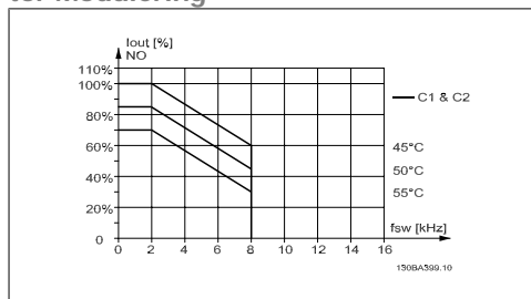
Bild 8.8: Nedstämpling av I_{out} för olika T_{AMB, MAX} för kapsling C med SFAVM i läget Normalt moment (110 % övermoment)
