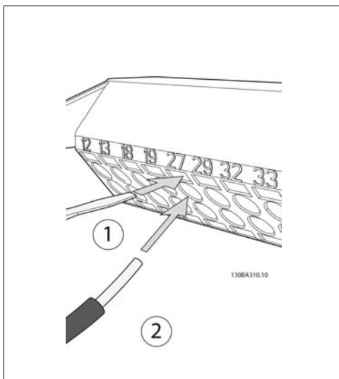
Bild 4.20: Steg 2: Infoga ena änden i plint 27 med hjälp av en lämplig skruvmejsel. (Observera: Den befintliga bygeln mellan plint 12 och 37 inte får avlägsnas på enheter med säkerhetsstopp om enheten ska kunna fungera!
