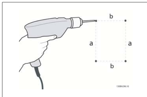
Bild 3.5: Borra hål
