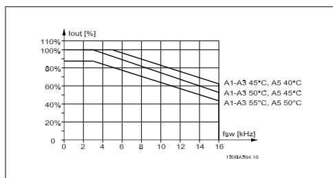
Bild 8.3: Nedstämpling av I_{out} för olika T_{AMB,MAX} för A-kapsling när 60 PWM används och maximalt 10 m motorkabel
