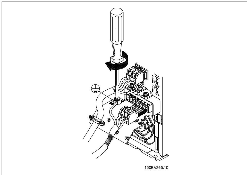
Bild 4.11: Avsluta först motorns jordanslutning, placera sedan motorns U-, V- och W-ledningar i kontakten och dra åt.
