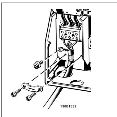
图 4.8: 如何连接主电源和接地。
