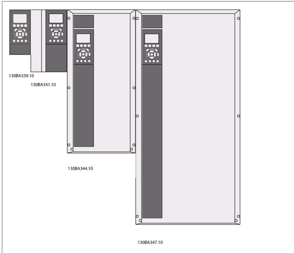
图 3.1: 无论机架尺寸如何, 均可并排安装。
