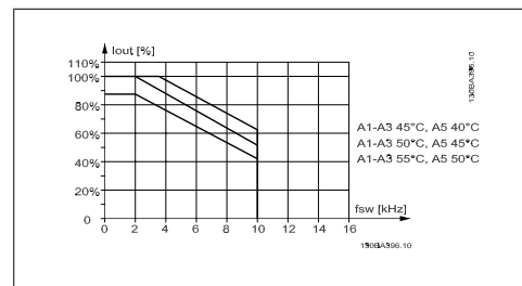
图 8.4: I_{out} 在不同 T_{AMB, MAX} 下的降容 - A 型机箱，开关模式为 SFAVM，电动机电缆的最大长度不超过 10 m
