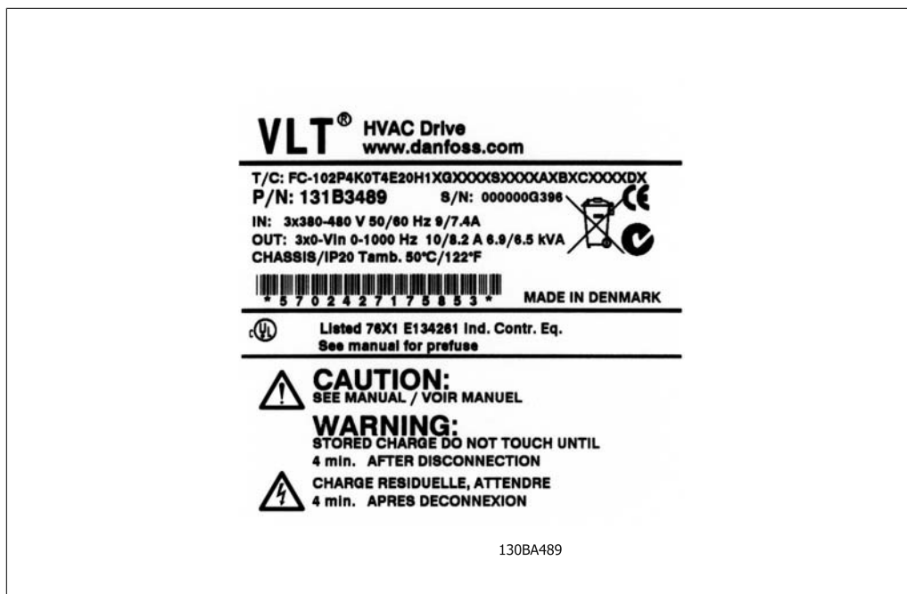
图 2.1: 该示例显示了一个标识标志。
