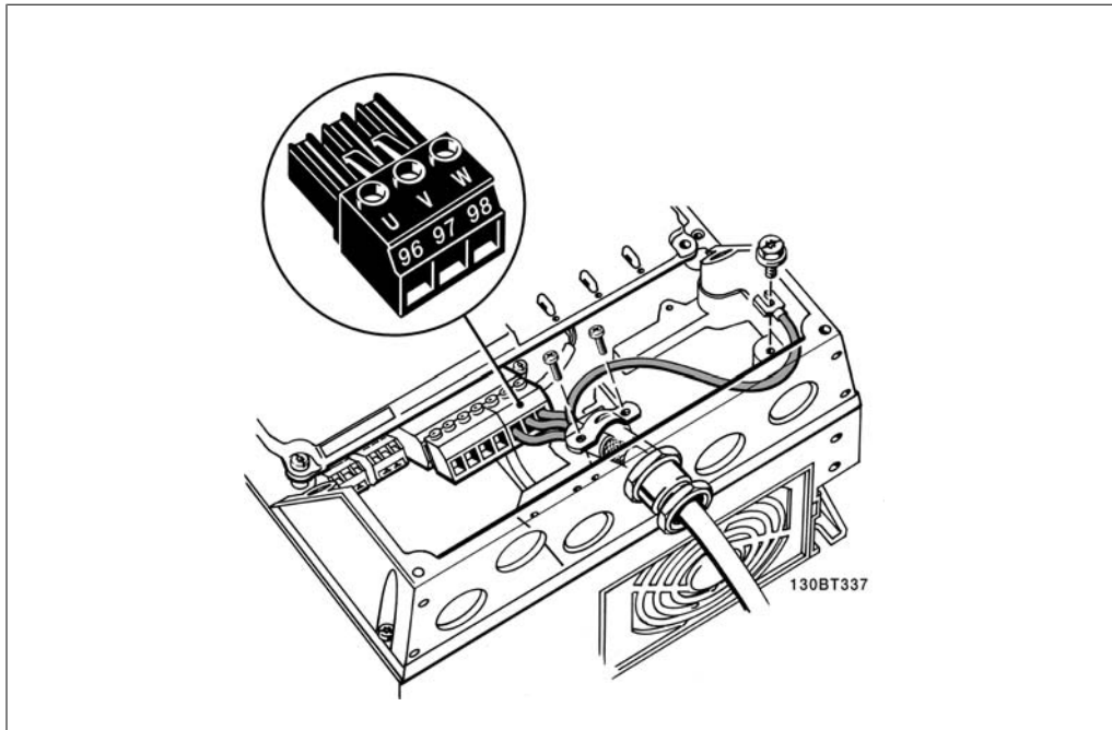
图 4.13: 首先端接电动机地线, 然后将电动机的 U、V 和 W 电线接入端子并拧紧。确保已剥去 EMC 线夹下方的电动机电缆的外部绝缘层。
