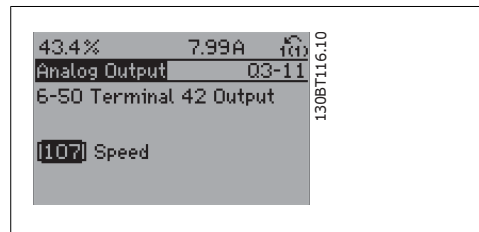
图 6.8: 步骤 7: 使用向上/向下导航键选择不同选项。按 [OK] (确定)。
