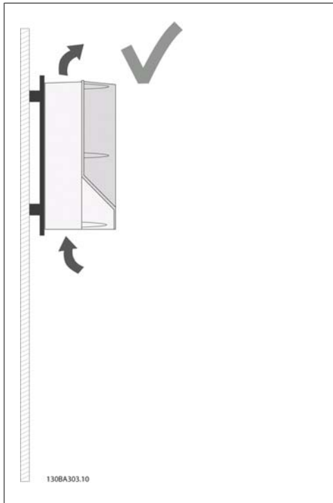
图 3.4: 如果设备必须安装在离墙很近的位置, 请订购该设备的背板 (请参阅订购类型代码, 第 14-15 位)。A2 和 A3 设备标配中就带有背板。
