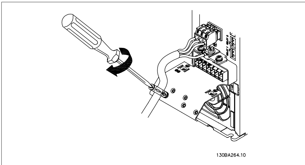
图 4.5: 最后，拧紧主电源电线的支持架。
