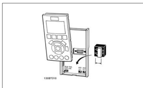
图 4.30: 开关位置。
