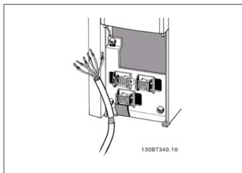
图 4.29: 控制电缆线夹。
