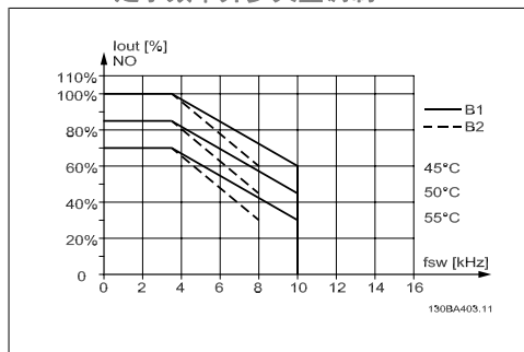
图 8.6: I_{out} 在不同 T_{AMB, MAX} 下的降容 - B 型机箱, 在正常转矩模式 (110% 过转矩) 下使用 SFAVM
