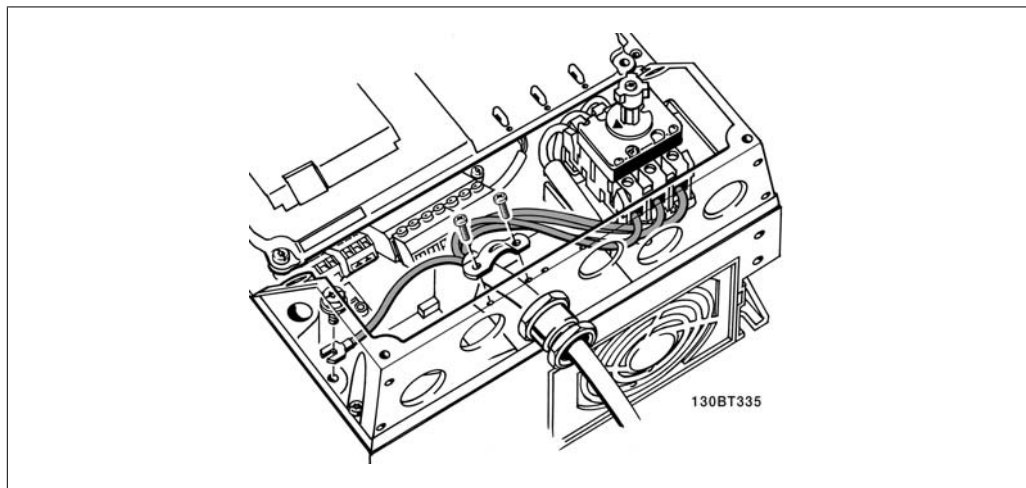
图 4.7: 如何使用主电源断路开关连接主电源和接地。
