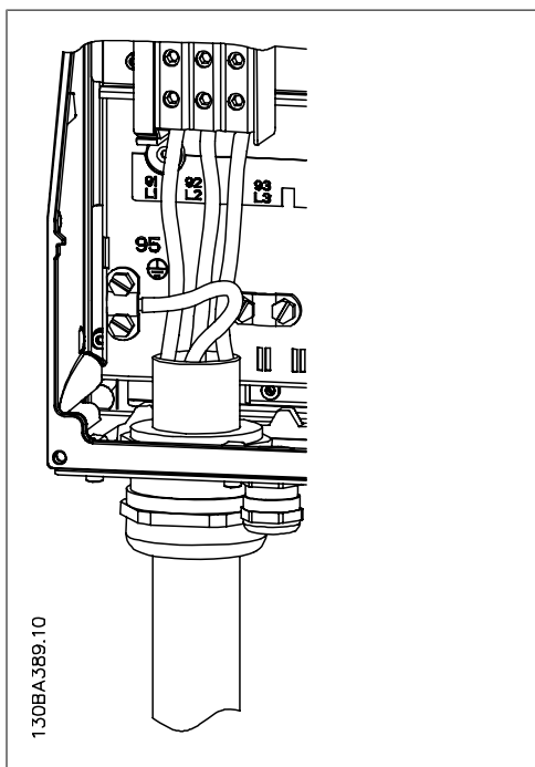
图 4.9: 如何连接主电源和接地。
