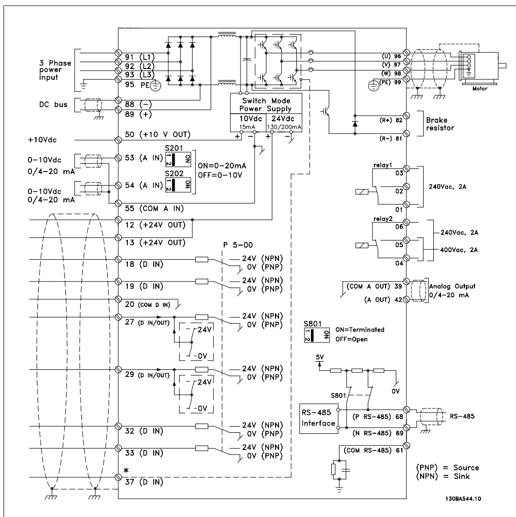
图 4.28: 图示显示了所有电气端子。(仅带有安全停止功能的设备才提供端子 37。)
