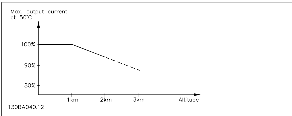
图 8.9: 在 T_{AMB, MAX} 下, 输出电流降容与海拔的关系。当海拔超过 2 km 时, 请向 Danfoss Drives 咨询 PELV 相关事宜。
