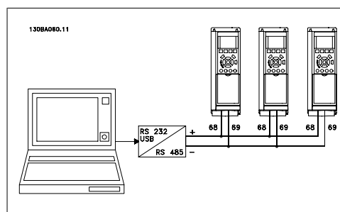
图 5.6: 连接示例。
