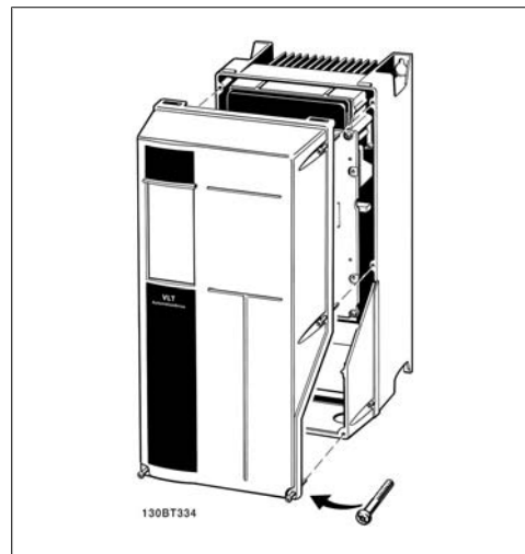
图 4.17: A5、B1、B2、C1 和 C2 机箱
