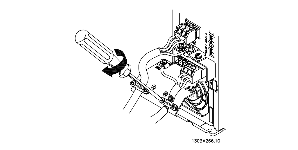
图 4.12: 安装电缆夹, 以确保机架和屏蔽丝网达到 360 度连接。注意, 请去除电缆夹下面电动机电缆的外部绝缘层。
