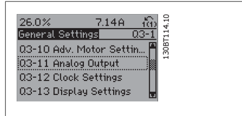
图 6.6: 步骤 5: 使用向上/向下导航键向下滚动到目标选项, 比如 03-11 模拟输出。按 [OK] (确定)。
