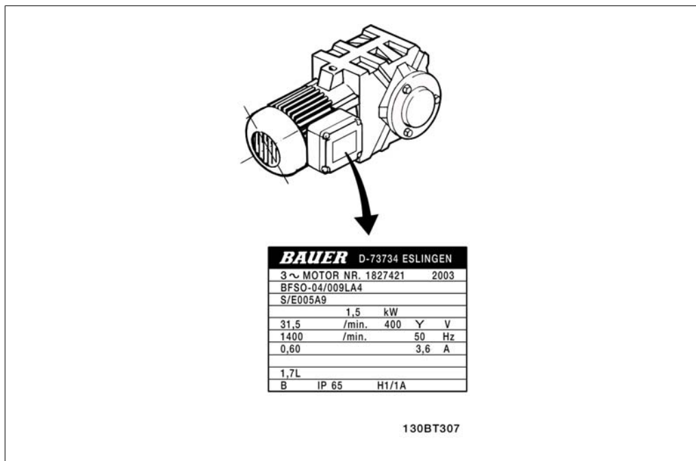
图 4.31: 电动机铭牌示例
