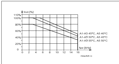
图 8.1: I_{out} 在不同 T_{AMB, MAX} 下的降容 - A 型机箱，开关模式为 60 PWM
