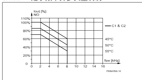
图 8.8: I_{out} 在不同 T_{AMB, MAX} 下的降容 - C 型机箱, 在正常转矩模式 (110% 过转矩) 下使用 SFAVM
