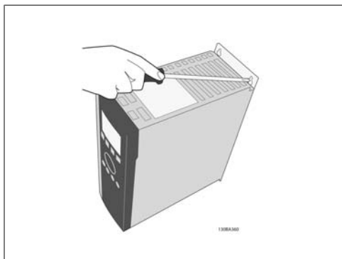
图 3.9: 拧紧螺钉
