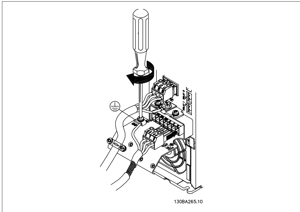
图 4.11: 首先, 断开电动机接地, 然后, 将电动机 U、V 和 W 电线插入插头并拧紧。
