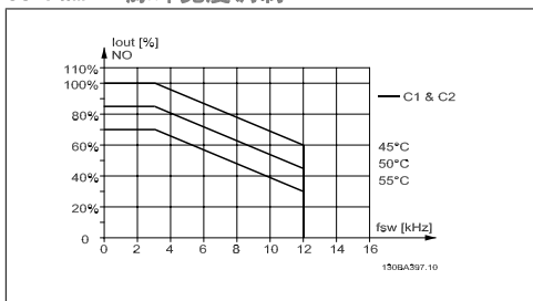
图 8.7: I_{out} 在不同 T_{AMB, MAX} 下的降容 - C 型机箱, 在正常转矩模式 (110% 过转矩) 下使用 60 PWM
