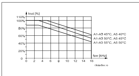
图 8.3: I_{out} 在不同 T_{AMB, MAX} 下的降容 - A 型机箱，开关模式为 60 PWM，电动机电缆的最大长度不超过 10 m
