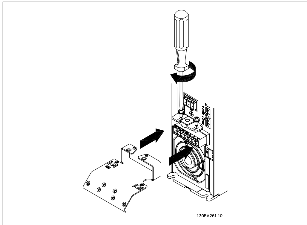
图 4.2: 首先, 将两个螺钉安装到固定板上, 然后将其滑动入位并完全拧紧。
