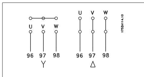
图 4.10: 电动机连接端子
