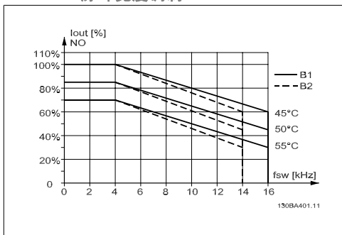
图 8.5: I_{out} 在不同 T_{AMB, MAX} 下的降容 - B 型机箱, 在正常转矩模式 (110% 过转矩) 下使用 60 PWM
