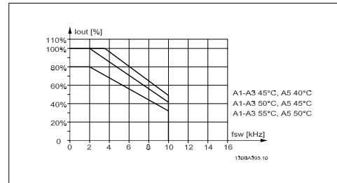
图 8.2: I_{out} 在不同 T_{AMB, MAX} 下的降容 - A 型机箱，开关模式为 SFAVM
