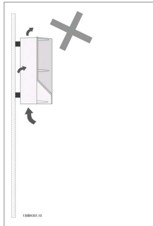
图 3.3: 在安装设备时切勿如图所示不安装背板 (A2 和 A3 机箱除外)。否则会导致冷却不充分并大大缩短设备的使用寿命。
