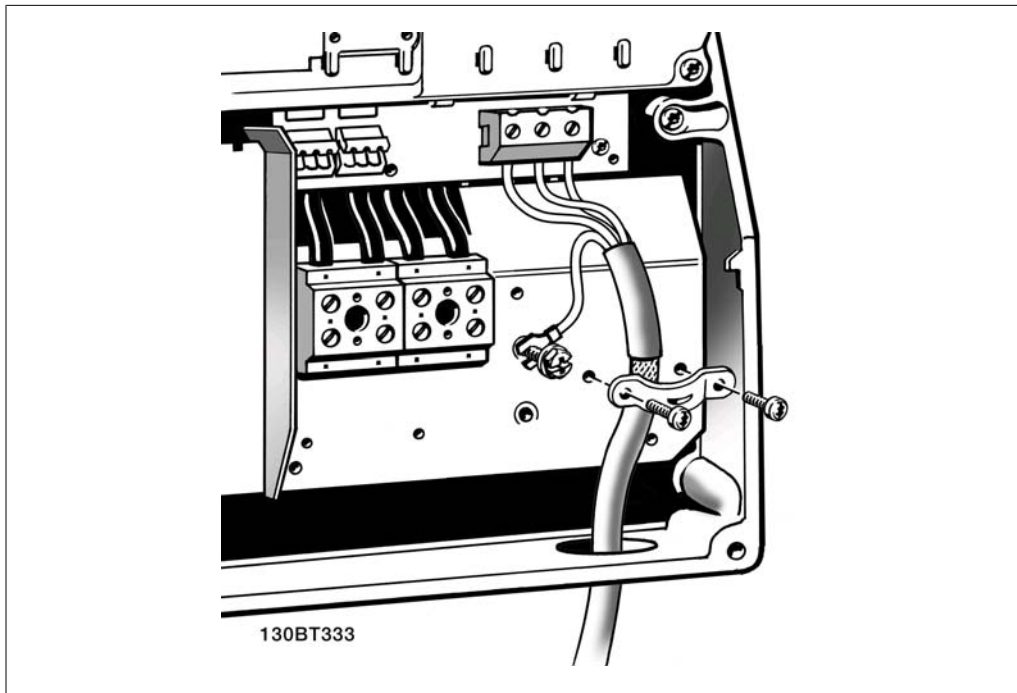
图 4.14: 首先, 断开电动机接地, 然后, 将电动机 U、V 和 W 电线接入端子并拧紧。请确保去除 EMC 电缆下面电动机电缆的外部绝缘层。
