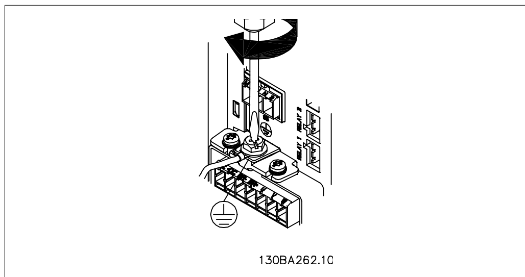
图 4.3: 安装电缆时, 首先安装并拧紧接地电线。
