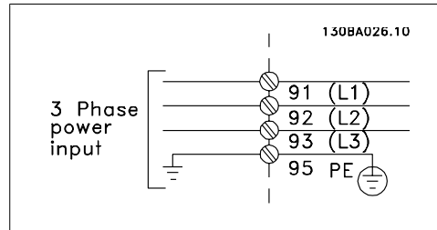
图 4.1: 主电源端子和接地端子。
