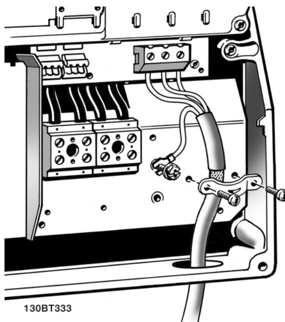
Ilustrația 4.14: Mai întâi conectați împământarea motorului, apoi introduceți în bornă firele U, V și W și strângeți-le. Asigurați-vă că izolația externă de pe cablul motorului este îndepărtată sub clema EMC.
