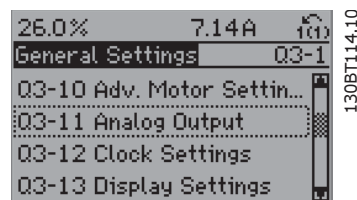
Obrázek 6.6: Krok 5: Pomocí navigačních tlačítek nahoru a dolů přejděte dolů např. na možnost 03-11 Analogové výstup . Stiskněte tlačítko [OK].
