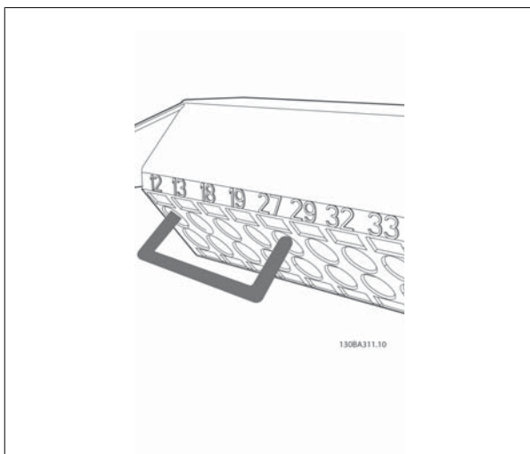
Abbildung 4.41: 3. Schritt: Stecken Sie das andere Ende in Klemme 12 oder 13. (Hinweis: dass für Geräte mit sicherer Stoppfunktion die vorhandene Brücke zwischen Klemme 12 und 37 nicht entfernt werden sollte, damit das Gerät laufen kann!)
