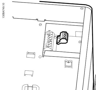
Illustration 4.37: Bornes pour le raccordement de relais pour C3 et C4. Situées dans l'angle supérieur droit du variateur de fréquence.
