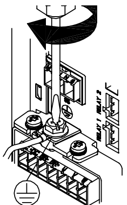
Illustration 4.4: Lors du montage des câbles, monter puis serrer le câble de terre en premier.
