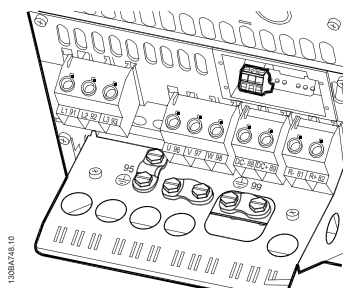
Illustration 4.36: Bornes pour le raccordement de relais pour B4.
