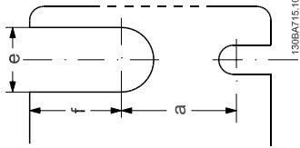
Afbeelding 3.2: Bovenste en onderste bevestigingsgaten. (alleen B4/C3/C4)
