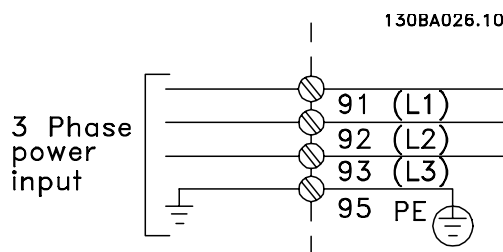
Илюстрация 4.2: Клеми за мрежата и заземяването
