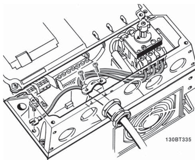
Илюстрация 4.8: Свързване към мрежата и заземяването с мрежов прекъсвач.
