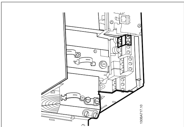
Илюстрация 4.26: Постояннотоково свързване на шината за обвивка В3.
