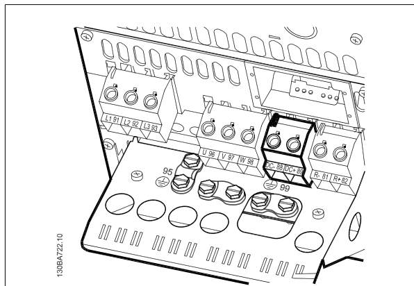
Илюстрация 4.27: Постояннотоково свързване на шината за обвивка В4.
