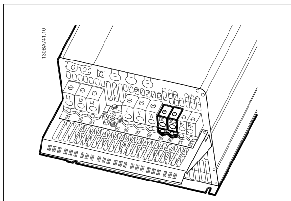
Илюстрация 4.29: Постояннотоково свързване на шината за обвивка С4.
