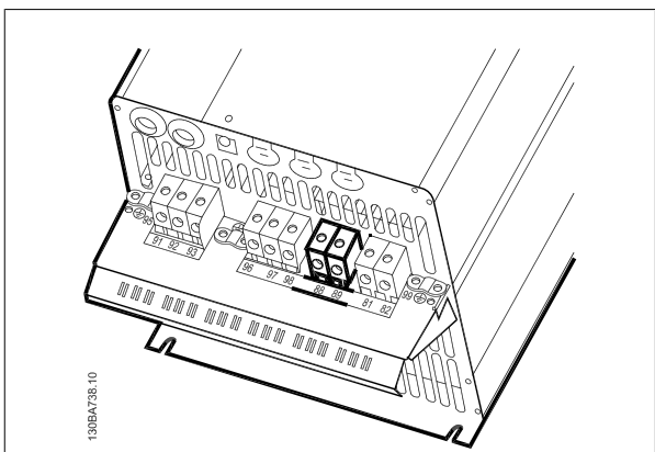
Илюстрация 4.28: Постояннотоково свързване на шината за обвивка С3.
