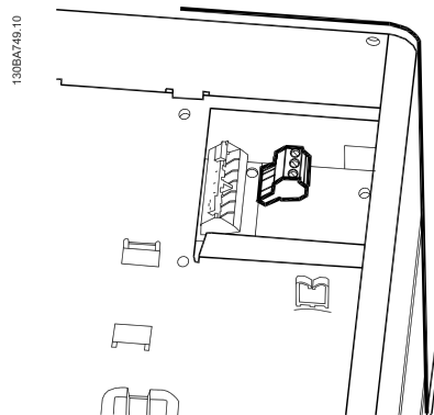
Ilustrația 4.37: Borne pentru conectările releului pentru C3 și C4. Aflate în colțul din partea dreaptă sus a convertorului de frecvență.
