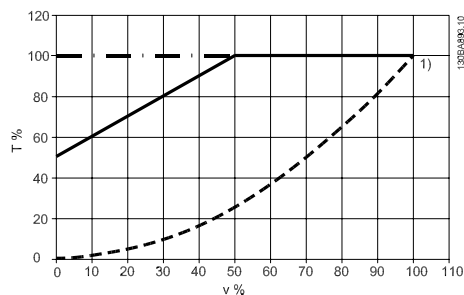
Sarcina maximă a unui motor standard la 40 °C acționat de un convertor de frecvență de tipul VLT FCxxx
