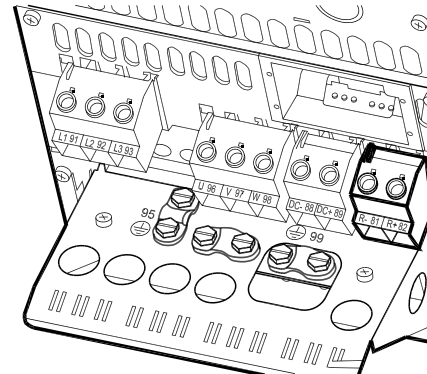
Ilustracija 4.31: Sponka za vezavo zavornega upora za B4.
