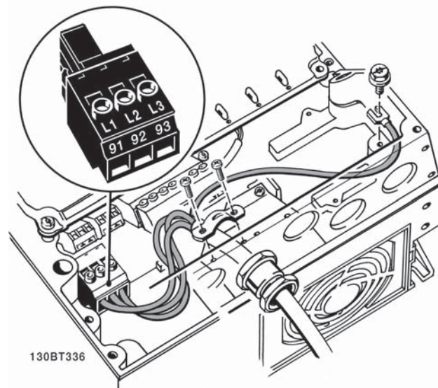
図 4.7: 主電源の断路器を使用する場合の主電源への接続と接地の方法。ケーブル・クランプを使用します。
