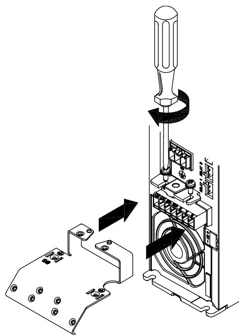
図 4.3: まず、取り付け板に 2 本のネジを取り付け、定位置までスライドしてから完全に締め付けます。
