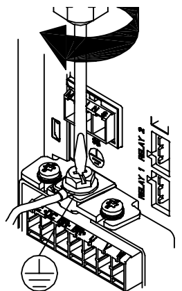
図 4.4: ケーブルを取り付けるとき、まず各ケーブルを取り付けてからそれぞれしっかり固定します。
