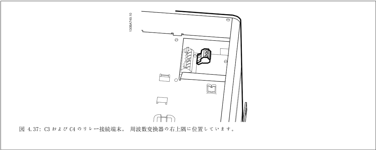
図 4.36: B4 のリレー接続用端末。
