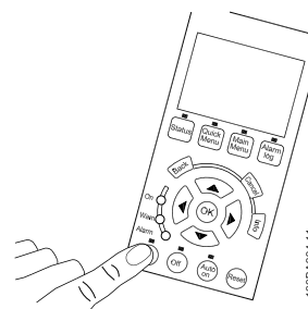
図 4.45: ステップ 5: [Hand on] ボタンを押して、ボタンの上側にある LED が点灯して、モーターが回転することを確認します。
