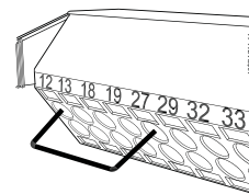
図 4.43: ステップ 3: 端末 12 と 13 の他端を挿入します。(注 意: 安全停止機能を持つユニットでは、端末 12 と 37 間 の既存のジャンパーは取り外さないでください。ユニット が稼動するために必要です。)
