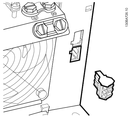
図 4.35: B3 のリレー接続用端末。工場では、ひとつのリレー入力のみ取り付けることができます。第二のリレーが必要な場合は、ノックアウトを外します。
