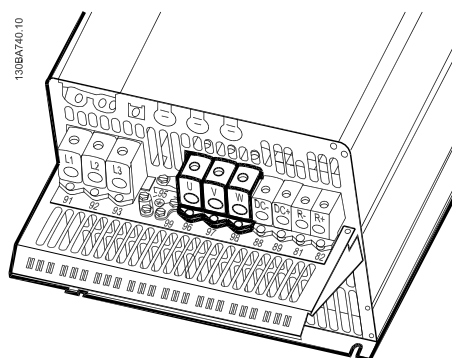
図 4.25: まずモーターの接地線を終端させ、モーターの U、V、W ワイヤを適切な端子板に取り付けて締め付けます。EMC クランプの下に来るモーター・ケーブル部分の外側の絶縁カバーが除去されていることを確認してください。
