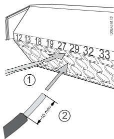
図 4.42: ステップ 2: 適切な端末用ねじ回しを使って端末 27 の一 端を挿入します。(注意: 安全停止機能を持つユニットで は、端末 12 と 37 間の既存のジャンパーは取り外さない てください。ユニットが稼動するために必要です。)
