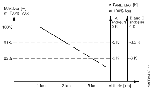
図 9.1: フレームサイズ A、B、C のための T_{AMB, MAX} における出力電流の定格値の低減。標高 2 km を超える場合の PELV については、Danfoss にお問い合わせください。
