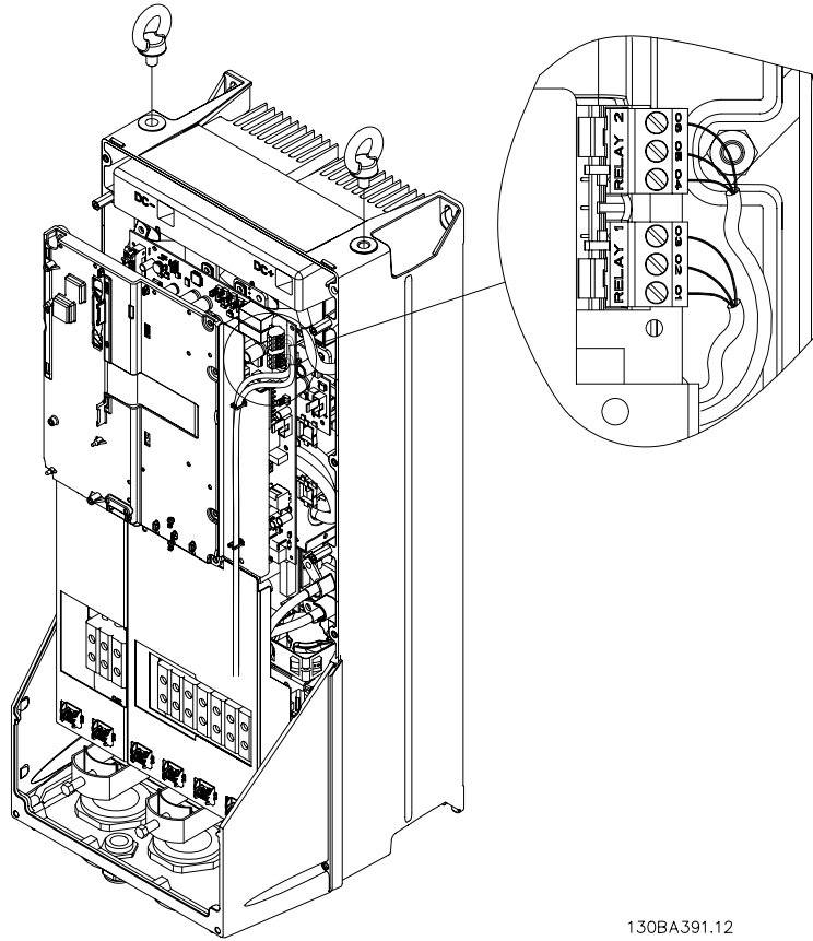
図 4.34: リレー接続用端末 C1 および C2 エンクロージャ リレー接続は、取り付けられたリレープラグ（アクセサリパックから）のカットアウトに示されます。
