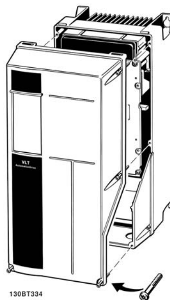
図 4.39: A5、B1、B2、C1、C2 エンクロージャのコントロール端子にアクセス
