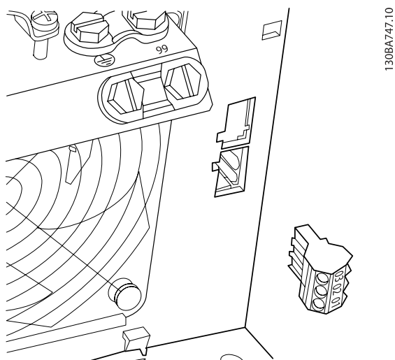
Ábra 4.35: Relécsatlakoztatás kapcsai (B3 készülékház). Gyárilag csak egy relébemenet van telepítve. Ha szükség van a második relére, távolítsa el a vaklapot.
