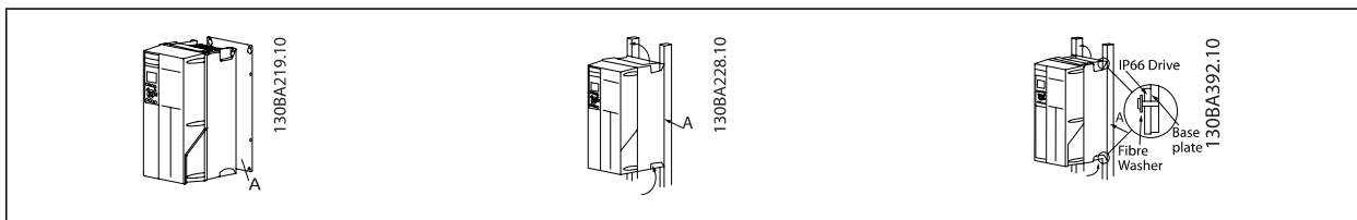
Táblázat 3.2: Ha nem tömör falra szereli az A5, B1, B2, B3, B4, C1, C2, C3 vagy C4 készülékházzal rendelkező berendezést, azt a hűtőborda elégtelen hűtőlevegője miatt A hátlappal kell ellátni.
