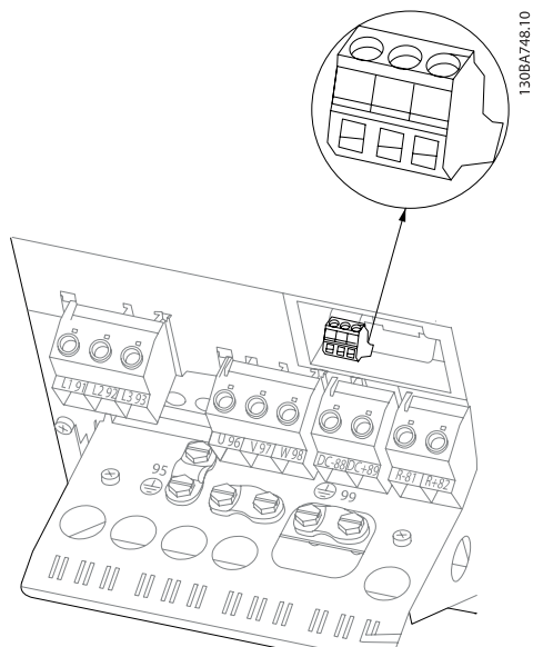
Ábra 4.36: Relécsatlakoztatás kapcsai (B4 készülékház).
