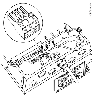
Ábra 4.19: Először csatlakoztassa a motor földelését, majd illessze a motor U, V és W vezetékét a csatlakozóba, és rögzítse őket. Ne feledje eltávolítani a motorkábel külső szigetelését az EMC-bilincs alatti részen.
