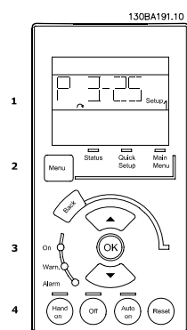
Obrázek 6.1: Numerický ovládací panel LCP (NLCP)
