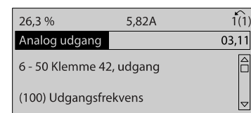
Illustration 7.6: Trin 6: Vælg par. 6-50. Tryk på [OK].
