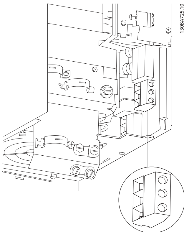
Illustration 4.10: Sådan udføres tilslutning til netforsyning og jording for B3 uden RFI.
