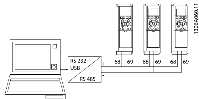
Illustration 5.2: Tilslutningseksempel.
