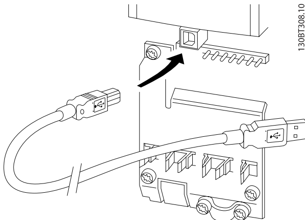
Illustration 5.3: Se afsnittet om Styreklemmer for styrekabeltilslutninger.
