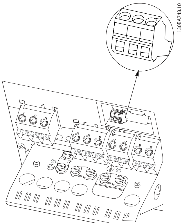
Illustration 4.30: Klemmer til relætilslutninger for B4.
