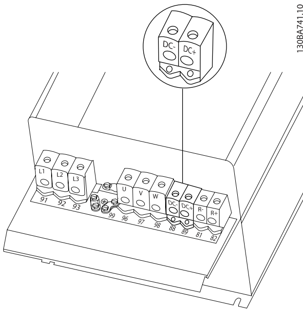
Illustration 4.23: DC-busforbindelse til kapsling C4.
