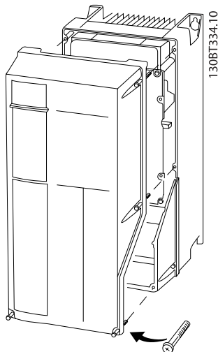
Illustration 4.33: Adgang til styreklemmerne for A4-, A5-, B1-, B2-, C1- og C2-kapslinger
