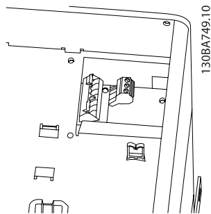
Illustration 4.31: Klemmer til relætilslutninger til C3 og C4. Placeret i frekvensomformerens øverste højre hjørne.
