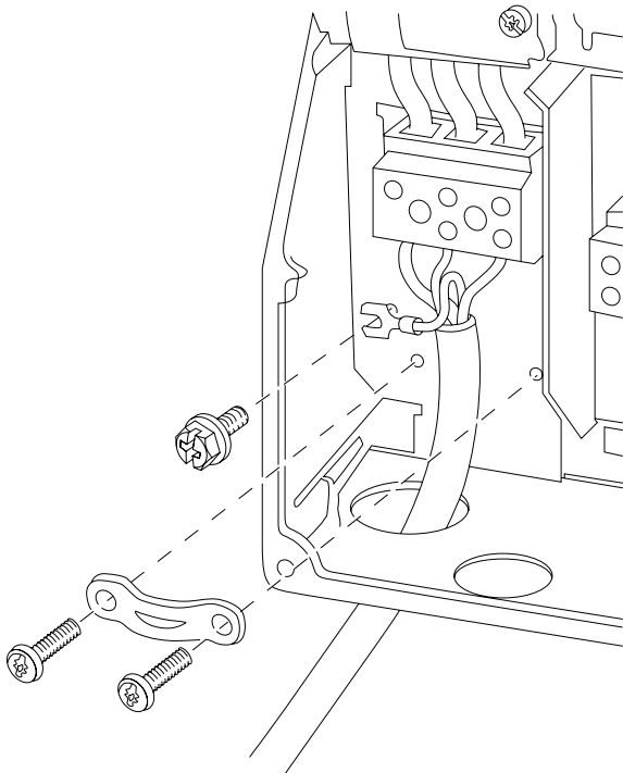
Illustration 4.9: Sådan udføres tilslutning til netforsyning og jording for B1 og B2
