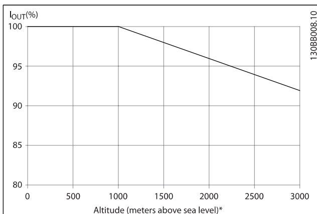
Derating af udgangsstrøm vs. højde ved TOMG, MAKS for stelstørrelser D, E og F.
