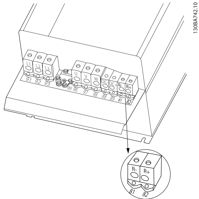
Illustration 4.27: Bremsetilslutningsklemme for C4.
