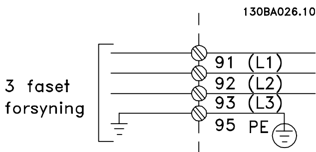
Illustration 4.2: Klemmer til net og jording.
