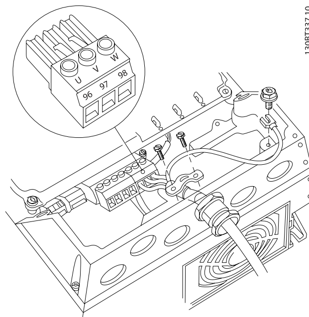
Illustration 4.19: Terminer først motorens jording, placer derefter motorens U-, V- og W-ledninger i klemmen, og spænd dem. Sørg for, at motorkablets udvendige isolering er fjernet under EMC-bøjlen.
