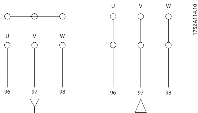
Illustration 4.16: Klemmer til motortilslutning
