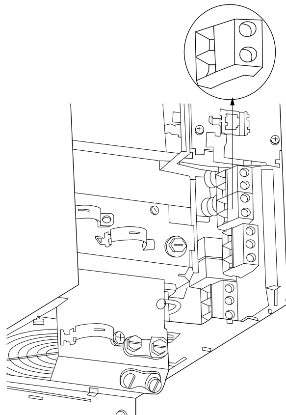
Illustration 4.24: Bremsetilslutningsklemme for B3.
