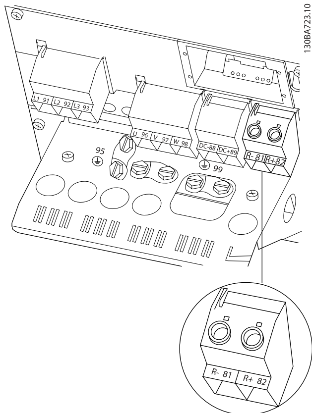
Illustration 4.25: Bremsetilslutningsklemme for B4.
