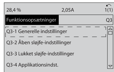
Illustration 7.4: Trin 4: Funktionsopsætningens valgmuligheder vises. Vælg Q3-1 Gen. indstillinger. Tryk på [OK].
