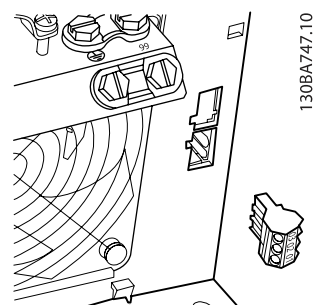
Illustration 4.29: Klemmer til relætilslutninger til B3. Der er kun installeret en relæindgang fra fabrikken. Fjern knock-out, når det andet relæ er nødvendigt.
