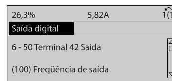
Ilustração 7.6: Etapa 6: Selecione o par. 6-50. Pressione [OK].
