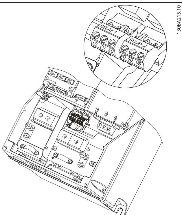
Terminais para conexão do relé ( gabinetes A4, A5, B1 e B2 ).
