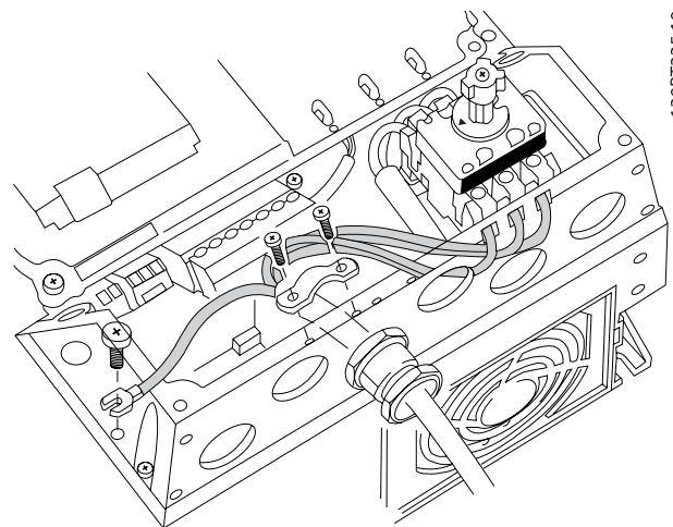
Ilustração 4.8: Como fazer a conexão à rede elétrica e ao ponto de aterramento com chave de desconexão.
