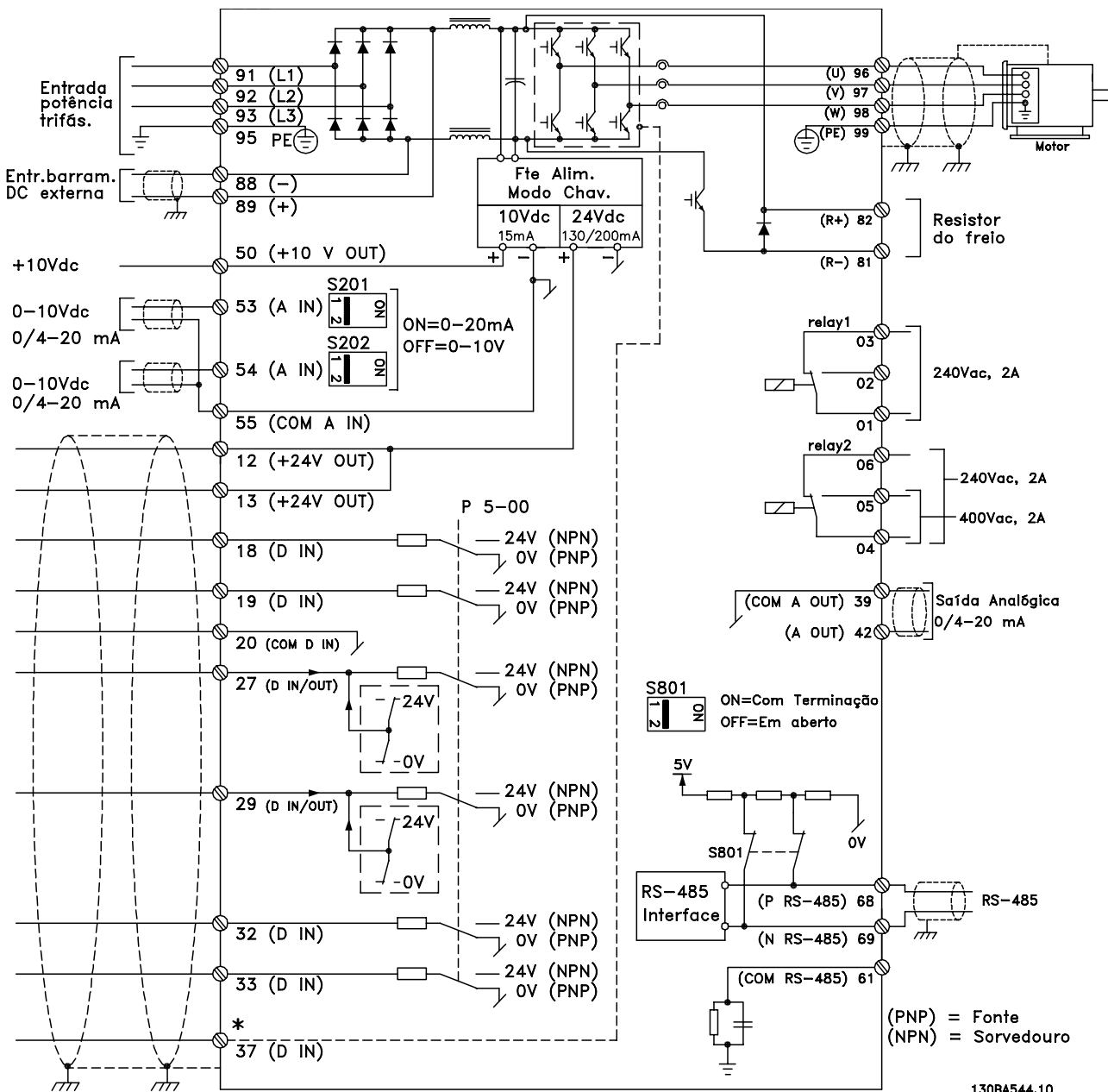
Ilustração 4.1: Diagrama exibindo todos os terminais elétricos. (O terminal 37 estará instalado somente nas unidades com a Função Parada Segura.)
