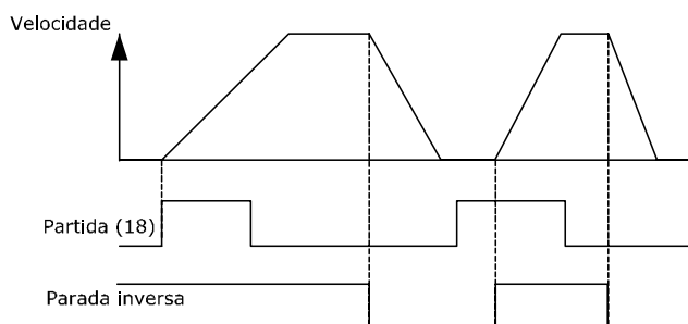
Ilustração 5.5: Terminal 37: Disponível somente com a Função de Parada Segura!
