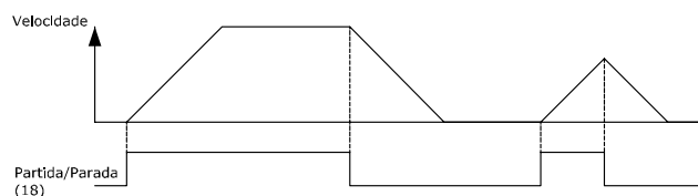
Ilustração 5.4: Terminal 37: Disponível somente com a Função de Parada Segura!
