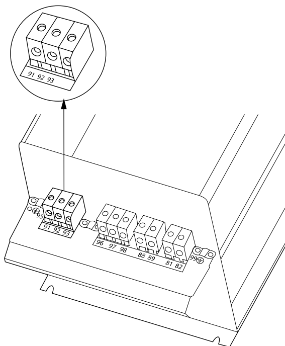
Ilustração 4.14: Como conectar o C3 à rede elétrica e ao ponto de aterramento.
