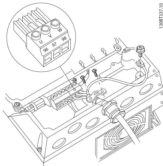
Ilustração 4.19: Primeiro, faça a terminação do terra do motor, em seguida, instale os fios U,V e W no terminal e aperte. Garanta que a isolação externa do cabo do sob a braçadeira de EMC seja removida.
