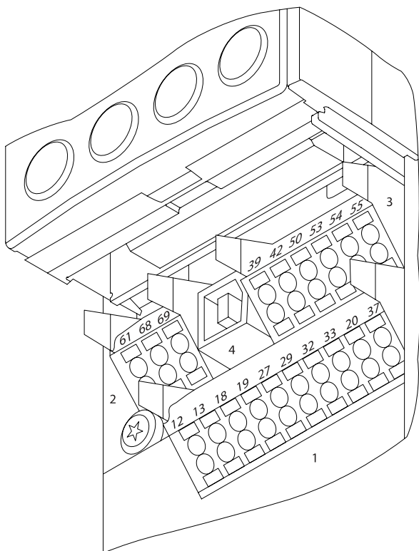
Ilustração 4.34: Terminais de controle (todos os gabinetes)
