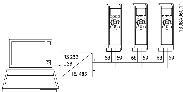
Ilustração 5.2: Exemplo de conexão.
