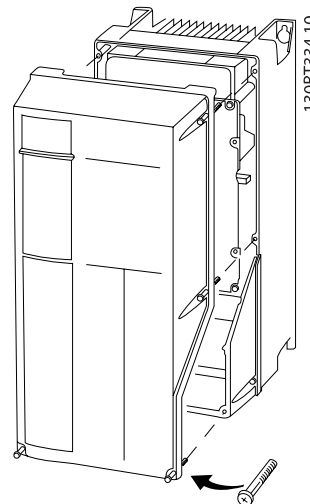
Ilustração 4.33: Acesso aos terminais de controle dos gabinetes metálicos A4, A5, B1, B2, C1 e C2
