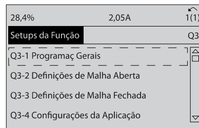
Ilustração 7.4: Passo 4: As opções de Setups de função são exibidas. Selecione Q3-1 Configurações Gerais . Pressione [OK]
