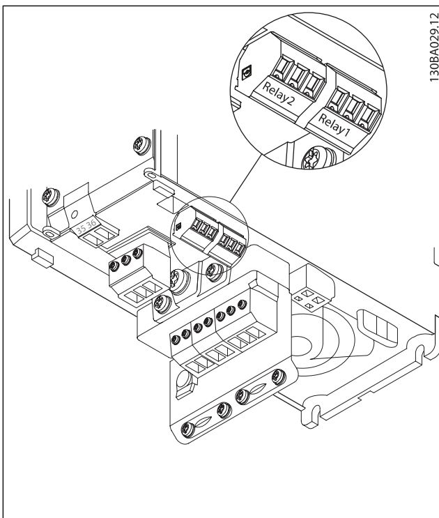
Terminais para conexão do relé (gabinetes metálicos A2 e A3).
