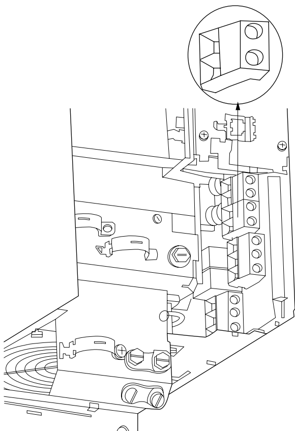
Ilustração 4.24: Terminal de conexão do freio para o B3.
