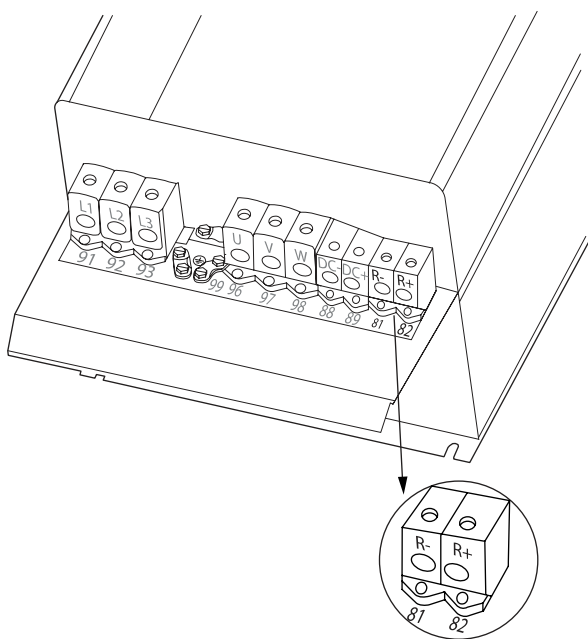
Ilustração 4.27: Terminal de conexão do freio para o C4.
