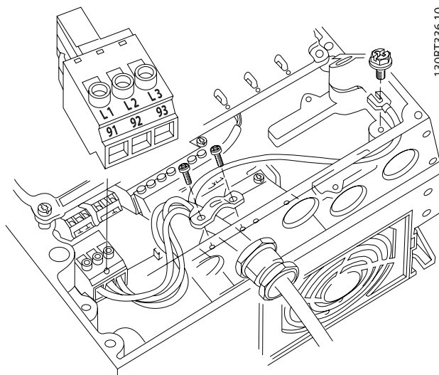
Ilustração 4.7: Como fazer a conexão à rede elétrica e ao ponto de aterramento, sem a de chaveamento de desconexão da rede elétrica. Observe que é utilizada uma braçadeira de cabo.
