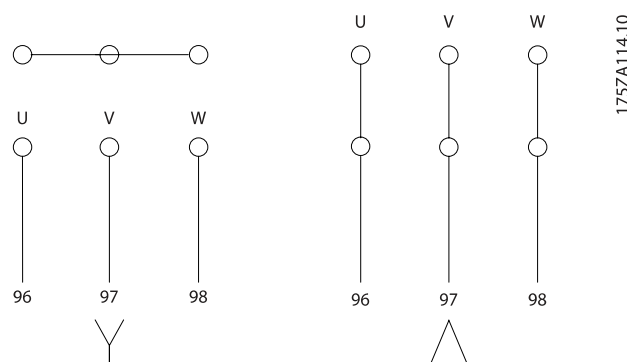
Ilustração 4.16: Terminais para conexão do motor
