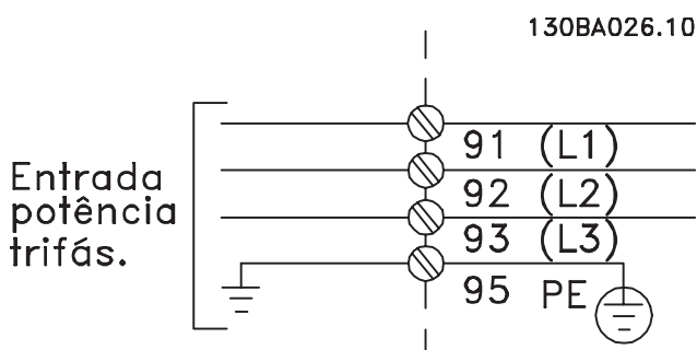
Ilustração 4.2: Terminais para rede elétrica e aterramento
