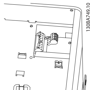
Ilustração 4.31: Terminais para conexão do relé do C3 e C4. Localiza-se no canto superior direito do conversor de frequência.
