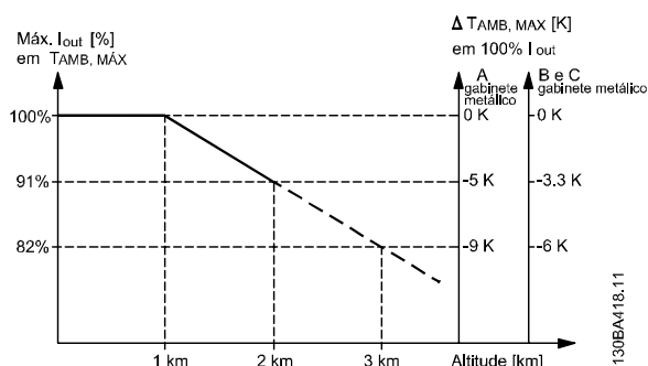
Ilustração 9.1: Derating da corrente de saída versus altitude na T_{AMB, MAX} para os chassis de tamanhos A, B e C. Para altitudes acima de 2 km, entre em contacto com a Danfoss em relação à PELV.
