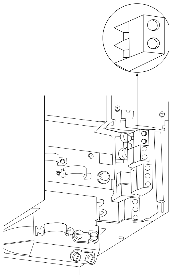
Ilustração 4.20: Conexões do barramento CC para o gabinete metálico B3..
