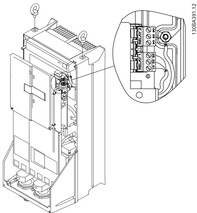
Ilustração 4.28: Terminais para conexão do relé (gabinetes C1 e C2). As conexões do relé são mostradas no desenho em corte com os plugues de relé (da Sacola de Acessórios) instalados.
