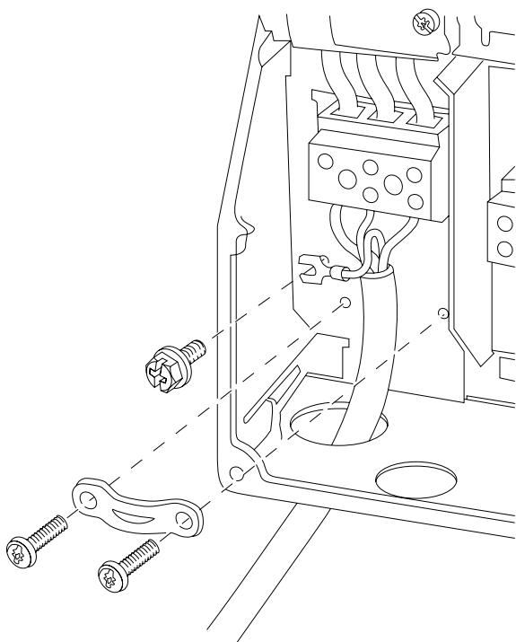
Ilustração 4.9: Como fazer a conexão na rede elétrica e no ponto de aterramento dos gabinetes metálicos B1 e B2
