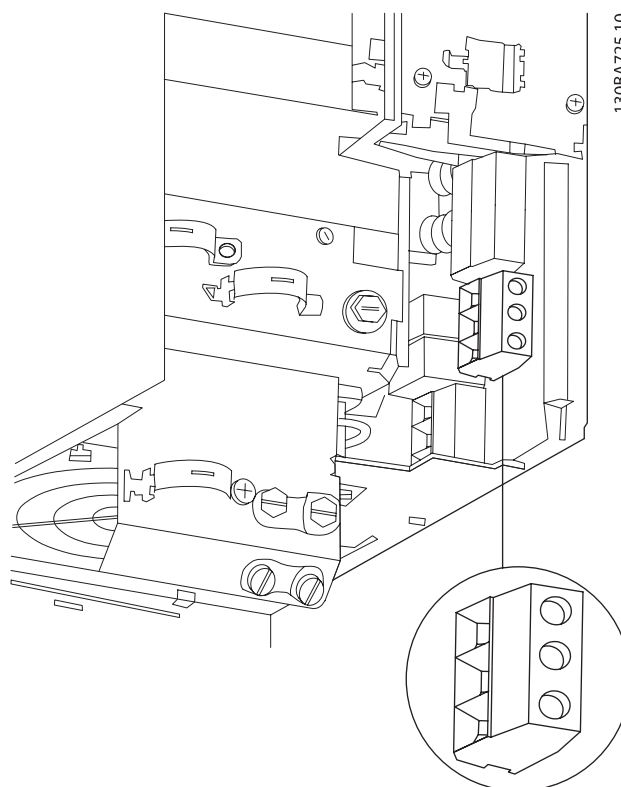
Ilustração 4.10: Como fazer a conexão na rede e no ponto de aterramento do B3 sem o RFI.
