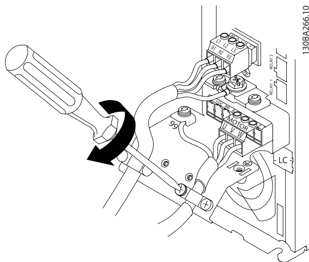
Ilustração 4.18: Monte a braçadeira de cabo, para assegurar conexão 360 graus entre o chassi e a tela, observe que a isolação externa do cabo, sob a braçadeira, está removida.
