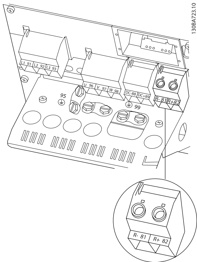
图 4.25: B4 的制动连接端子。
