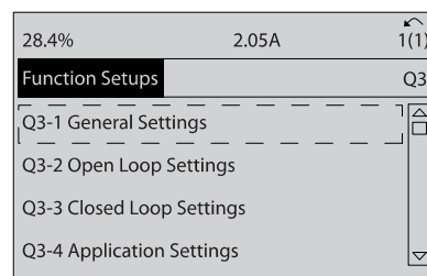
图 7.4: 步骤 4: 功能设置选项随即显示。选择 Q3-1 一般设置。按 [OK] (确定)。
