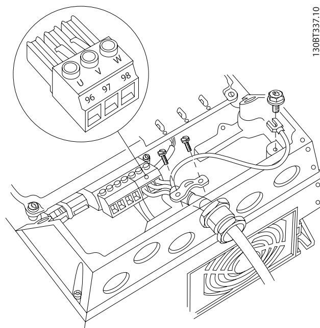
图 4.19: 首先端接电动机地线, 然后将电动机的 U、V 和 W 电线接入端子并拧紧。请确保去除 EMC 电缆夹下面电动机电缆的外部绝缘层。
