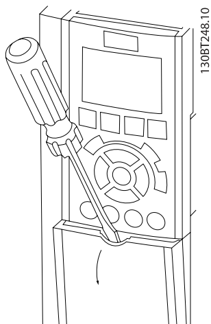
图 4.32: 访问 A2、A3、B3、B4、C3 和 C4 机箱的控制端子
