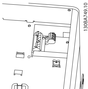
图 4.31: C3 和 C4 的继电器连接端子。位于变频器的右上角。
