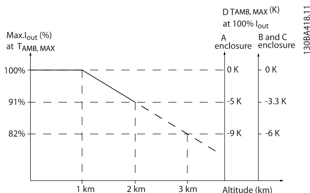
图 9.1: 在 T_{AMB, MAX} 下，输出电流降容与海拔的关系（机架规格 A、B 和 C）。当海拔超过 2 km 时，请向 Danfoss 咨询 PELV 事宜。
