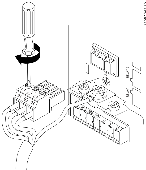
图 4.5: 然后, 安装主电源插头并拧紧电线。
