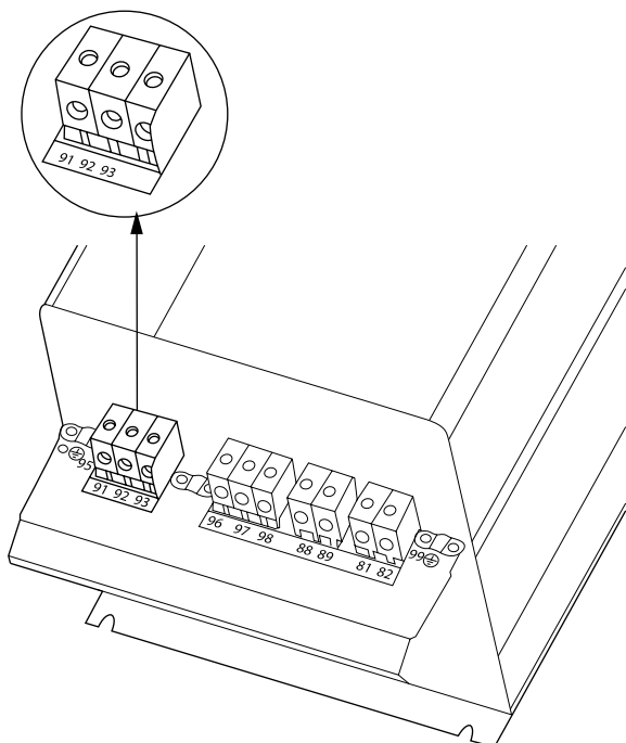
图 4.14: 如何为 C3 连接主电源和接地。
