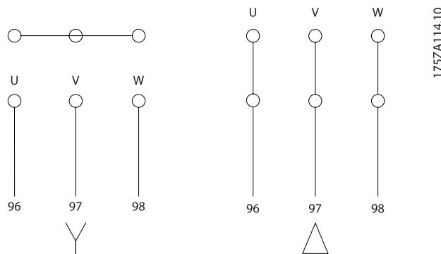
图 4.16: 电动机连接端子
