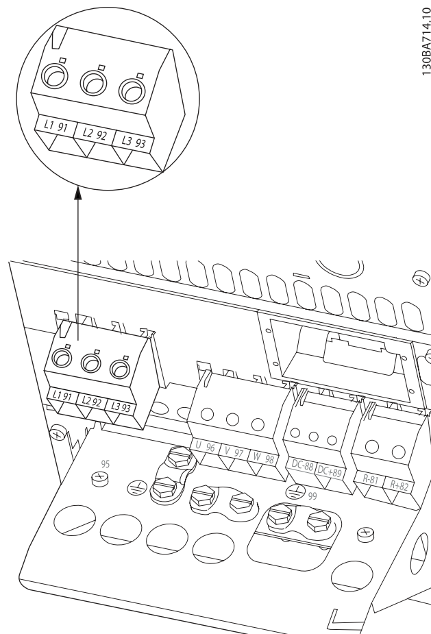
图 4.12: 如何为 B4 连接主电源和接地。
