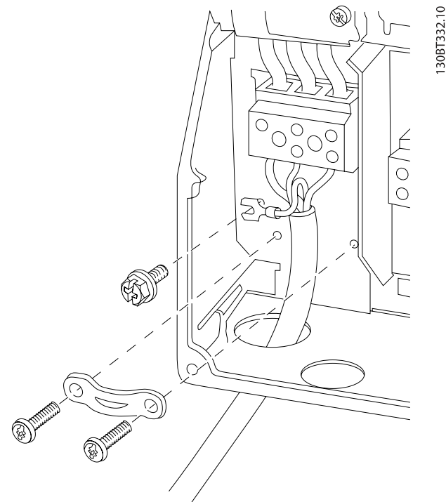
图 4.9: 如何为 B1 和 B2 连接主电源和接地
