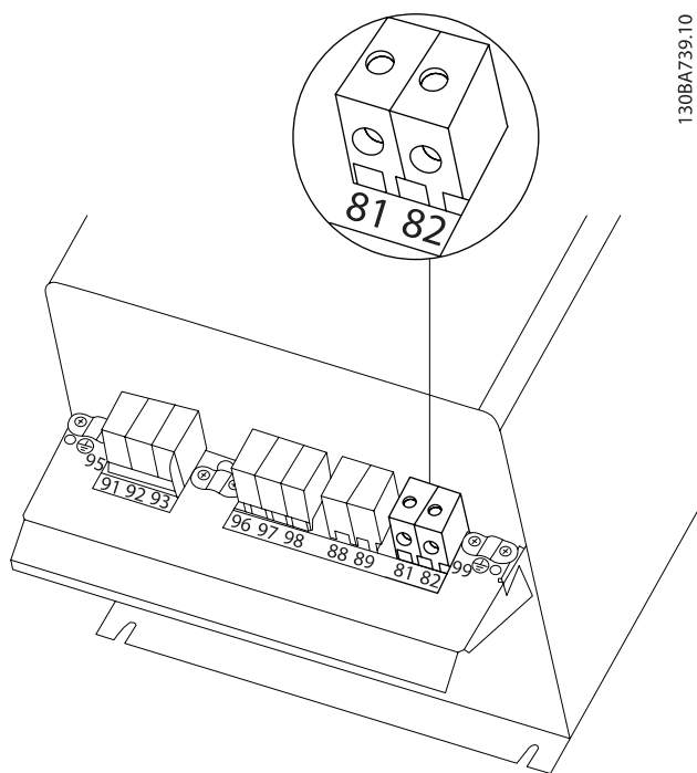
图 4.26: C3 的制动连接端子。
