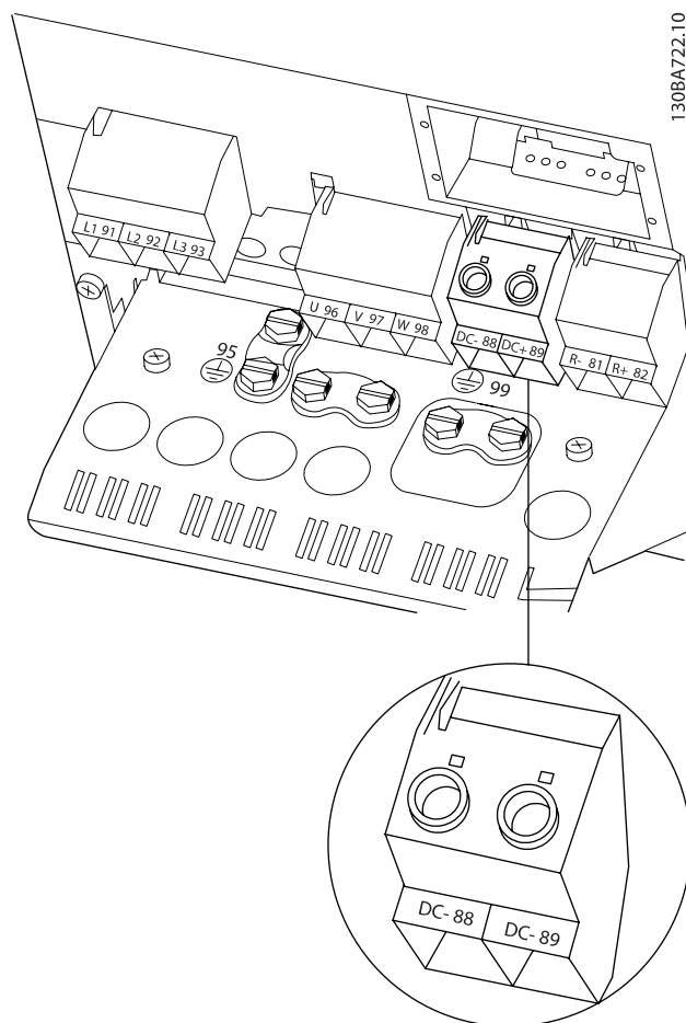
图 4.21: 机箱 B4 的直流总线连接。
