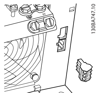
图 4.29: B3 的继电器连接端子。出厂时仅配备一个继电器输入。 如果需要另外的继电器, 请拆除挡板。
