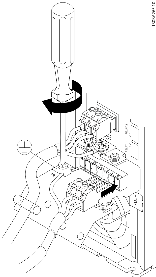
图 4.17: 首先, 断开电动机接地, 然后, 将电动机 U、V 和 W 电线插入插头并拧紧。
