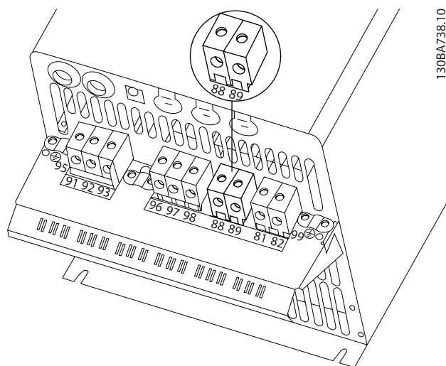
图 4.22: 机箱 C3 的直流总线连接。
