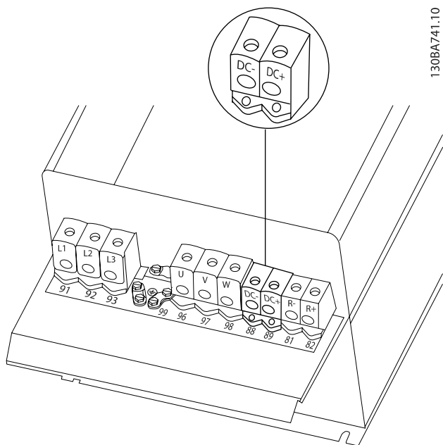
图 4.23: 机箱 C4 的直流总线连接。
