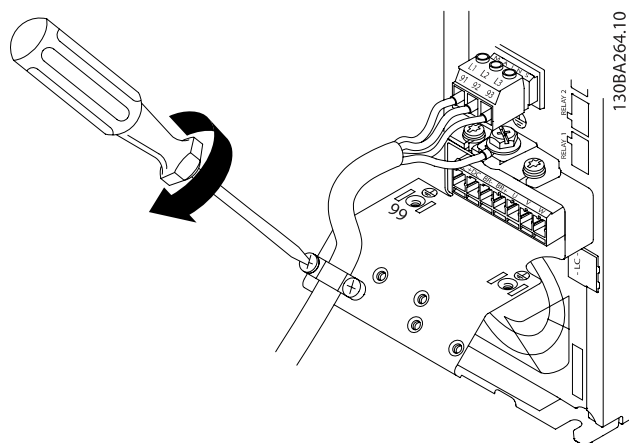
图 4.6: 最后, 拧紧主电源电线的支持架。
