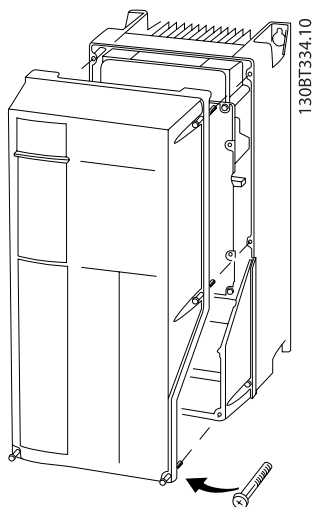
图 4.33: 访问 A4、A5、B1、B2、C1 和 C2 机箱的控制端子
