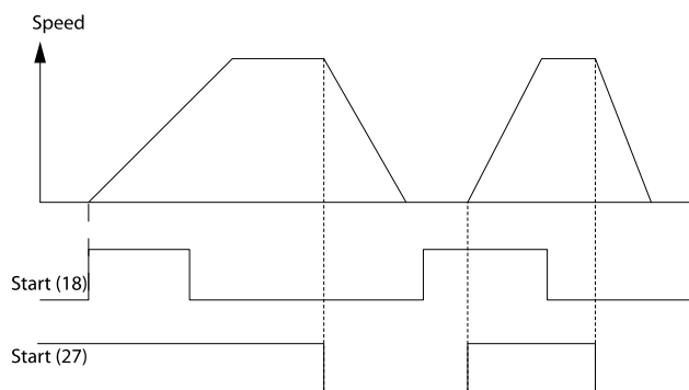
图 5.5: 端子 37: 仅随安全停止功能一起提供!
