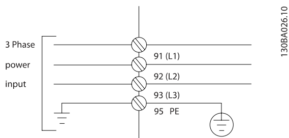
图 4.2: 主电源端子和接地端子。
