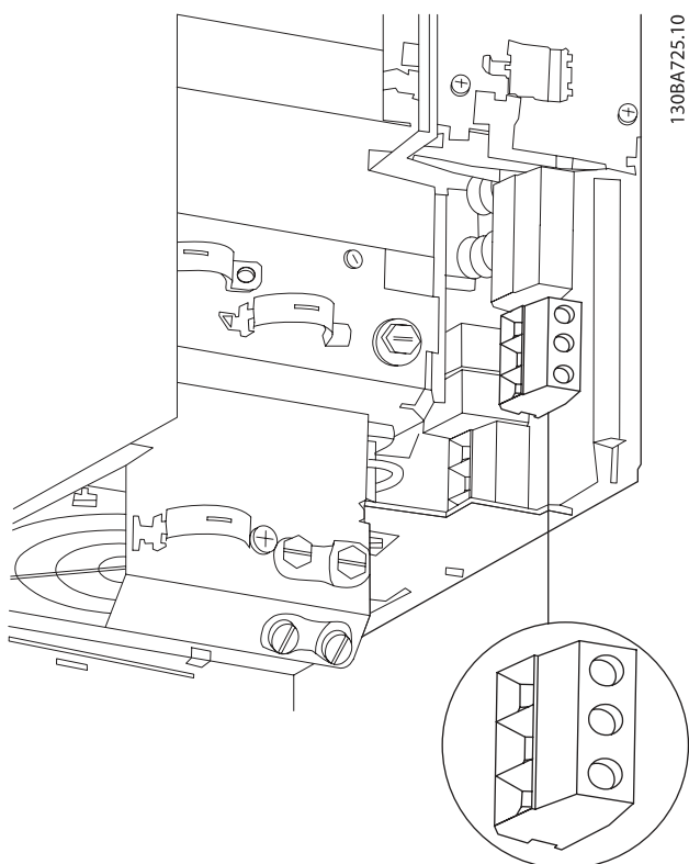
图 4.10: 如何为不带 RFI 的 B3 连接主电源和接地。
