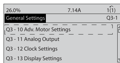
图 7.5: 步骤 5: 使用向上/向下导航键向下滚动到目标选项, 比如 Q3-11 模拟输出。按 [OK] (确定)。
