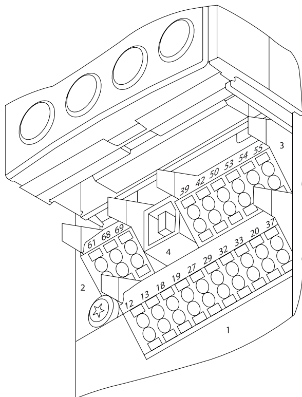
图 4.34: 控制端子 (所有机箱)
