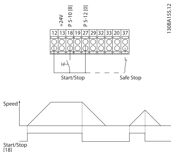
图 5.4：端子 37： 仅随安全停止功能一起提供！
