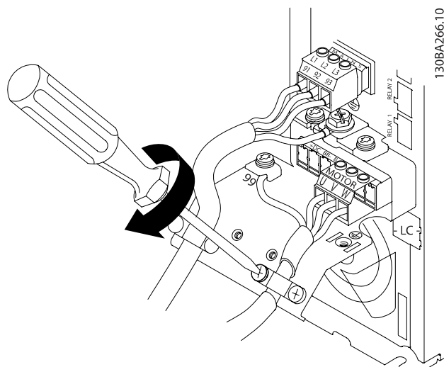
图 4.18: 安装电缆夹, 以确保机架和屏蔽丝网达到 360 度连接。注意, 请去除电缆夹下面电动机电缆的外部绝缘层。
