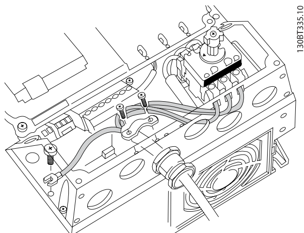
图 4.8: 如何使用主电源断路器连接主电源和接地。
