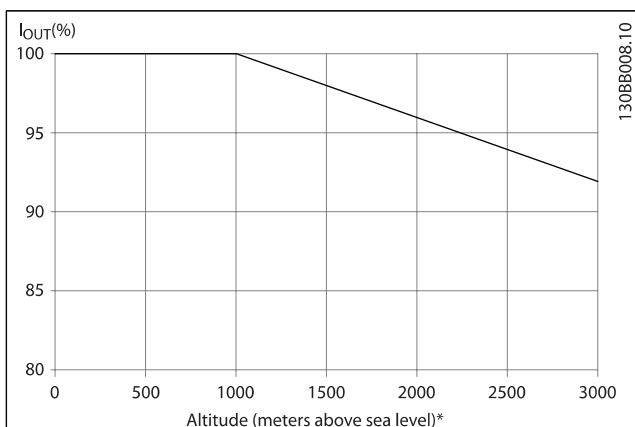
在 T_{AMB, MAX} 下，输出电流降容与海拔的关系（机架规格 D、E 和 F）。
