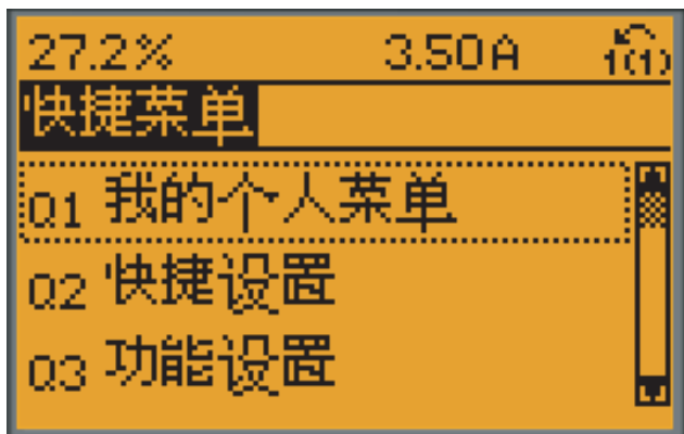
130BP064.11 图 5.1: 快捷菜单视图。
