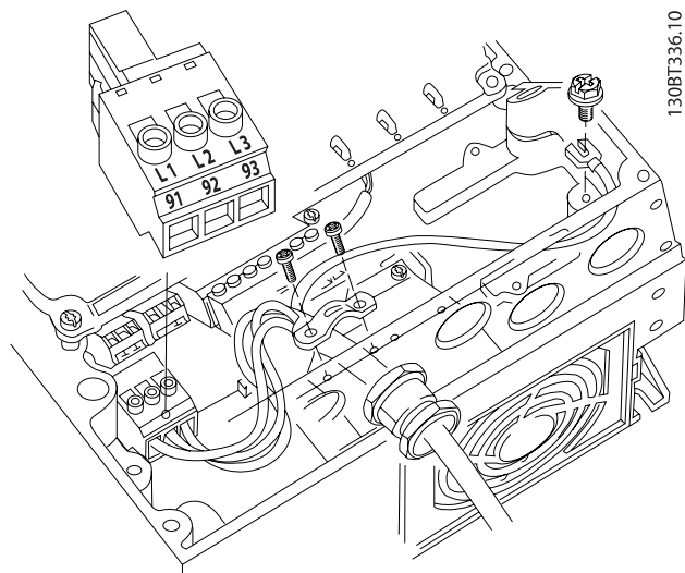
图 4.7: 如何在不使用主电源断路器的情况下连接主电源和接地。注意, 需要使用电缆夹。
