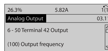
图 7.6: 步骤 6: 选择参数 6-50。按 [OK] (确定)。
