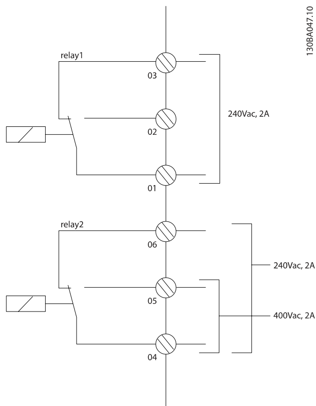
图 4.31: C3 和 C4 的继电器连接端子。位于变频器的右上角。
