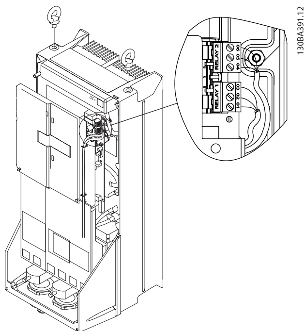
图 4.28: 继电器连接端子 (C1 和 C2 机箱)。 显示的继电器连接位于安装有继电器插头 (位于附件包中) 的断开中。
