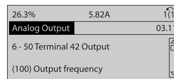
Илюстрация 7.6: Стъпка 6: Изберете пар. 6-50. Натиснете [OK].
