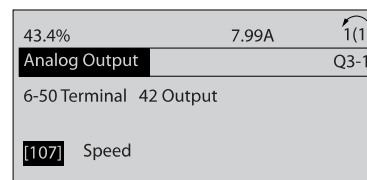
Илюстрация 7.7: Стъпка 7: Използвайте бутоните за навигация нагоре/надолу, за да изберете от различните възможности. Натиснете [OK].
