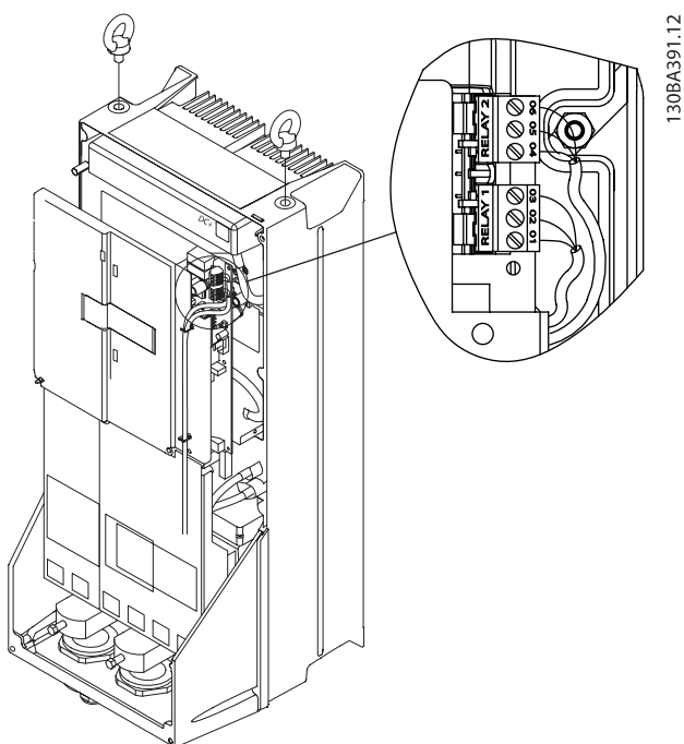
Илюстрация 4.28: Клеми за релейна връзка (обвивки C1 и C2). Релейните връзки се показват в сечението с включени релейни куплунги (от плика с принадлежности).
