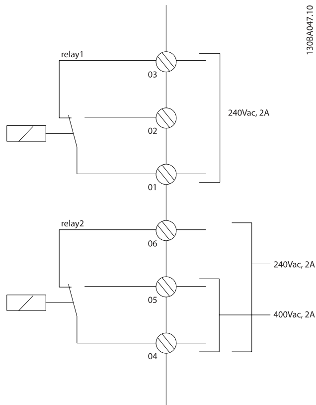
Илюстрация 4.31: Клеми за релейни връзки за C3 и C4. Намират се в горния ляв ъгъл на честотния преобразувател.
