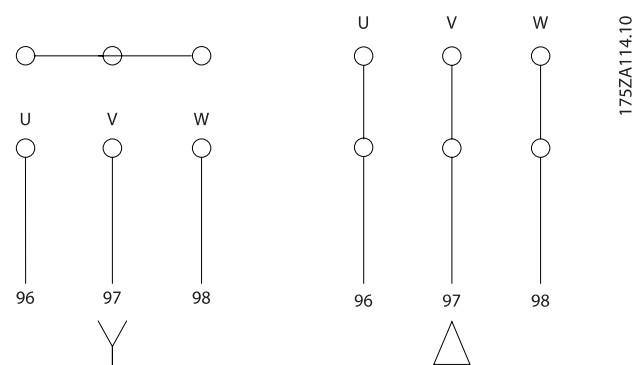
Илюстрация 4.16: Клеми за свързване на електродвигателя
