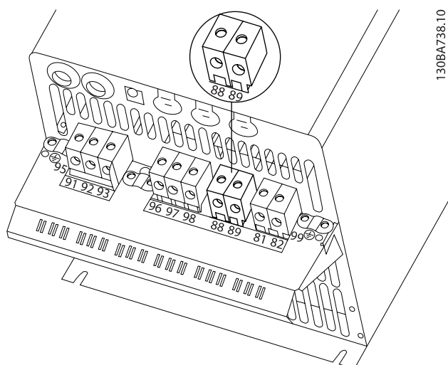
Илюстрация 4.22: Постояннотоково свързване на шината за обвивка С3.
