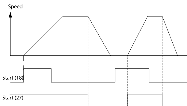
Илюстрация 5.5: Клема 37: Налична само с функция безопасен стоп!
