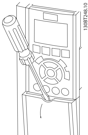
Илюстрация 4.32: Достъп до клемите на управлението за обвивки A2, A3, B3, B4, C3 и C4
