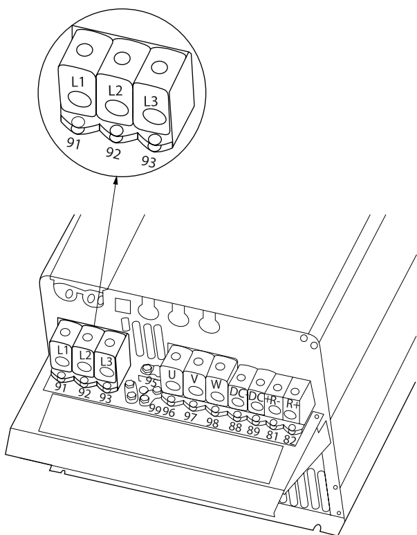
Илюстрация 4.15: Свързване на С4 с мрежа и земя.
