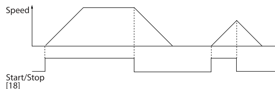
Илюстрация 5.4: Клема 37: Налична само с функция безопасен стоп!
