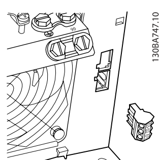
Илюстрация 4.29: Клеми за релейни връзки за В3. Фабрично е монтиран само един релейен вход. Когато е необходимо второ реле, премахнете избутвача.
