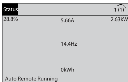
Илюстрация 7.1: Стъпка 1: Включете честотния преобразувател (жълтият светодиоден индикатор светва)
