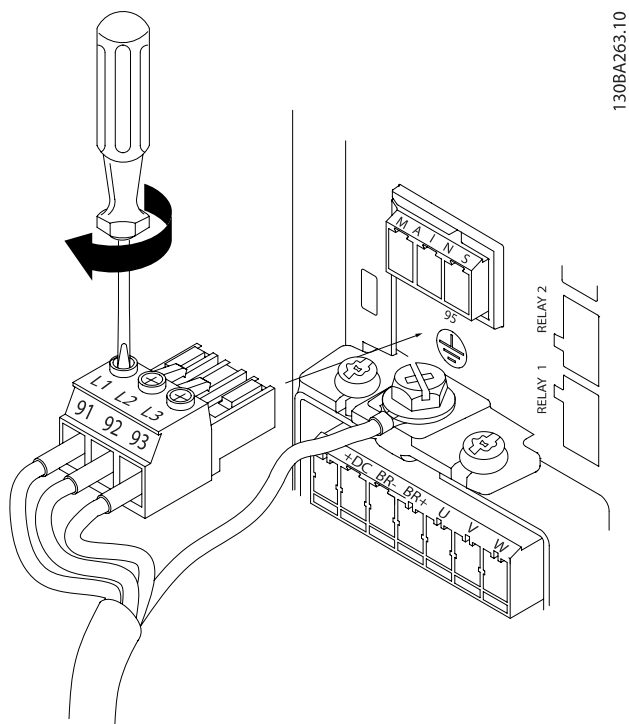
Илюстрация 4.5: След това монтирайте мрежовия щепсел и затегнете проводниците.
