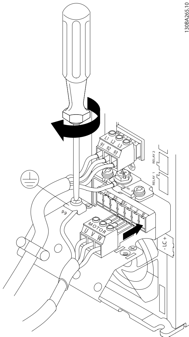
Илюстрация 4.17: Първо прекъснете заземяването на електродвигателя, след това поставете проводници U, V и W в клемата и затегнете.
