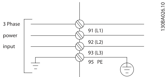
Илюстрация 4.2: Клеми за мрежата и заземяването
