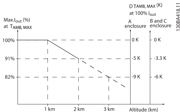
Илюстрация 9.1: Занижение на номиналните данни на изходния ток срещу височината на T_{AMB, MAX} за размери на рамката A, B и C. При надморска височина над 2 км, моля, свържете се с Danfoss относно PELV.
