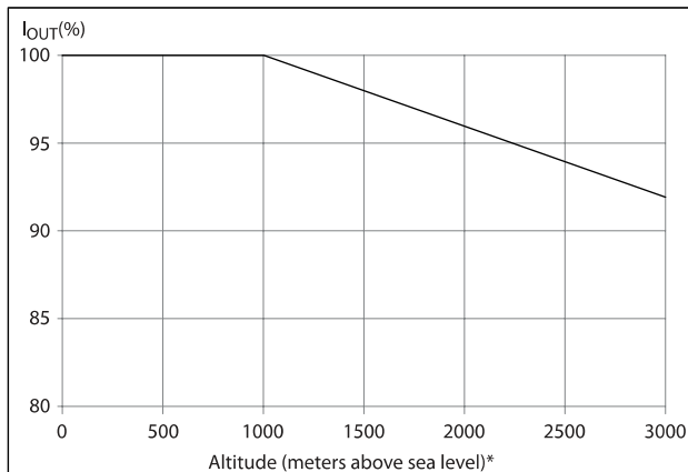
Занижение на номиналните данни на изходния ток срещу височината на T_{AMB, MAX} за размери на рамката D, E и F.
