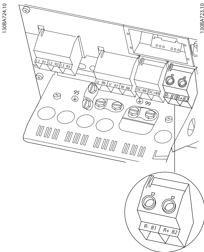
Илюстрация 4.25: Клема за свързване на спирачката за V4.
