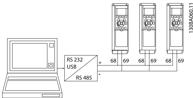
Илюстрация 5.2: Пример за свързване.
