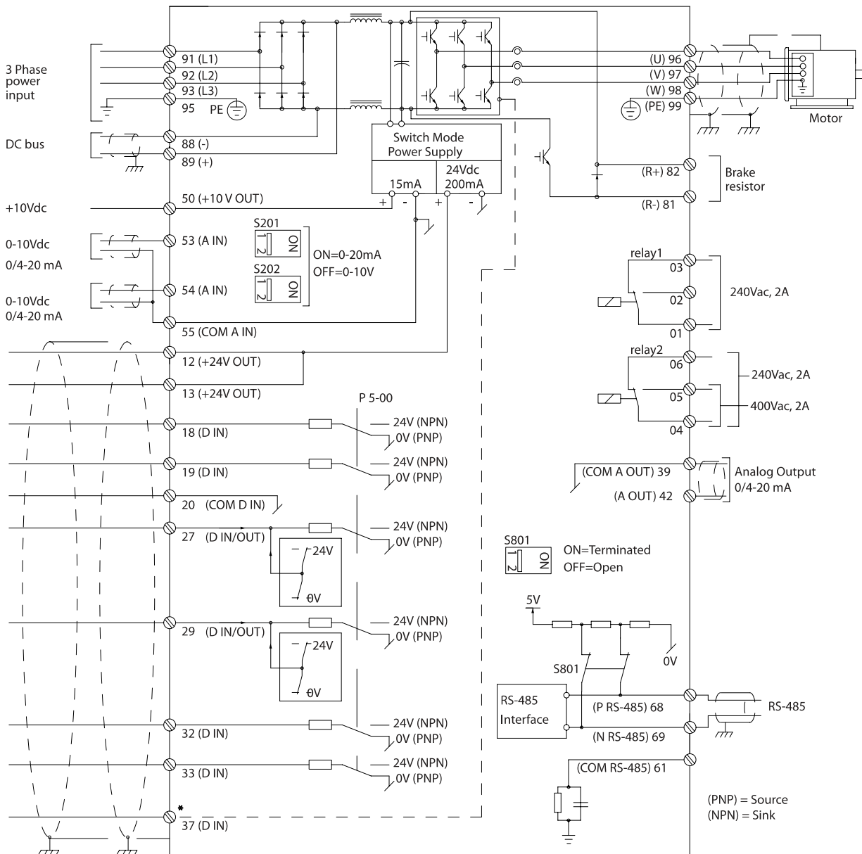
Илюстрация 4.1: Схема, показваща всички електрически клеми. (Клема 37 присъства само за устройства с функция безопасен стоп.)
