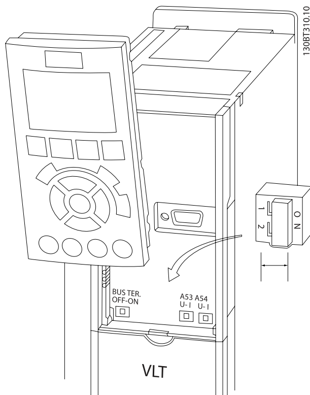
Илюстрация 4.44: Място на превключвателите.
