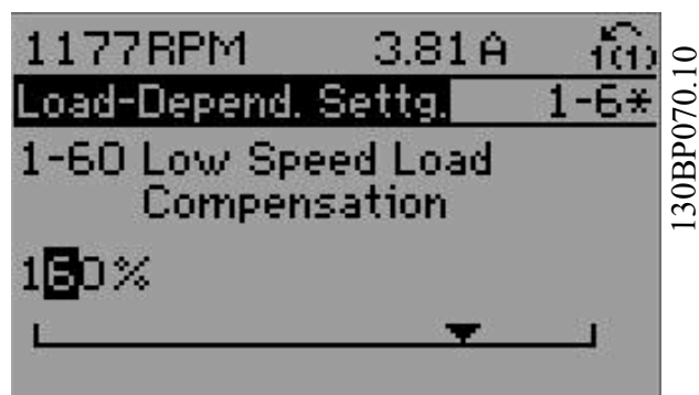
Илюстрация 7.11: Пример за показване на дисплея.
