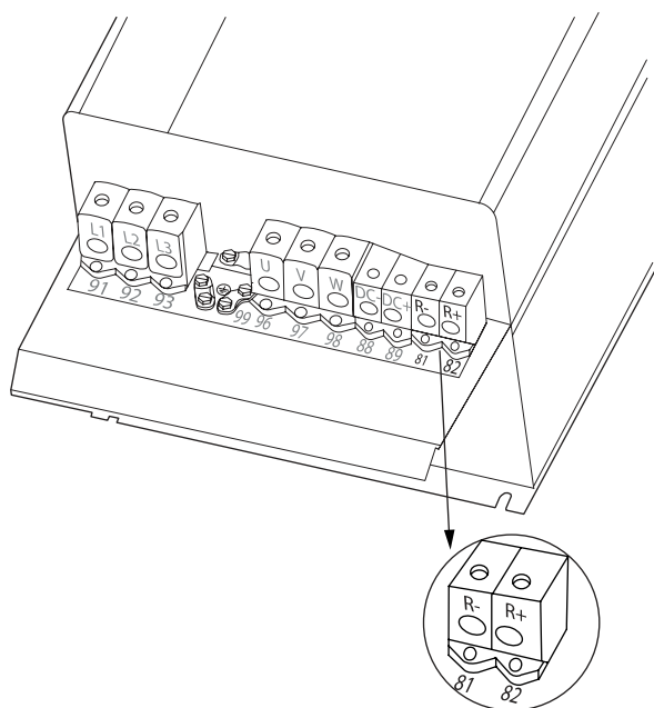
Илюстрация 4.27: Клема за свързване на спирачката за С4.
