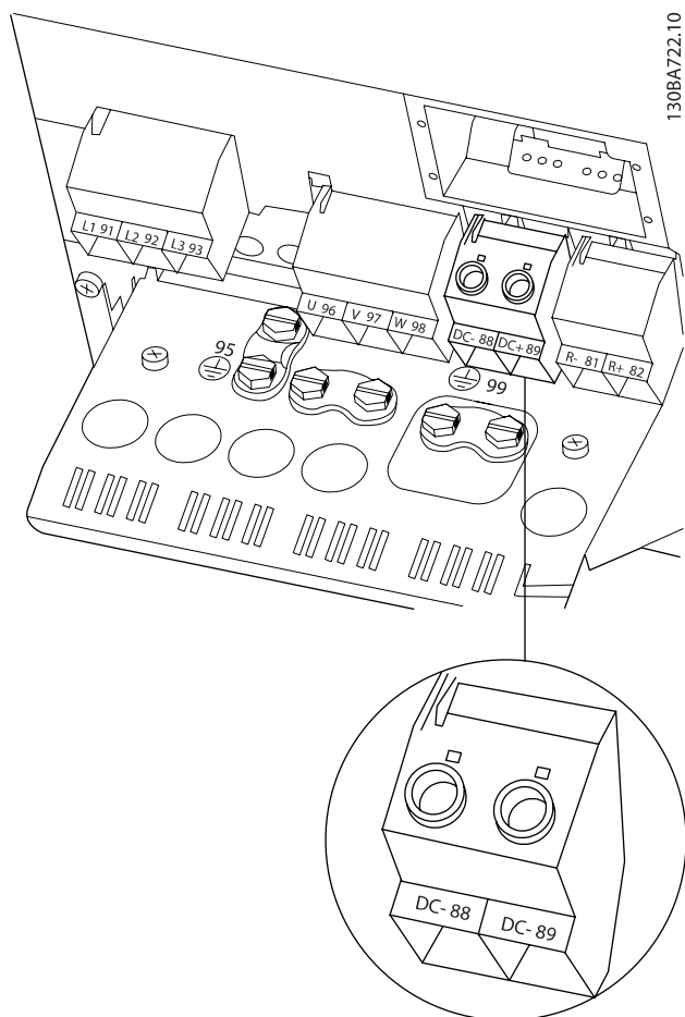
Илюстрация 4.21: Постояннотоково свързване на шината за обвивка В4.
