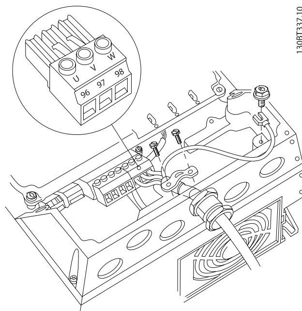
Илюстрация 4.19: Първо прекъснете заземяването на електродвигателя, след това пхнете проводници U, V и W в клемата и затегнете. Проверете дали външната изолация на кабела на електродвигателя под EMC скобата е махната.
