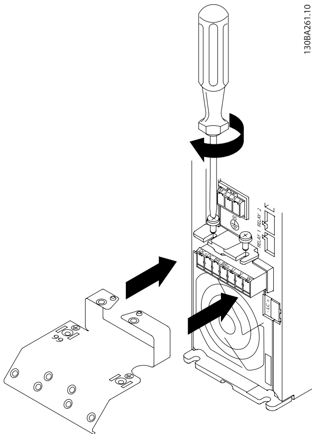
Илюстрация 4.3: Първо поставете двата винта в монтажната пластина, плъзнете я на място и затегнете докрай.
