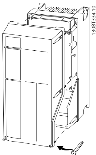
Илюстрация 4.33: Достъп до клемите на управлението за обвивки A4, A5, B1, B2, C1 и C2
