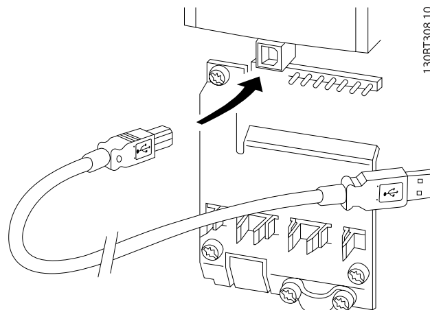
Илюстрация 5.3: За свързването на кабелите за управление вижте раздела за Клемите на управлението .
