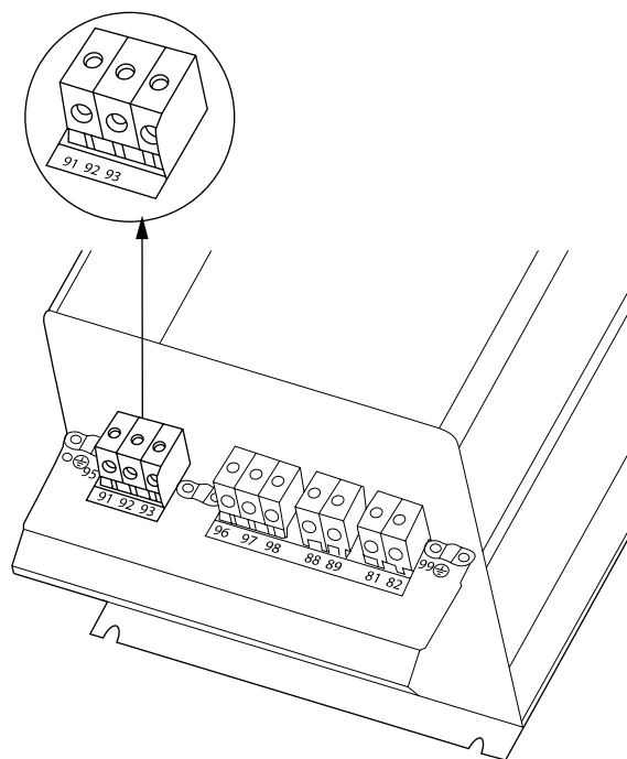
Илюстрация 4.14: Свързване на С3 с мрежа и земя.
