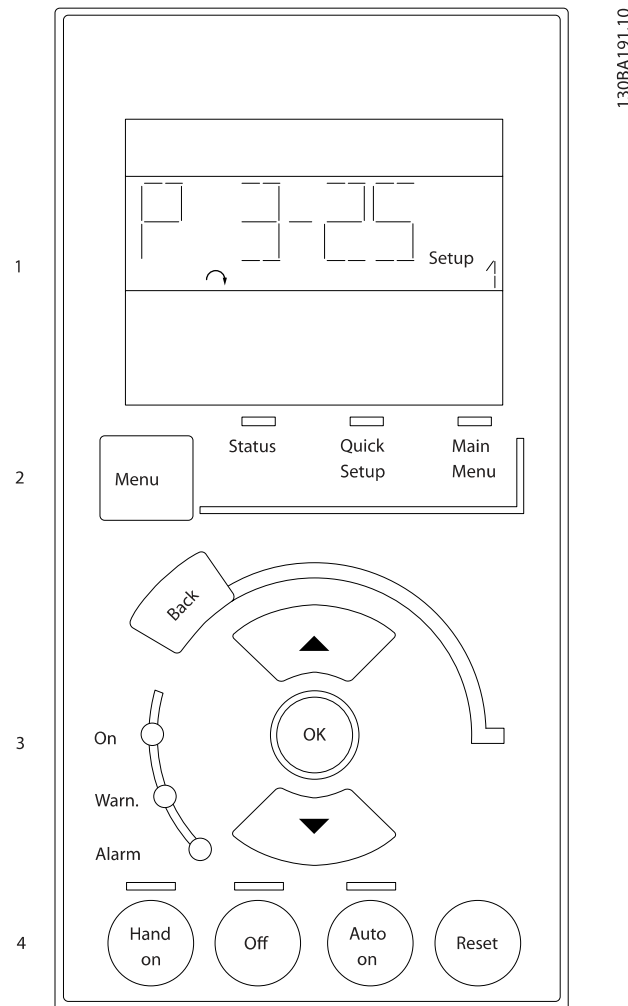
Илюстрация 6.1: Цифров LCP (NLCP)
