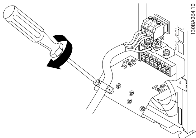
Илюстрация 4.6: Накрая затегнете скобата за закрепване върху мрежовите проводници.
