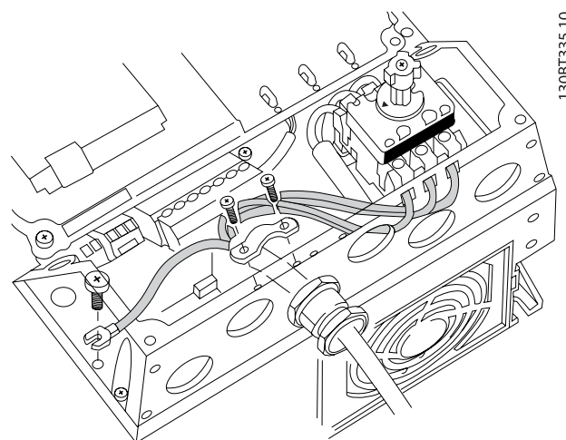
Илюстрация 4.8: Свързване към мрежата и заземяването с мрежов прекъсвач.
