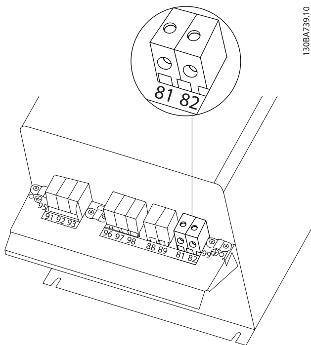
Ilustracja 4.26: Zacisk podłączenia rezystora hamowania dla C3.
