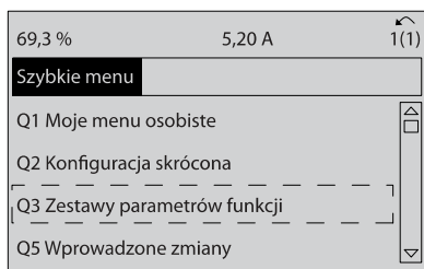
Ilustracja 7.3: Krok 3: Za pomocą przycisków nawigacji góra/dół przejść do zestawów parametrów funkcji. Nacisnąć przycisk [OK].
