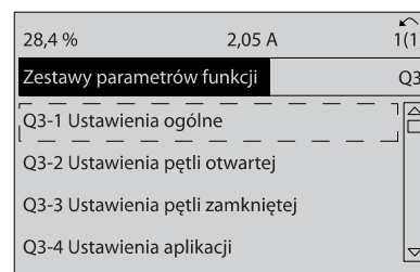
Ilustracja 7.4: Krok 4: Na ekranie pojawią się opcje zestawów parametrów funkcji. Wybrać Q3-1 Ustawienia ogólne. Nacisnąć przycisk [OK].
