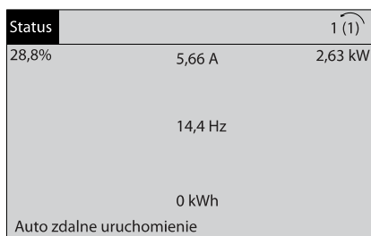
Ilustracja 7.1: Krok 1: Włączyć przetwornicę częstotliwości (zapala się żółta dioda)
