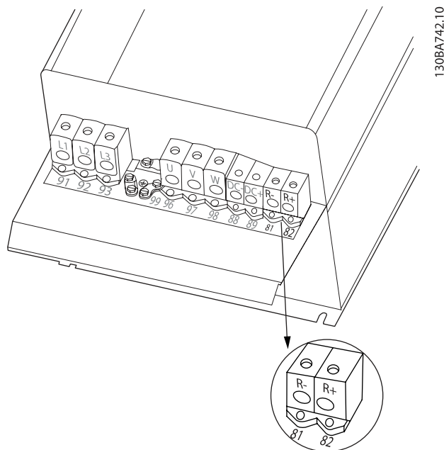
Ilustracja 4.27: Zacisk podłączenia rezystora hamowania dla C4
