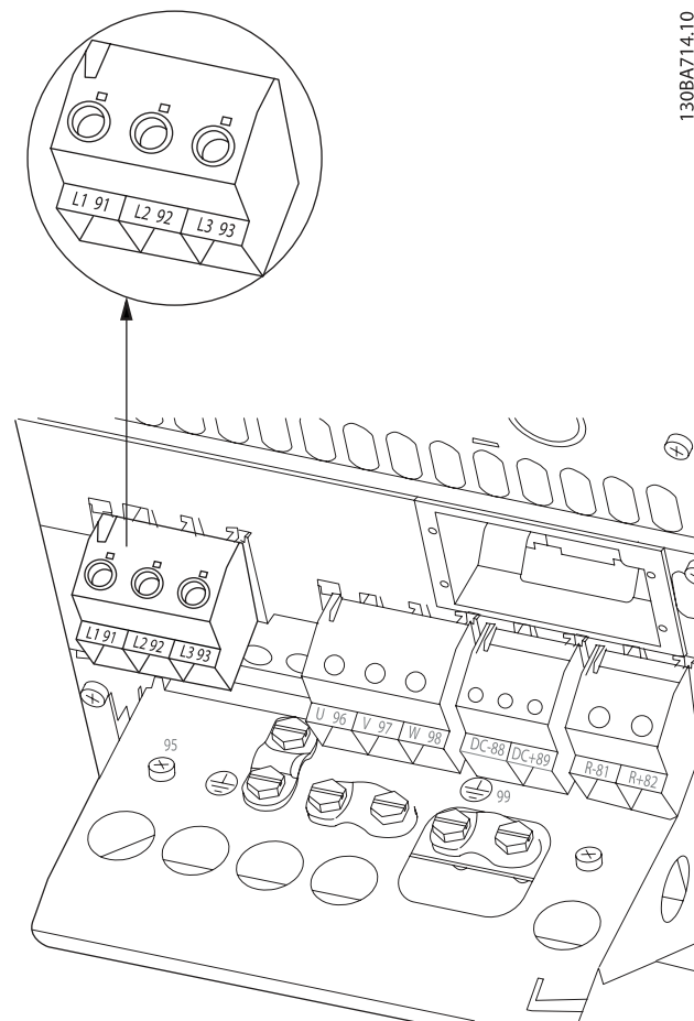
Рисунок 4.12: Подключение к сети и заземлению для V4.
