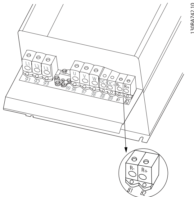
Рисунок 4.27: Клемма подключения тормоза для C4.
