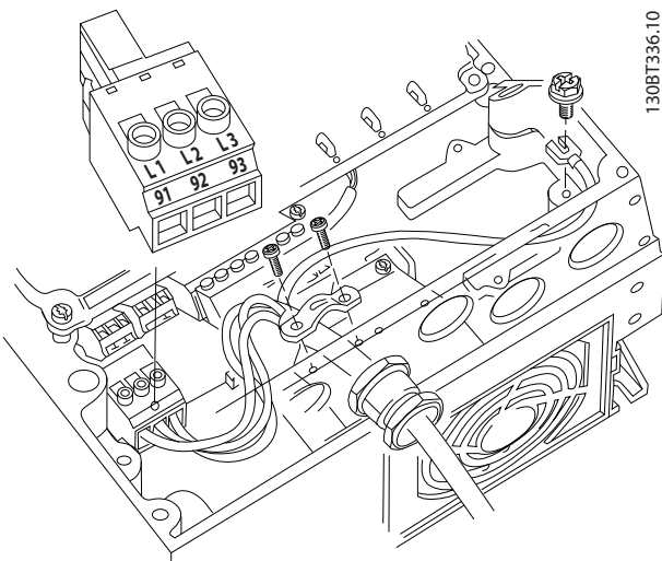
그림 2.13 교류 주전원에 연결하는 방법
