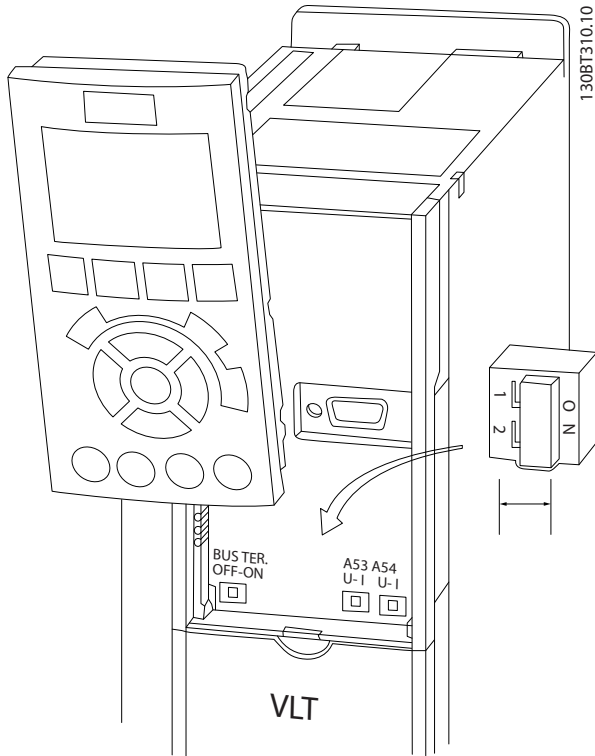
그림 2.19 단자 53 및 54 스위치의 위치
