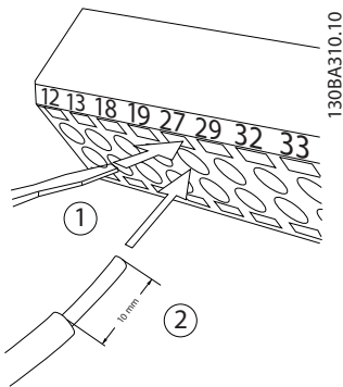
그림 2.18 제어부 배선 연결
