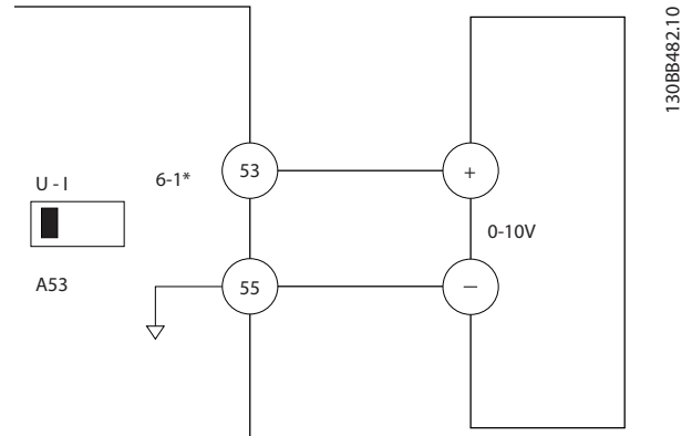
그림 5.1 0-10V 제어 신호를 제공하는 외부 장치를 위한 배선 예시
