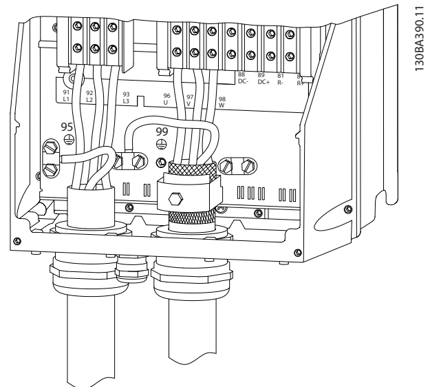
그림 2.11 차폐 케이블을 사용한 B 프레임 용량 이상의 모터, 주전원 및 접지 배선
