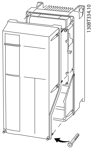
그림 2.15 A4, A5, B1, B2, C1 및 C2 외함의 제어부 배선 접근 방법
