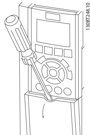
그림 2.14 A2, A3, B3, B4, C3 및 C4 외함의 제어부 배선 접근 방법
