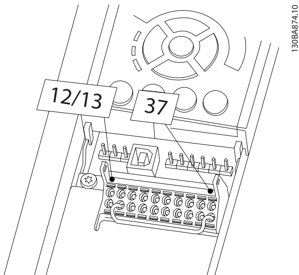
그림 2.20 단자 12/13(24V)과 37 간의 점퍼
