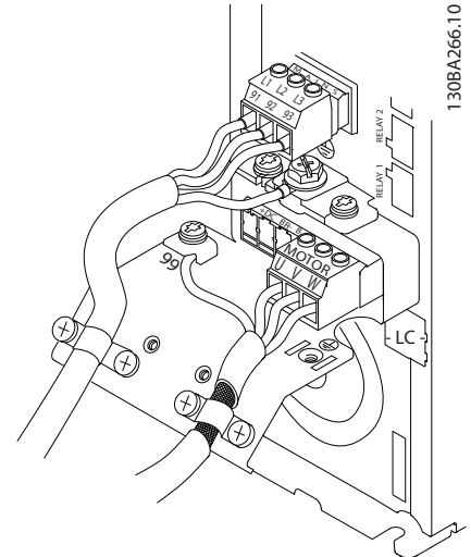
그림 2.10 A 프레임 용량의 모터, 주전원 및 접지 배선
