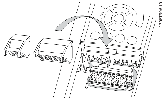
그림 2.17 제어 단자 분리
