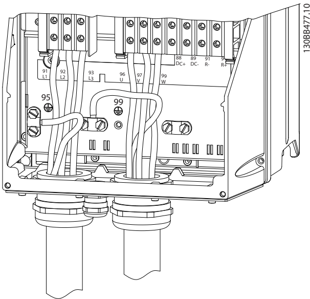
그림 2.9 도관을 이용한 접지
