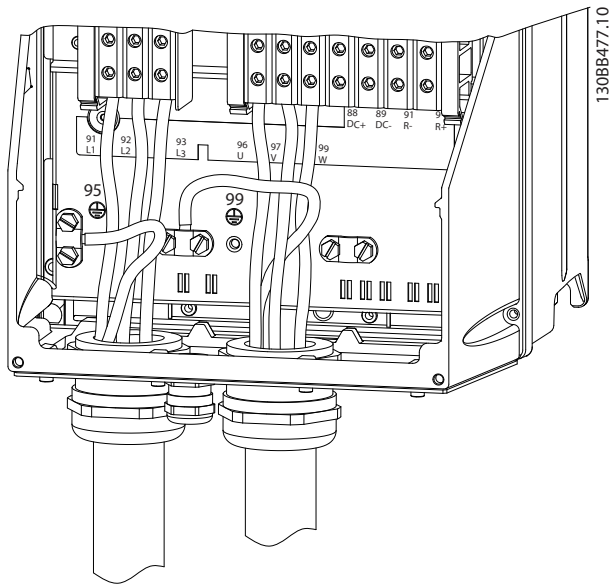
그림 2.12 도관을 사용한 B 프레임 용량 이상의 모터, 주전원 및 접지 배선
