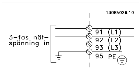
Bild 5.5: Plintar för nät och jordning.
