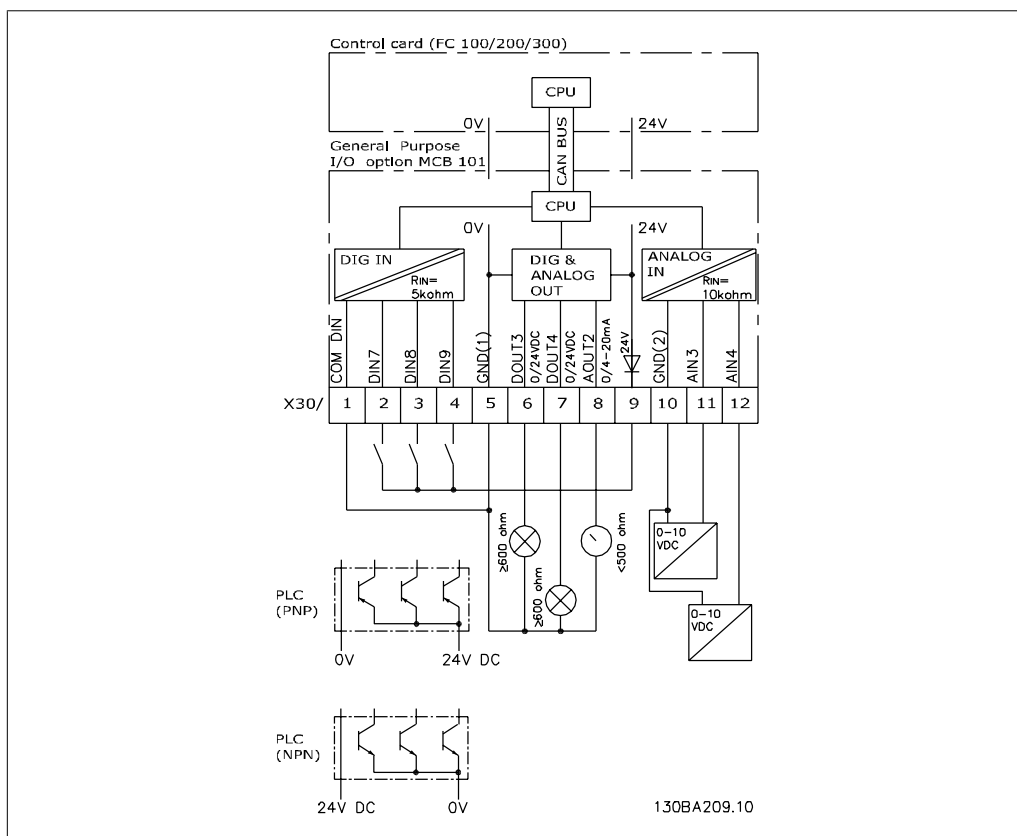
Bild 3.10: Kopplingschema
