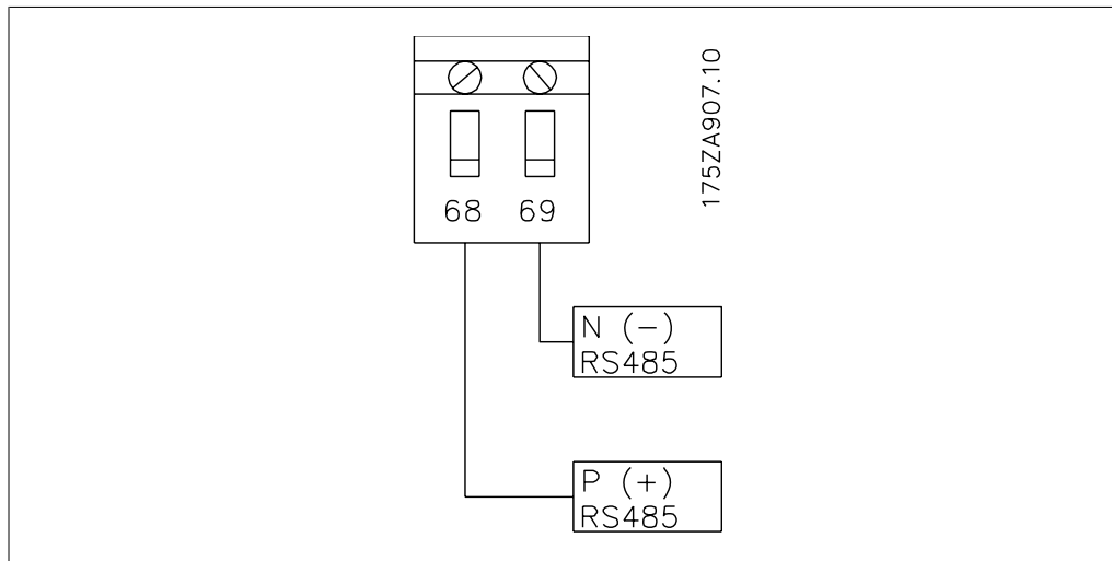
Bild 7.1: Nätverkskabelanslutning
