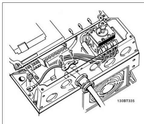
Bild 5.6: Så här ansluter du till nät och jordning med fränkskiltare (A5-kapsling).
