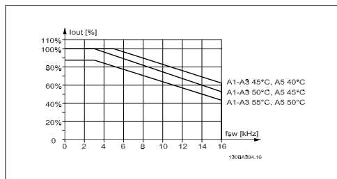
Bild 3.3: Nedstämpling av I_{out} för olika T_{AMB,MAX} för A-kapsling när 60 PWM används och maximalt 10 m motorkabel
