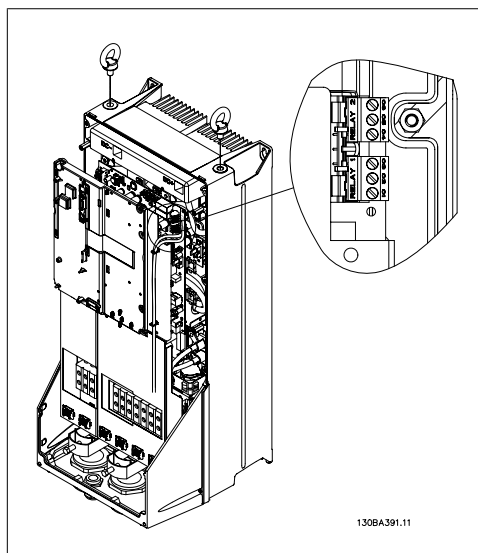
Bild 5.17: Plintar för reläanslutning (C1- och C2-kapslingar).
