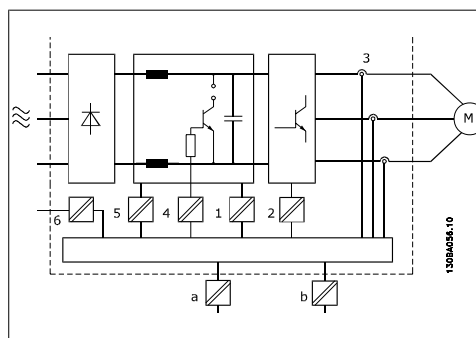
Bild 2.2: Galvanisk isolation
