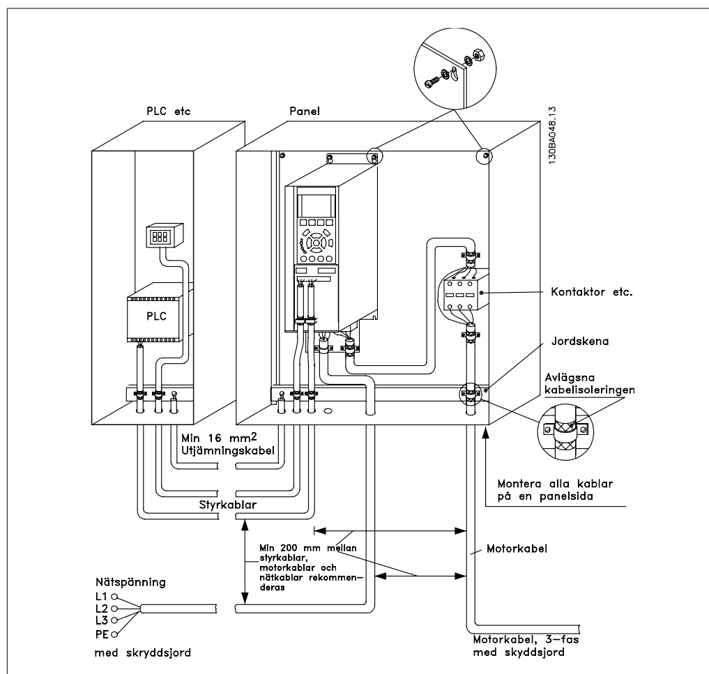
Bild 5.18: EMC-korrekt elektrisk installation av en frekvensomformare i apparatskåp.
