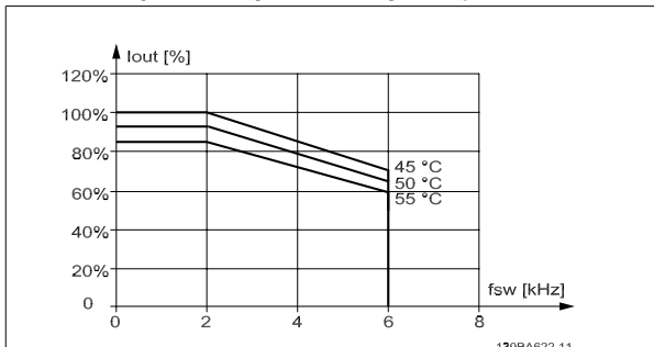
Рисунок 3.15: Снижение тока I_{out} для различных значений T_{AMB, MAX} для корпуса E при напряжении 480 В при использовании модели коммутации 60 AVM в режиме нормального крутящего момента (перегрузка по крутящему моменту 110 %).
