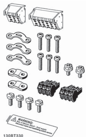
Типоразмеры B1 и B2 IP21/IP55/тип 1/тип 12
