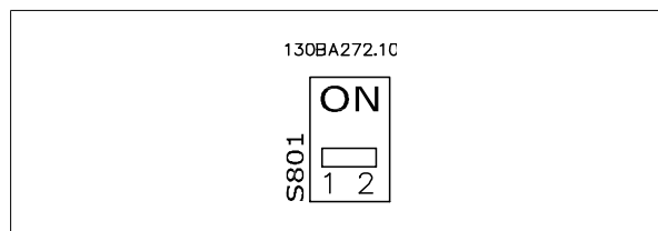
Заводская установка переключателя
