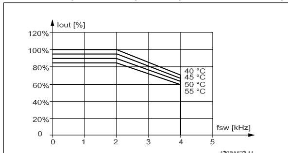
Рисунок 3.16: Снижение тока I_{out} для различных значений T_{AMB, MAX} для корпуса E при напряжении 480 В при использовании модели коммутации SFAVM в режиме нормального крутящего момента (перегрузка по крутящему моменту 110 %).
