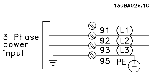
Рисунок 5.5: Клеммы сетевого питания и заземления.
