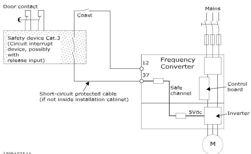
Рисунок 2.5: Рисунок, поясняющий основные особенности установки, необходимые для осуществления останова категории 0 (EN 60204-1), отвечающего требованиям категории безопасности 3 (EN 954-1).
