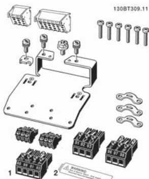
Типоразмеры A1, A2 и A3 IP 20 / Шасси
