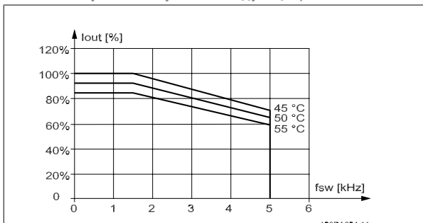
Рисунок 3.17: Снижение тока I_{out} для различных значений T_{AMB, MAX} для корпуса E при напряжении 600 В при использовании модели коммутации 60 AVM в режиме нормального крутящего момента (перегрузка по крутящему моменту 110 %).
