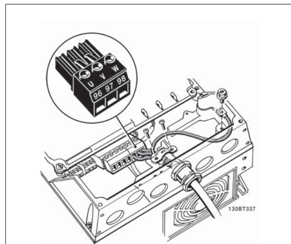
Рисунок 5.9: Подключение двигателя в случае корпуса А5
