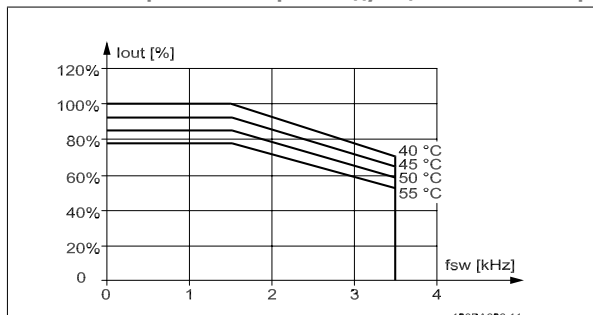
Рисунок 3.18: Снижение тока I_{out} для различных значений T_{AMB, MAX} для корпуса E при напряжении 600 В при использовании модели коммутации SFAVM в режиме нормального крутящего момента (перегрузка по крутящему моменту 110 %).
