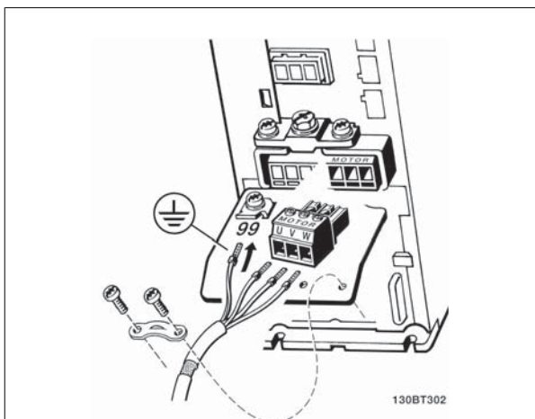
Рисунок 5.8: Подключение двигателя в случае корпусов А2 и А3
