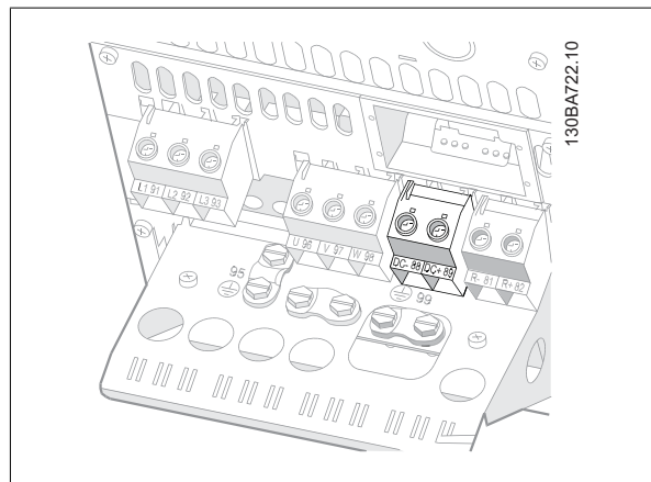
Illustration 5.36: DC bus-tilslutning til kapsling B4.
