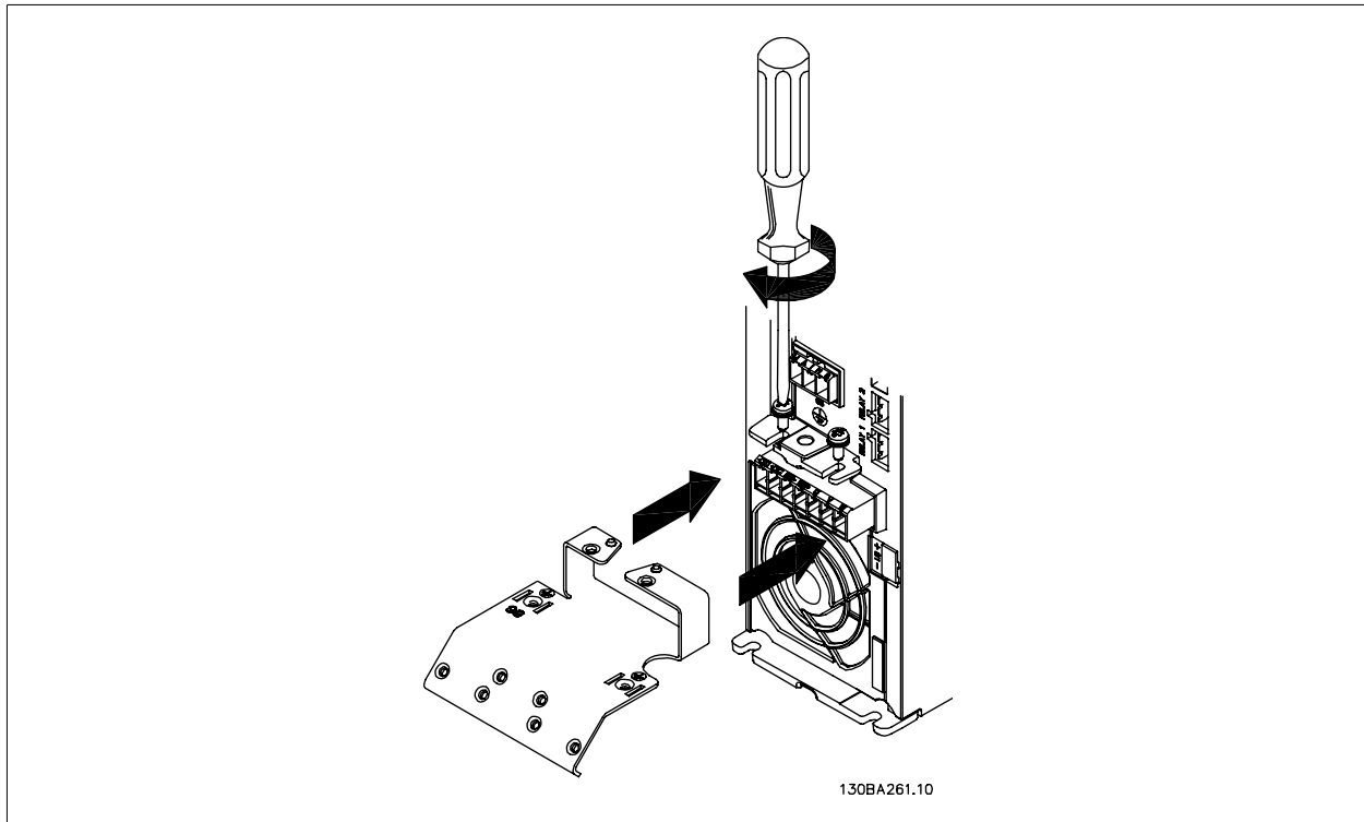
Illustration 5.7: Monter først de to skruer i monteringspladen, skub den på plads, og spænd fuldstændigt.
