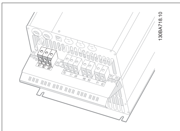
Illustration 5.18: Sådan slutes C3 til netforsyning og jording.
