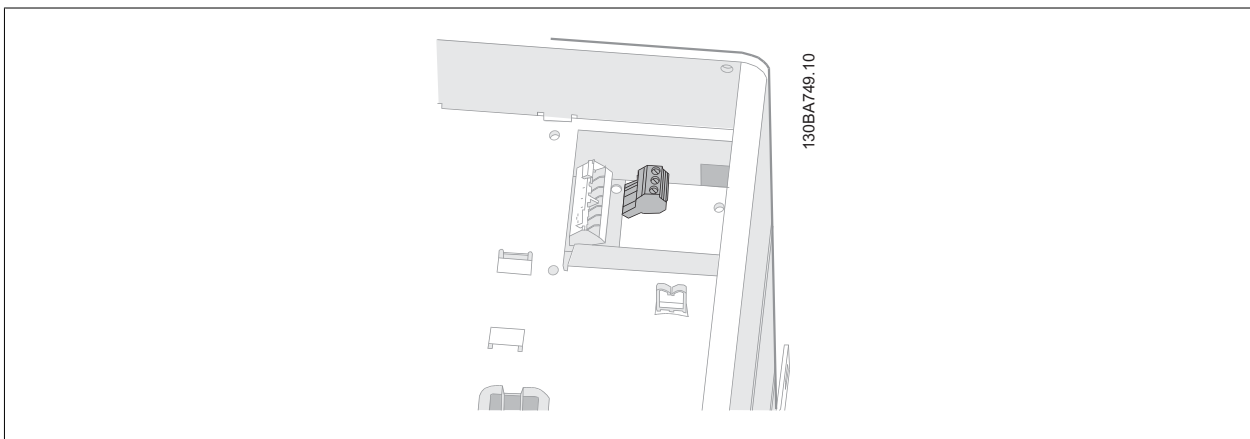
Illustration 5.46: Terminaler for relætilslutninger til C3 og C4. Placeret i frekvensomformerens øverste højre hjørne.
