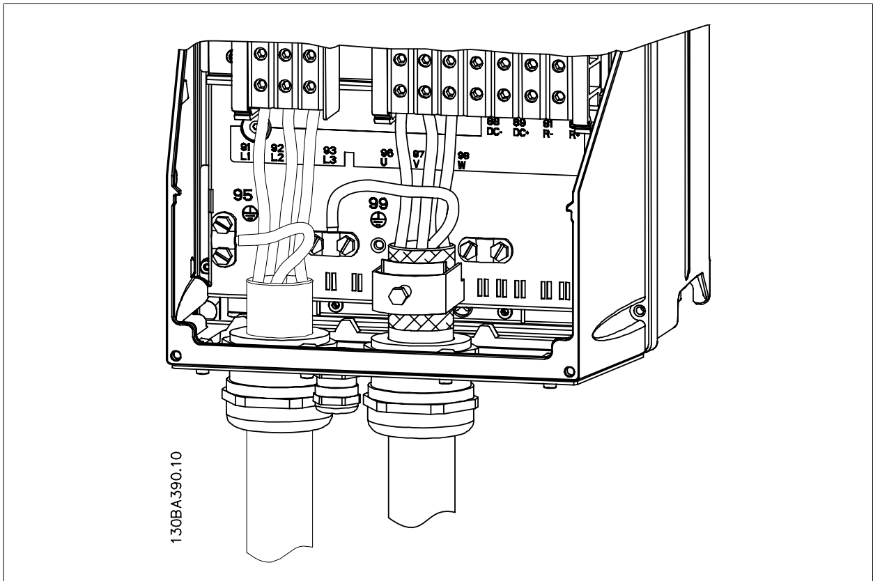
Illustration 5.27: Terminer først motorens jording, placer derefter motorens U-, V- og W-ledninger i klemmen, og spænd dem. Sørg for, at motorkablets udvendige isolering er fjernet under EMC-bøjlen.
