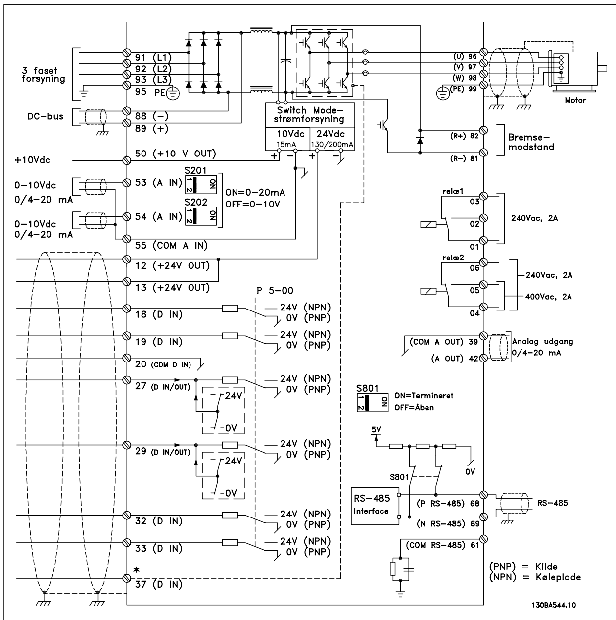
Illustration 5.34: Diagram over samtlige elektriske klemmer. (Klemme 37 findes kun på enheder med funktionen Sikker standsning).
