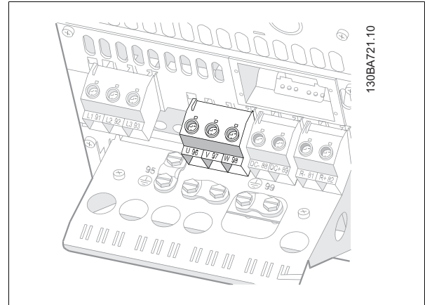
Illustration 5.26: Terminer først motorens jording, placer derefter motorens U-, V- og W-ledninger i klemmen, og spænd dem. Sørg for, at motorkablets udvendige isolering er fjernet under EMC-bøjlen.
