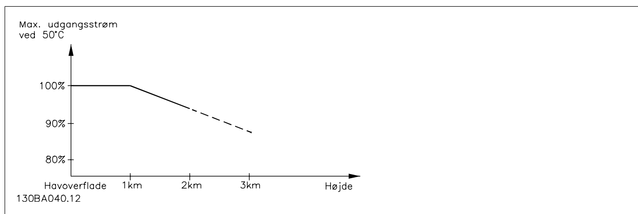
Illustration 8.1: Derating af udgangsstrøm kontra højde ved T_{OMG, MAXS} . Kontakt Danfoss i forbindelse med PELV ved højder på mere end 2 km.
