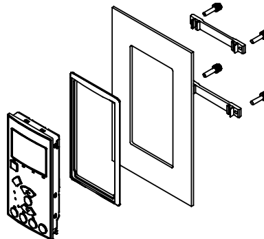
Illustration 3.6: LCP-sæt med numerisk LCP, fastgøringsele og pakning.
