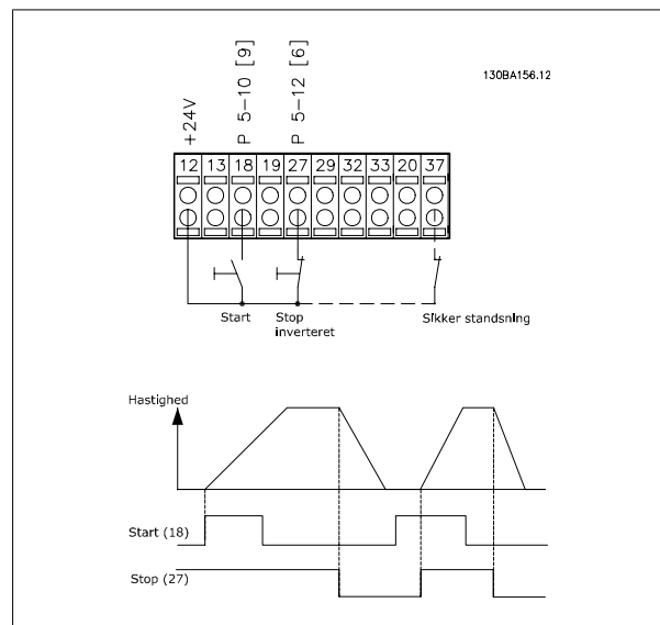
Illustration 5.33: Klemme 37 er kun disponibel sammen med funktionen Sikker standsning!
