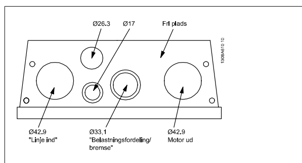
Illustration 5.2: Kabelindgangshuller til kapsling B2. Den foreslåede brug af hullerne er udelukkende anbefalinger. Andre løsninger er mulige.
