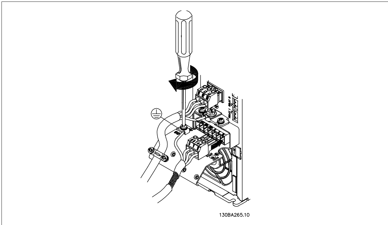
Illustration 5.21: Terminer først motorens jording, placer derefter motorens u-, v- og w-ledninger i stikket, og spænd dem.
