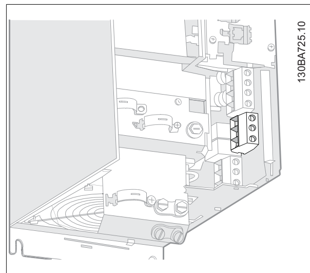
Illustration 5.15: Sådan udføres tilslutning til netforsyning og jording for B3 uden RFI.
