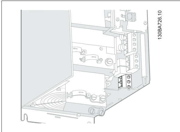
Illustration 5.25: Terminer først motorens jording, placer derefter motorens U-, V- og W-ledninger i klemmen, og spænd dem. Sørg for, at motorkablets udvendige isolering er fjernet under EMC-bøjlen.
