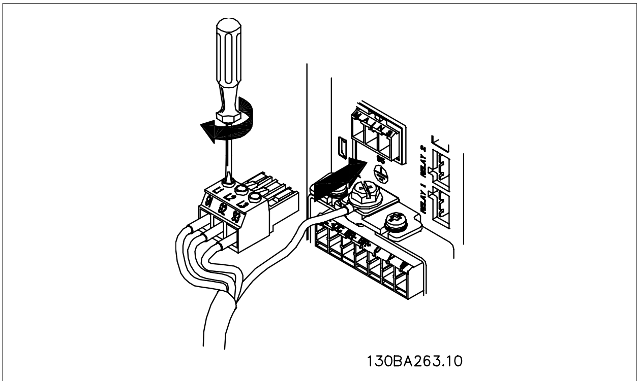
Illustration 5.9: Derefter monteres netstikket, og ledningerne tilspændes.
