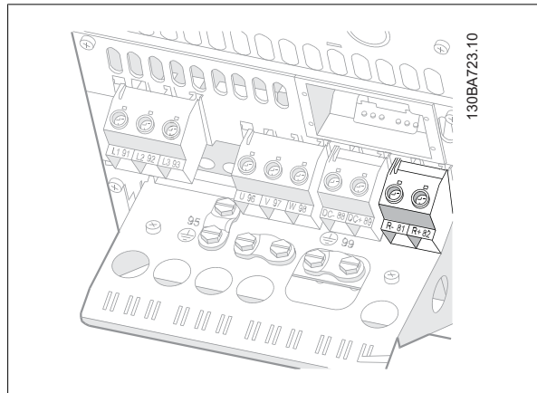
Illustration 5.40: Bremsetilslutningsklemme for B4.
