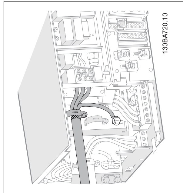
Illustration 5.14: Sådan udføres tilslutning til netforsyning og jording for B3 med RFI.
