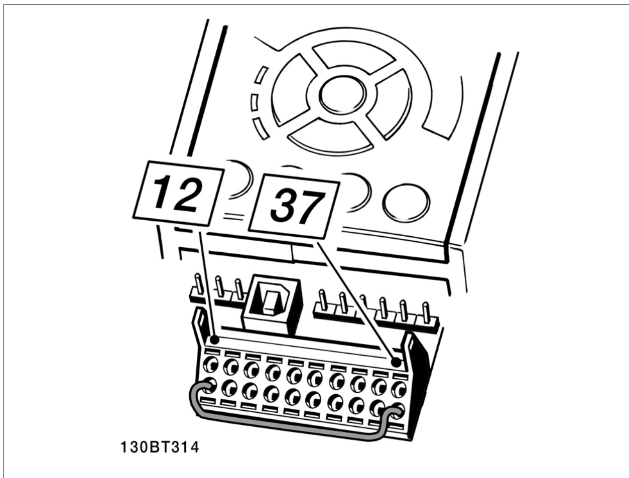
Illustration 2.8: Opret en bro for jumperen mellem klemme 37 og 24 V DC
