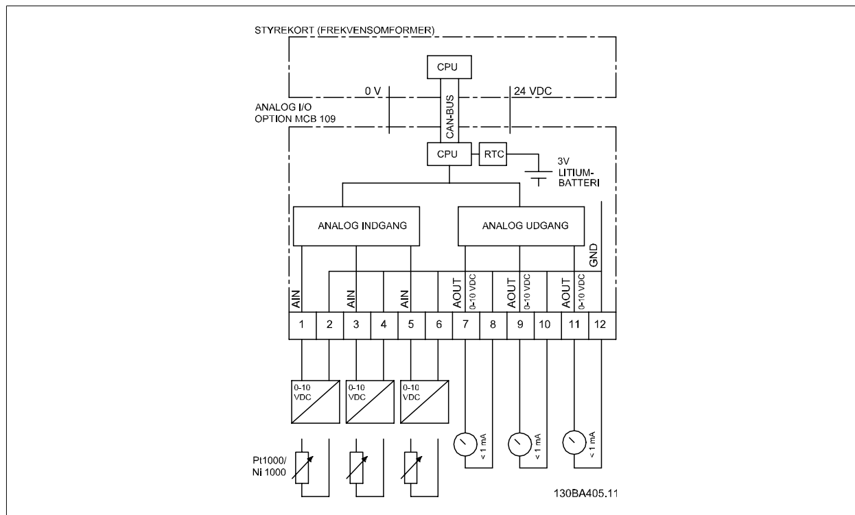
Illustration 3.4: Principdiagram til analog I/O monteret i frekvensomformer.
