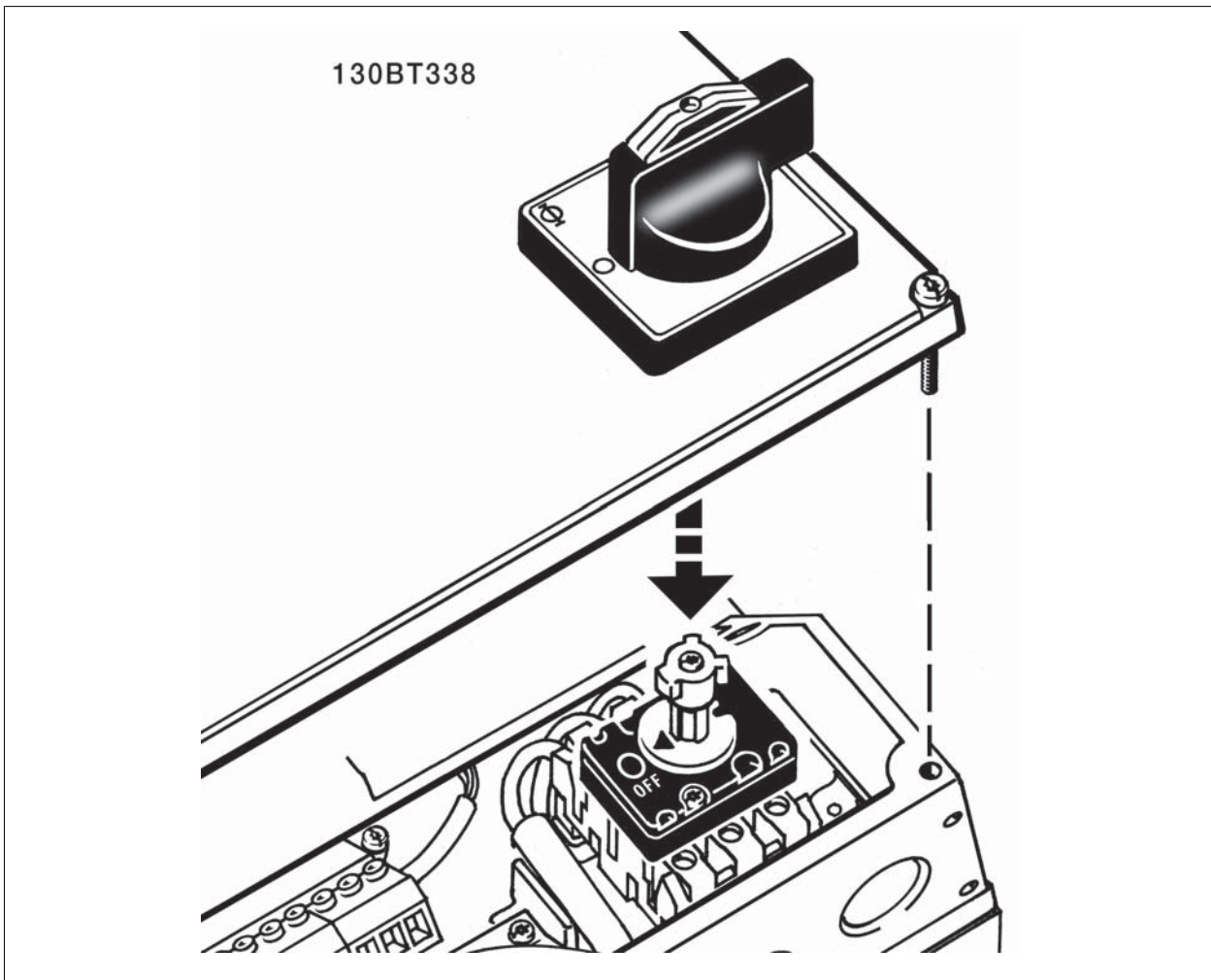
Illustration 5.32: Samling af IP 21/IP 55/NEMA TYPE 12-hus med netforsyningsafbryder.
