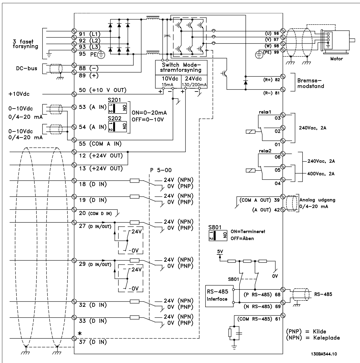
Illustration 2.7: Diagram over samtlige elektriske klemmer. (Klemme 37 findes kun på enheder med funktionen Sikker standsning).
