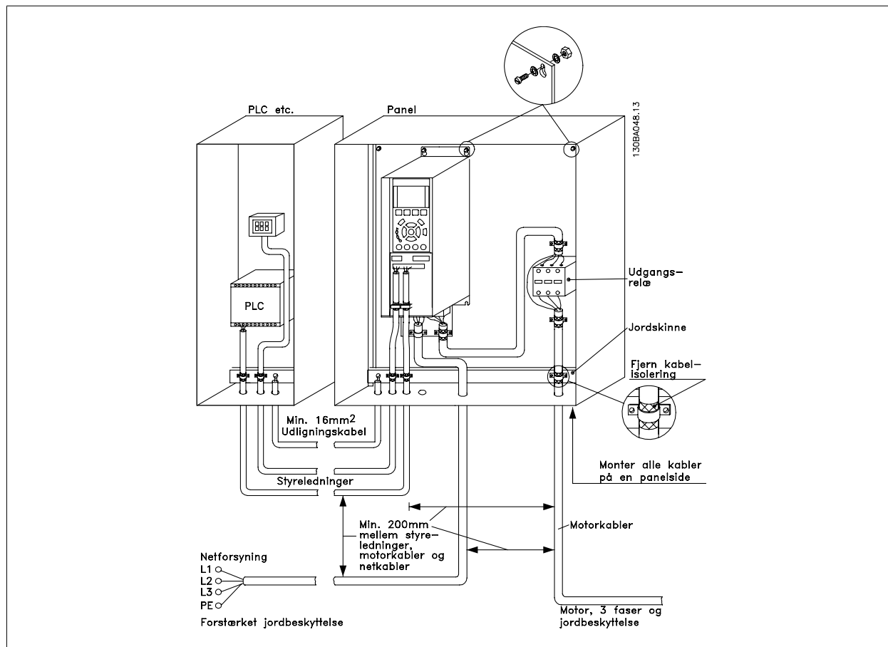
Illustration 5.48: EMC-korrekt elektrisk installation af en frekvensomformer i kabinnet.
