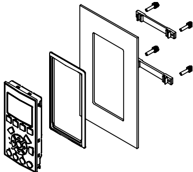
Illustration 3.5: LCP-sæt med grafisk LCP, fastgøringsele, 3 m kabel og pakning.
