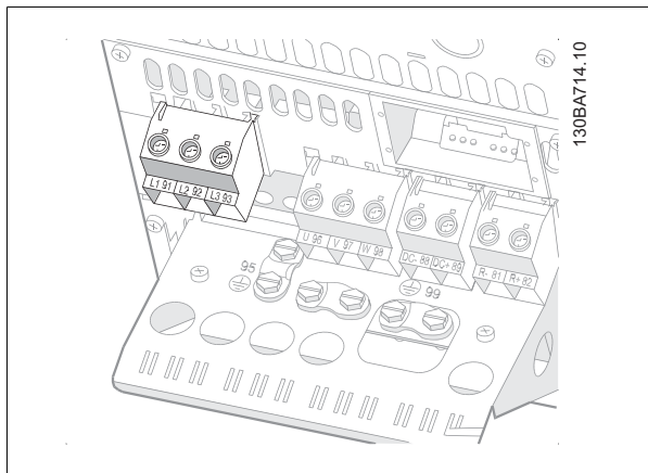
Illustration 5.16: Sådan udføres tilslutning til netforsyning og jording for B4.
