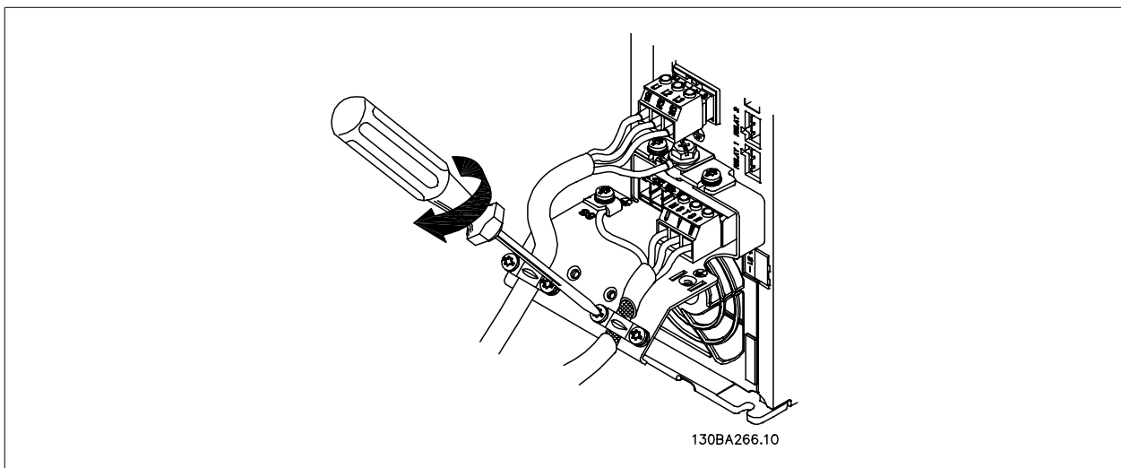
Illustration 5.22: Monter kabelbøjlen for at sikre 360 graders forbindelse imellem chassiset og skærmen. Vær opmærksom på, at motorkabelisoleringen skal fjernes under bøjlen.
