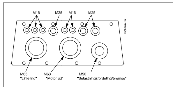
Illustration 5.4: Kabelindgangshuller til kapsling C2. Den foreslåede brug af hullerne er udelukkende anbefalinger. Andre løsninger er mulige.
