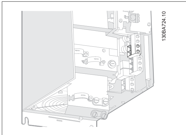
Illustration 5.39: Bremsetilslutningsklemme for B3.
