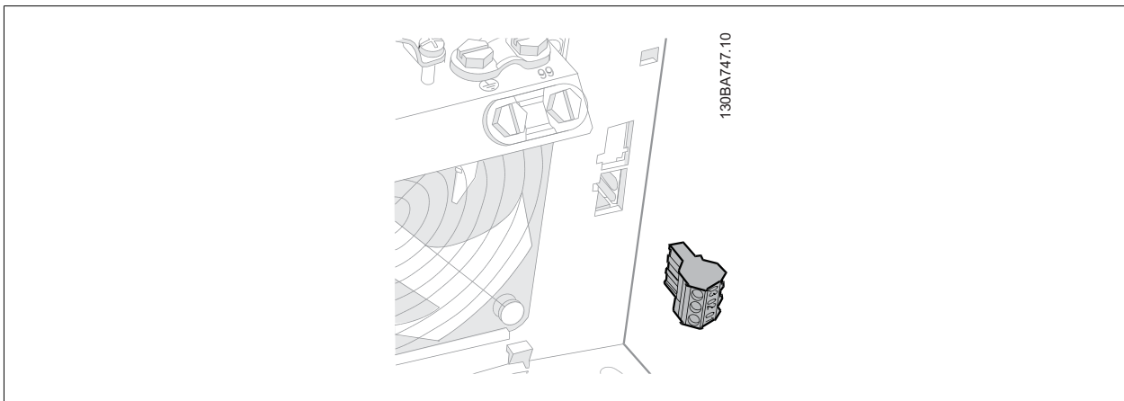
Illustration 5.44: Klemmer til relætilslutninger til B3. Der er kun installeret en knock-out fra fabrikken.
