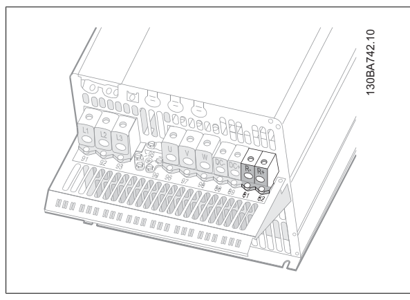
Illustration 5.42: Bremsetilslutningsklemme for C4.
