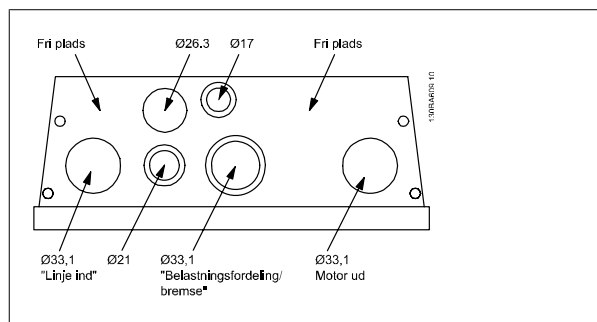
Illustration 5.1: Kabelindgangshuller til kapsling B1. Den foreslåede brug af hullerne er udelukkende anbefalinger. Andre løsninger er mulige.
