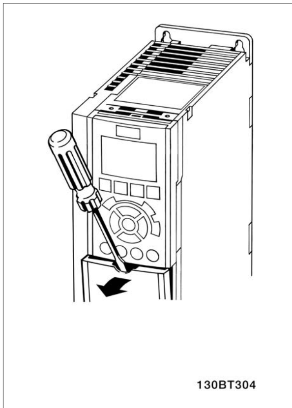
Illustration 5.29: A1-, A2-, A3-, B3-, B4-, C3- og C4-kapslinger
