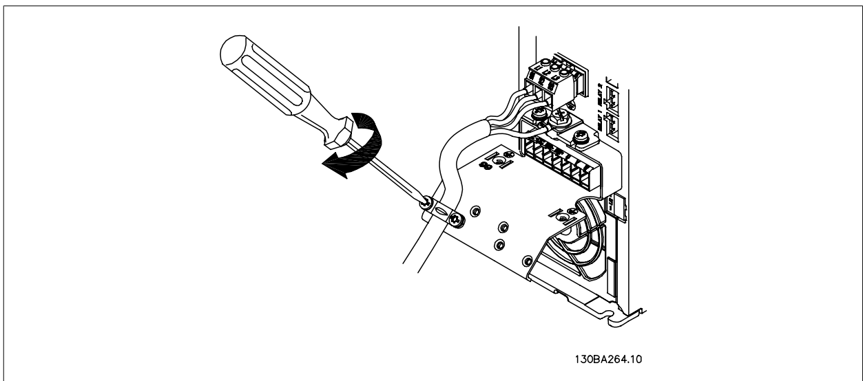
Illustration 5.10: Spænd til sidst støttebeslaget på netledningerne.
