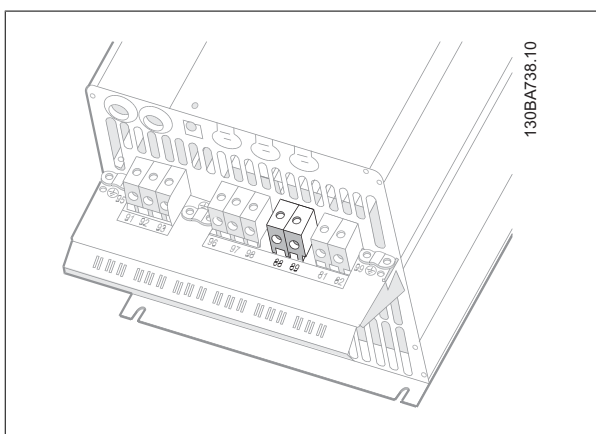
Illustration 5.37: DC bus-tilslutning til kapsling C3.
