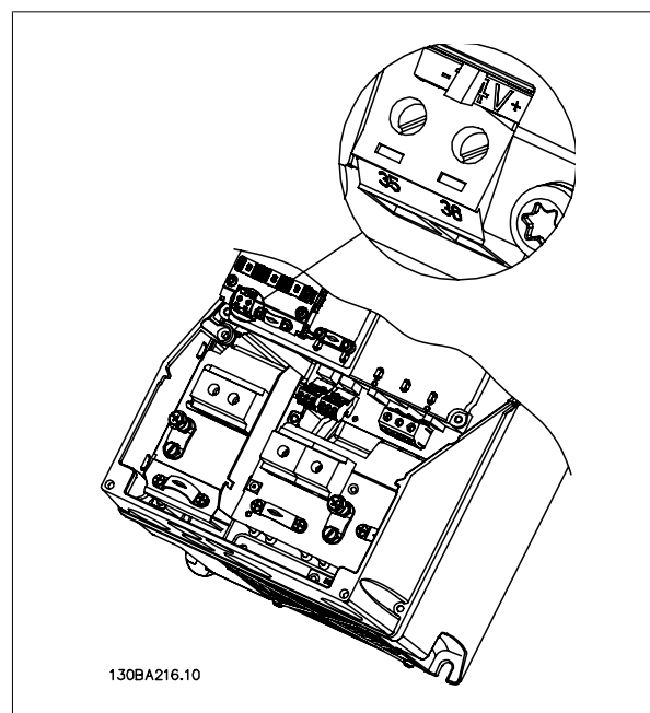
Illustration 3.3: Tilknytning til 24 V backup-forsyning (A5-C2).
