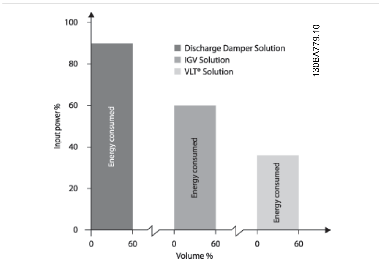
Illustration 2.4: Afladningsfugtere reducerer strømforbruget en del. Inlet Guide Vans tilbyder en 40 % reducereing, men er dyre at installere. Danfoss VLT®-løsningen reducerer energiforbruget med mere end 50 % og er let at installere.
