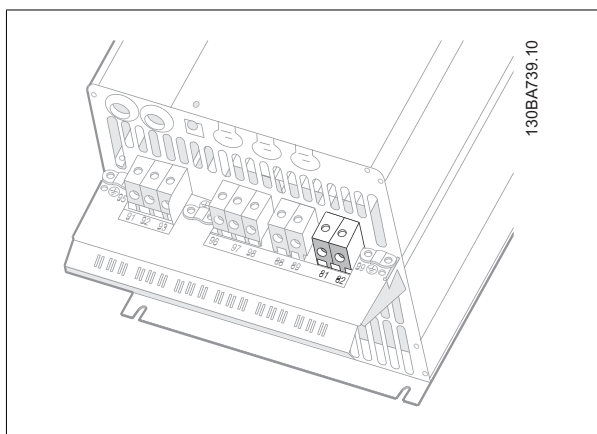
Illustration 5.41: Bremsetilslutningsklemme for C3.
