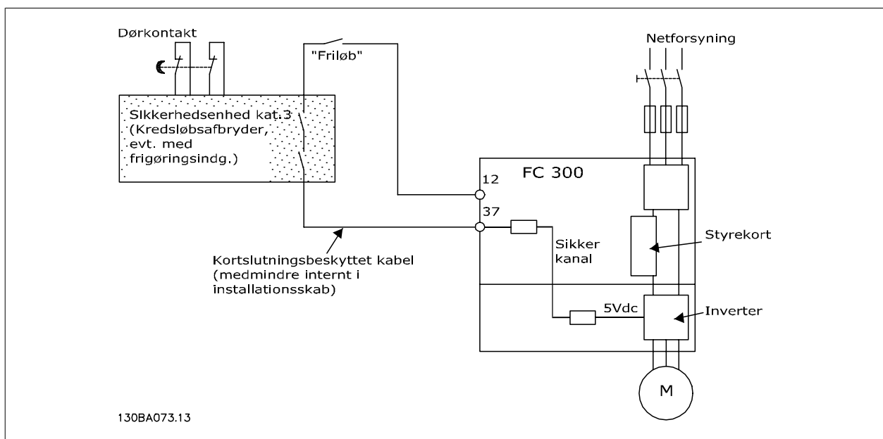
Illustration 2.9: Illustration af de vigtigste aspekter af en installation for at opnå en Stopkategori 0 (EN 60204-1) med sikkerhedskategori 3 (EN 954-1).
