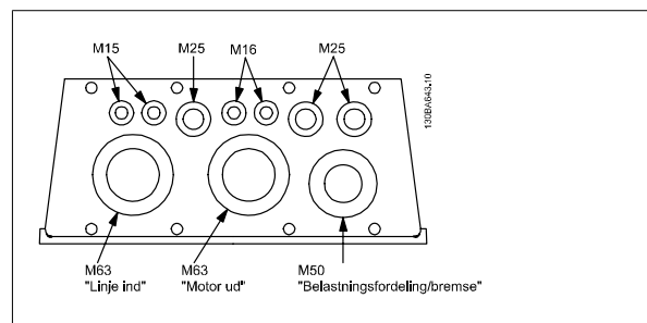
Illustration 5.3: Kabelindgangshuller til kapsling C1. Den foreslåede brug af hullerne er udelukkende anbefalinger. Andre løsninger er mulige.
