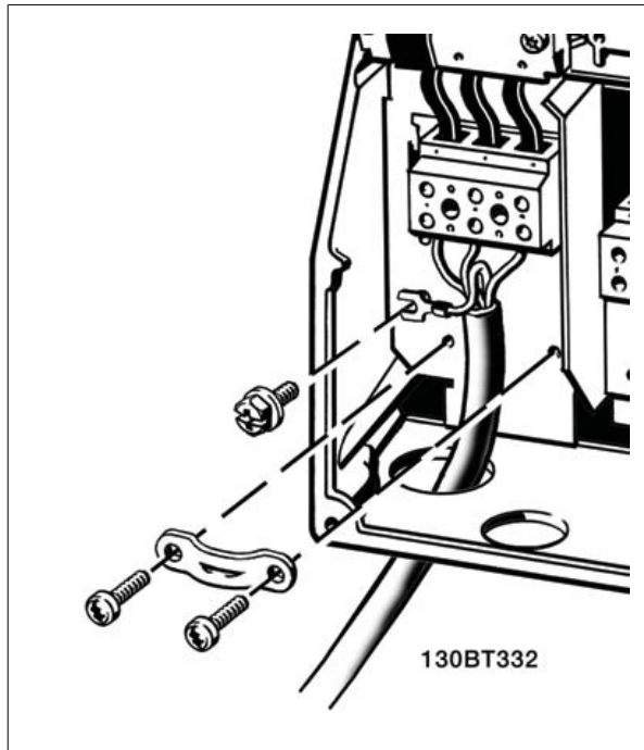
Illustration 5.13: Sådan udføres tilslutning til netspænding og jording for B1 og B2.
