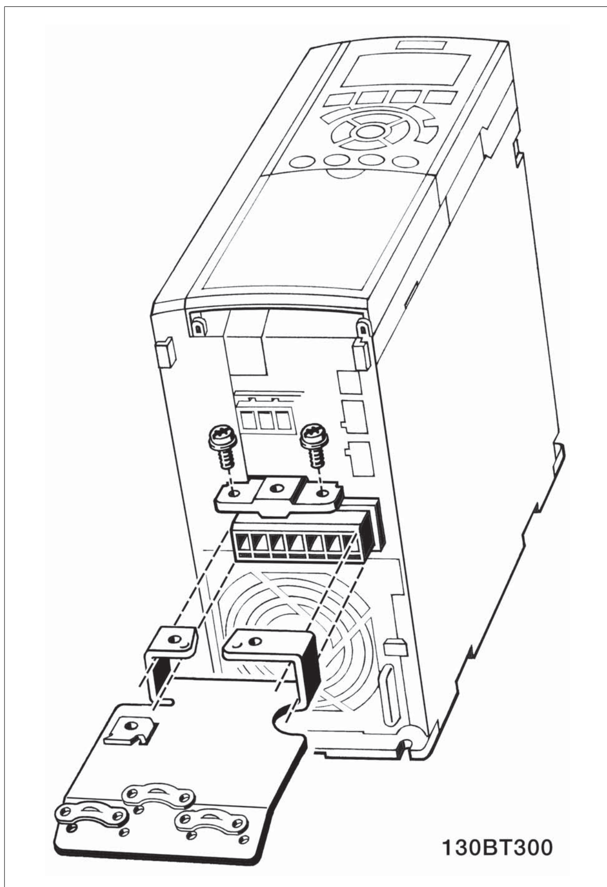
Illustration 5.20: Montering af frakoblingspladen.
