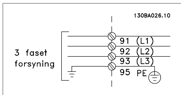
Illustration 5.5: Klemmer til net og jording.
