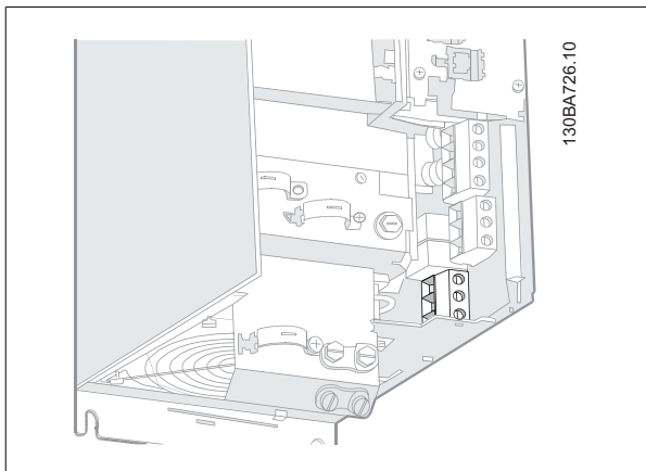
Ilustración 5.25: En primer lugar, termine la toma de tierra del motor y, a continuación, instale en sus terminales los cables U, V y W del motor y fíjelos. Asegúrese de que el aislamiento exterior del cable de motor esté retirado bajo la abrazadera EMC.
