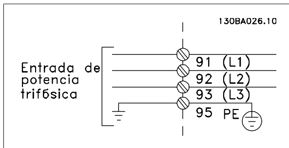
Ilustración 5.5: Terminales para la red de alimentación y la toma de tierra.
