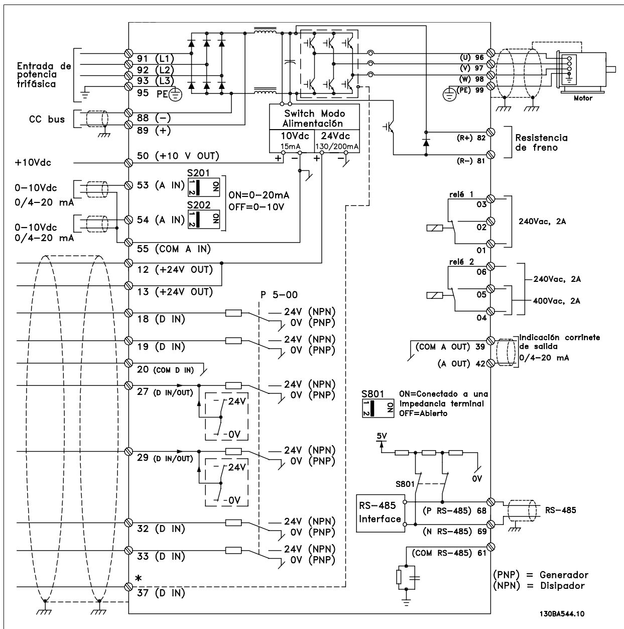
Ilustración 5.34: Diagrama que muestra todos los terminales eléctricos. (El Terminal 37 sólo está presente en unidades con función de parada de seguridad.)
