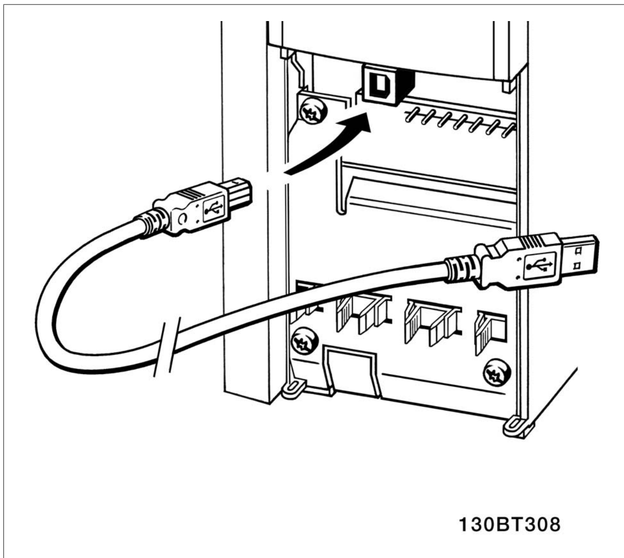
Ilustración 5.47: Para la instalación del cableado de control consulte el apartado Terminales de Control .
