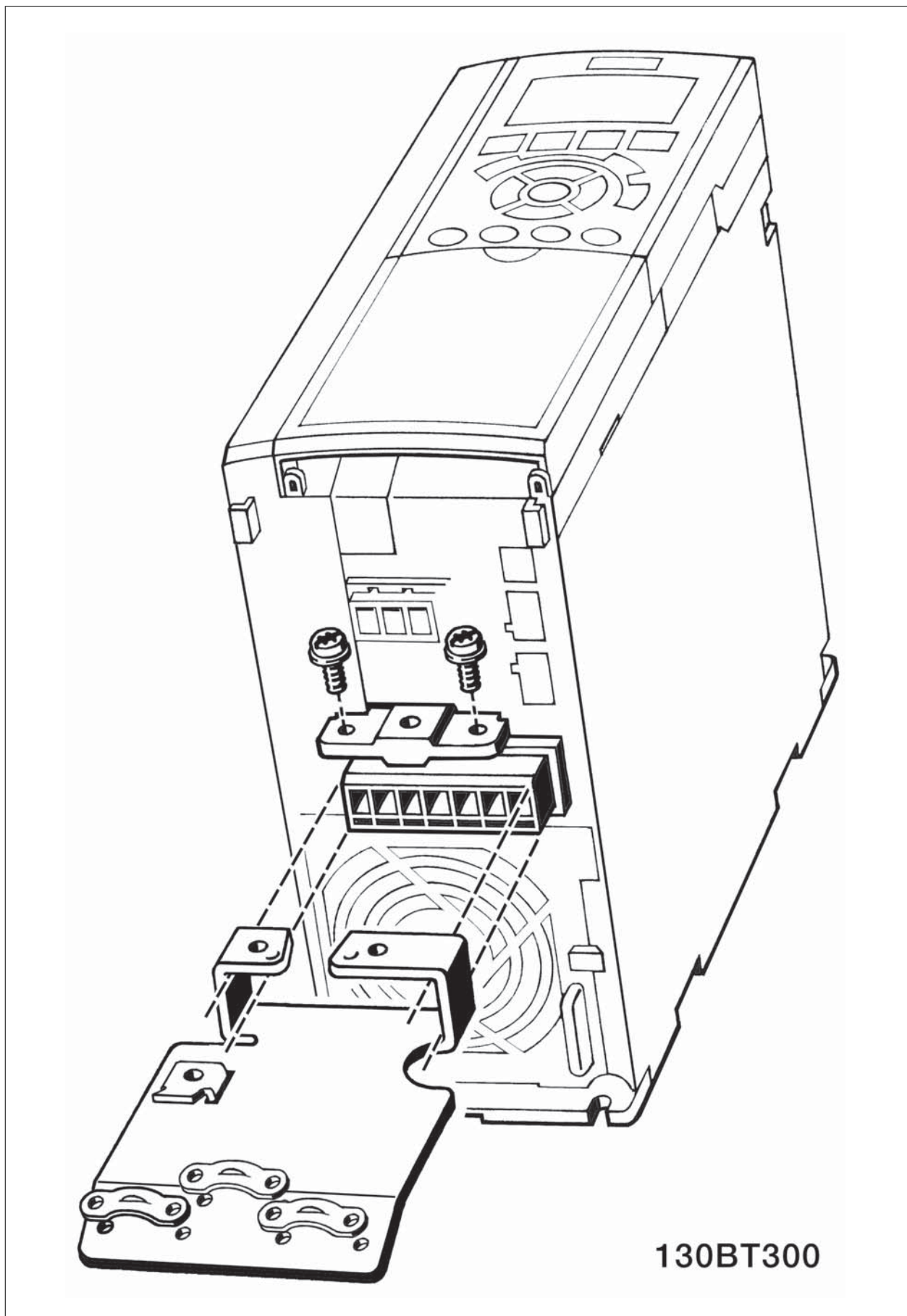
Ilustración 5.20: Montaje de la placa de conexión de pantallas
