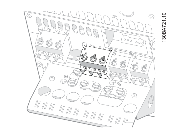
Ilustración 5.26: En primer lugar, termine la toma de tierra del motor y, a continuación, instale en sus terminales los cables U, V y W del motor y fíjelos. Asegúrese de que el aislamiento exterior del cable de motor esté retirado bajo la abrazadera EMC.
