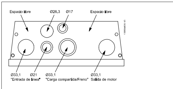
Ilustración 5.1: Orificios de entrada para cables en el armario B1. La utilización que se sugiere de los orificios es solo una recomendación, siendo posibles otras soluciones.
