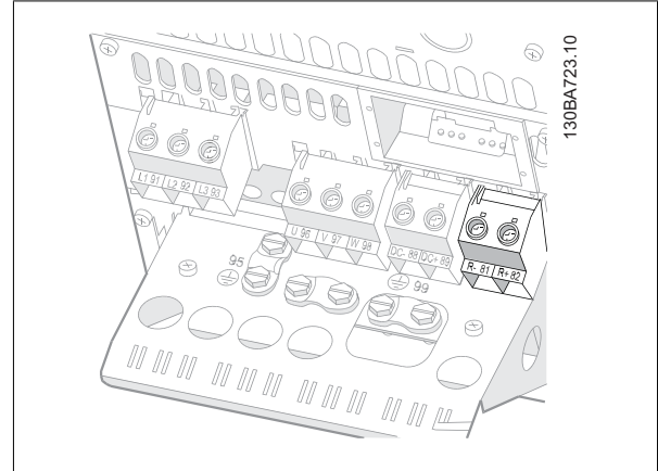
Ilustración 5.40: Terminal de conexión de freno para B4.
