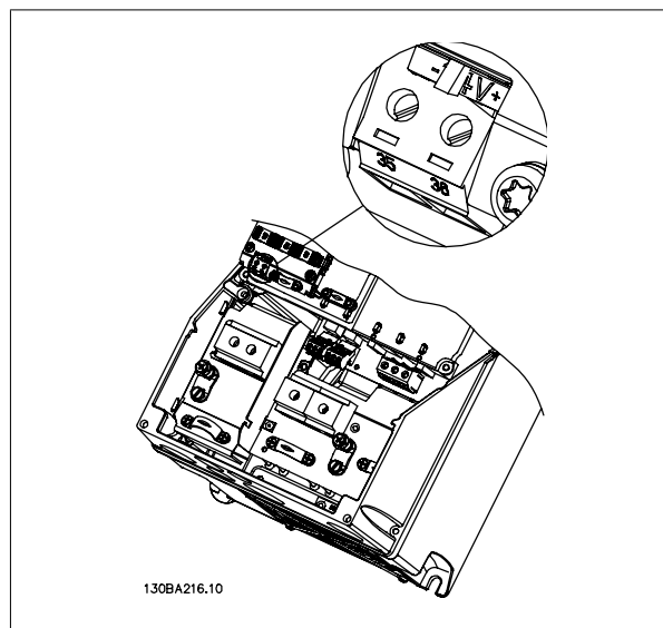
Ilustración 3.3: Conexión al suministro externo de 24 V (A5-C2).
