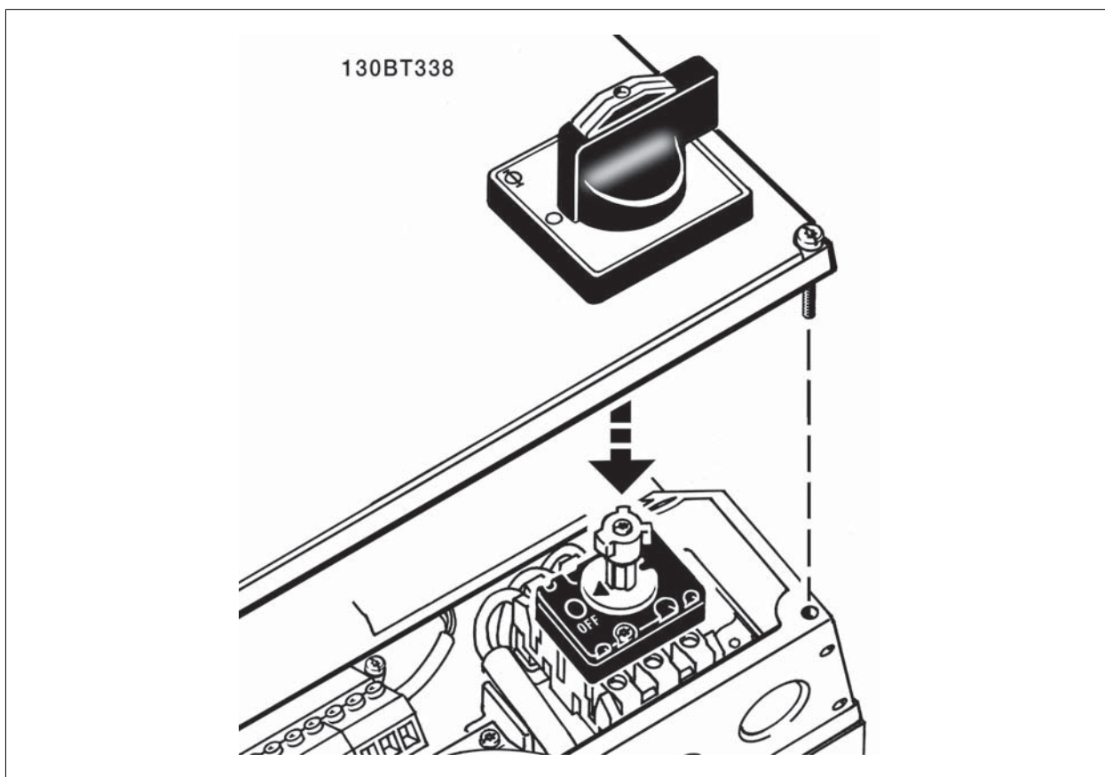
Ilustración 5.32: Montaje de alojamiento IP55 / NEMA TIPO 12 con desconector de red
