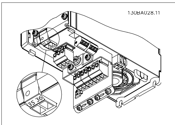
Ilustración 3.2: Conexión al suministro externo de 24 V (A2-A3).
