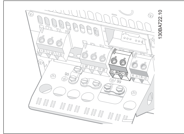
Ilustración 5.36: Conexiones de bus de CC para protección B4.
