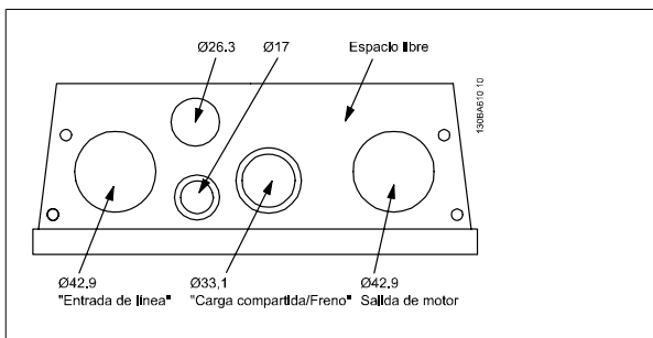
Ilustración 5.2: Orificios de entrada para cables en el armario B2. La utilización que se sugiere de los orificios es solo una recomendación, siendo posibles otras soluciones.
