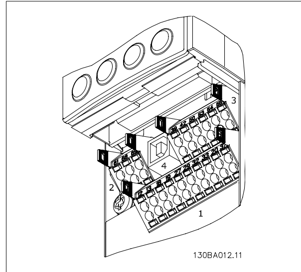
Ilustración 5.31: Terminales de control (todas las protecciones)
