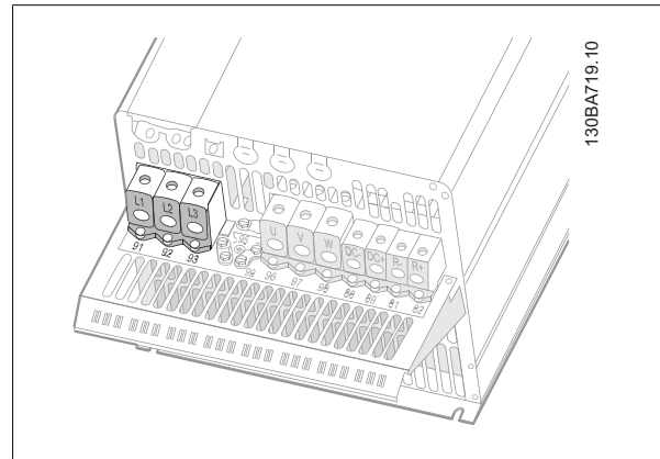
Ilustración 5.19: Cómo realizar la conexión a red de alimentación y a tierra de C4.
