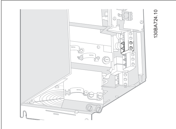
Ilustración 5.39: Terminal de conexión de freno para B3.
