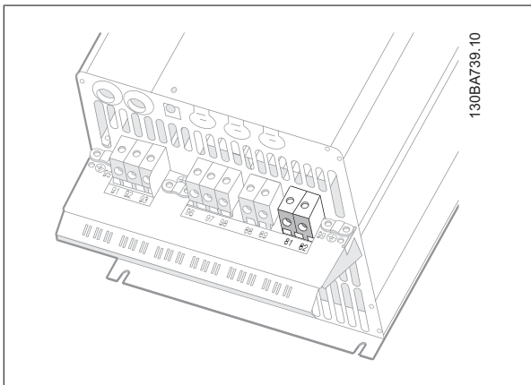
Ilustración 5.41: Terminal de conexión de freno para C3.
