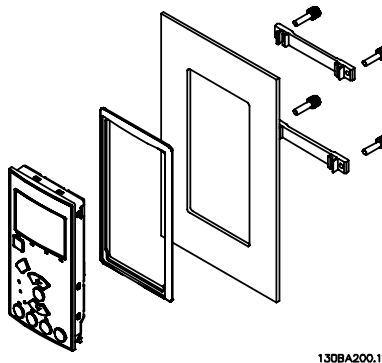
Ilustración 3.6: Kit LCP con LCP numérico, sujeciones y junta.
