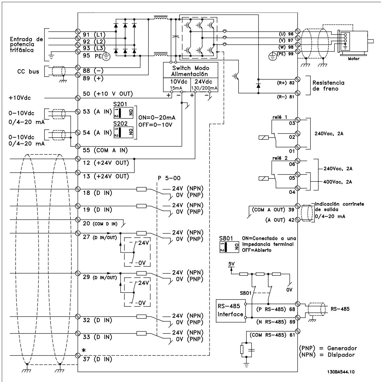
Ilustración 2.7: Diagrama que muestra todos los terminales eléctricos. (El Terminal 37 sólo está presente en unidades con función de parada de seguridad.)
