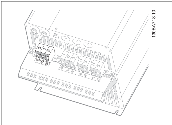
Ilustración 5.18: Cómo realizar la conexión a red de alimentación y a tierra de C3.
