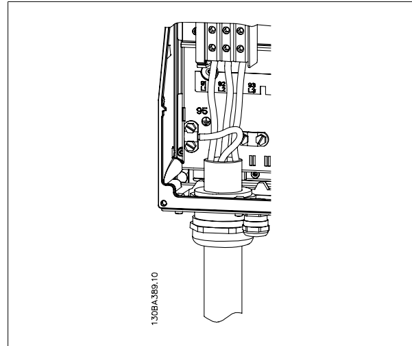
Ilustración 5.17: Cómo realizar la conexión a la red de alimentación y a tierra de C1 y C2.
