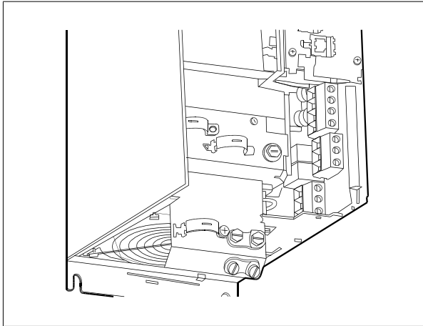
Ilustración 5.35: Conexiones de bus de CC para protección B3.
