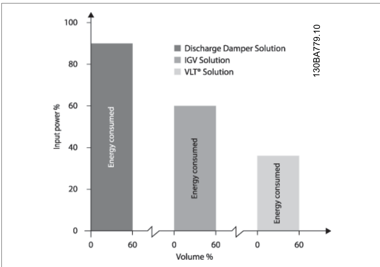
Ilustración 2.4: Los atenuadores de descarga reducen el consumo de potencia en cierta medida. Las aletas guiadoras variables de entrada ofrecen un 40% de reducción pero su instalación es costosa. El Danfoss VLT® reduce el consumo de energía en más de un 50% y es fácil de instalar.
