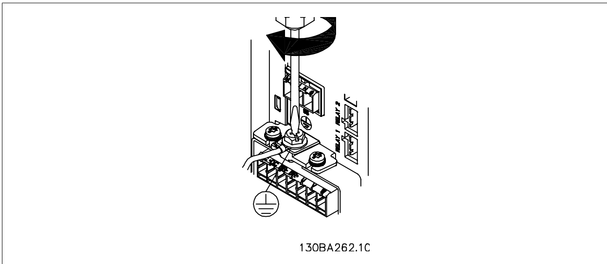
Ilustración 5.8: Cuando instale los cables, monte y ajuste en primer lugar el cable de tierra.
