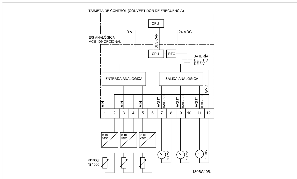
Ilustración 3.4: Esquema de principio para las E/S analógicas montadas en el convertidor de frecuencia.
