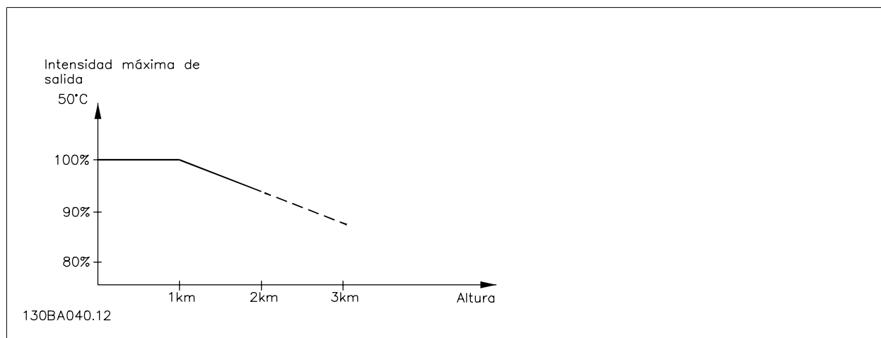
Ilustración 8.1: Reducción de la intensidad de salida en relación con la altitud a T_{AMB, MAX} . Para altitudes superiores a 2 km, póngase en contacto con Danfoss en relación con PELV.
