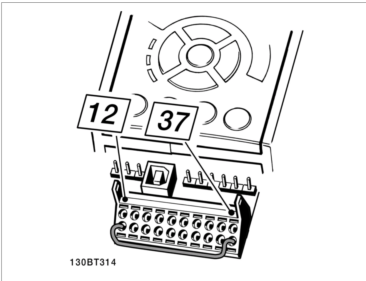
Ilustración 2.8: Puente de conexión entre el terminal 37 y 24 V CC.
