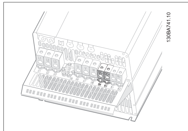
Ilustración 5.38: Conexiones de bus de CC para protección C4.
