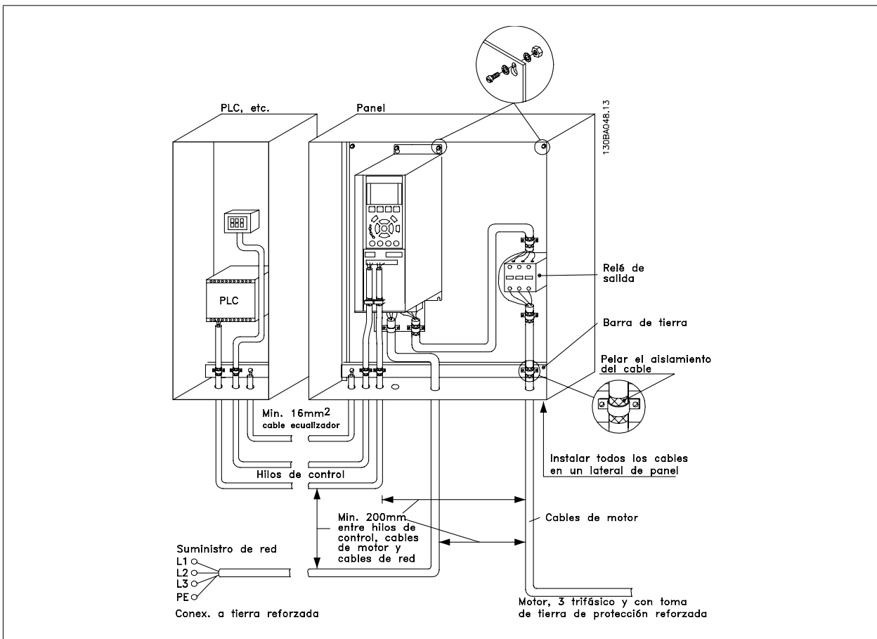
Ilustración 5.48: EMC - instalación eléctrica correcta de un convertidor de frecuencia en el alojamiento.
