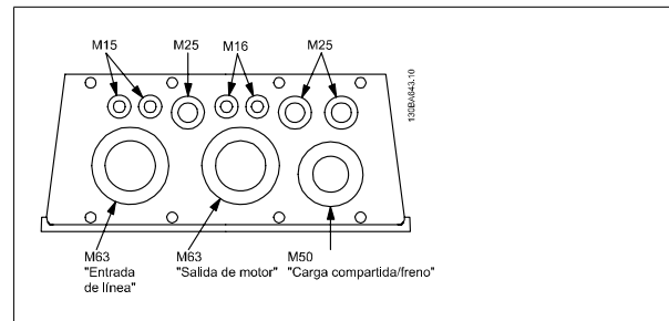
Ilustración 5.3: Orificios de entrada para cables en el armario C1. La utilización que se sugiere de los orificios es solo una recomendación, siendo posibles otras soluciones.
