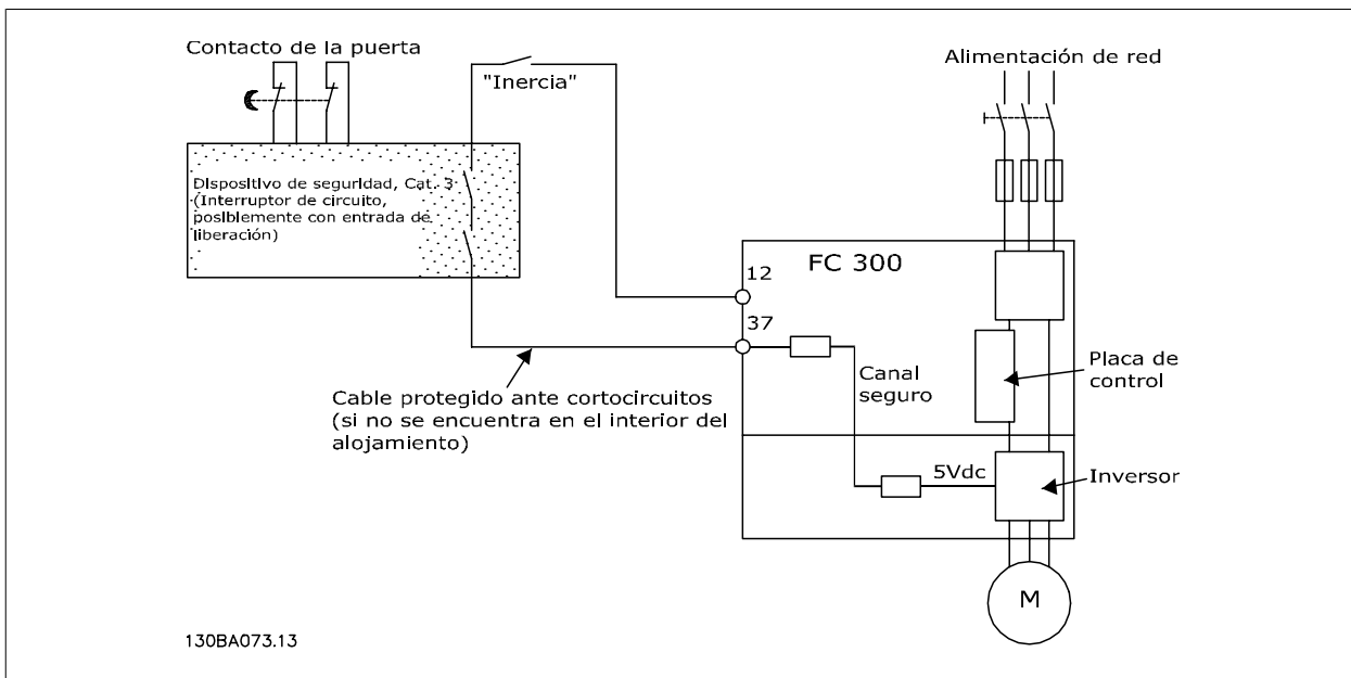
Ilustración 2.9: Ilustración de los aspectos esenciales de una instalación para lograr una parada de categoría 0 (EN 60204-1) con seguridad de categoría 3 (EN 954-1).
