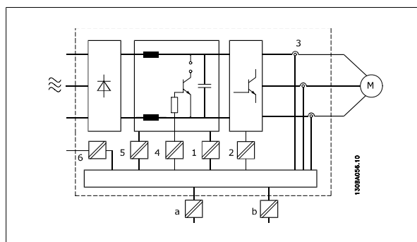
Ilustración 2.6: Aislamiento galvánico
