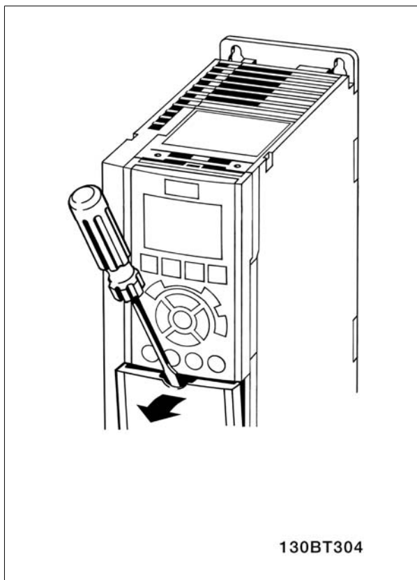
Ilustración 5.29: Armarios A1, A2, A3, B3, B4, C3 y C4
