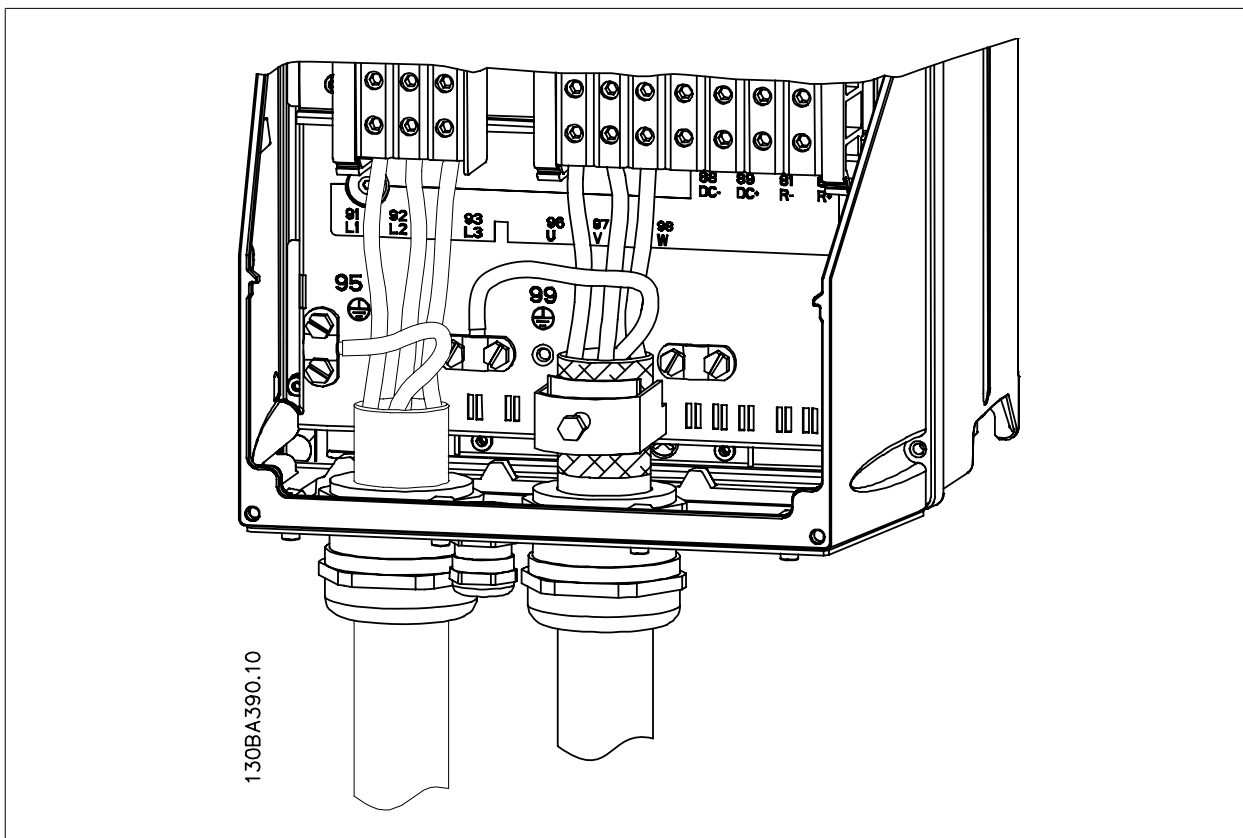
Ilustración 5.27: En primer lugar, termine la toma de tierra del motor y, a continuación, instale en sus terminales los cables U, V y W del motor y fíjelos. Asegúrese de que el aislamiento exterior del cable de motor esté retirado bajo la abrazadera EMC.
