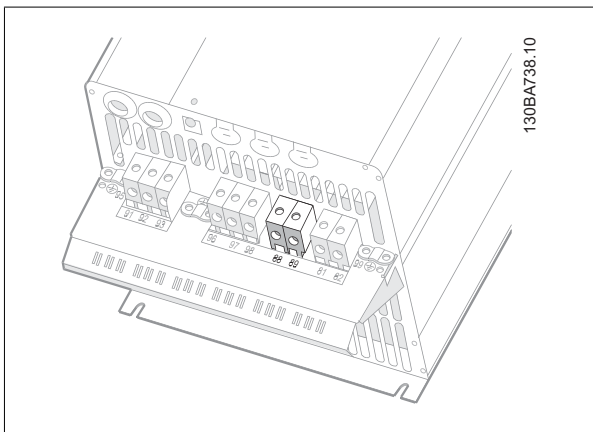
Ilustración 5.37: Conexiones de bus de CC para protección C3.
