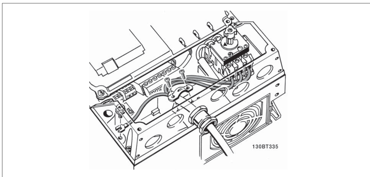
Ilustración 5.12: Cómo realizar la conexión a la red de alimentación y a tierra con interruptor de desconexión de la red.
