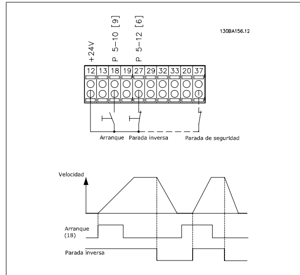
Ilustración 5.33: El terminal 37 sólo está disponible con la función de parada de seguridad
