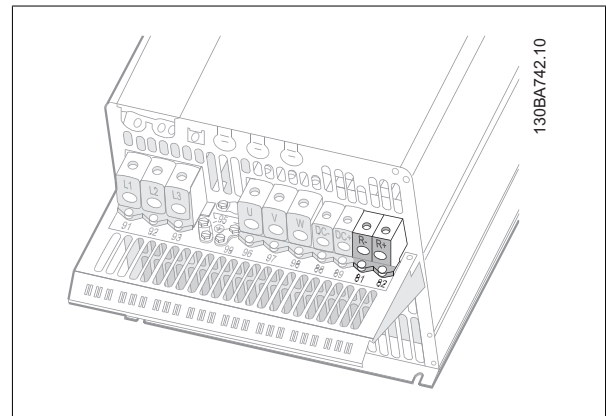
Ilustración 5.42: Terminal de conexión de freno para C4.
