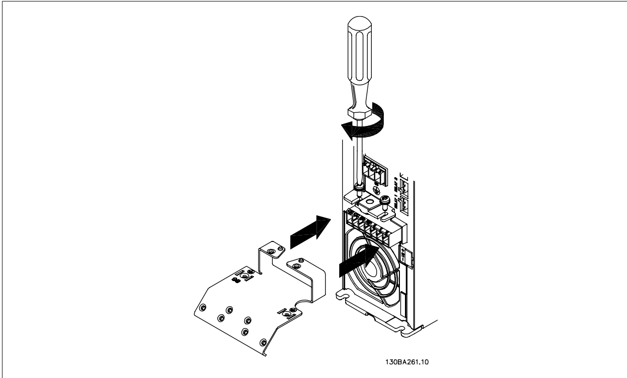
Ilustración 5.7: En primer lugar, coloque los dos tornillos de la placa de montaje, coloque la placa en su sitio y apriete los tornillos completamente.
