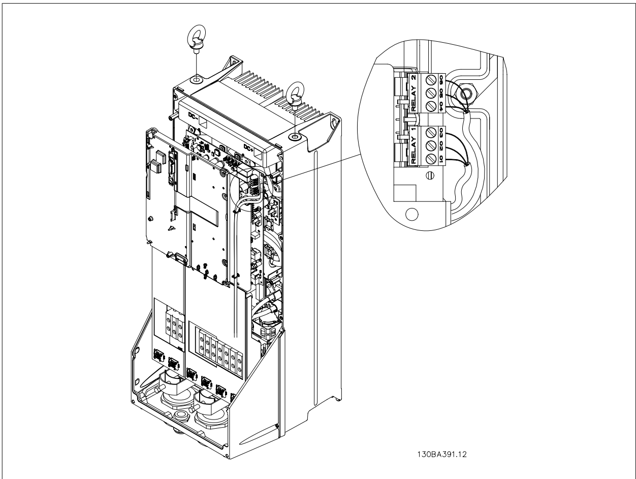
Ilustración 5.43: Terminales para conexión de relés (protecciones C1 y C2).
