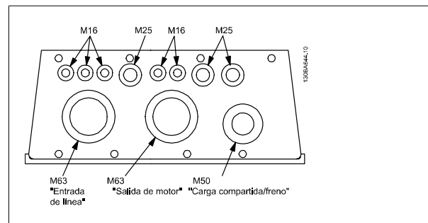
Ilustración 5.4: Orificios de entrada para cables en el armario C2. La utilización que se sugiere de los orificios es solo una recomendación, siendo posibles otras soluciones.
