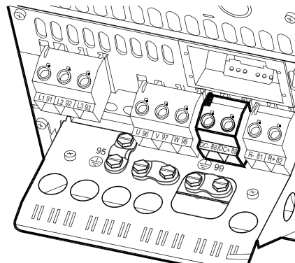
Bild 5.36: DC-bussanslutningar för kapsling B4.
