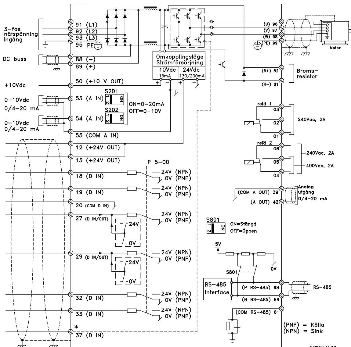
Bild 2.7: Diagram som visar alla elektriska plintar. (Plint 37 fungerar enbart med enheter som har funktionen säkerhetsstopp.)
