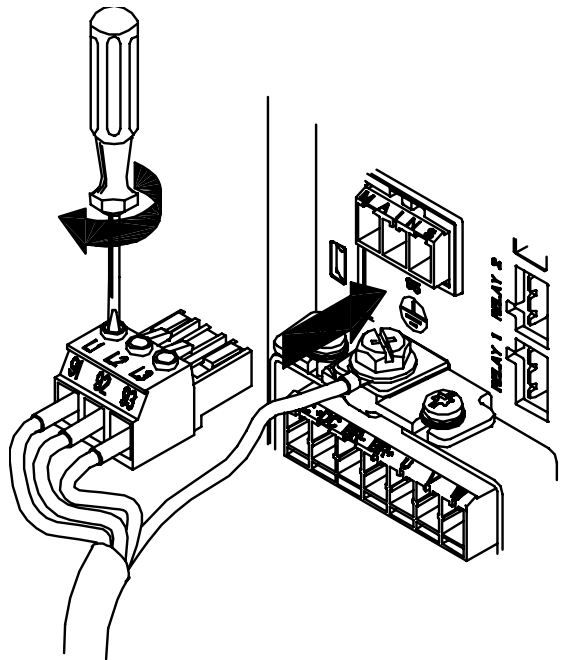
Bild 5.9: Montera sedan nätkontakten och dra åt skruvarna för kablarna.
