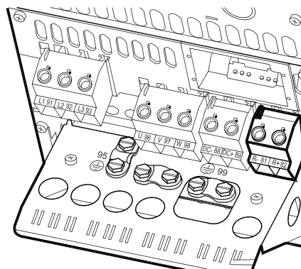
Bild 5.40: Bromsanslutningsplinten för B4.
