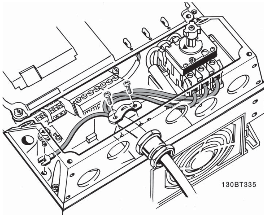
Bild 5.6: Så här ansluter du till nät och jordning med frånskiljare (A5-kapsling).
