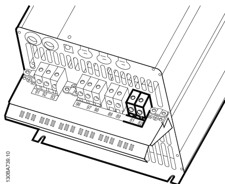
Bild 5.41: Bromsanslutningsplinten för C3.
