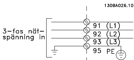
Bild 5.5: Plintar för nät och jordning.
