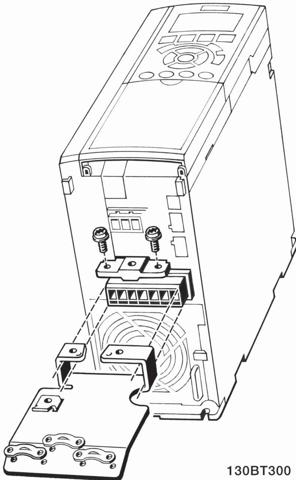
Bild 5.20: Montering av frånkopplingsplatta.
