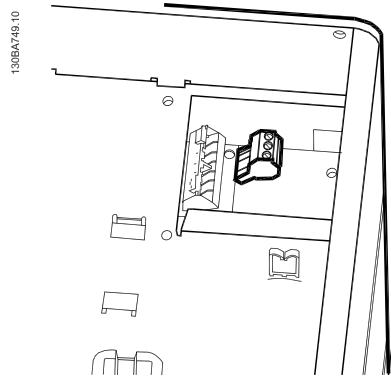
Bild 5.46: Plintar för reläanslutningar för C3 och C4. Sitter i det övre högra hörnet på frekvensomformaren.
