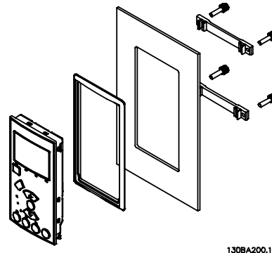
Bild 3.6: LCP-kit med numerisk LCP, fästdon och packning.
