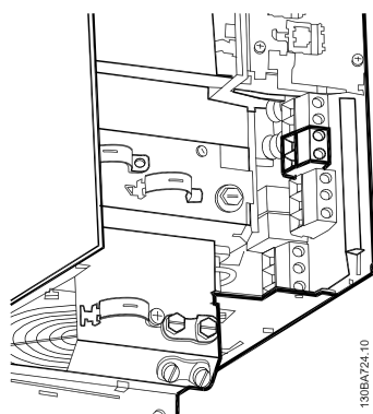
Bild 5.39: Bromsanslutningsplinten för B3.
