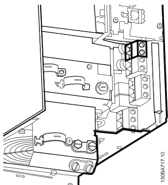
Bild 5.35: DC-bussanslutningar för kapsling B3.
