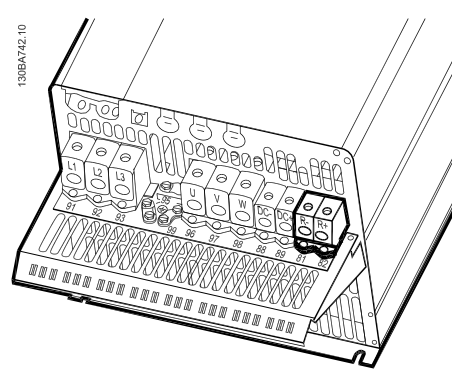
Bild 5.42: Bromsanslutningsplinten för C4.
