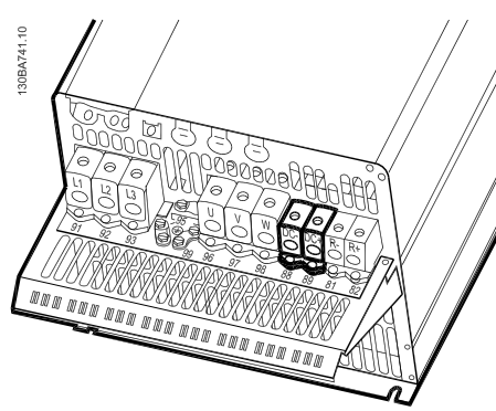
Bild 5.38: DC-bussanslutningar för kapsling C4.
