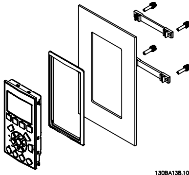
Bild 3.5: LCP-kit med grafisk LCP, fästdon, 3 m kabel och packning.
