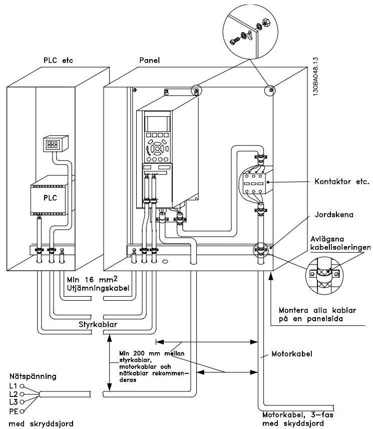
Bild 5.48: EMC-korrekt elektrisk installation av en frekvensomformare i apparatskåp.
