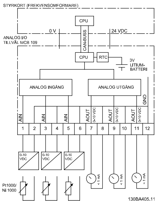
Bild 3.4: Principdiagram för analoga I/O som monterats i frekvensomformaren.
