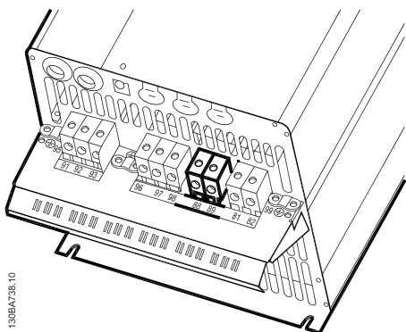
Bild 5.37: DC-bussanslutningar för kapsling C3.
