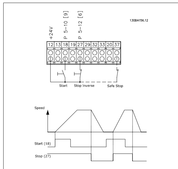
图 5.33: 端子 37 仅随安全停止功能一起提供!
