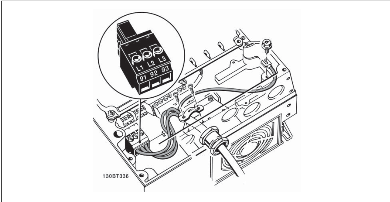
图 5.11: 如何在不使用主电源断路开关的情况下连接主电源和接地。注意, 需要使用电缆夹。
