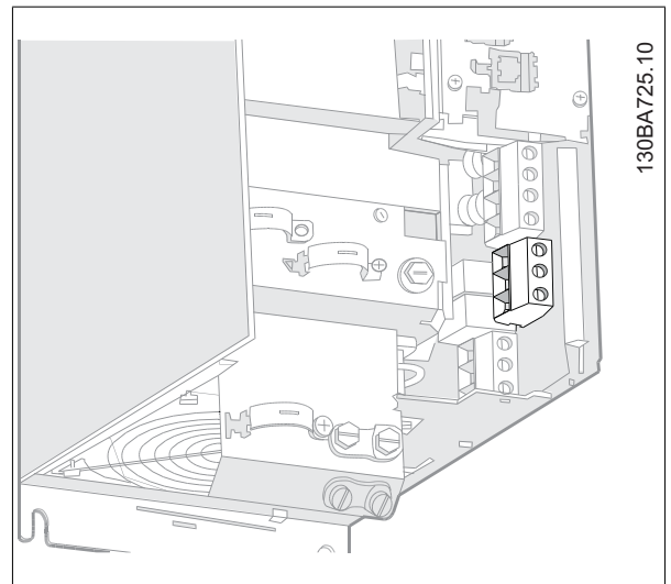
图 5.15: 如何连接不带 RFI 的 B3 的主电源和接地。
