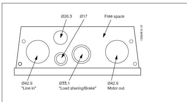
图 5.2: B2 机箱的电缆入口。入口的用途仅为建议，您也可以采用其它方案。
