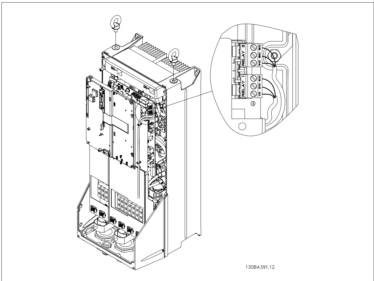
图 5.43: 继电器连接端子 (C1 和 C2 机箱) 显示的继电器连接位于安装有继电器插头 (位于附件包中) 的断开中。
