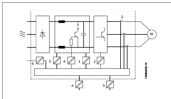
图 2.6: 高低压绝缘
