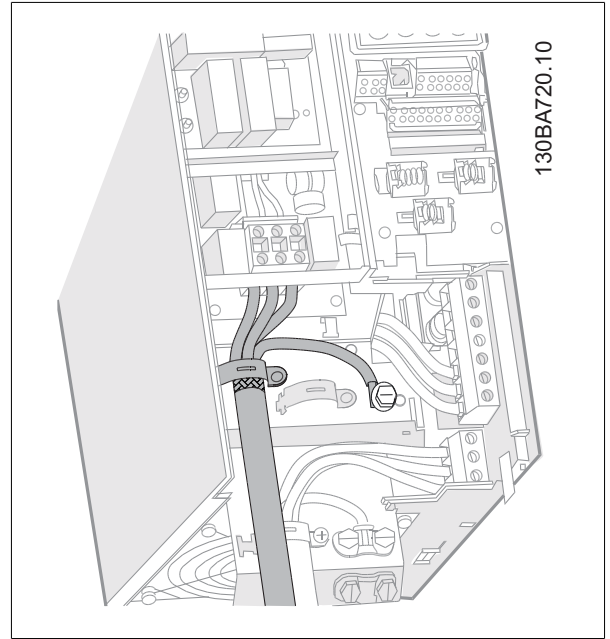
图 5.14: 如何连接带 RFI 的 B3 的主电源和接地。
