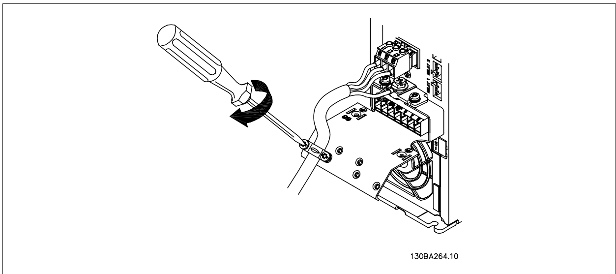
图 5.10: 最后, 拧紧主电源电线的支持架。
