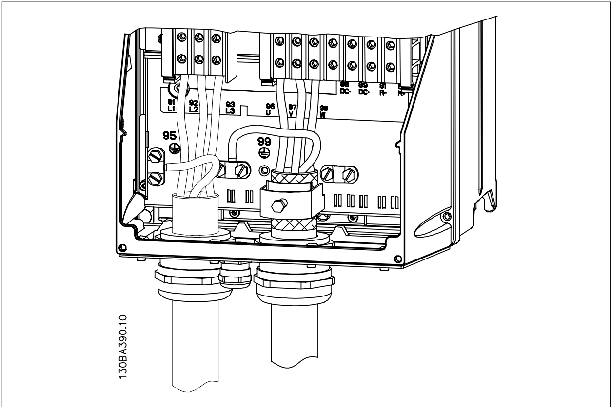
图 5.27: 首先, 断开电动机接地, 然后, 将电动机 U、V 和 W 电线接入端子并拧紧。请确保去除 EMC 电缆夹下面电动机电缆的外部绝缘层。
