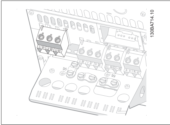
图 5.16: 如何连接 B4 的主电源和接地。
