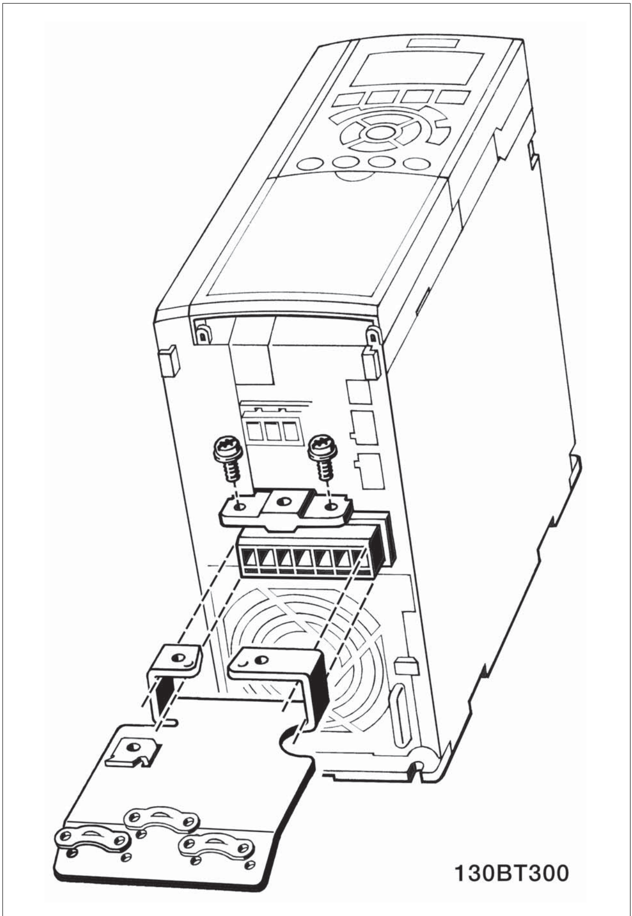
图 5.20: 安装去耦板。
