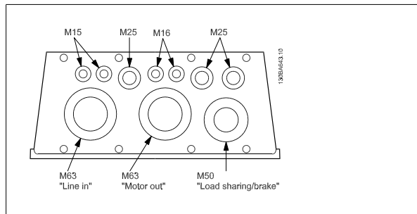
图 5.3: C1 机箱的电缆入口。入口的用途仅为建议，您也可以采用其它方案。
