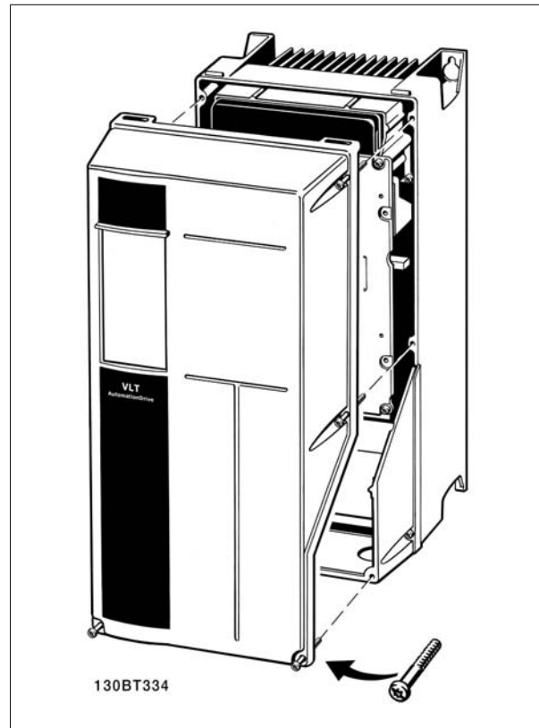
图 5.30: A5、B1、B2、C1 和 C2 机箱
