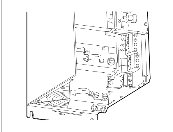
图 5.35: 机箱 B3 的直流总线连接。
