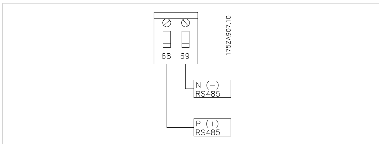
图 7.1：网络端子连接
