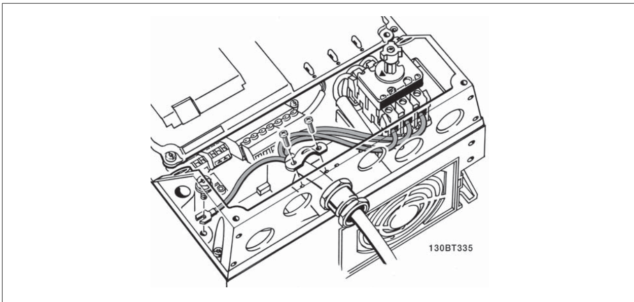
图 5.12: 如何使用主电源断路开关连接主电源和接地。
