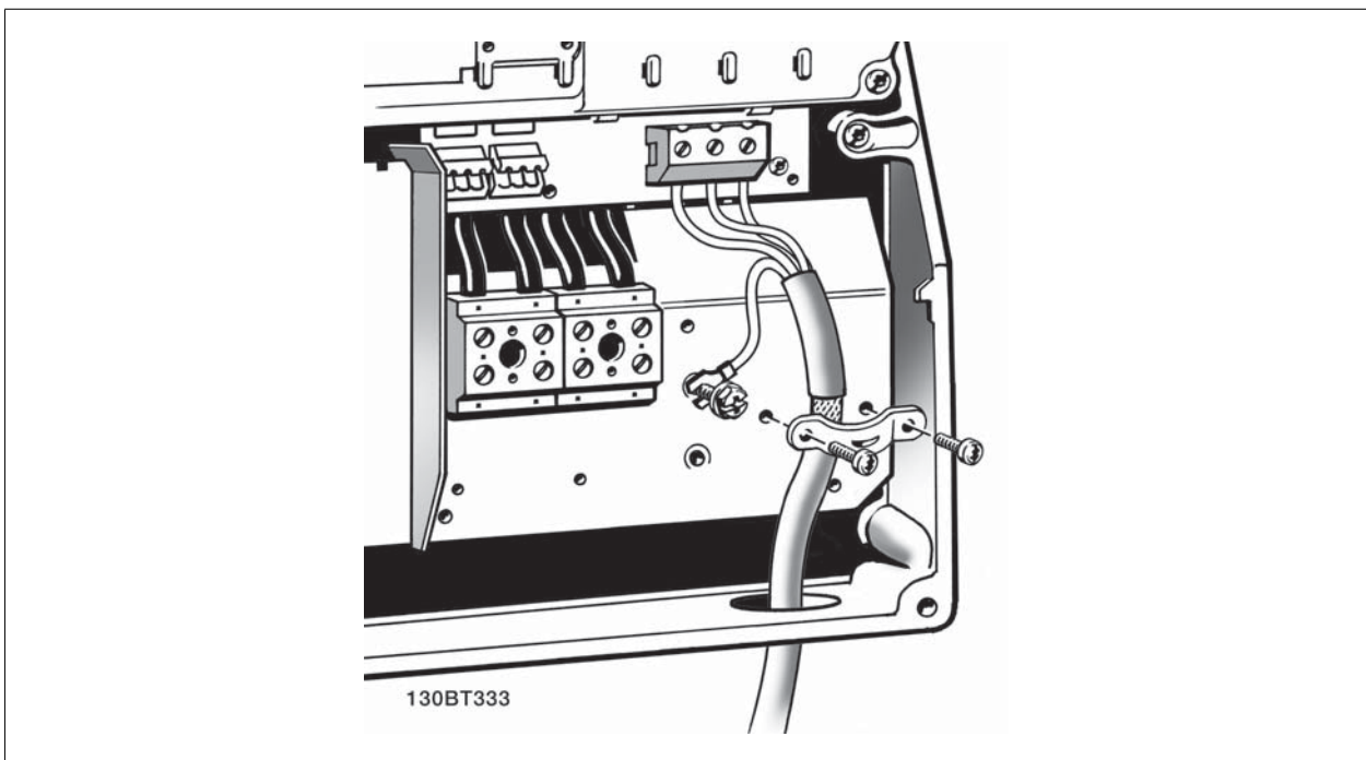
图 5.24: 首先, 断开电动机接地, 然后, 将电动机 U、V 和 W 电线接入端子并拧紧。请确保去除 EMC 电缆夹下面电动机电缆的外部绝缘层。
