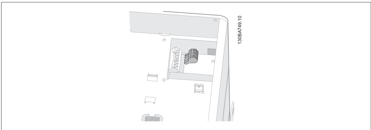
图 5.46: C3 和 C4 的继电器连接端子。位于变频器的右上角。
