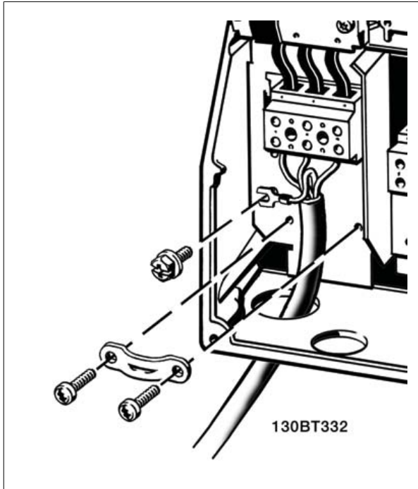
图 5.13: 如何连接 B1 和 B2 的主电源和接地。
