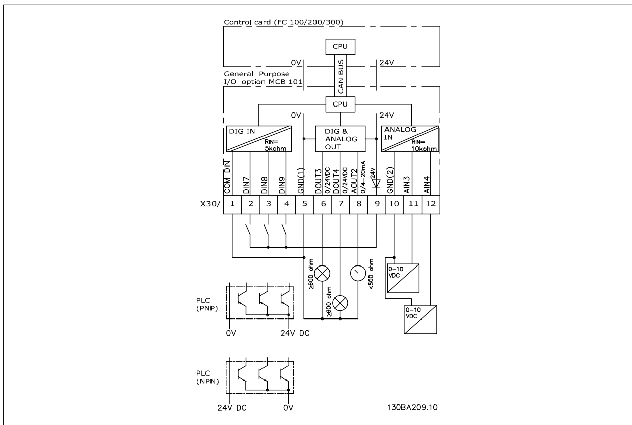
图 3.1: 原理图
