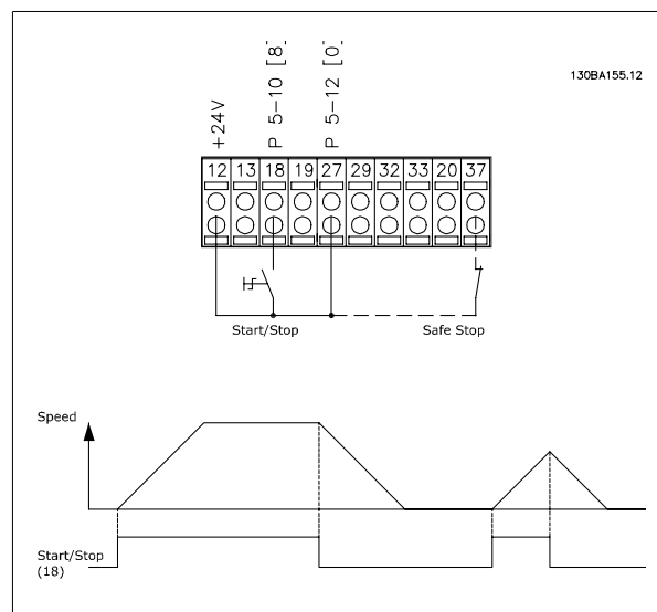
图 6.1: 端子 37: 仅随安全停止功能一起提供!
