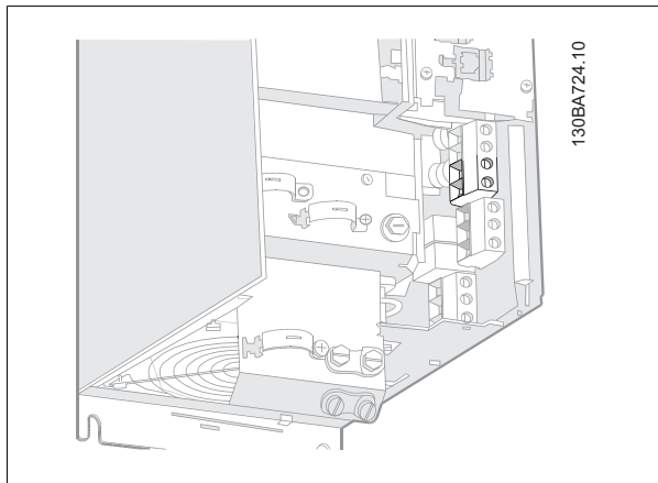
图 5.39: B3 的制动连接端子。
