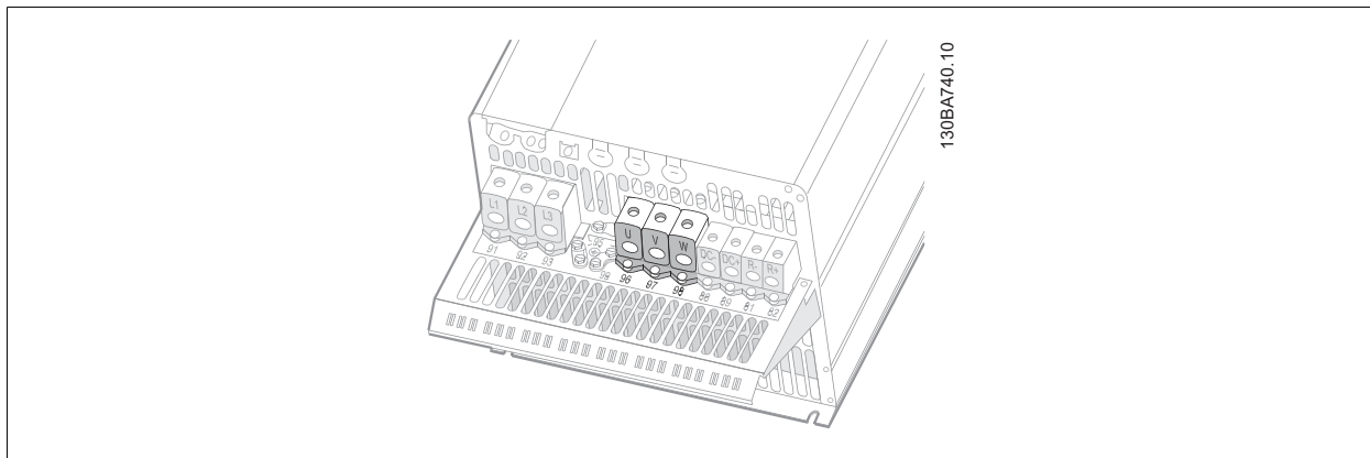
图 5.28: 首先, 断开电动机接地, 然后, 将电动机 U、V 和 W 电线接入端子并拧紧。请确保去除 EMC 电缆夹下面电动机电缆的外部绝缘层。
