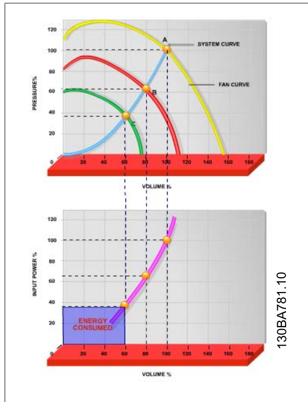
图 2.2: 使用变频器将风扇容量降低到 60% 时 - 在典型应用中可以达到超过 50% 的能量节省。
