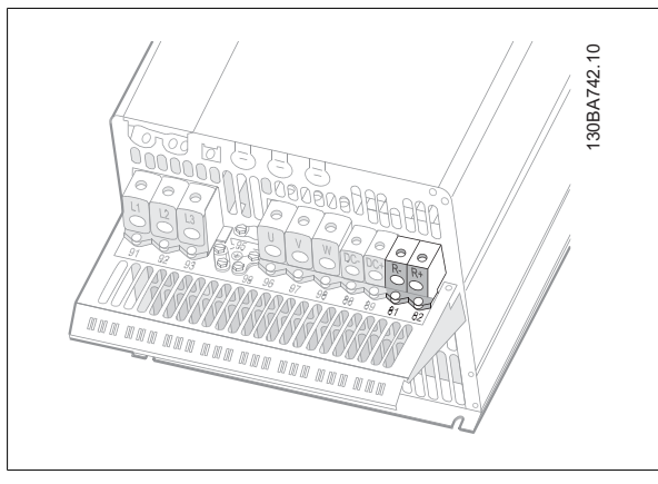
图 5.42: C4 的制动连接端子。
