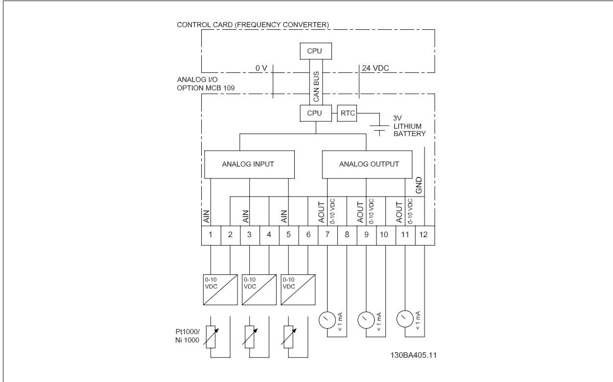
图 3.4: 安装在变频器中的模拟输入输出的原理图。
