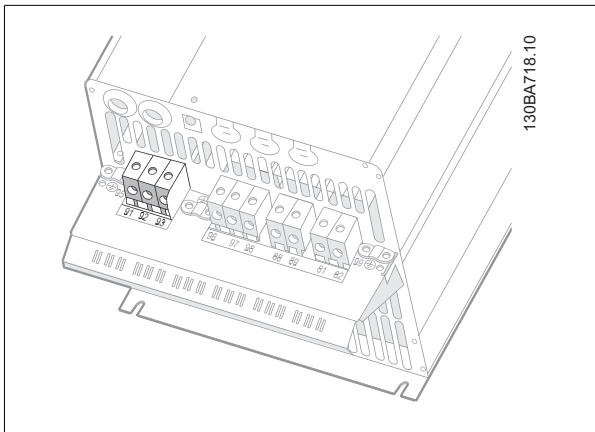
图 5.18: 如何连接 C3 的主电源和接地。
