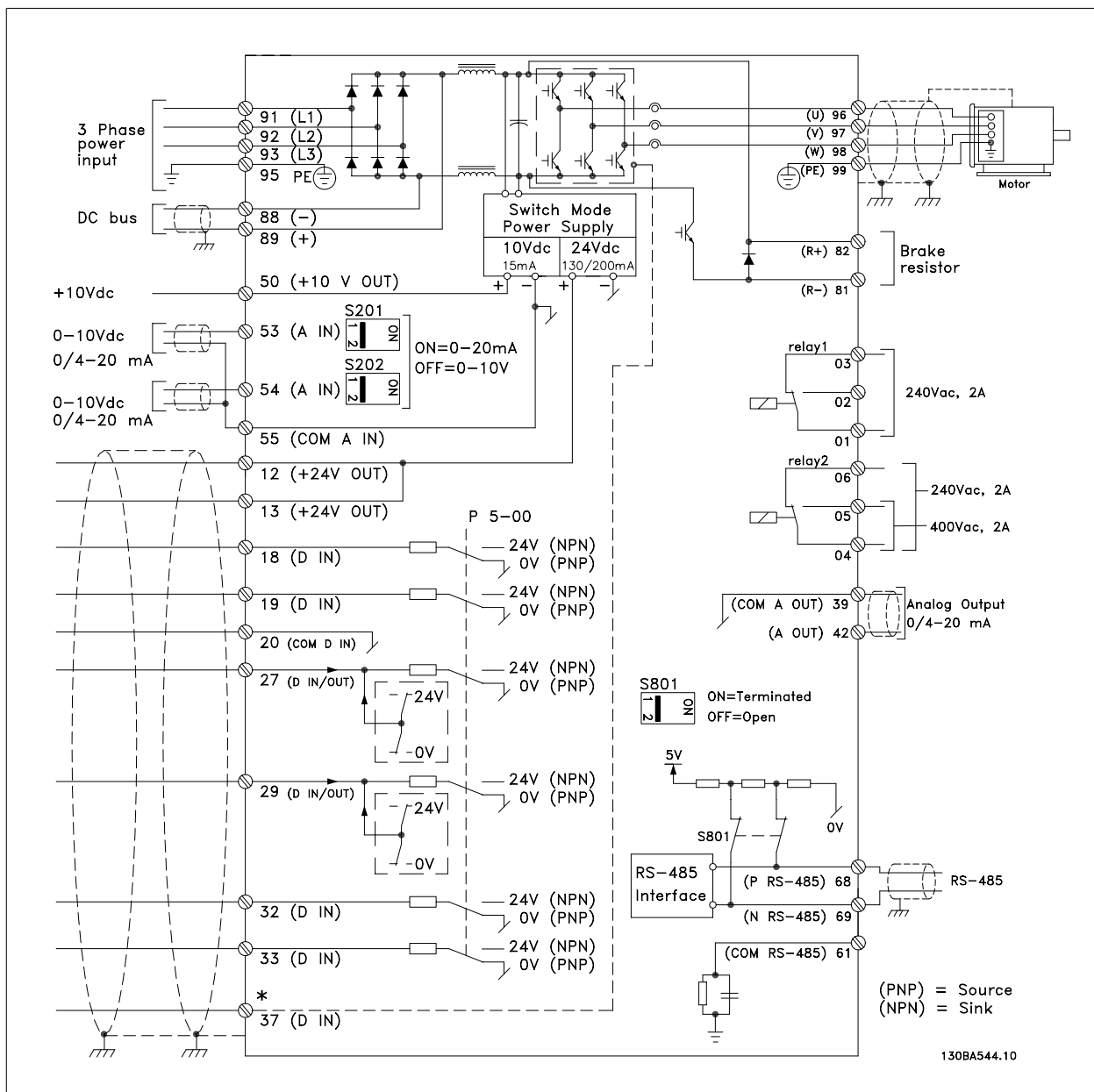
图 5.34: 图示显示了所有电气端子。(仅带有安全停止功能的设备才提供端子 37。)
