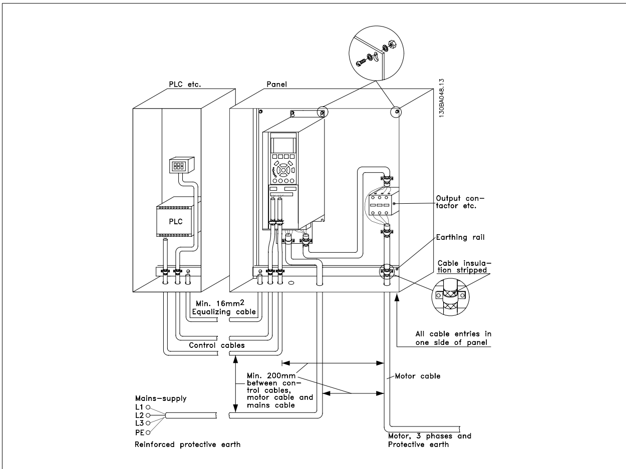
图 5.48: 在机柜中对变频器执行符合 EMC 规范的电气安装。
