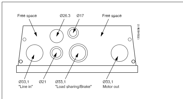
图 5.1: B1 机箱的电缆入口。入口的用途仅为建议，您也可以采用其它方案。
