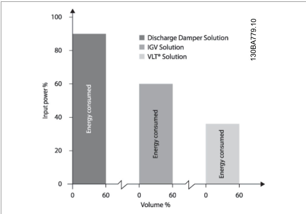
图 2.4: 排风阀会在某种程度上降低能耗。入口导流箱提供了 40% 的降低, 但安装费用昂贵。Danfoss VLT® 解决方案降低能耗超过 50% 并且安装简便。
