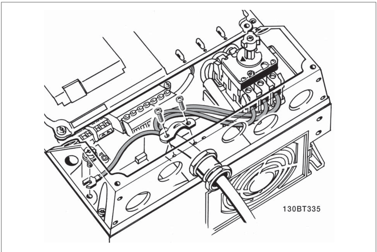
图 5.6: 如何使用断路器连接主电源和接地（A5 机箱）。
