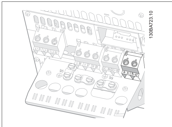
图 5.40: B4 的制动连接端子。
