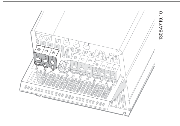
图 5.19: 如何连接 C4 的主电源和接地。
