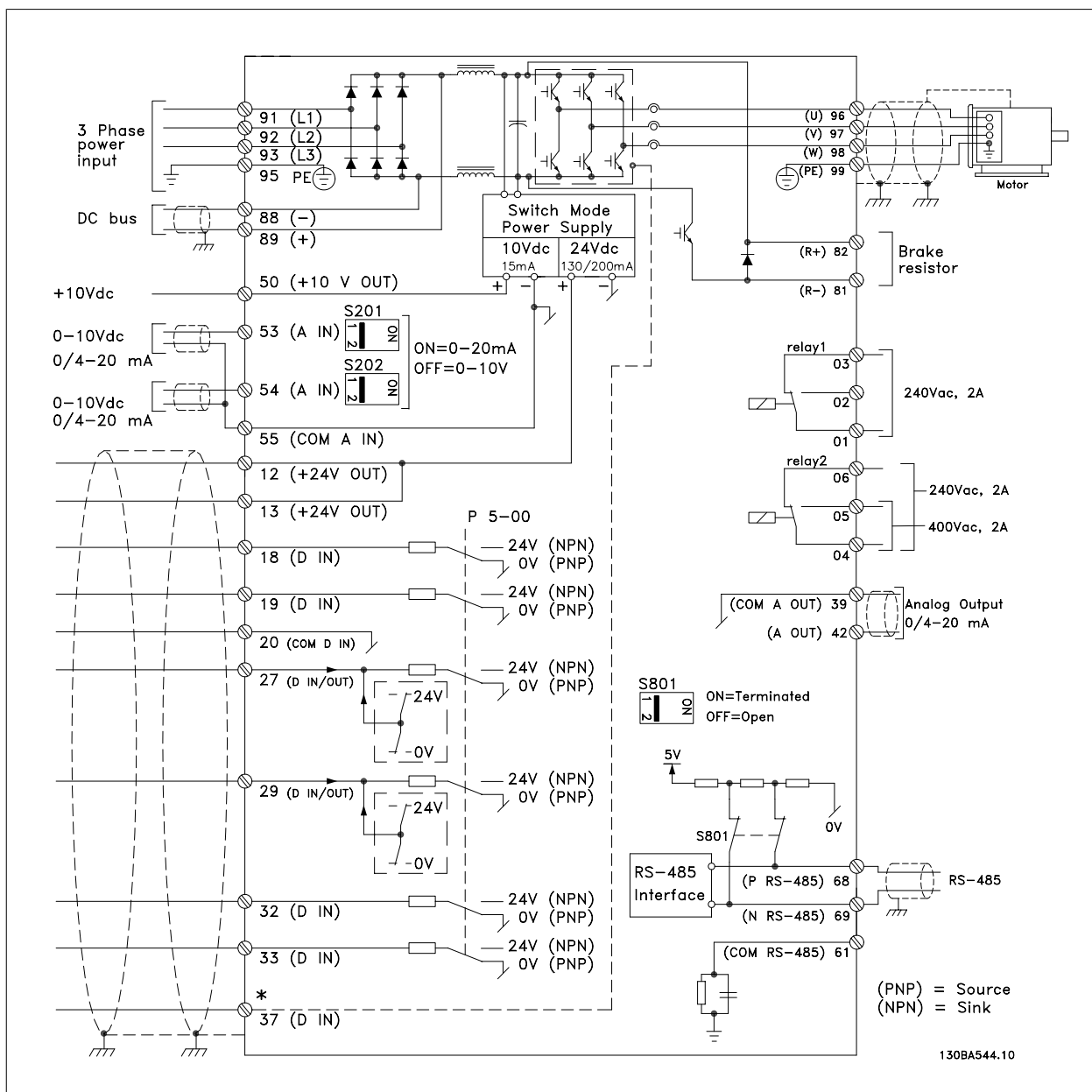
图 2.7: 图示显示了所有电气端子。（仅带有安全停止功能的设备才提供端子 37。）
