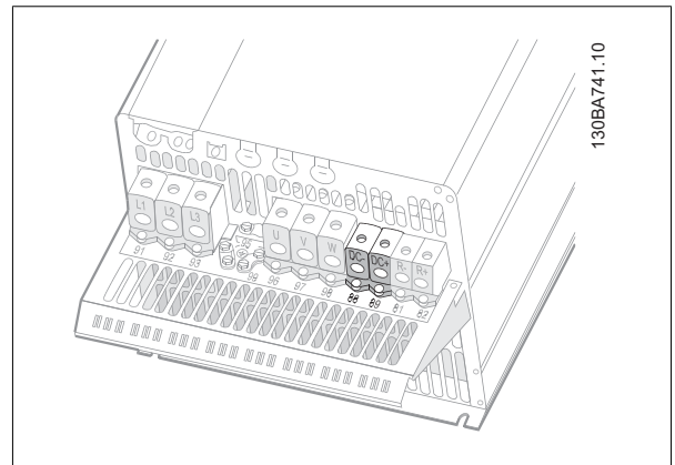
图 5.38: 机箱 C4 的直流总线连接。
