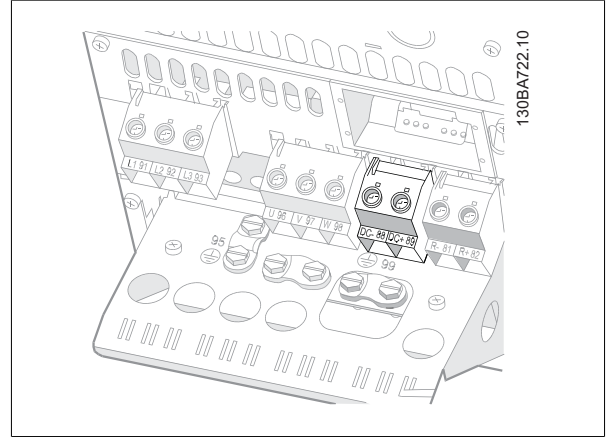
图 5.36: 机箱 B4 的直流总线连接。
