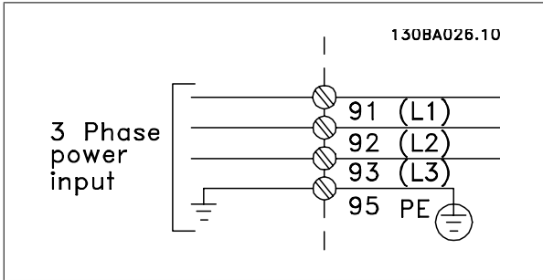
图 5.5: 主电源端子和接地端子。
