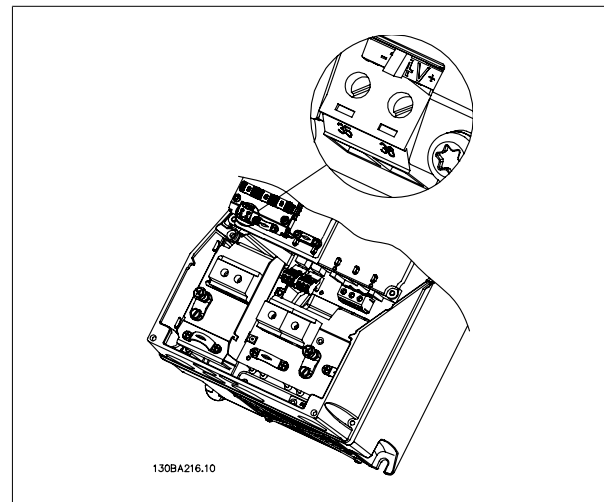
图 3.3: 24 V 备用电源的连接 (A5-C2)。
