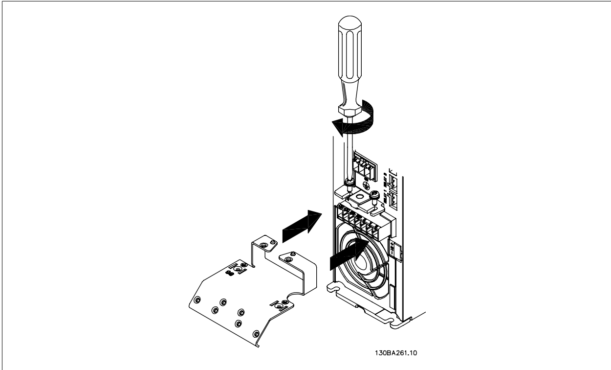
图 5.7: 首先, 将两个螺钉安装到固定板上, 然后将其滑动入位并完全拧紧。
