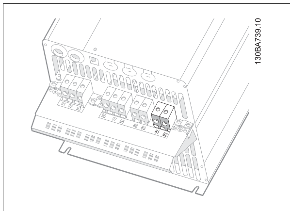
图 5.41: C3 的制动连接端子。
