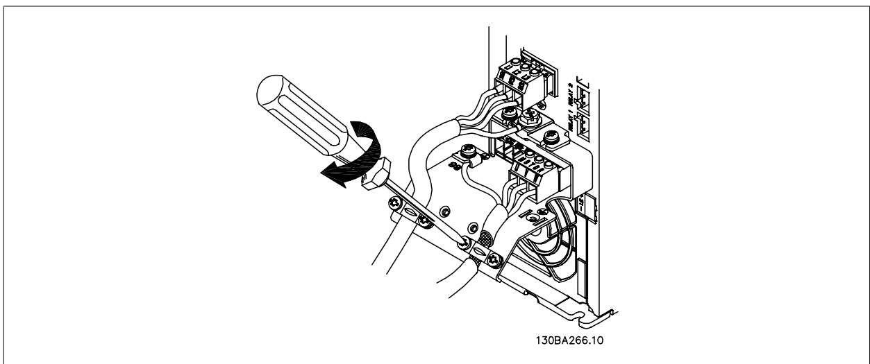
图 5.22: 安装电缆夹, 以确保机架和屏蔽丝网达到 360 度连接。注意, 请去除电缆夹下面电动机电缆的外部绝缘层。
