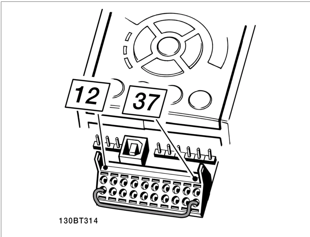
图 2.8: 端子 37 和 24 VDC 之间的桥接器 (跳线)
