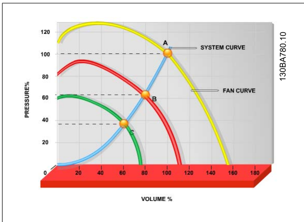
图 2.1: 下图显示了降低风扇容量时的风扇曲线（A、B 和 C）。
