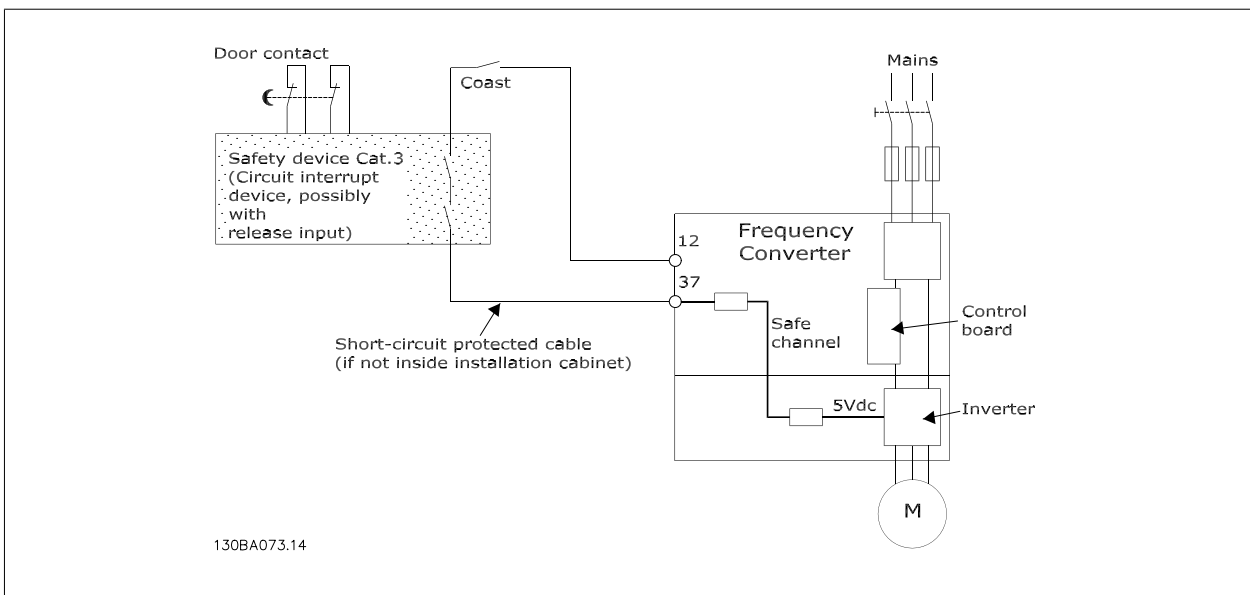
图 2.9: 符合安全类别 3 (EN 954-1) 停止类别 0 (EN 60204-1) 的安装基本配置的简图。
