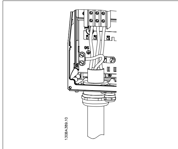
图 5.17: 如何连接 C1 和 C2 的主电源和接地。
