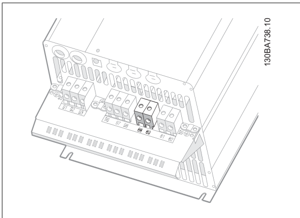
图 5.37: 机箱 C3 的直流总线连接。
