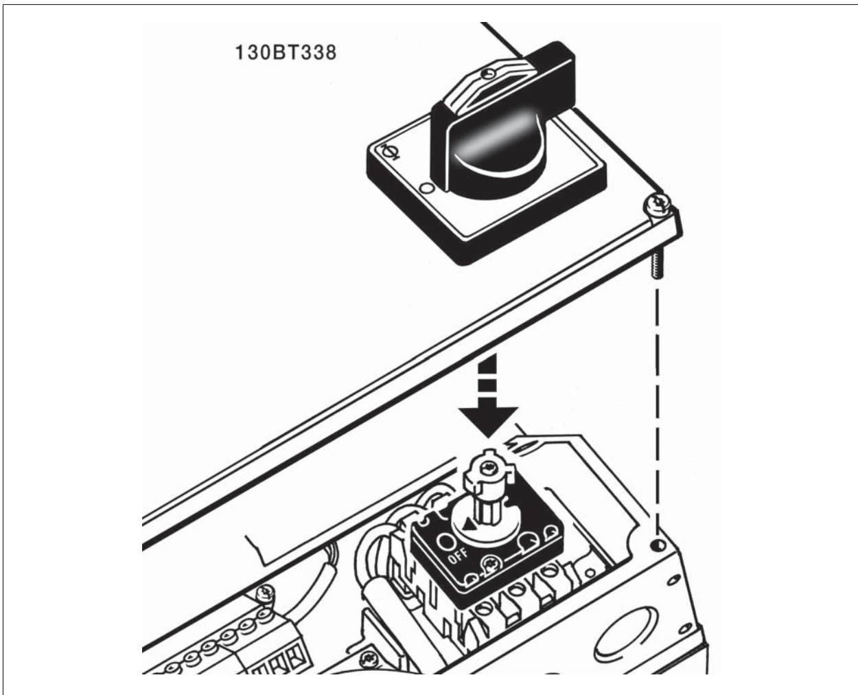
图 5.32: 装配带有主电源断路器的 IP21 / IP55 / NEMA TYPE 12 机箱。
