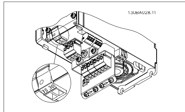
图 3.2: 24 V 备用电源的连接 (A2-A3)。
