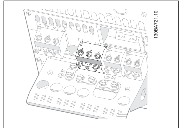
图 5.26: 首先, 断开电动机接地, 然后, 将电动机 U、V 和 W 电线接入端子并拧紧。请确保去除 EMC 电缆夹下面电动机电缆的外部绝缘层。
