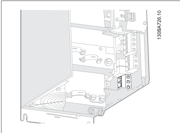
图 5.25: 首先, 断开电动机接地, 然后, 将电动机 U、V 和 W 电线接入端子并拧紧。请确保去除 EMC 电缆夹下面电动机电缆的外部绝缘层。
