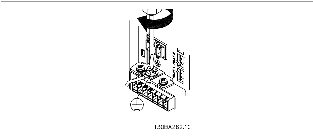
图 5.8: 安装电缆时, 首先安装并拧紧接地电线。
