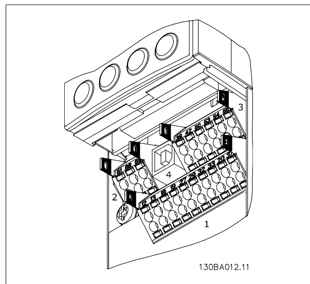
图 5.31: 控制端子（所有机箱）
