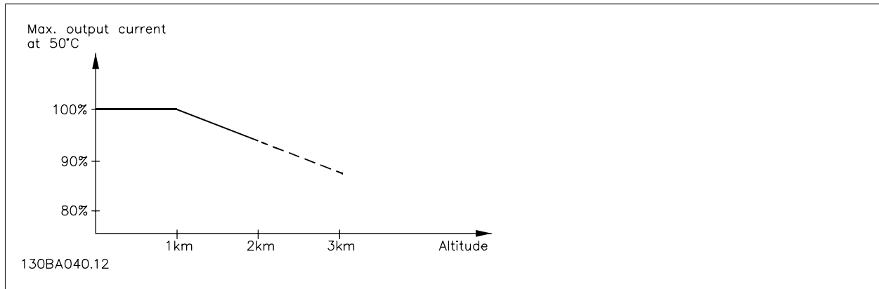
图 8.1: 在 T_{AMB, MAX} 下，输出电流降容与海拔的关系。当海拔超过 2 km 时，请向 Danfoss 咨询 PELV 事宜。
