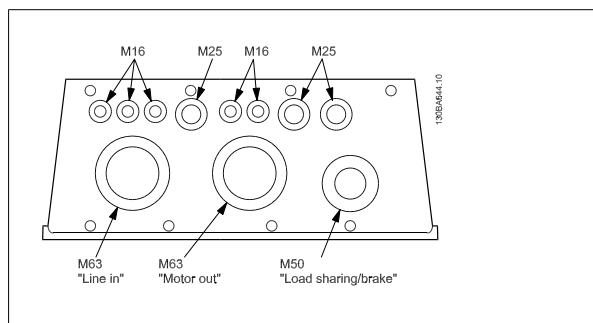
图 5.4: C2 机箱的电缆入口。入口的用途仅为建议，您也可以采用其它方案。
