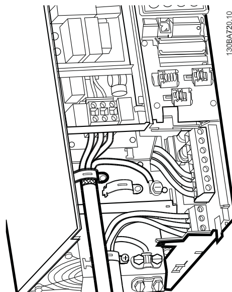
Bild 5.17: Så här ansluter du till nät och jordning för B3 med RFI.
