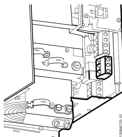
Bild 5.16: Anslutning till nät och jordning för B3 utan RFI.
