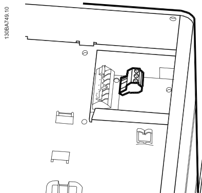
Bild 5.49: Plintar för reläanslutningar för C3 och C4. Sitter i det övre högra hörnet på frekvensomformaren.
