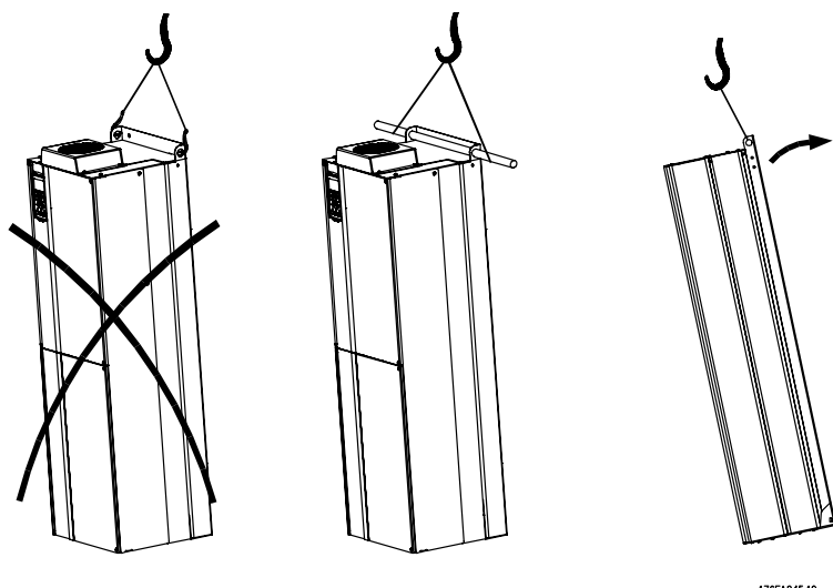
Bild 5.1: Tyngre frekvensomformare ska lyftas med lyft. Vägghontera först de två nedre bultarna. Lyft sedan frekvensomformaren upp på de nedre bultarna. Fäst slutligen frekvensomformaren mot väggen med de två övre bultarna.
