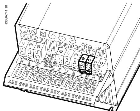
Bild 5.41: Likströmsbussanslutningar för kapsling C4.
