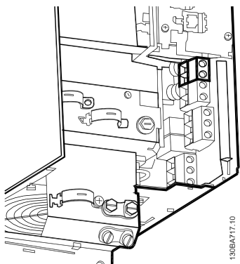
Bild 5.38: Likströmsbussanslutningar för kapsling B3.
