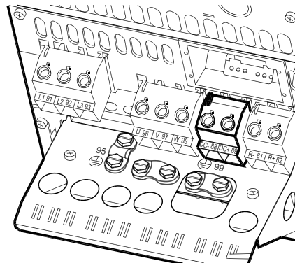
Bild 5.39: Likströmsbussanslutningar för kapsling B4.
