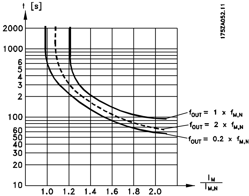
Bild 2.7: X-axeln visar förhållandet mellan I_{motor} och I_{motor} nominellt. Y-axeln visar tiden i sekunder innan ETR stänger av och trippar frekvensomformaren. Kurvorna visar det karakteristiska nominella varvtalet vid dubbla det nominella varvtalet och vid 0,2 x det nominella motorvarvtalet.
