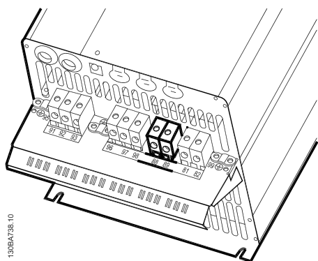
Bild 5.40: Likströmsbussanslutningar för kapsling C3.
