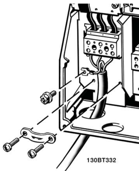
Bild 5.15: Så här ansluter du till nät och jordning för B1 och B2
