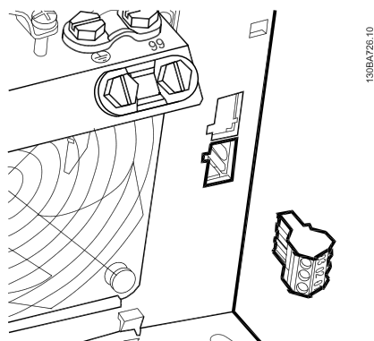
Bild 5.47: Plintar för reläanslutning för B3. Endast en håltagning är monterad från fabrik.
