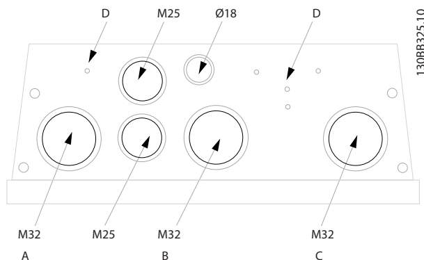
Abbildung 5.9 Kabeleingänge für Gehäuse B1. Die vorgeschlagenen Verwendungszwecke der Bohrungen sind reine Empfehlungen; andere Lösungen können ebenfalls umgesetzt werden.
