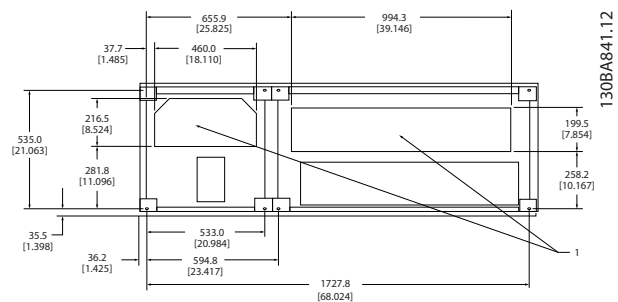
Abbildung 5.18 Baugröße F2
