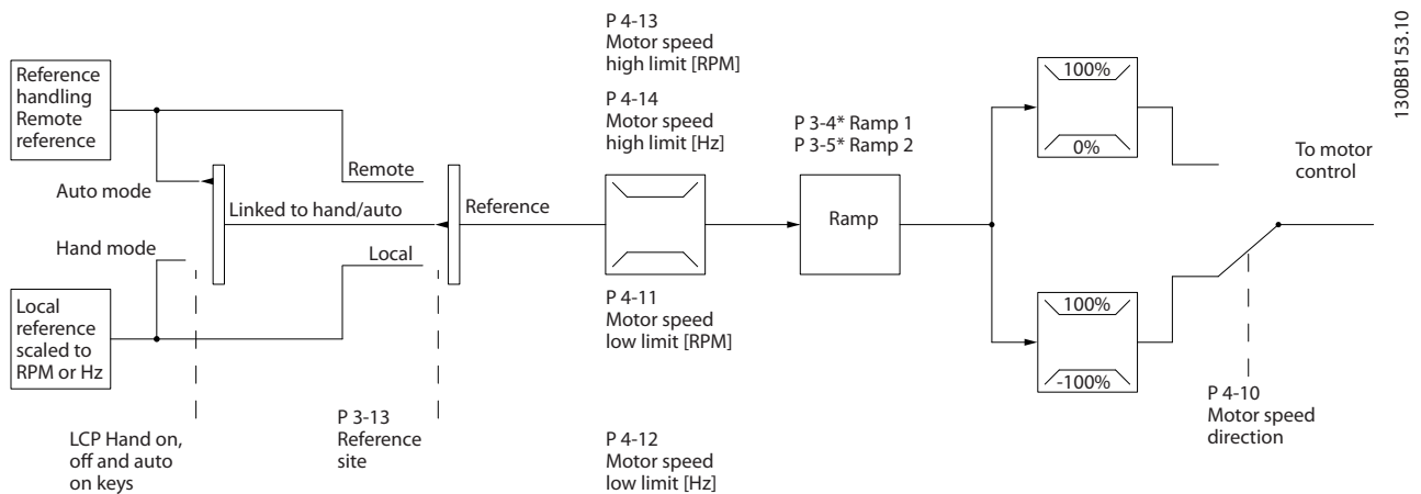
Abbildung 2.10 Struktur ohne Rückführung.
