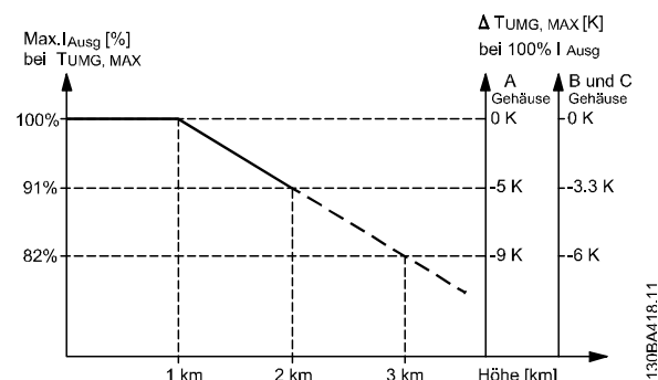
Abbildung 8.2 Leistungsreduzierung des Ausgangsstroms in Bezug auf die Höhe T_{AMB, MAX} für die Baugrößen A, B und C. Wenden Sie sich bei einer Installation in einer Höhe von mehr als 2 km hinsichtlich PELV (Protective extra low voltage / Schutzkleinspannung) an Danfoss.
