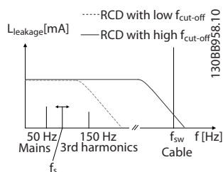
Abbildung 2.17 Zeichnung der Hauptbeitragsfaktoren zum Erdableitstrom
