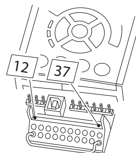
Abbildung 2.2 Kabelbrücke (Jumper) zwischen Klemme 37 und Klemme 12 (24 V DC)
