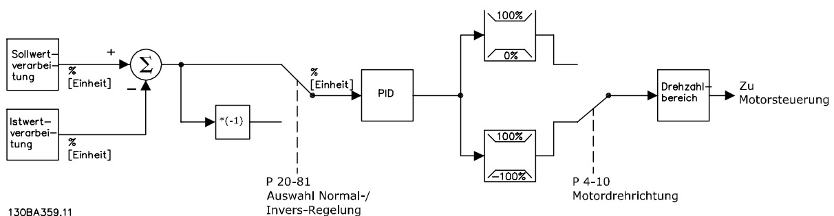
Abbildung 2.11 Blockschaltbild des Reglers
