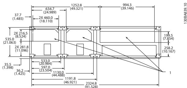
Abbildung 5.20 Baugröße F4
