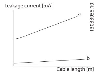
Abbildung 2.15 Prinzipschaltbild zeigt die Beeinflussung des Erdableitstroms durch die Kabellänge und Leistungsgröße. Pa > Pb.
