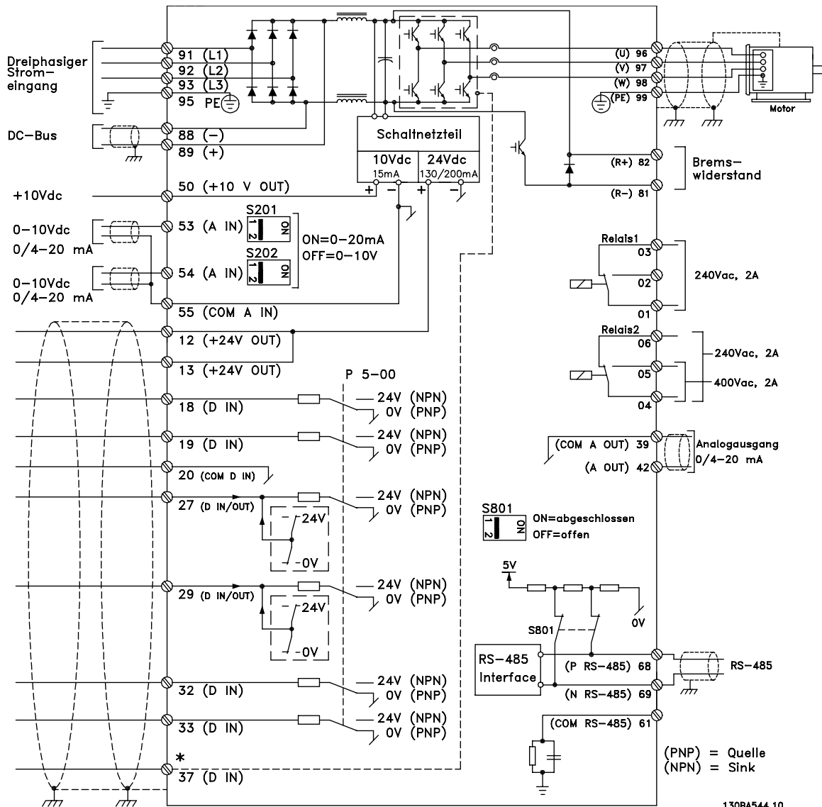
Abbildung 5.23 Schaltbild mit allen elektrischen Klemmen.
