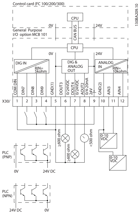
Abbildung 3.3 Prinzipschaltbild
