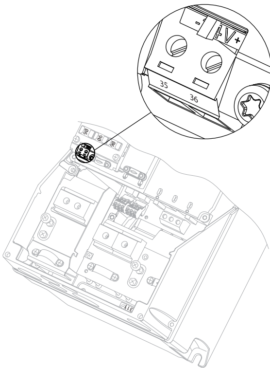
Abbildung 3.5 Anschluss an die 24-V-Backup-Versorgung (A5-C2).
