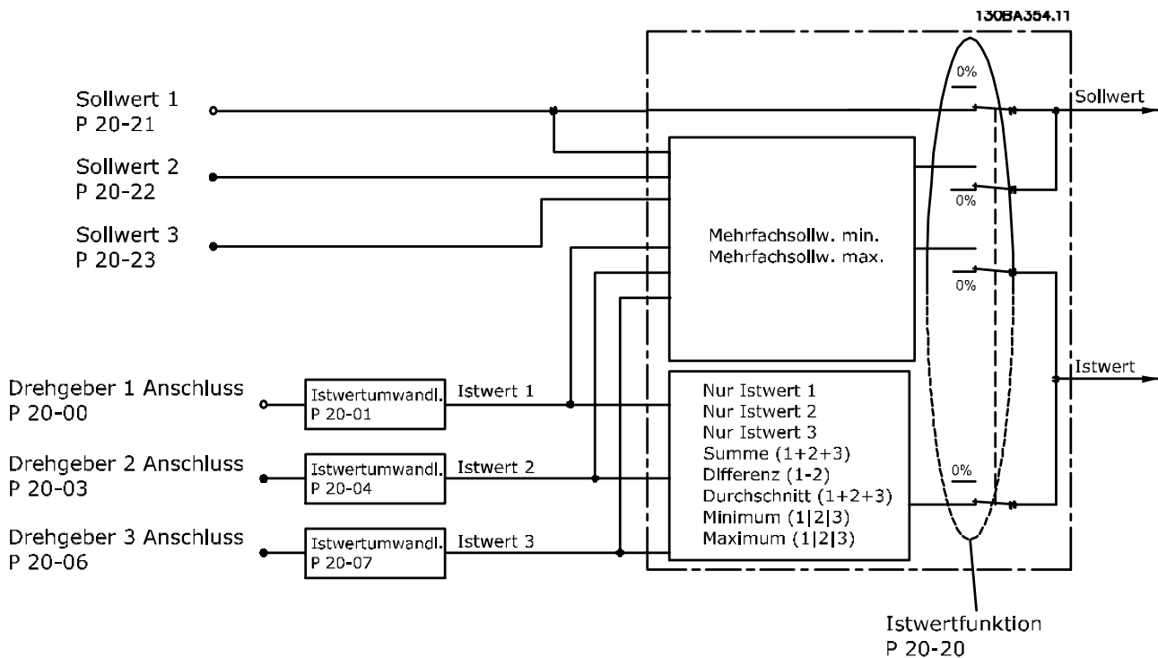
Abbildung 2.12 Blockschaltbild der Istwertsignalverarbeitung
