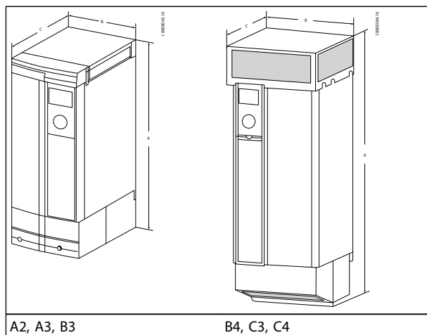
Gehäuse A3
