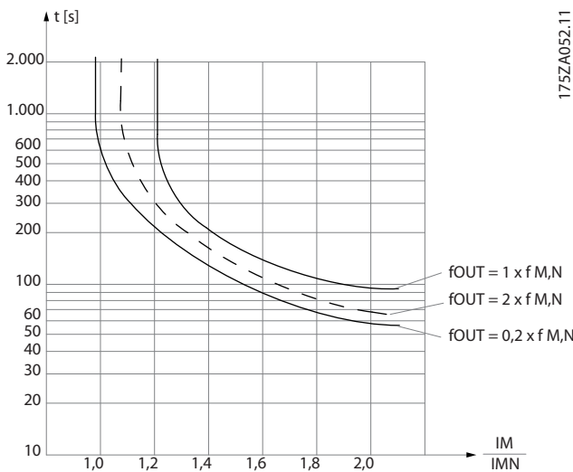
Abbildung 2.19 Die X-Achse zeigt das Verhältnis zwischen I_{Motor} und I_{MN} . Die Y-Achse zeigt die Zeit in Sekunden, bevor ETR eingreift und den Frequenzumrichter abschaltet. Die Kennlinien zeigen das Verhalten der Nenndrehzahl bei Nenndrehzahl x 0,2 und Nenndrehzahl x 2.
