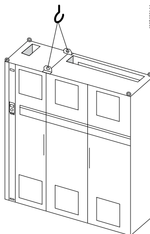
Abbildung 5.3 Empfohlene Hubmethode, Baugröße F2 (460 V, 1000 bis 1200 HP, 575/690 V, 1250 bis 1350 HP).
