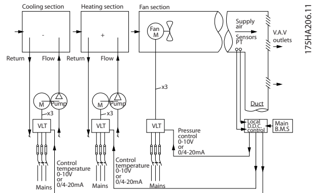
Abbildung 2.8 In der Abbildung ist ein durch Frequenzumrichter geregeltes Lüftersystem dargestellt.
