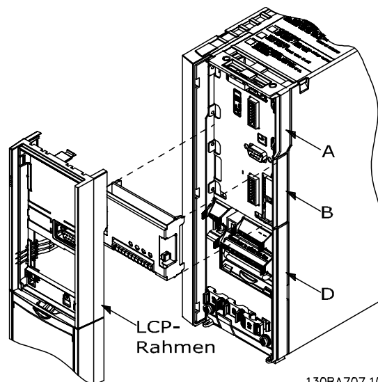
Abbildung 3.1 Gehäuse A2, A3 und B3
