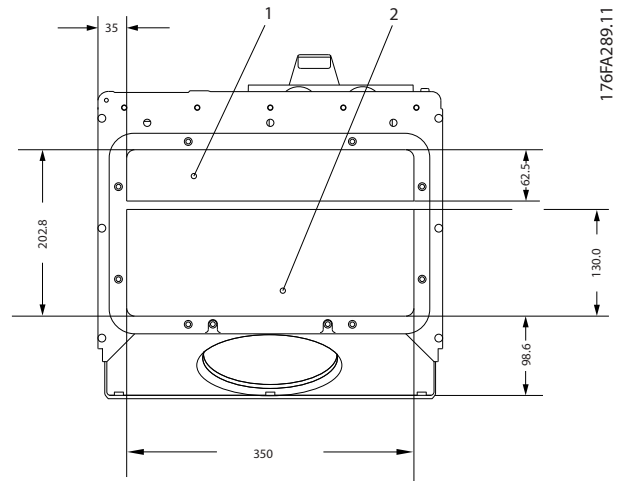
Abbildung 5.16 Baugröße E1
