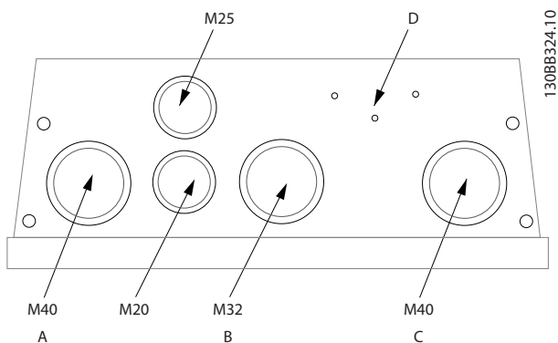
Abbildung 5.11 Kabeleingänge für Gehäuse B2. Die vorgeschlagenen Verwendungszwecke der Bohrungen sind reine Empfehlungen; andere Lösungen können ebenfalls umgesetzt werden.
