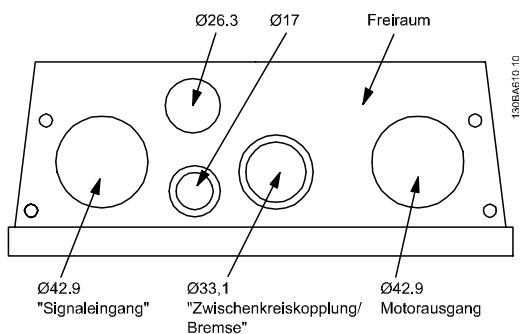
Abbildung 5.10 Kabeleingänge für Gehäuse B2. Die vorgeschlagenen Verwendungszwecke der Bohrungen sind reine Empfehlungen; andere Lösungen können ebenfalls umgesetzt werden.
