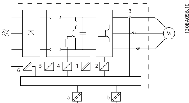
Abbildung 2.14 Galvanische Trennung
