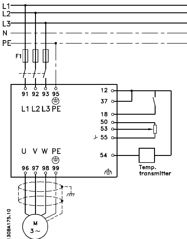
Abbildung 5.26 Elektrisches Anschlussbild.
