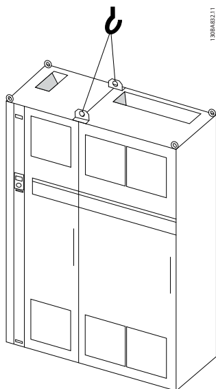
Abbildung 5.2 Empfohlene Hubmethode, Baugröße F1 (460 V, 600 bis 900 HP, 575/690 V, 900 bis 1150 HP).
