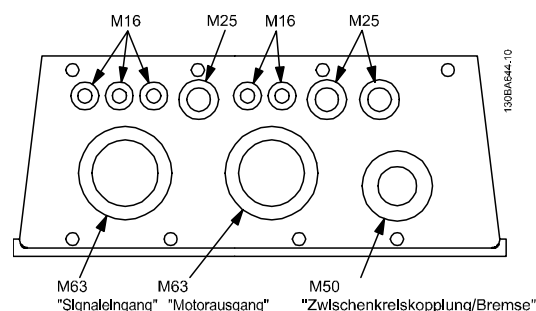
Abbildung 5.13 Kabeleingänge für Gehäuse C2. Die vorgeschlagenen Verwendungszwecke der Bohrungen sind reine Empfehlungen; andere Lösungen können ebenfalls umgesetzt werden.
