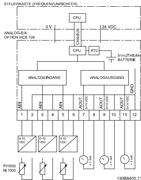
Abbildung 3.6 Prinzipschaltbild für Analogen I/O im Frequenzumrichter.
