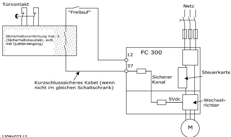
Abbildung 2.3 Abbildung der wesentlichen Aspekte einer Installation, um Stoppkategorie 0 (EN 60204-1) mit Sicherheitskategorie 3 (EN 954-1) zu erzielen.
