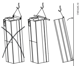
Abbildung 5.1 Empfohlene Hubmethode, Baugrößen D und E .
