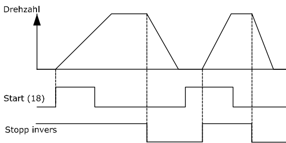
Abbildung 5.22 Klemme 37 nur mit Sicherer Stopp-Funktion verfügbar!
