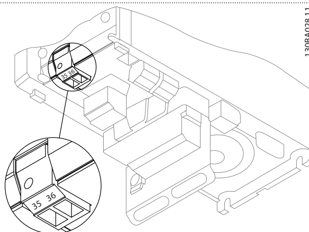
Abbildung 3.4 Anschluss an die 24-V-Backup-Versorgung (A2-A3).
