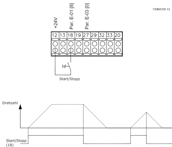
Abbildung 6.1 Klemme 37: Nur verfügbar mit Sicherer Stopp-Funktion!
