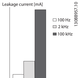
Abbildung 2.18 Prinzipschaubild zeigt Beeinflussung der Ansprech-/Messgrößen durch die Trennfrequenz des Fehlerstromschutzschalters.
