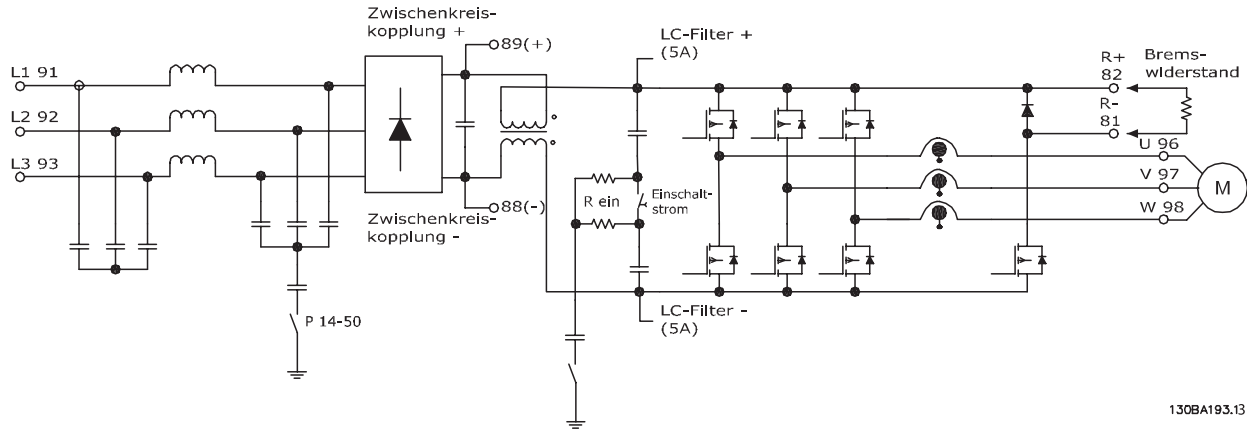
Abbildung 2.9 Regelungsstrukturen.
