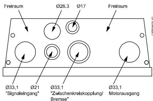
Abbildung 5.8 Kabeleingänge für Gehäuse B1. Die vorgeschlagenen Verwendungszwecke der Bohrungen sind reine Empfehlungen; andere Lösungen können ebenfalls umgesetzt werden.
