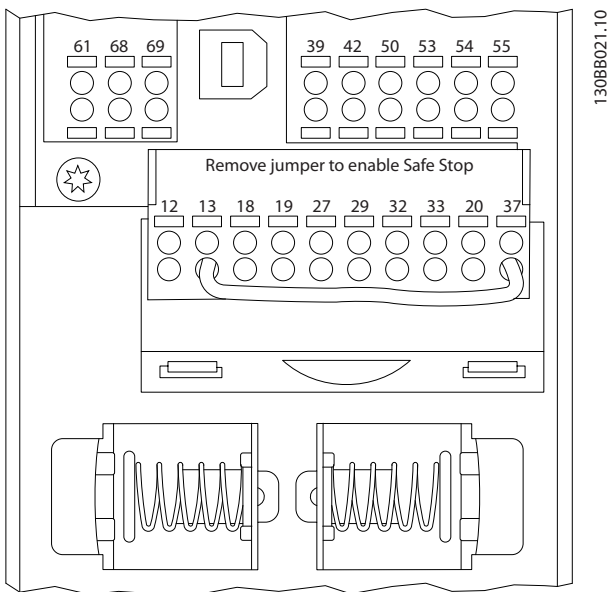
Abbildung 7.2 Steuerkartenklemmen
