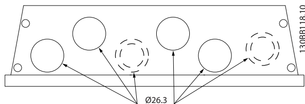
Abbildung 5.7 Kabeleingänge für Gehäuse A5. Die vorgeschlagenen Verwendungszwecke der Löcher sind reine Empfehlungen und es sind andere Lösungen möglich.
