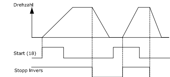
Abbildung 6.2 Klemme 37: Nur verfügbar mit Sicherer Stopp-Funktion
