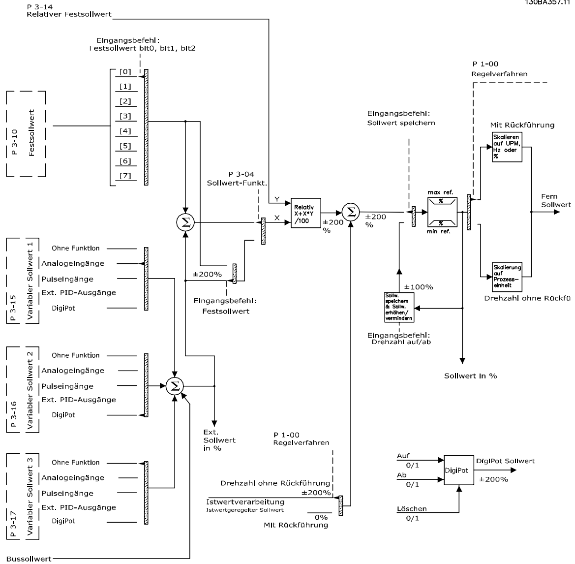
Abbildung 2.13 Blockschaubild mit Fernsollwert
