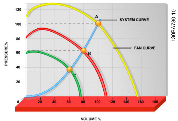
Abbildung 2.4 Die Grafik zeigt Lüfterkurven (A, B und C) für reduzierte Lüftervolumen.
