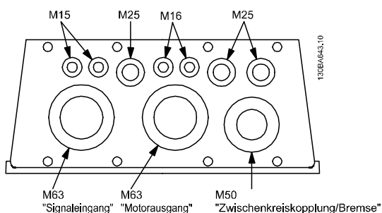
Abbildung 5.12 Kabeleingänge für Gehäuse C1. Die vorgeschlagenen Verwendungszwecke der Bohrungen sind reine Empfehlungen; andere Lösungen können ebenfalls umgesetzt werden.
