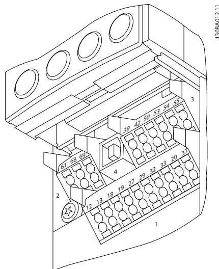
Abbildung 5.21 Steuerklemmen (alle Gehäuse)
