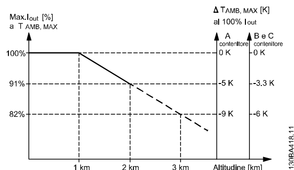
Disegno 8.2 Declassamento della corrente di uscita rispetto all'altitudine, con T_{AMB, MAX} per dimensioni telaio A, B e C. Per altitudini superiori ai 2 km, contattare Danfoss per informazioni sulle caratteristiche PELV.
