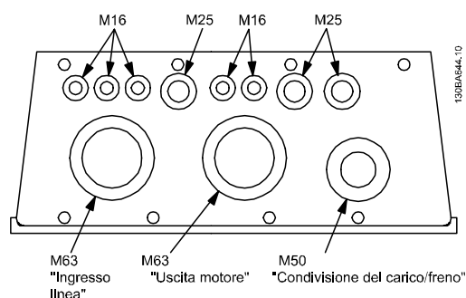
Disegno 5.13 Fori di ingresso dei cavi per custodia C2. La soluzione proposta per l'uso dei fori di ingresso è solo a titolo di esempio; sono possibili anche altre soluzioni.
