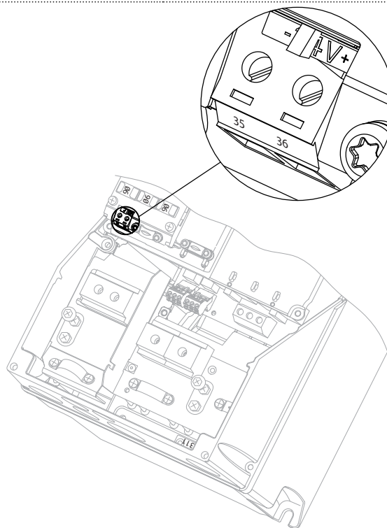
Disegno 3.5 Collegamento all'alimentazione di backup 24 V (A5-C2).
