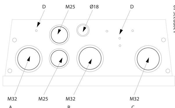
Disegno 5.9 Fori di ingresso dei cavi per custodia B1. La soluzione proposta per l'uso dei fori di ingresso è solo a titolo di esempio; sono possibili anche altre soluzioni.
