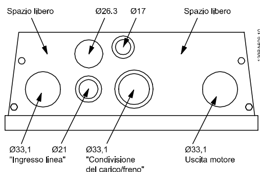
Disegno 5.8 Fori di ingresso dei cavi per custodia B1. La soluzione proposta per l'uso dei fori di ingresso è solo a titolo di esempio; sono possibili anche altre soluzioni.
