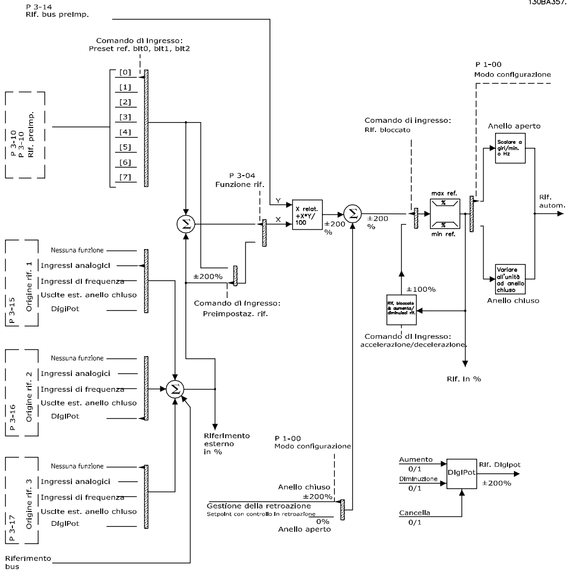
Disegno 2.13 Diagramma riferimento remoto o locale
