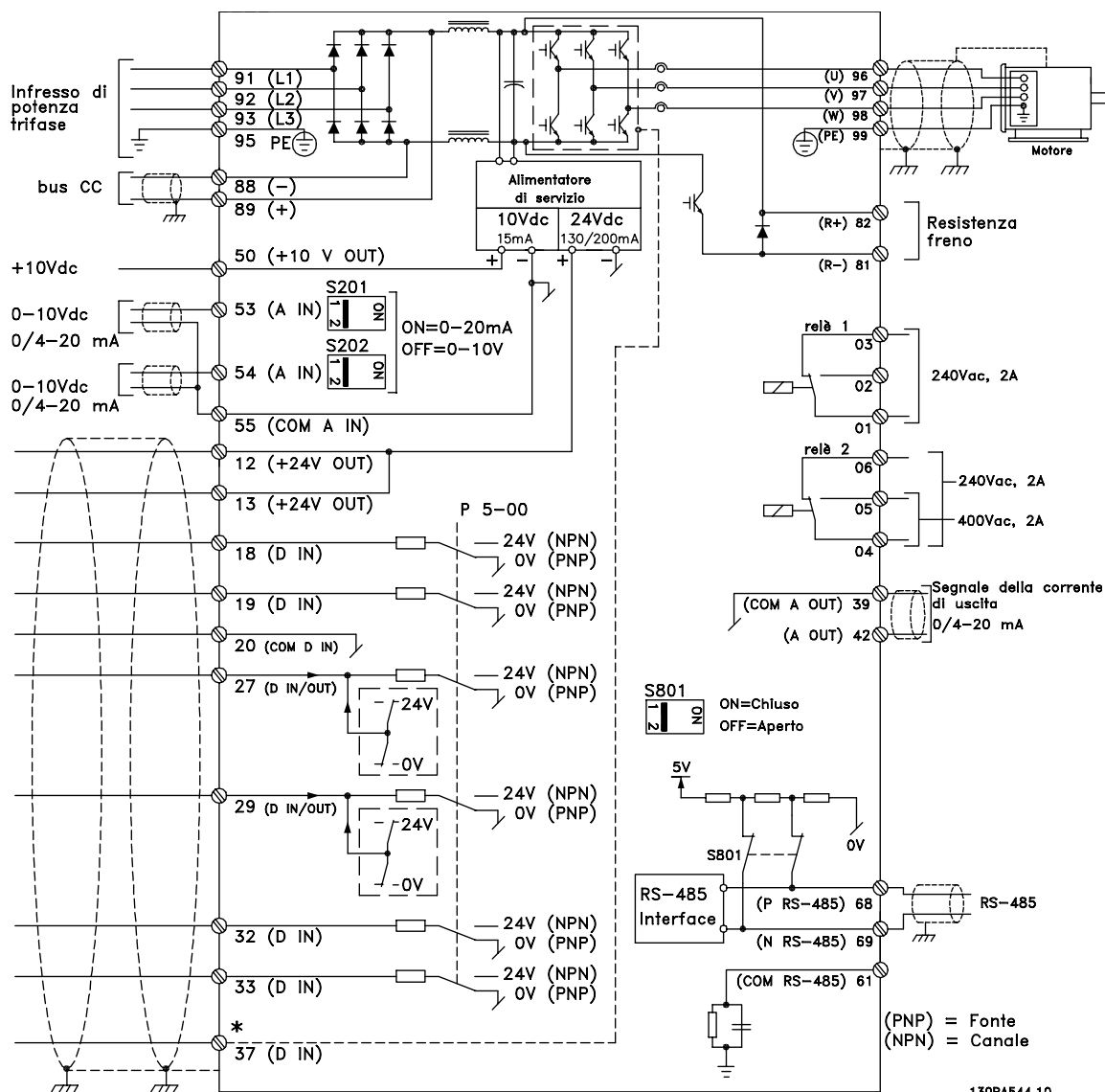
Disegno 5.23 Grafico mostrante tutti i morsetti elettrici.
