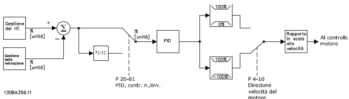
Disegno 2.11 Diagramma a blocchi del controllore ad anello chiuso
