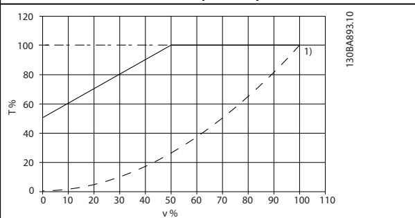
Carico massimo per un motore standard a 40 °C pilotato da un convertitore di frequenza tipo VLT FCxxx
