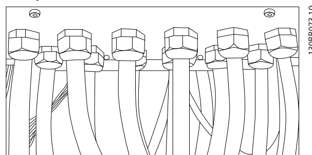
Disegno 5.14 Esempio di corretta installazione della piastra passacavi.
