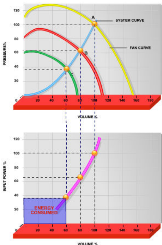
Disegno 2.5 Quando si utilizza un convertitore di frequenza per ridurre la capacità della ventola al 60 %, in certe applicazioni si può ottenere oltre il 50% di risparmio energetico.
