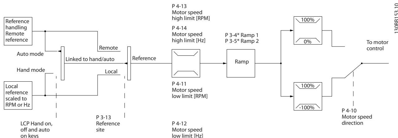
Disegno 2.10 Anello aperto
