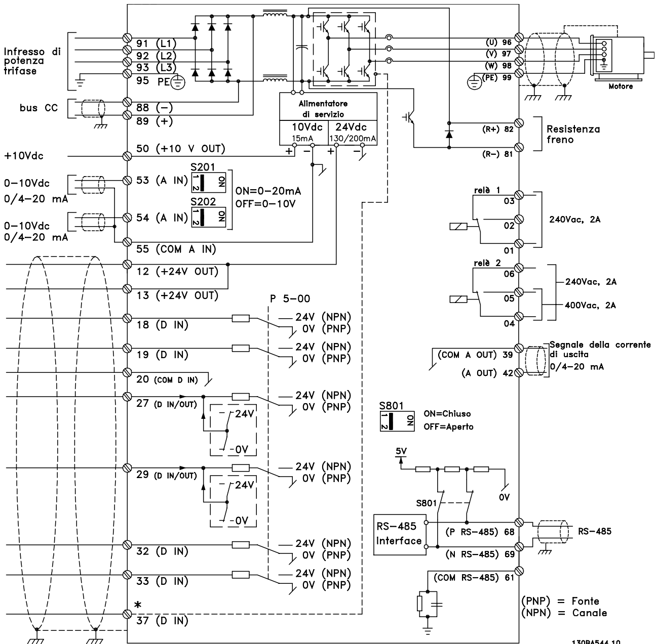
Disegno 5.6 Grafico mostrante tutti i morsetti elettrici. (Il morsetto 37 è solo presente per unità con funzione di arresto di sicurezza).
