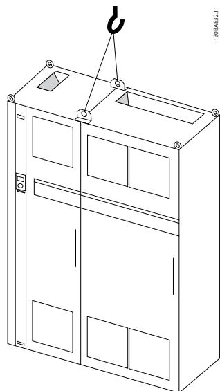
Disegno 5.2 Metodo consigliato per il sollevamento, dimensioni telaio F1 (460V, da 600 a 900 HP, 575/690 V, da 900 a 1150 HP).
