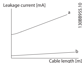
Disegno 2.15 Il disegno principale mostra come la corrente di dispersione viene influenzata dalla lunghezza del cavo e dalla taglia di potenza. P_a > P_b .
