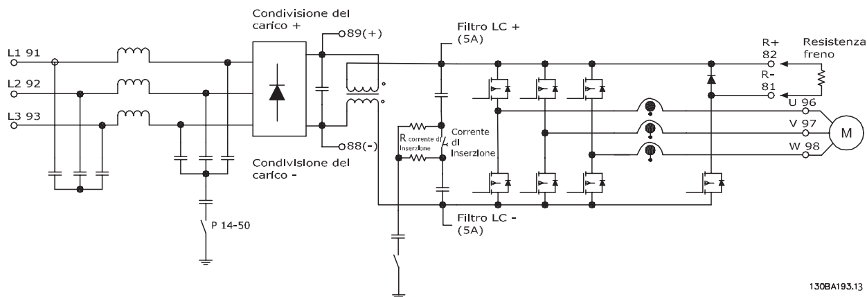
Disegno 2.9 Strutture di comando
