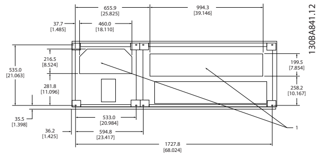
Disegno 5.18 Dimensioni telaio F2
