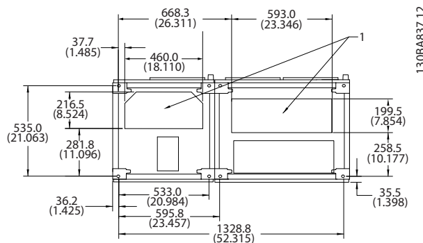
Disegno 5.17 Dimensioni telaio F1
