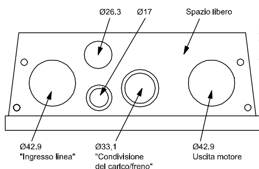
Disegno 5.10 Fori di ingresso dei cavi custodia B2. La soluzione proposta per l'uso dei fori di ingresso è solo a titolo di esempio; sono possibili anche altre soluzioni.
