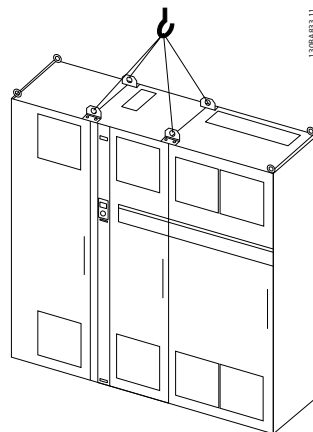
Disegno 5.4 Metodo consigliato per il sollevamento, dimensione di telaio (460 V, da 600 a 900 HP, 575/690 V, da 900 a 1150 HP).
