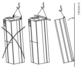
Disegno 5.1 Metodo consigliato per il sollevamento, dimensioni telaio D e E .
