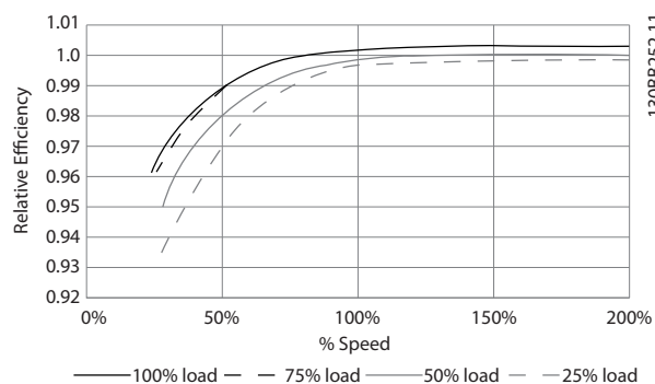
Disegno 8.1 Curve di rendimento tipiche
