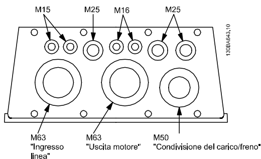
Disegno 5.12 Fori di ingresso dei cavi per custodia C1. La soluzione proposta per l'uso dei fori di ingresso è solo a titolo di esempio; sono possibili anche altre soluzioni.
