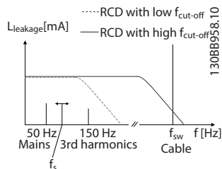
Disegno 2.17 Abbozzo dei contributi principali alla corrente di dispersione.
