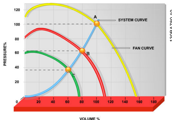
Disegno 2.4 Il grafico mostra le curve della ventola (A, B e C) per portate ridotte della ventola.
