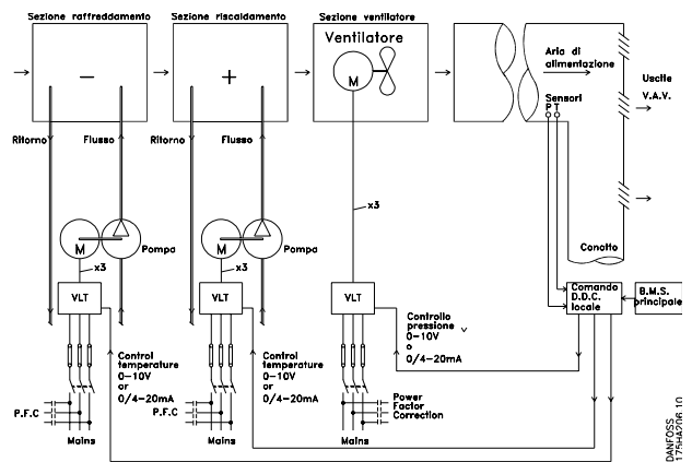
Disegno 2.8 La figura mostra un sistema di ventilazione controllato da convertitori di frequenza.
