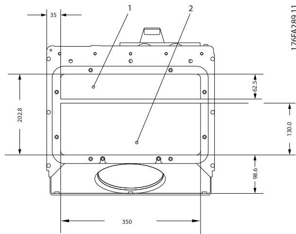
Disegno 5.15 Dimensioni telaio D1 + D2
