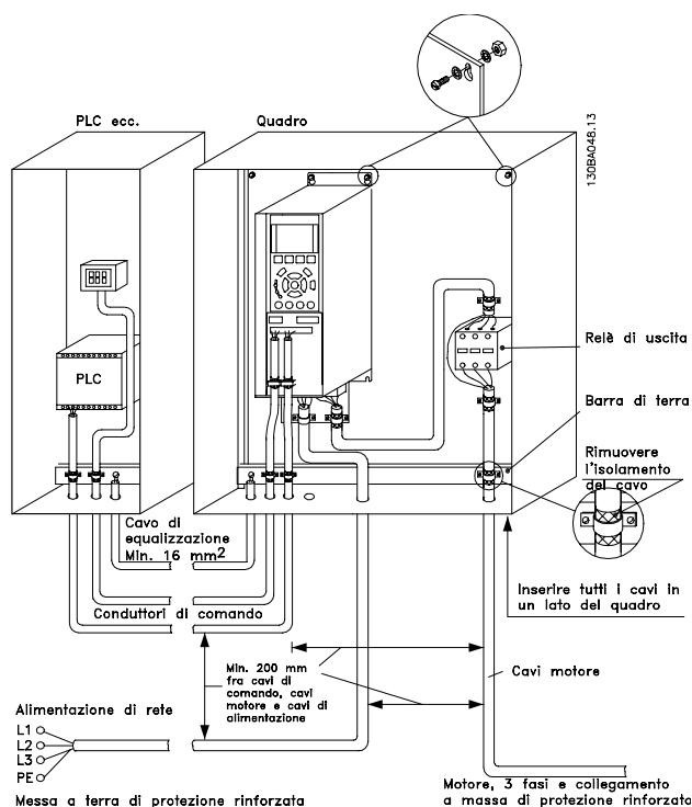
Disegno 5.25 Installazione elettrica nell'armadio conforme ai requisiti EMC di un Convertitore di frequenza.
