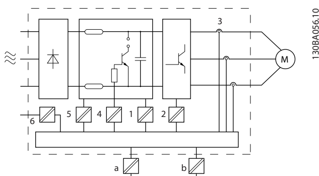
Disegno 2.14 Isolamento galvanico
