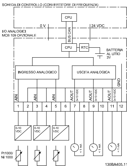
Disegno 3.6 Diagramma di principio per I/O analogici montati nel convertitore di frequenza.
