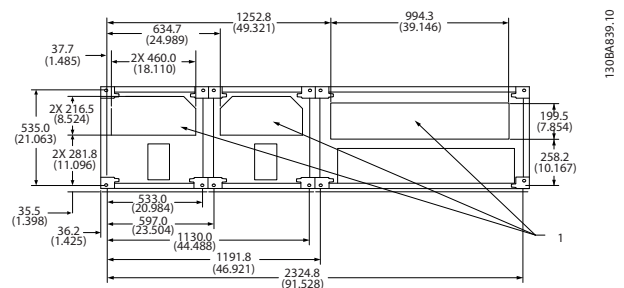
Disegno 5.20 Dimensioni telaio F4
