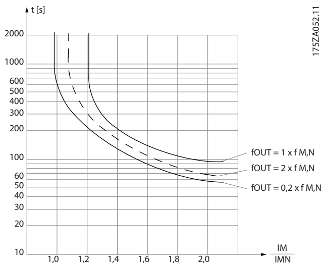
Disegno 2.19 L'asse X mostra il rapporto tra I_{motor} e I_{motor} nominale. L'asse Y riporta il tempo in secondi che precede il momento in cui l'ETR scatta e scollega il convertitore di frequenza. Le curve illustrano la caratteristica ad una velocità doppia della velocità nominale e a una velocità pari a 0,2 volte la velocità nominale.
