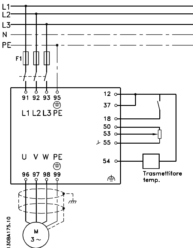
Disegno 5.26 Schema dei collegamenti elettrici.
