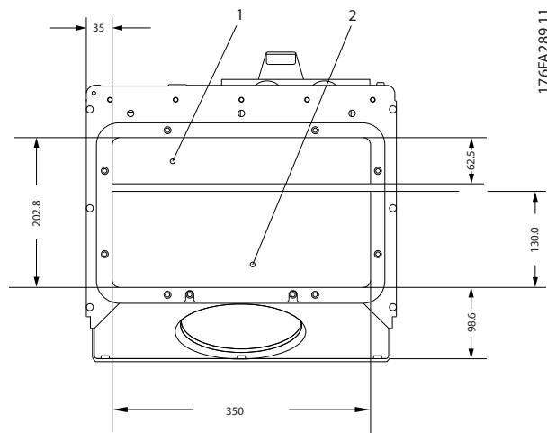
Disegno 5.16 Dimensioni telaio E1
