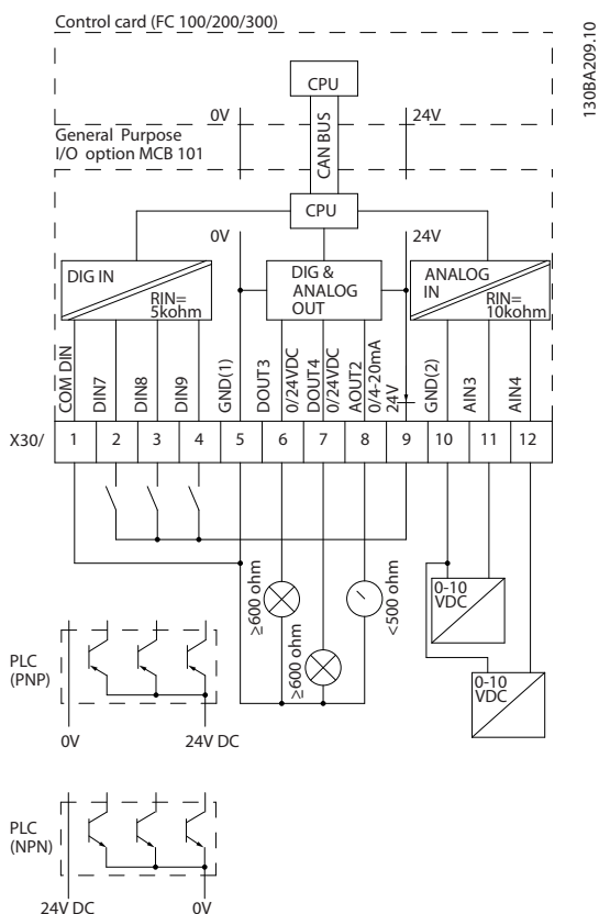
Disegno 3.3 Diagramma di principio
