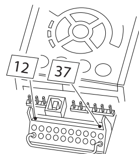
Disegno 2.2 Jumper tra il morsetto 37 e i 24 V CC
