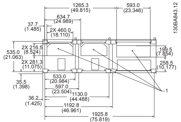
Disegno 5.19 Dimensioni telaio F3
