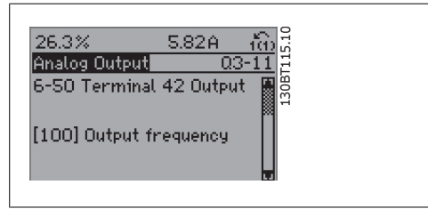
图 1.12: 步骤 6: 选择参数 6-50 端子 42 输出。按 [OK] (确定)。
