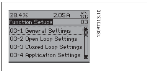
图 1.10: 步骤 4: 随即会显示功能设置选项。选择 Q3-1 一般设置。按 [OK] (确定)。
