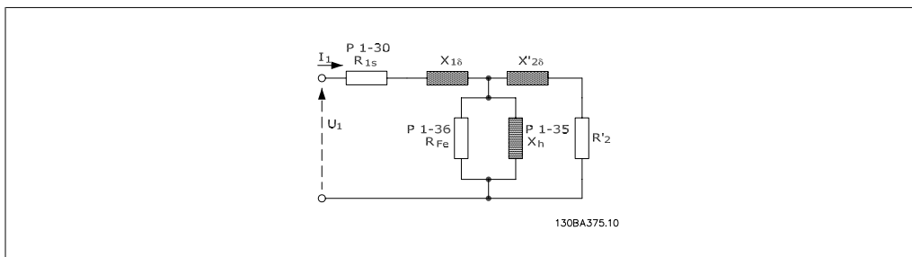
图 2.1: 异步电动机的电动机当量图
