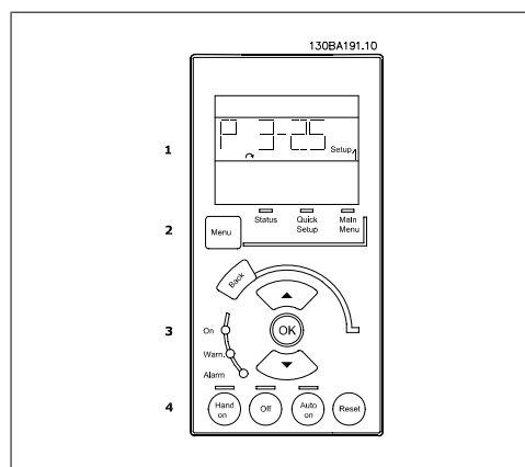
图 1.1: 数字式 LCP (NLCP)
