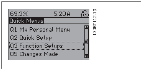
图 1.9: 步骤 3: 使用向上/向下导航键向下滚动到“功能设置”。按 [OK] (确定)。
