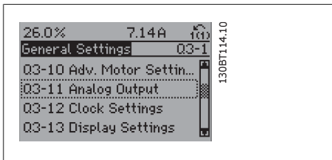
图 1.11: 步骤 5: 使用向上/向下导航键向下滚动到目标选项, 比如 Q3-11 模拟输出。按 [OK] (确定)。
