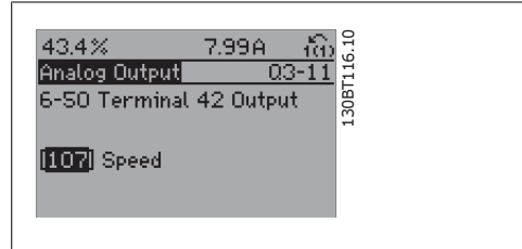
图 1.13: 步骤 7: 使用向上/向下导航键选择不同选项。按 [OK] (确定)。
