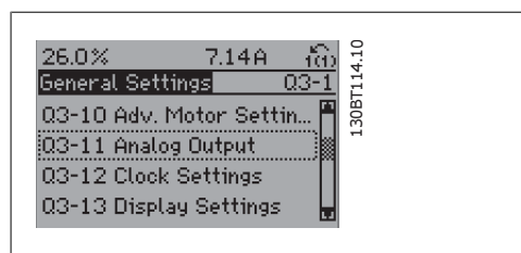
Ábra 1.11: 5. lépés: A felfelé/lefelé mutató nyíllal görgessen lefelé a Q3-11 Analog kimenet pontra. Nyomja meg az [OK] gombot
