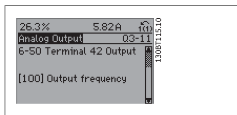
Ábra 1.12: 6. lépés: Válassza ki a 6-50-es, 42-es kimenet paramétert. Nyomja meg az [OK] gombot
