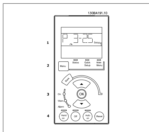
Ábra 1.1: Numerikus LCP (NLCP)
