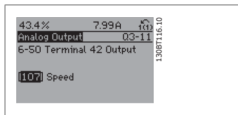
Ábra 1.13: 7. lépés: A különböző lehetőségek közül a felfelé/lefelé mutató nyíllal választhat. Nyomja meg az [OK] gombot
