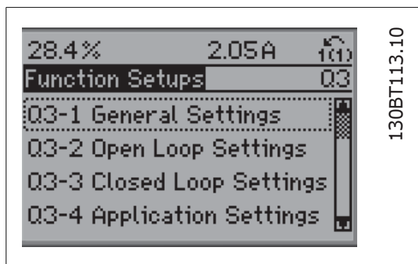
Illustration 2.10: Étape 4 : les choix de configuration des fonctions apparaissent. Choisir 03-1 Régl. généraux . Appuyer sur [OK].
