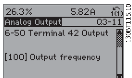
图 2.12: 步骤 6: 选择参数 6-50。按 [OK] (确定)。
