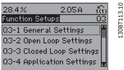
图 2.10: 步骤 4: 随即会显示功能设置选项。选择 03-1 一般设置。按 [OK] (确定)。
