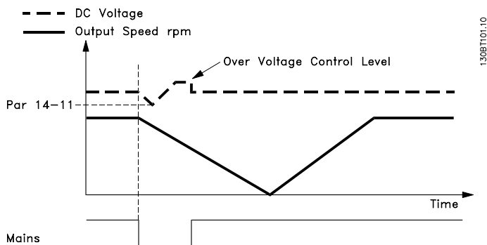
图 3.2: 受控减速—主电源短时间故障。 减速直到停止, 接着减速到参考值。
