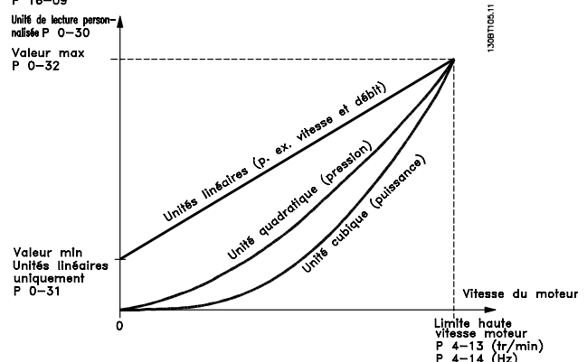
Lecture personnalisée (valeur) P 16-09
