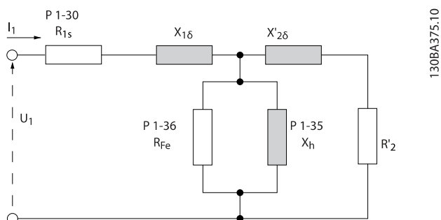
Illustration 3.1: Diagramme d'équivalence moteur pour un moteur asynchrone
