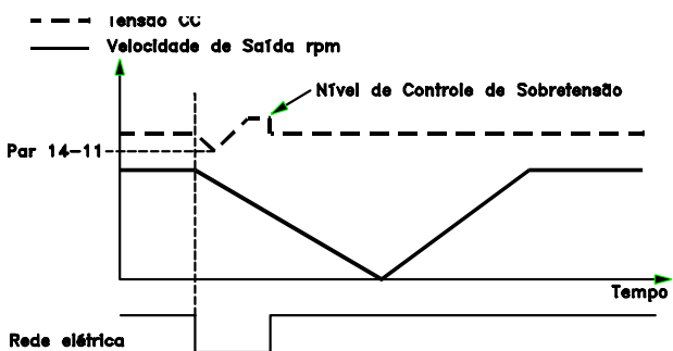
Ilustração 3.2: Desaceleração Controlada - falha de curta duração da rede elétrica. Desaceleração para parada seguida por aceleração até a referência.
