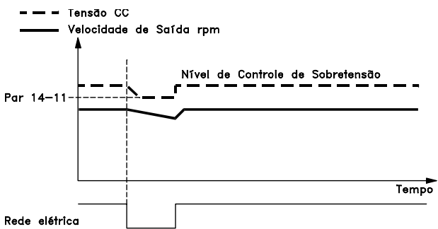
Ilustração 3.4: Back-up Cinético, falha de curta duração da rede elétrica. Prossiga enquanto a energia no sistema permiti-lo.
